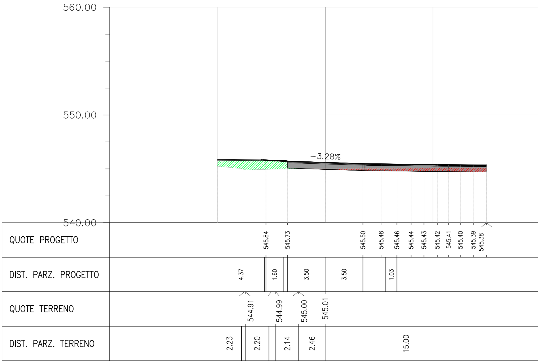
Rotatoria - SEZ. R1 - PROGRESSIVA 0+000.00
