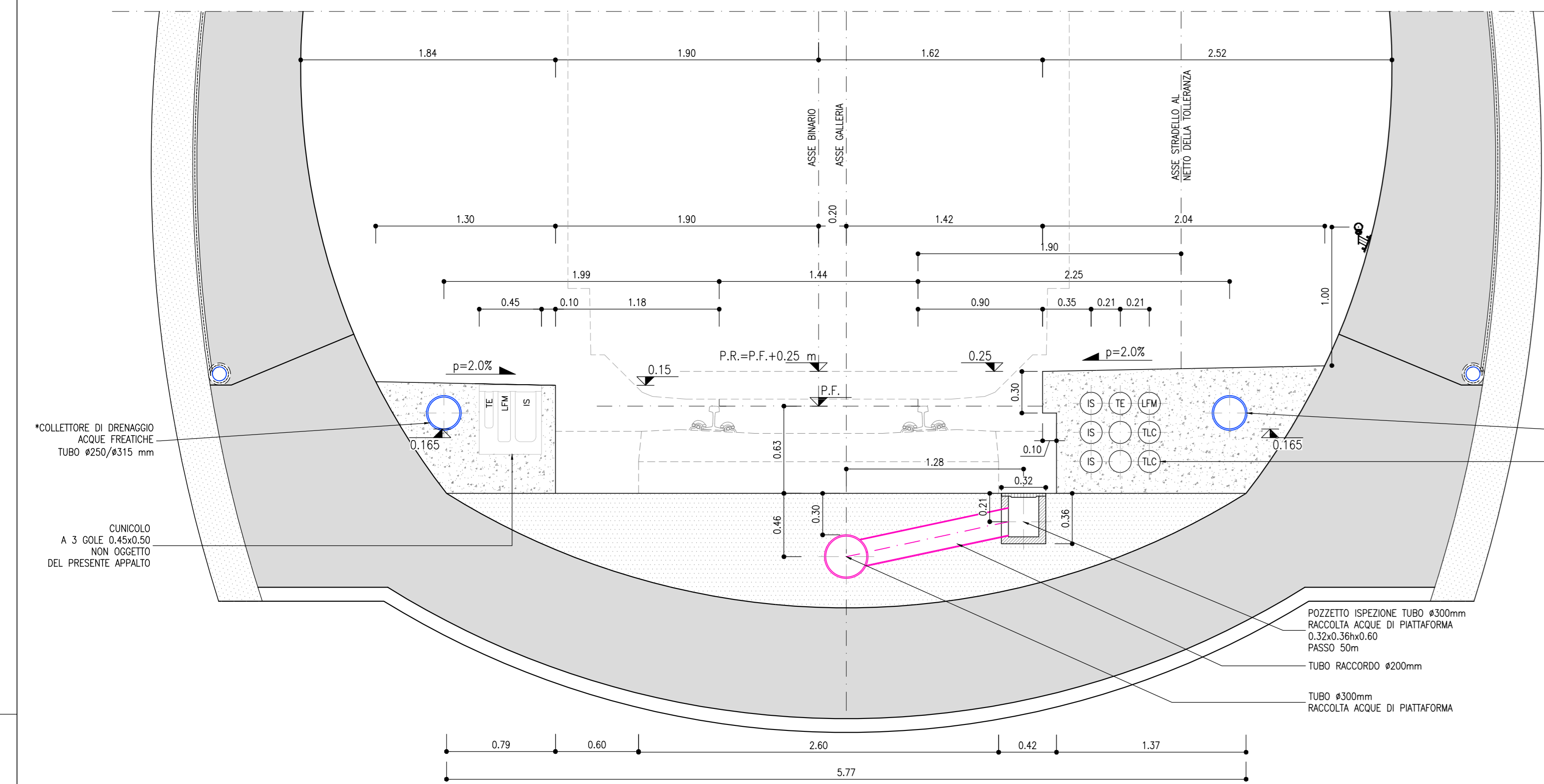
SEZIONE IN RETTA IN CORRISPONDENZA DEL POZZETTO DI ISPEZIONE ACQUE DI PIATTAFORMA SCALA 1:25
