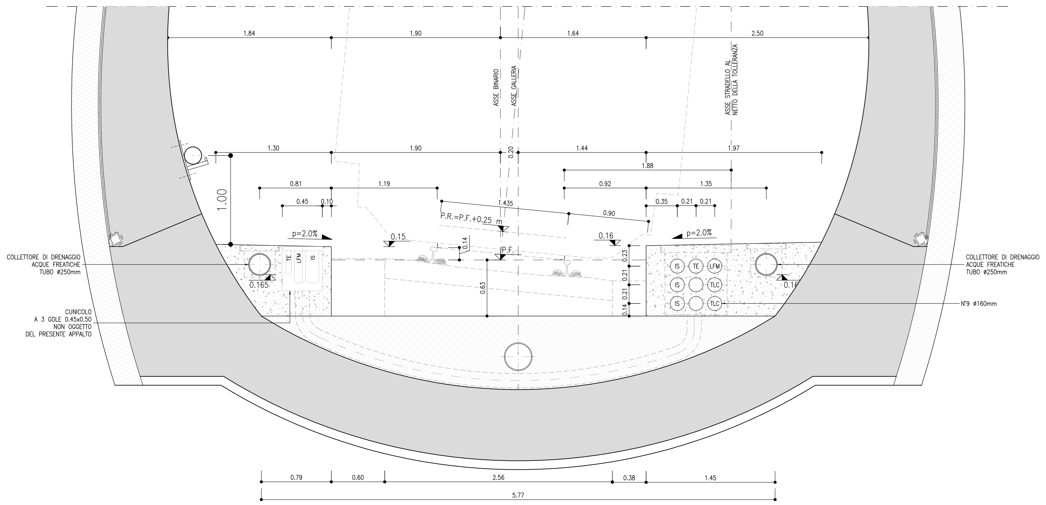
SEZIONE IN CURVA IN DX (STRADELLO INTERNO, SOPRAELEVAZIONE 140mm) SCALA 1:25
