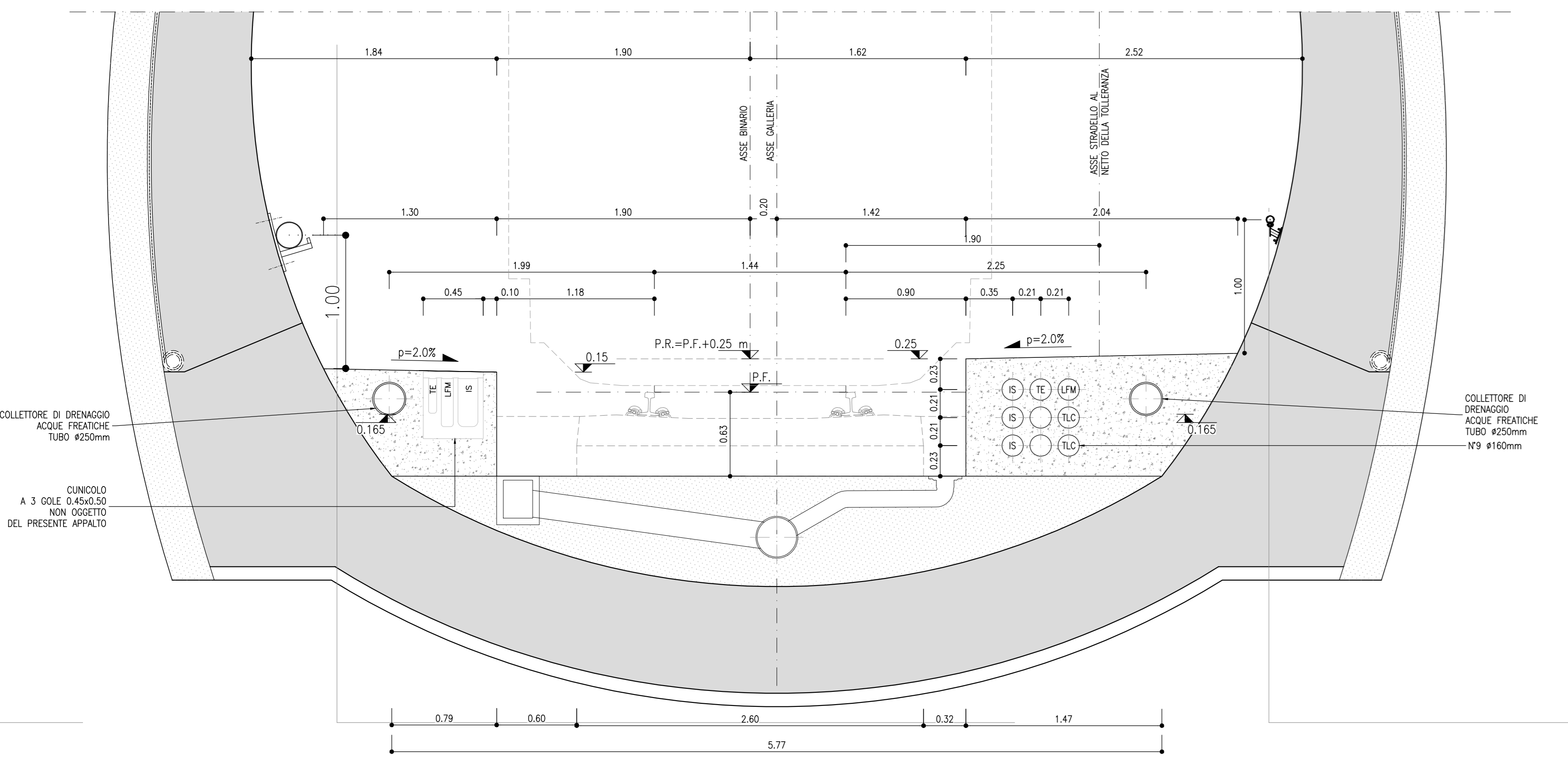
SEZIONE IN RETTA IN CORRISPONDENZA DEL TUBO DI ADDUZIONE ACQUE DI PIATTAFORMA SCALA 1:25
