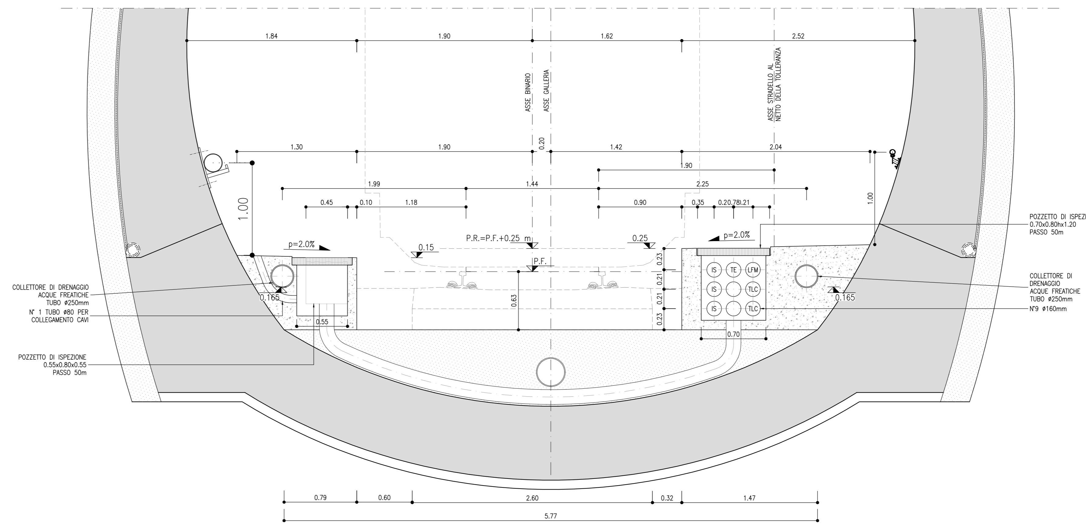
SEZIONE IN RETTA IN CORRISPONDENZA DEL SOTTOATTRAVERSAMENTO E DEL TUBO DI COLLEGAMENTO CANALINA PORTACAVI SCALA 1:25
