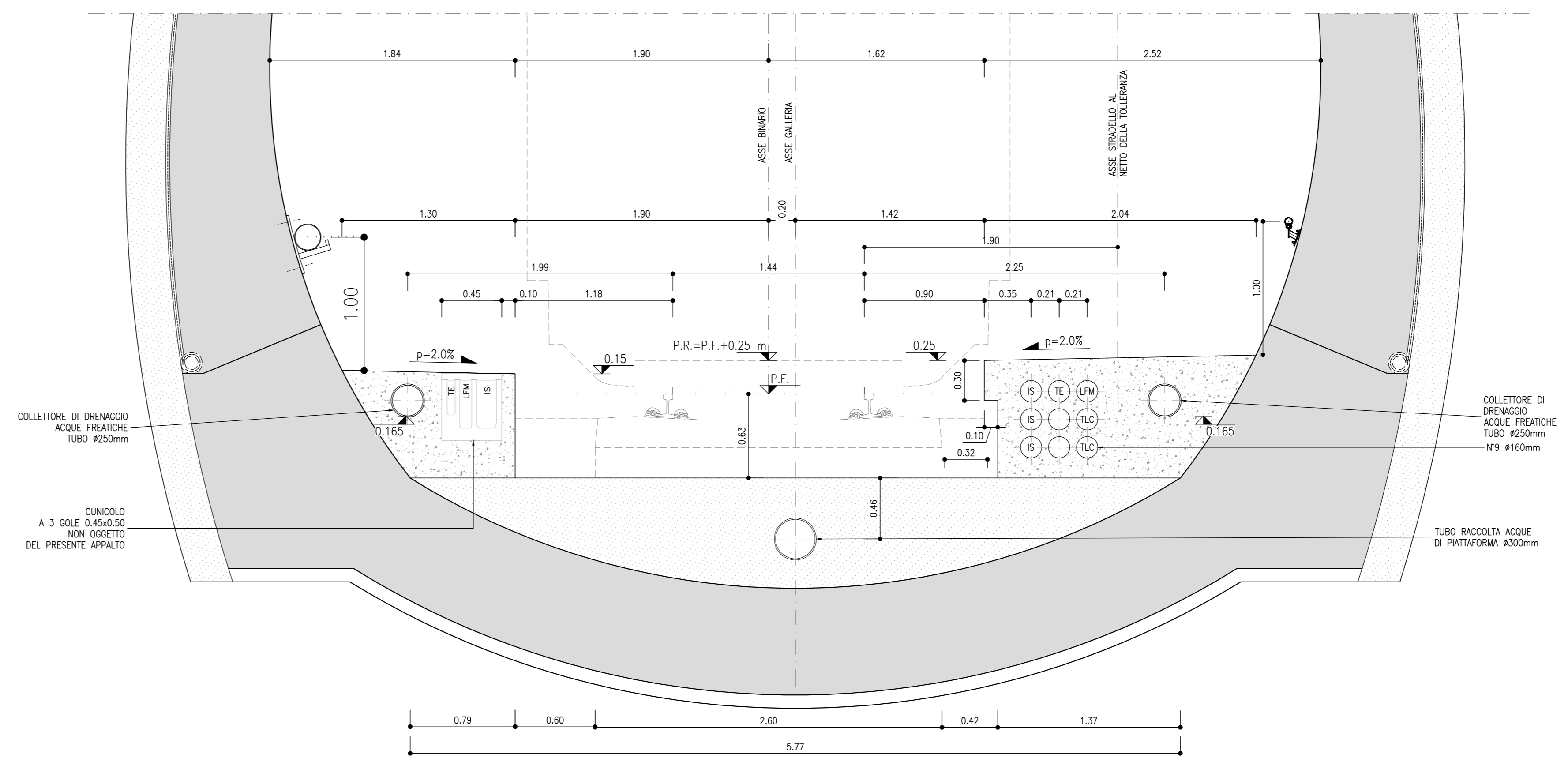
SEZIONE IN RETTA IN CORRISPONDENZA DEL POZZETTO DI ISPEZIONE ACQUE DI PIATTAFORMA SCALA 1:25
