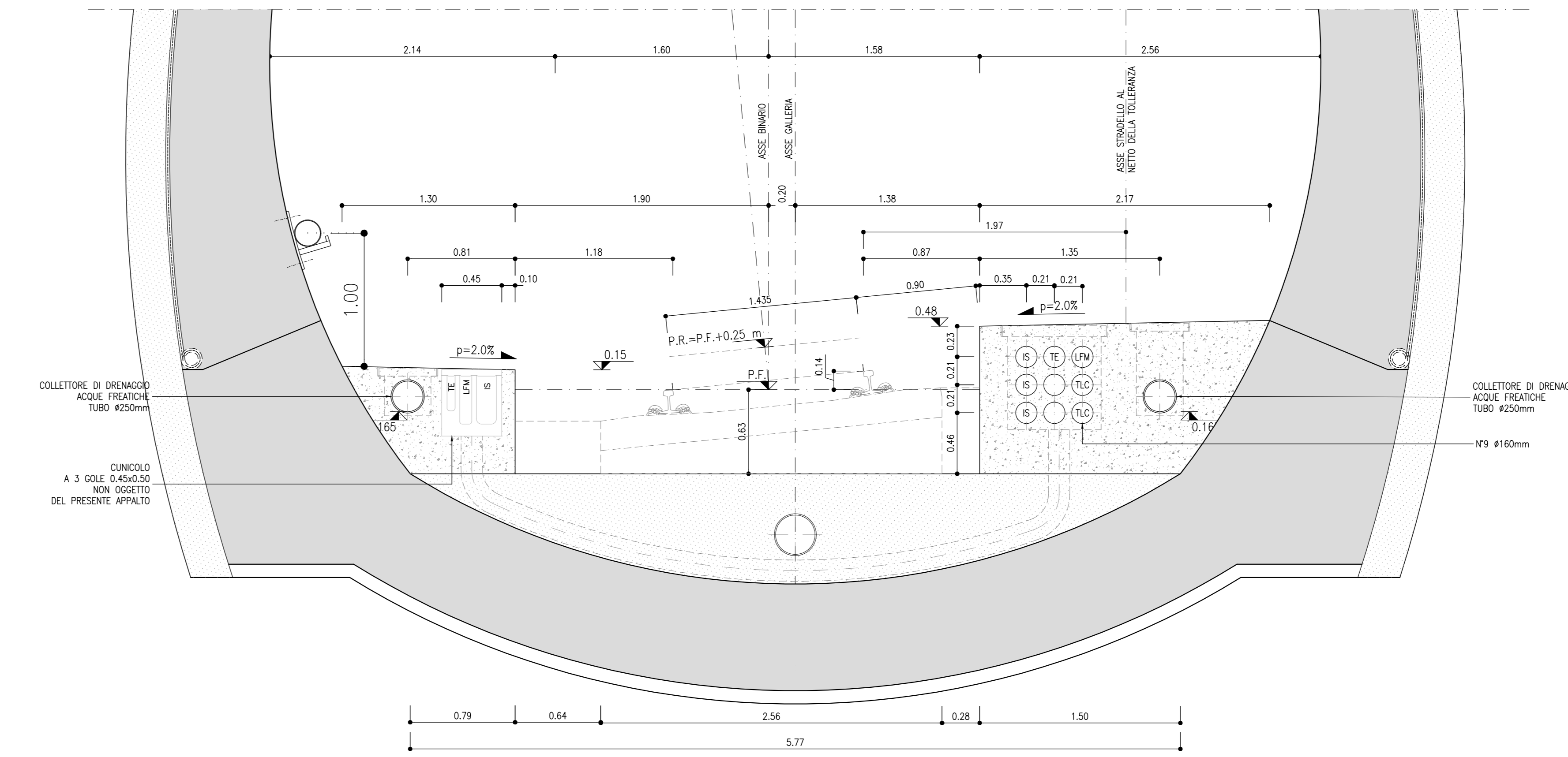
SEZIONE IN CURVA IN SX (STRADELLO ESTERNO, SOPRAELEVAZIONE 140mm) SCALA 1:25
