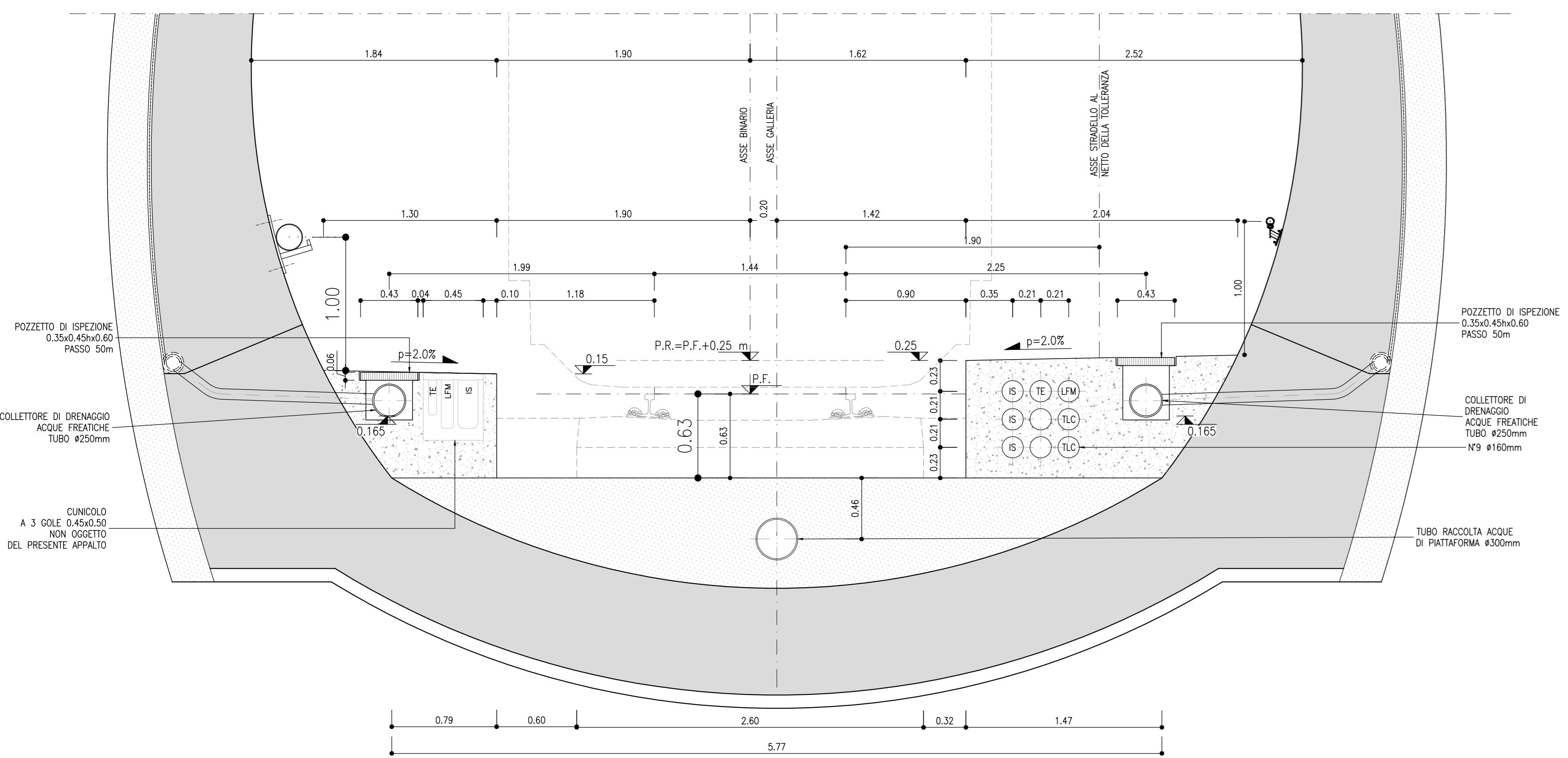
SEZIONE IN RETTA IN CORRISPONDENZA DEI POZZETTI DI ISPEZIONE DELLE ACQUE FREATICHE SCALA 1:25
