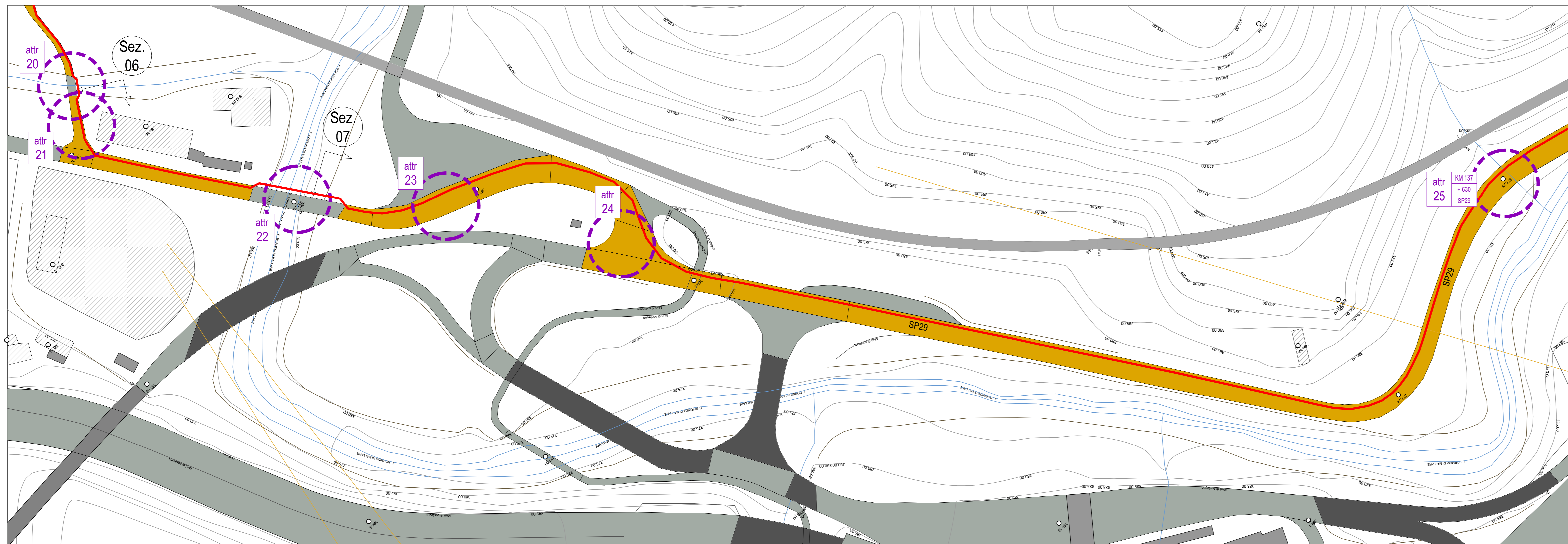
PLANIMETRIA DI INTERVENTO 04 base CTR - scala 1:1000
