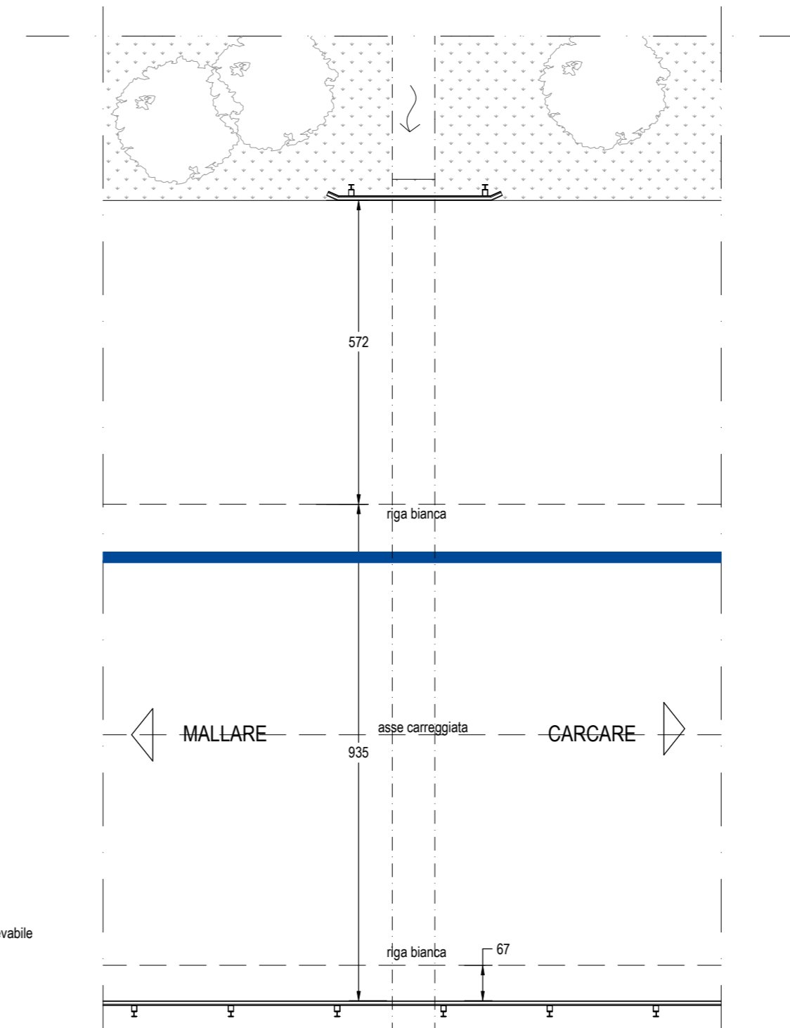
Planimetria generale attraversamento - 1:100
