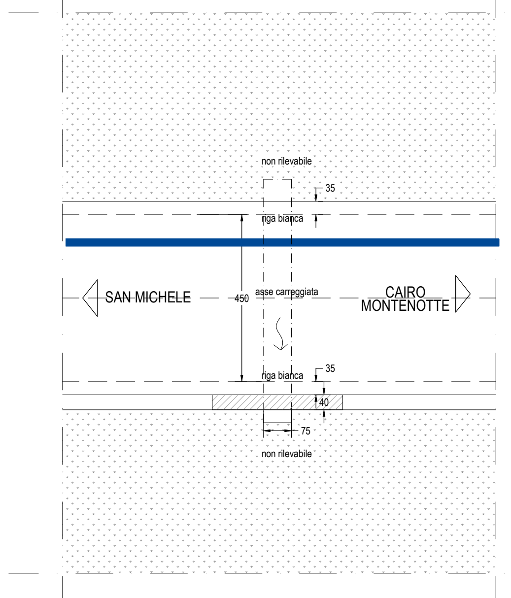
Planimetria generale attraversamento - 1:100
