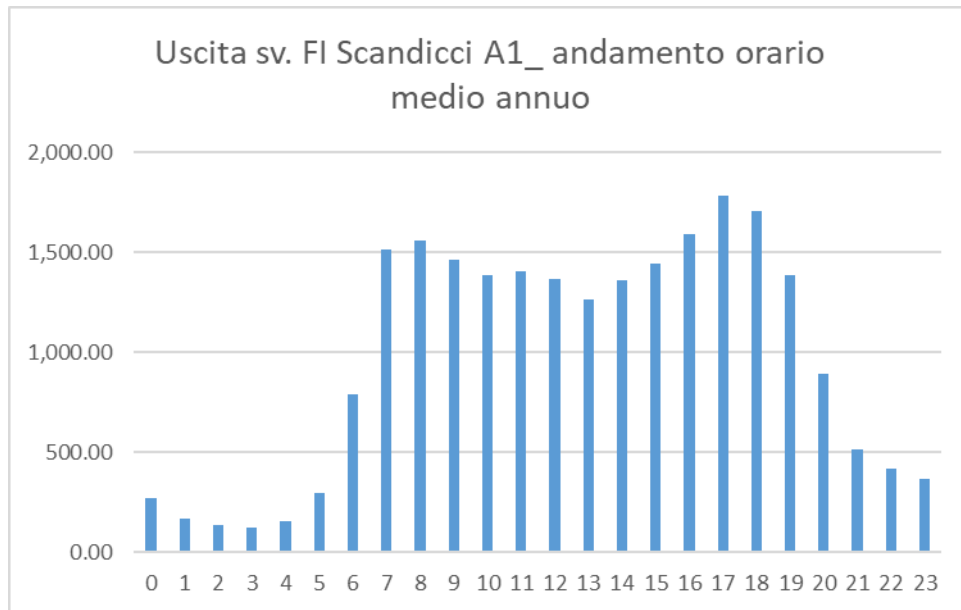
Figura 5-9 TGM annua svincolo Firenze Scandicci, veicoli in uscita
