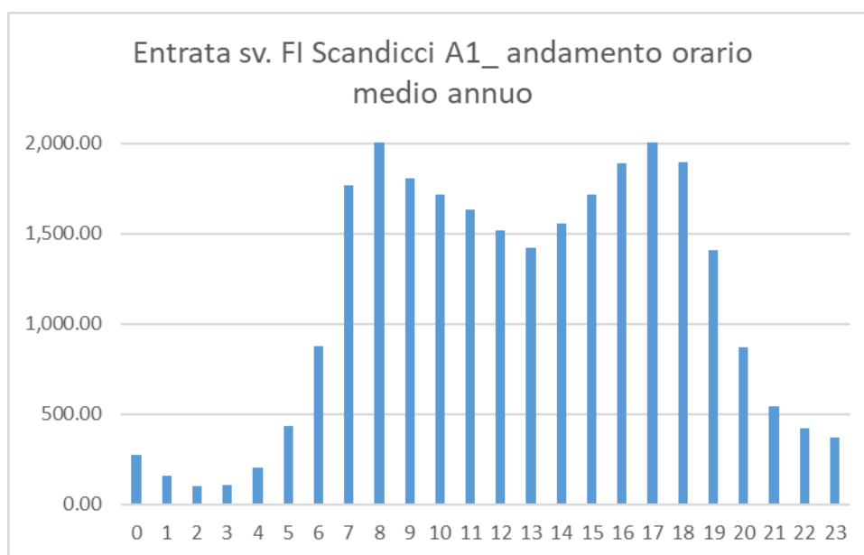
Figura 5-8 TGM annua svincolo Firenze Scandicci, veicoli in entrata
