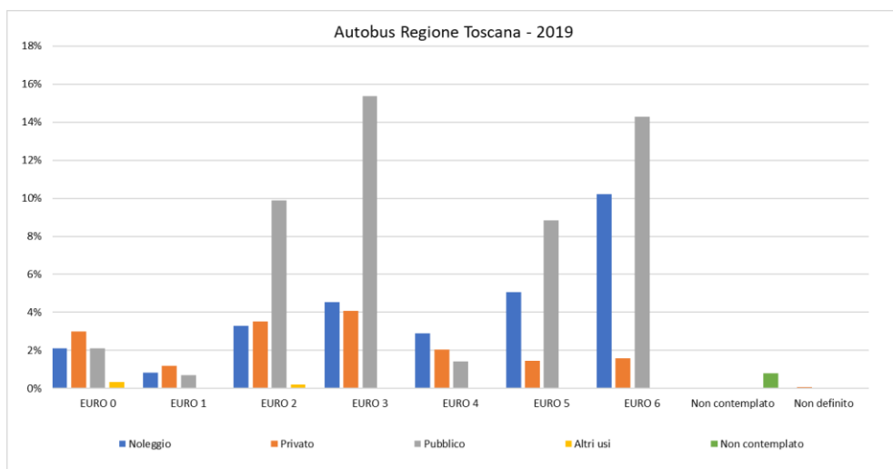
Figura 5-6: Suddivisione percentuale Autobus, Regione Toscana (fonte: Elaborazione da dati ACI Autoritratto 2019)
