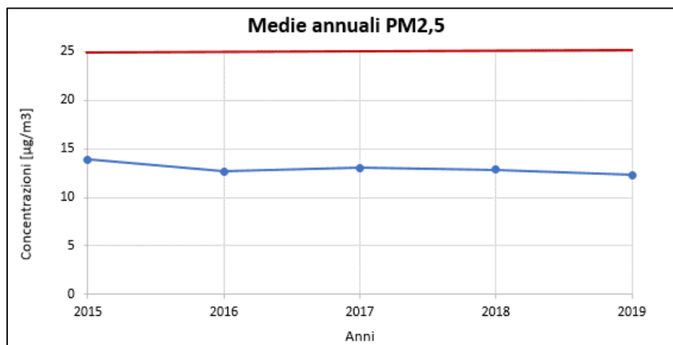
Figura 3-17 Medie annuali PM 2.5 - confronto con limite normativo (Fonte: elaborazione dati ARPA Toscana)
