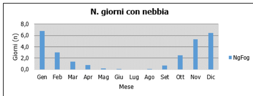
Figura 2-17 Numero di giorni medio al mese con presenza di nebbia (Fonte: elaborazione da dati Atlante Climatico AM)
