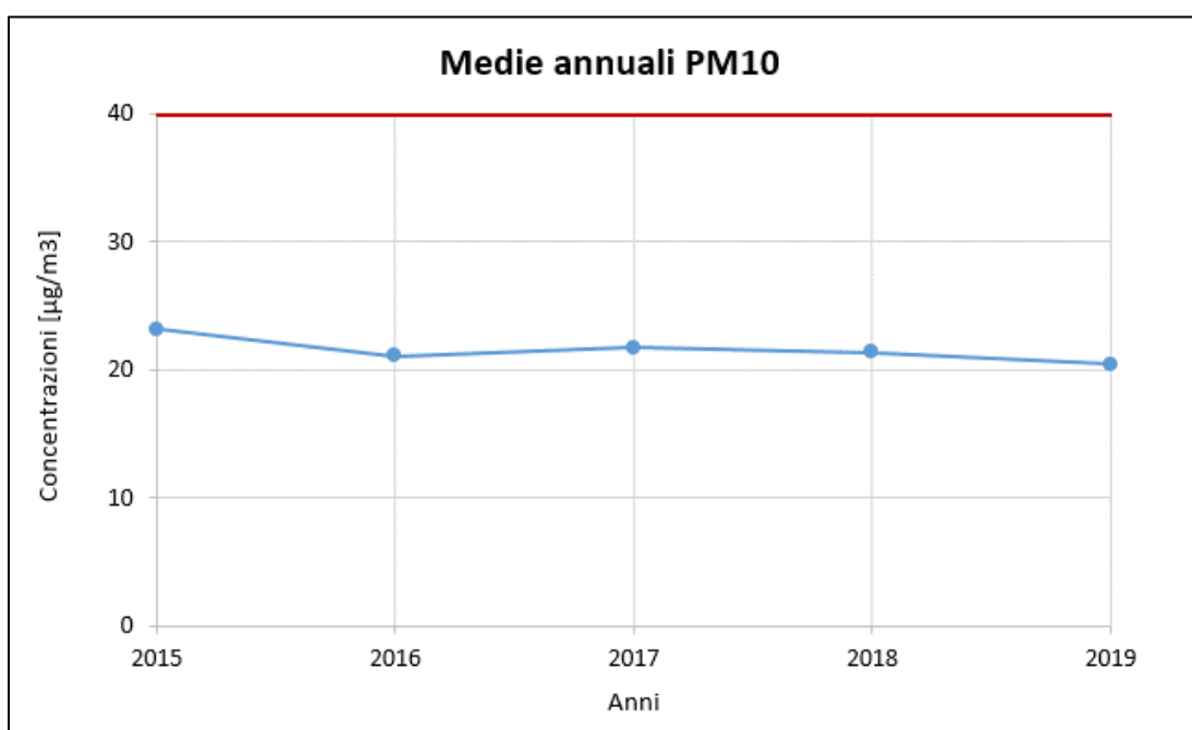
Figura 3-15 Medie annuali PM10- confronto con limite normativo (Fonte: elaborazione dati ARPA Toscana)
