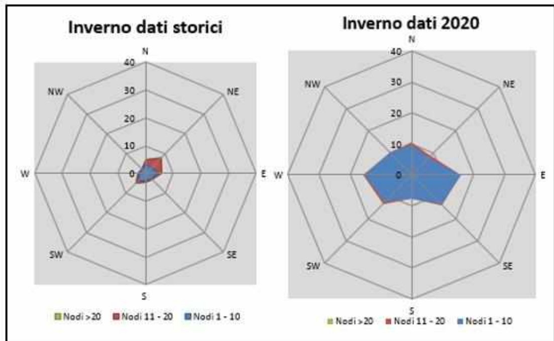
Figura 2-31 Confronto dati anemometrici stagione invernale (Fonte: elaborazione dati della Stazione di Firenze – Aeroporto Amerigo Vespucci)
