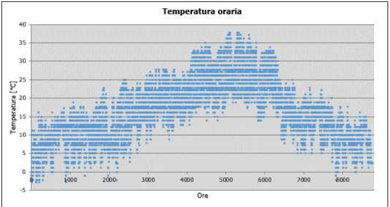
Figura 2-24 Temperatura oraria (Fonte: elaborazione dati della Stazione di Firenze – Aeroporto Amerigo Vespucci)
