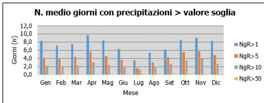
Figura 2-16 N° di giorni medio al mese con precipitazioni superiori a 1, 5, 10 e 50 mm di precipitazioni (Fonte: elaborazione da dati Atlante Climatico AM)
