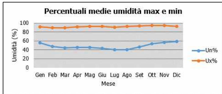
Figura 2-18 Media mensile dell'umidità percentuale massima e minima (Fonte: elaborazione da dati Atlante Climatico AM)
