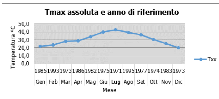
Figura 2-10 Temperatura massima assoluta ed anno di riferimento (Fonte: elaborazione da dati Atlante Climatico AM)
