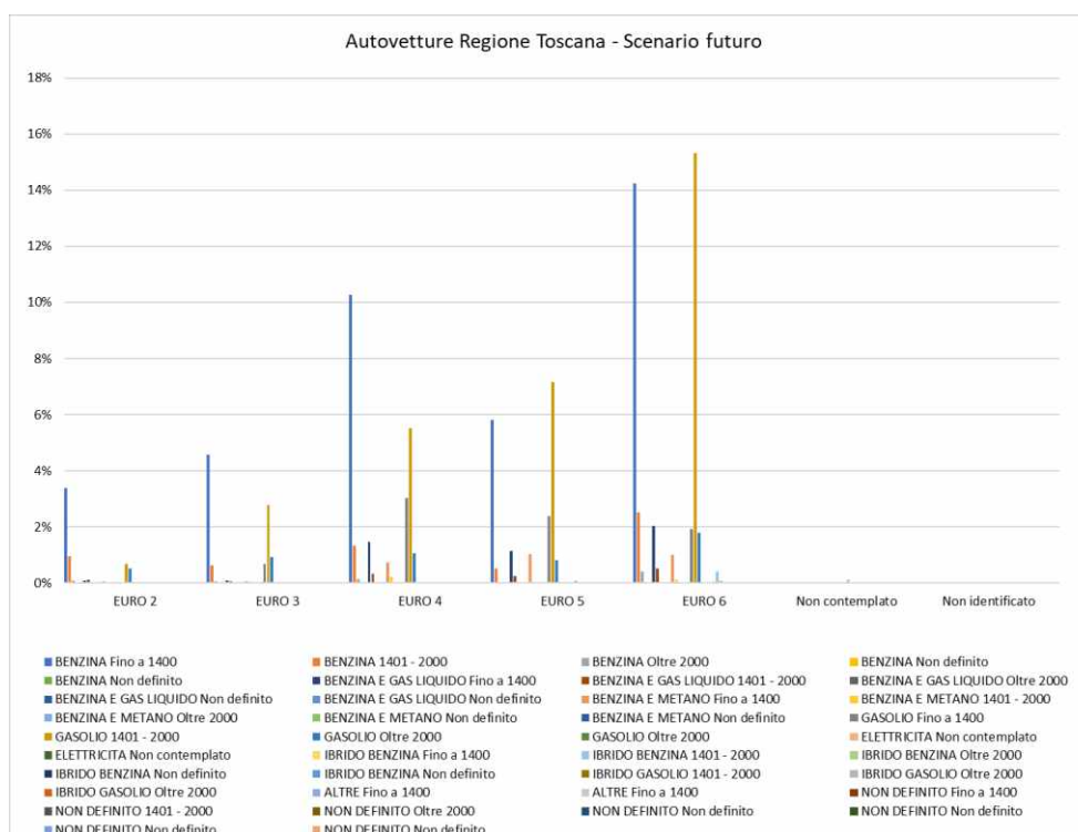
Figura 6-3: Suddivisione percentuale Autovetture, Regione Toscana (fonte: Elaborazione da dati ACI Autoritratto 2019)
