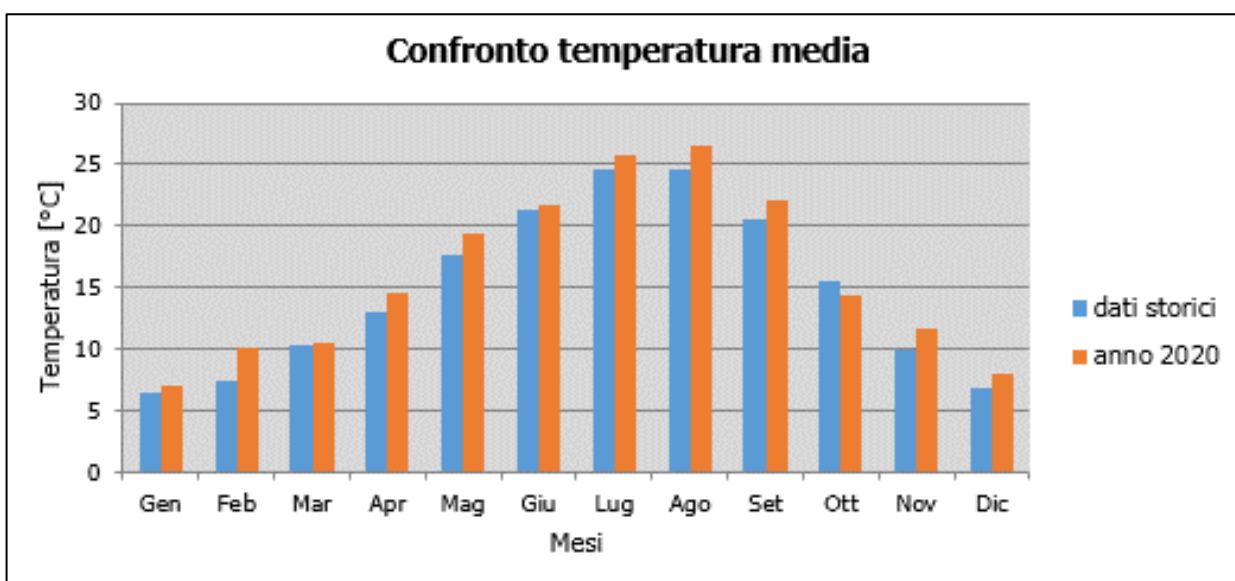
Figura 2-28 Confronto temperatura media (Fonte: elaborazione dati della Stazione di Firenze – Aeroporto Amerigo Vespucci)
