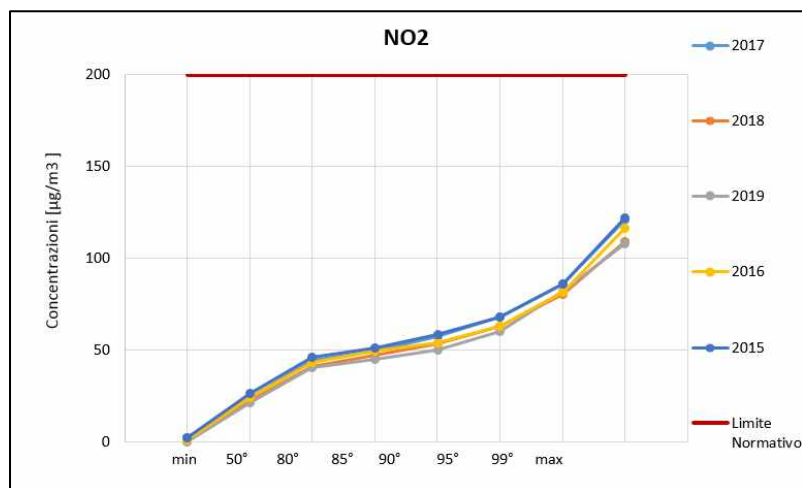
Figura 3-8 Percentili e valori massimi annuali NO2 (Fonte: elaborazione dati ARPA Toscana)
