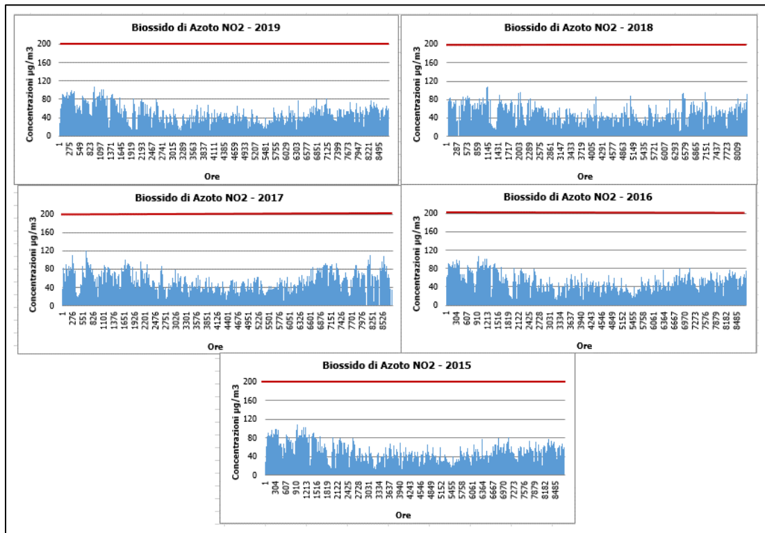
Figura 3-10 Valori orari di NO 2 anni 2015-2019 Centralina di Firenze - Scandicci (Fonte: elaborazione dati ARPA Toscana)
