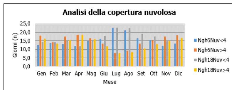
Figura 2-19 Analisi della copertura nuvolosa (Fonte: elaborazione da dati Atlante Climatico AM)
