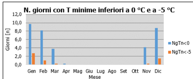
Figura 2-8 N° giorni con temperature minime inferiori a 0° e a -5° (Fonte: elaborazione da dati Atlante Climatico AM)
