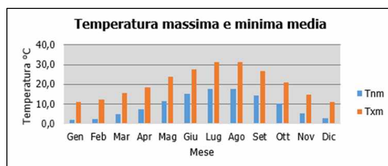
Figura 2-3 Temperatura massima e minima media nelle tre decadi di riferimento (Fonte: elaborazione da dati Atlante Climatico AM)
