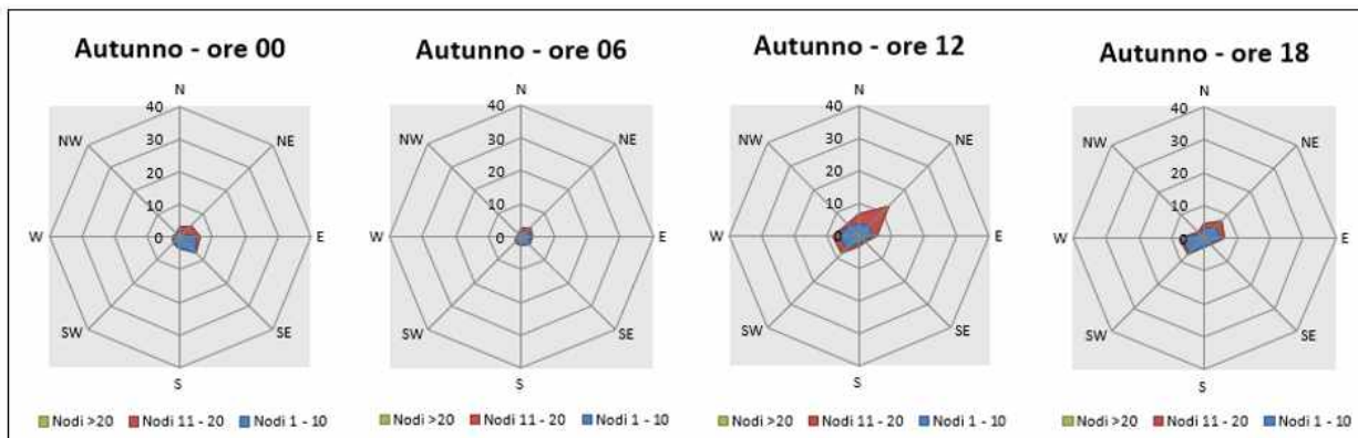
Figura 2-23 Regime anemometrico autunnale nelle 4 ore di riferimento (Fonte: elaborazione da dati Atlante Climatico)
