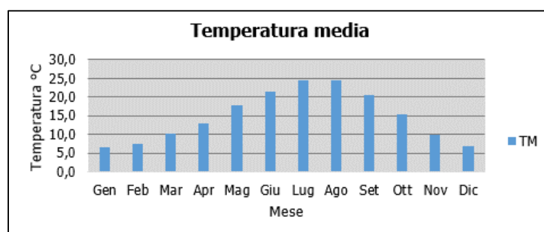
Figura 2-2 Temperatura media nelle tre decadi di riferimento (Fonte: elaborazione da dati Atlante Climatico AM)
