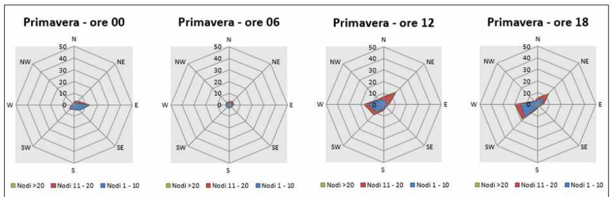
Figura 2-21 Regime anemometrico primaverile nelle 4 ore di riferimento (Fonte: elaborazione da dati Atlante Climatico)
