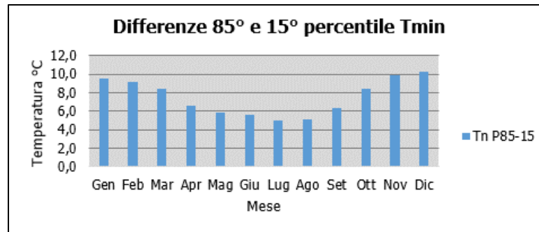
Figura 2-7 Differenza 85 – 15 percentile temperatura minima (Fonte: elaborazione da dati Atlante Climatico AM)
