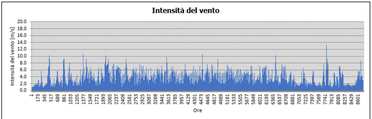
Figura 2-25 Intensità del vento (fonte: elaborazione dati della Stazione di Firenze – Aeroporto Amerigo Vespucci)
