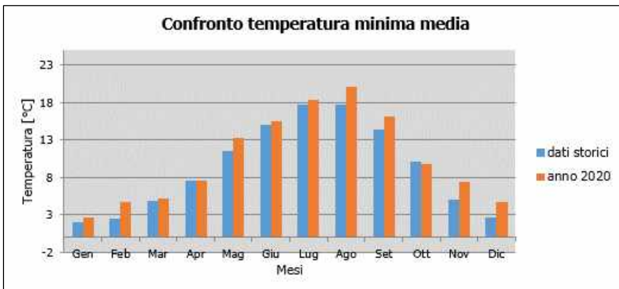
Figura 2-30 Confronto temperatura minima media (Fonte elaborazione dati della Stazione di Firenze – Aeroporto Amerigo Vespucci)
