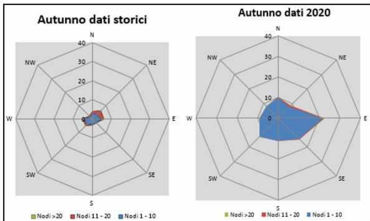
Figura 2-34 Confronto dati anemometrici stagione autunnale (Fonte: elaborazione dati della Stazione di Firenze – Aeroporto Amerigo Vespucci)
