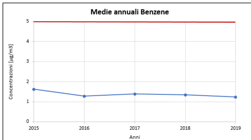
Figura 3-18 Medie annuali C6H6 -confronto con limite normativo (Fonte: elaborazione dati ARPA Toscana)
