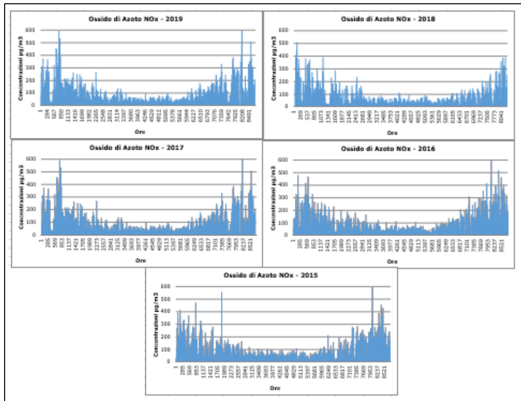
Figura 3-7 Valori orari di NOx anni 2015-2019 Centralina di Firenze – Scandicci (Fonte: elaborazione dati ARPA Toscana)
