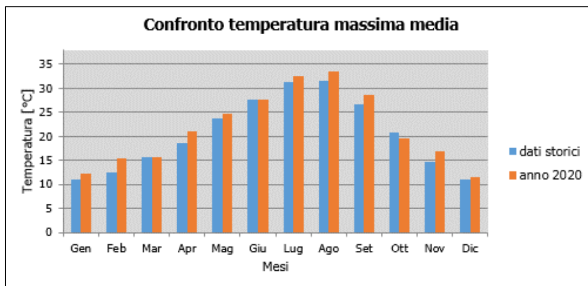
Figura 2-29 Confronto temperatura massima media (Fonte: elaborazione dati della Stazione di Firenze – Aeroporto Amerigo Vespucci)
