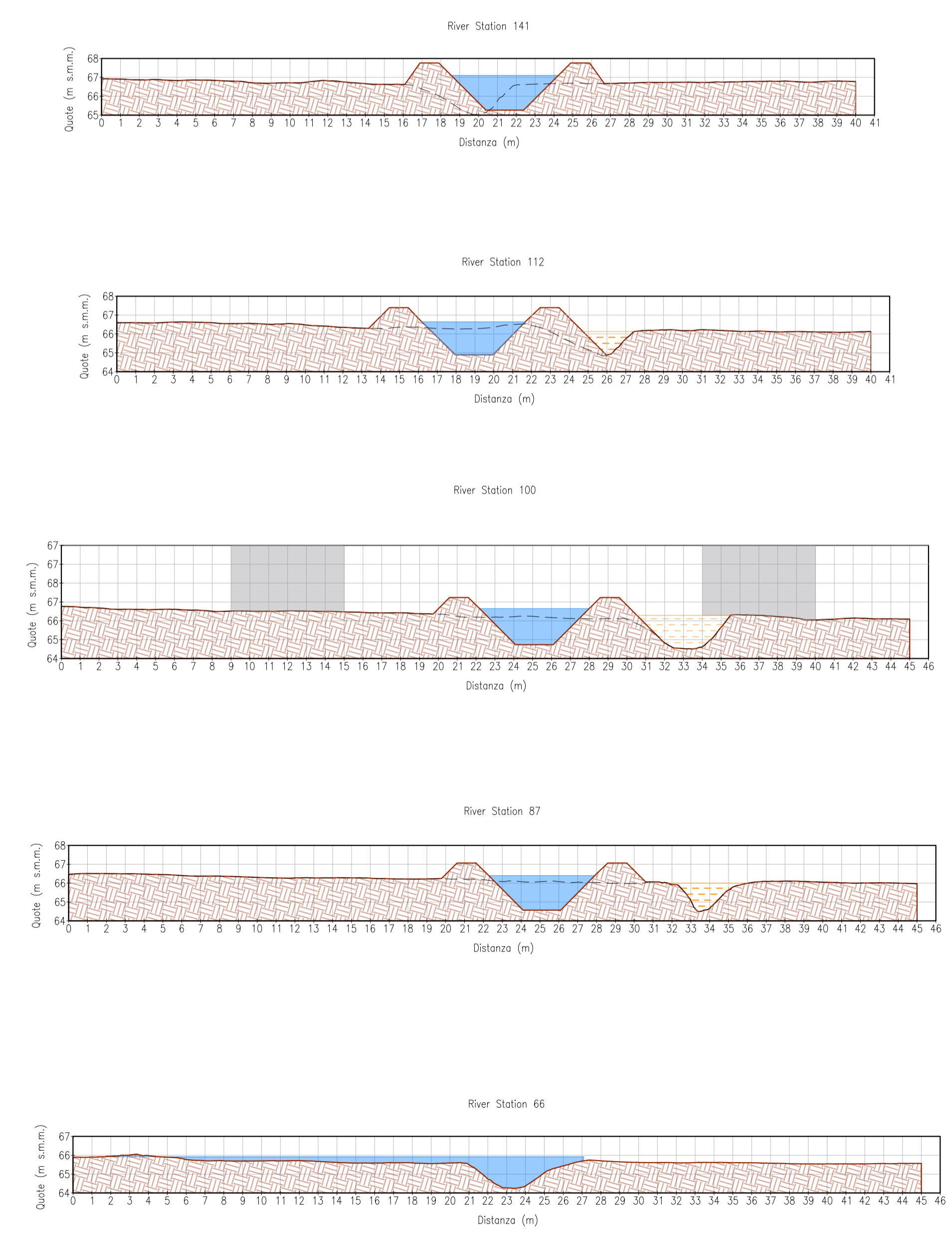
Bacino 4 - Reach 4 - Sezioni post operam - Scala 1:200
