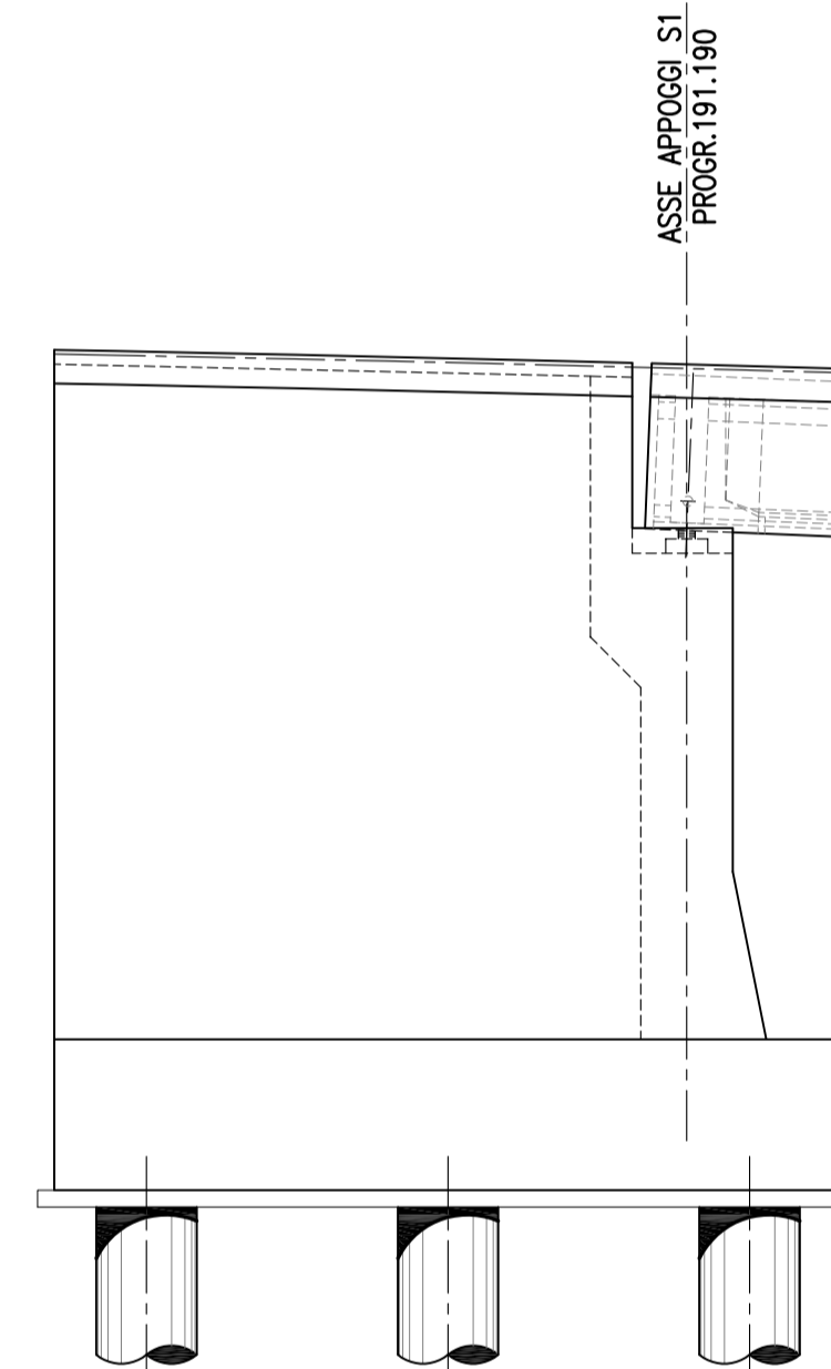
PROSPETTO LATERALE-Scala 1:100
