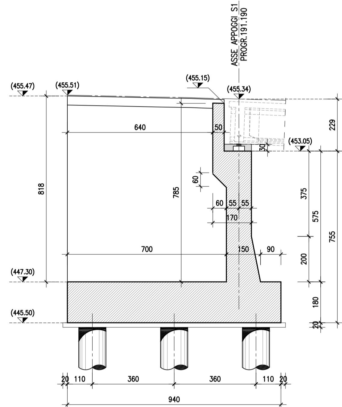
SEZIONE B-B-Scala 1:100
