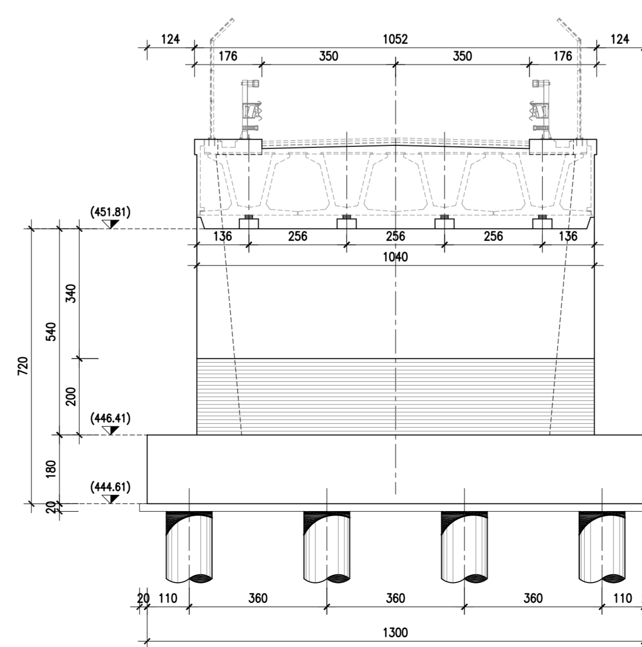
PROSPETTO FRONTALE—Scala 1:100
