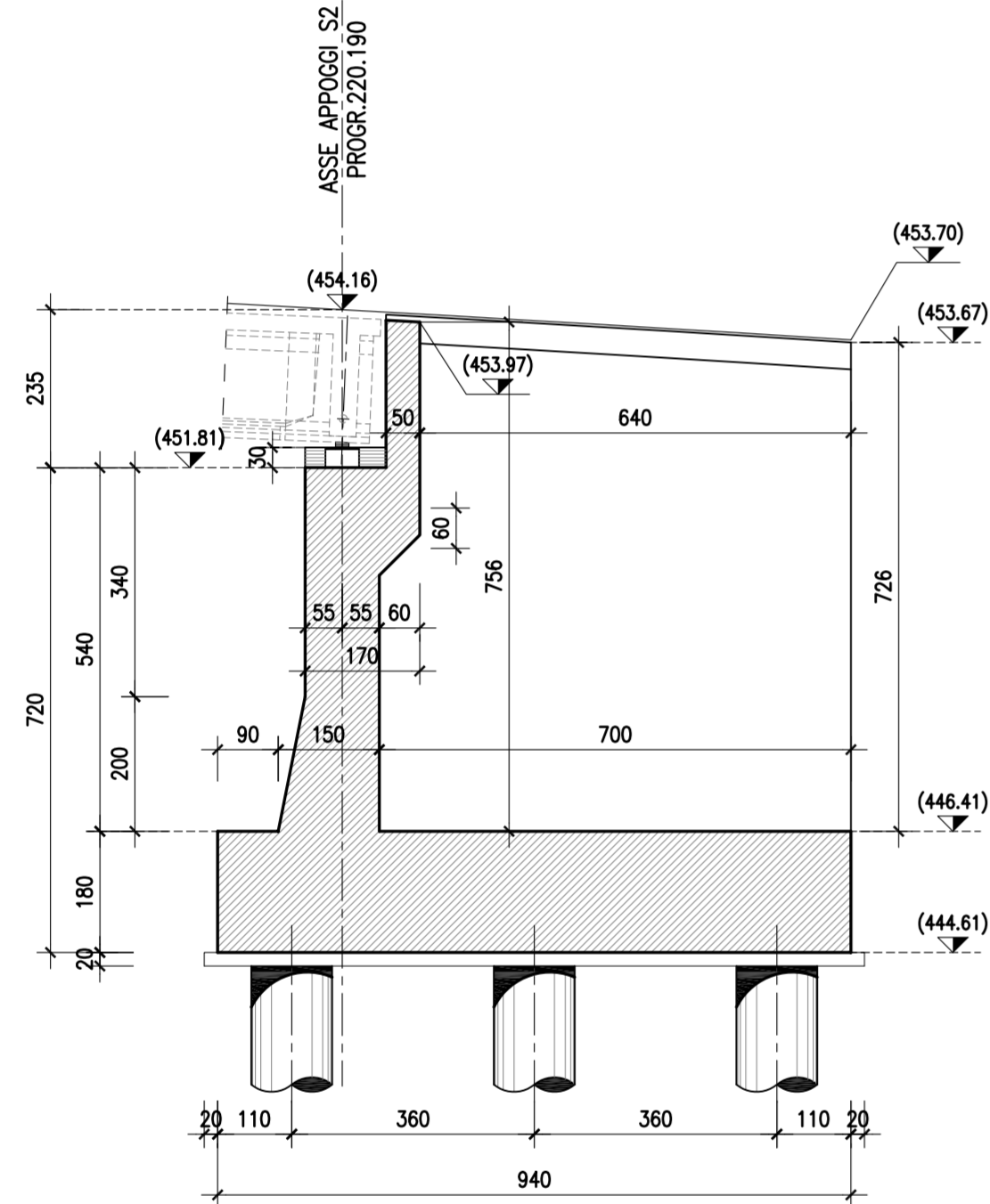
SEZIONE B-B—Scala 1:100
