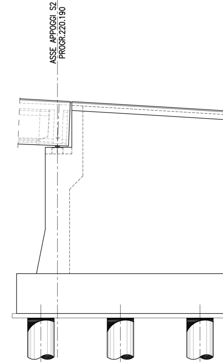
PROSPETTO LATERALE—Scala 1:100
