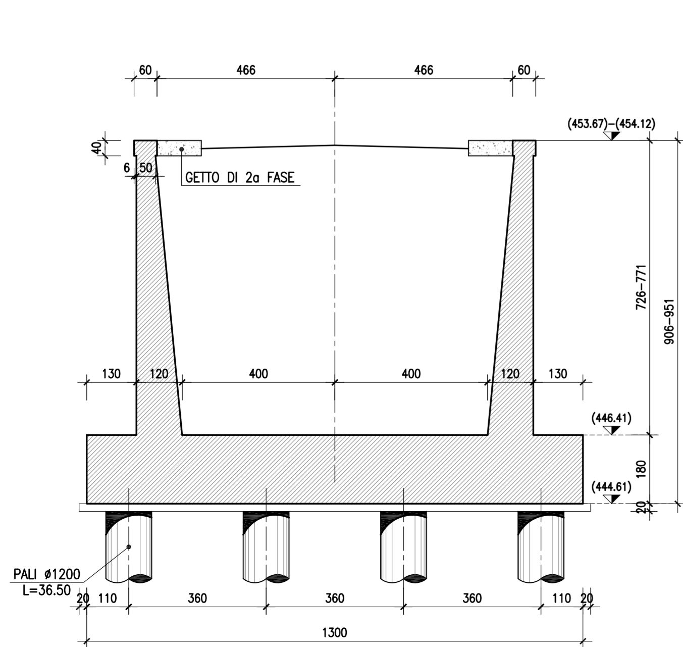
SEZIONE B-B—Scala 1:100
