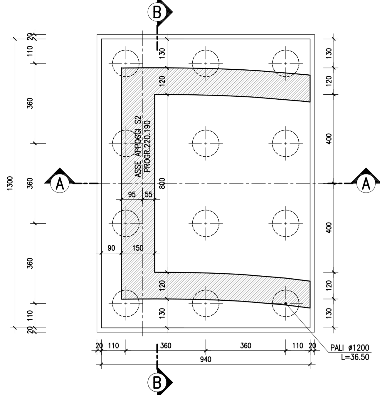
SEZIONE A-A—Scala 1:100
