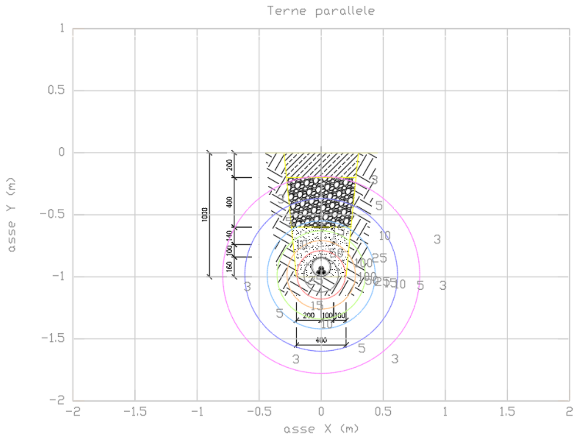
Figura 1 – Livelli di campo magnetico per i cavidotti nei tratti a posa singola
