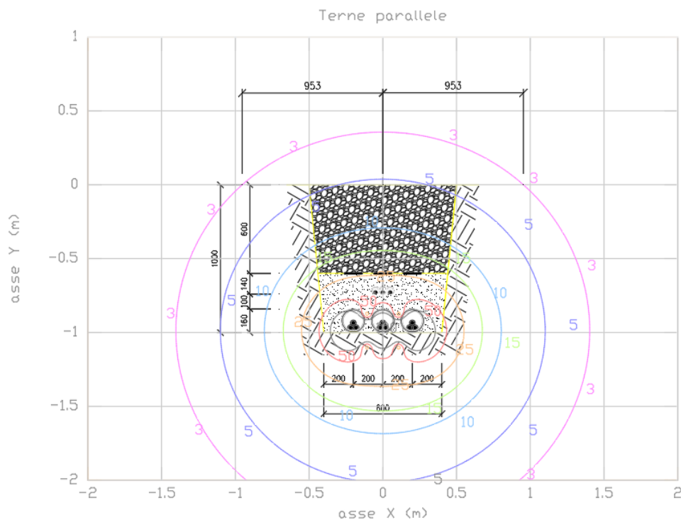
Figura 2 – Livelli di campo magnetico per il tratto dei 3 cavidotti posati parallelamente
