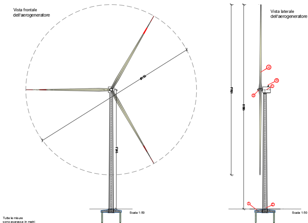
Figura 6 - Schema aerogeneratore H totale 200 m, diametro rotore fino a 155,0 m
