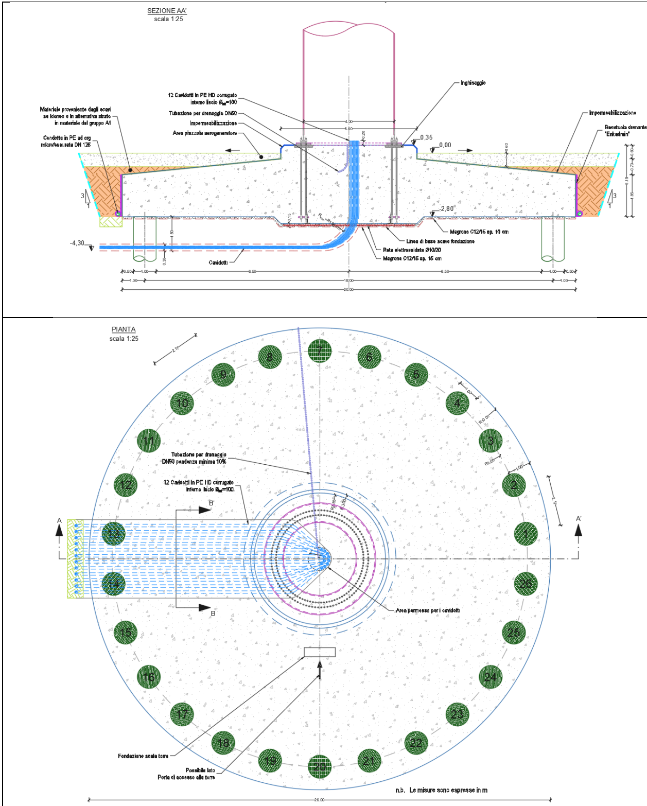
Figura 3.10 - Pianta e sezione del plinto su pali - diametro fondazione 20,00 m
