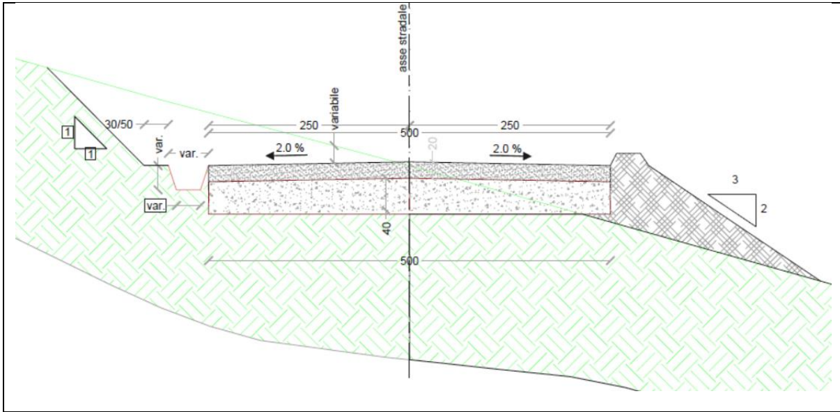
Figura 3.8 - Sezione tipo di scavo a mezzacosta
