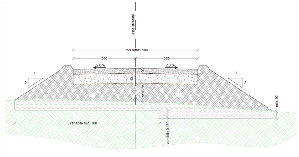
Figura 3.7 - Sezione tipo stradale in rilevato
