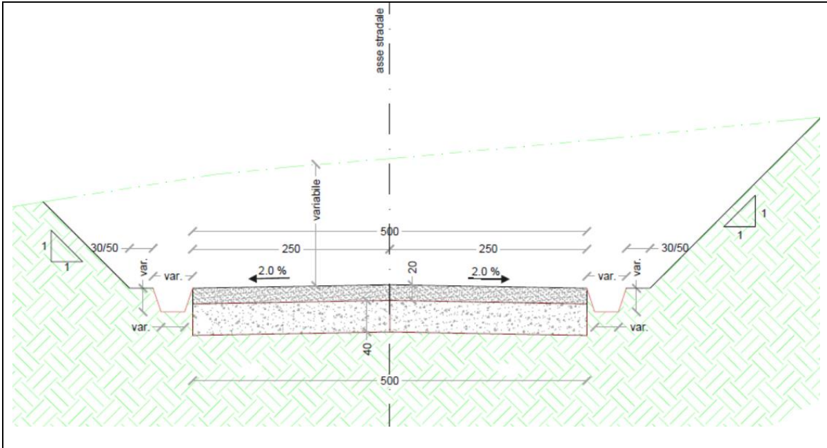
Figura 3.6 – Sezione tipo stradale in scavo
