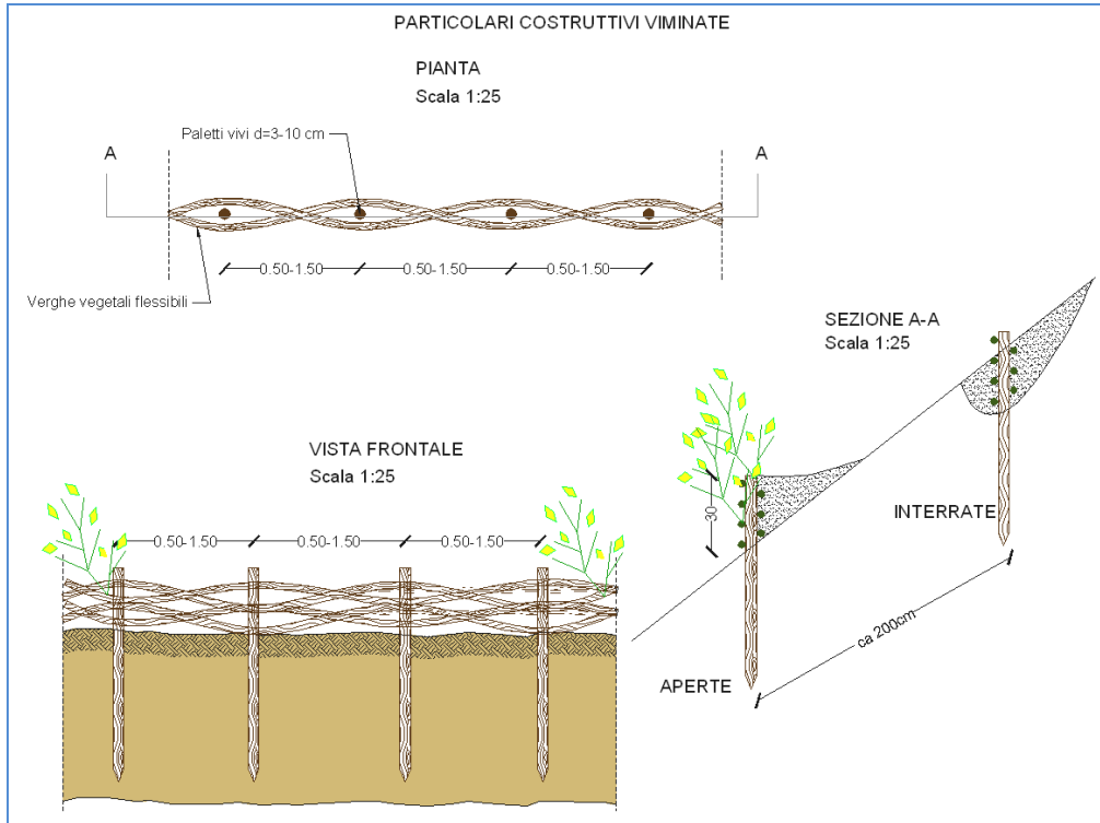
Figura 8.4 – Esempio di viminate - Fonte HE
