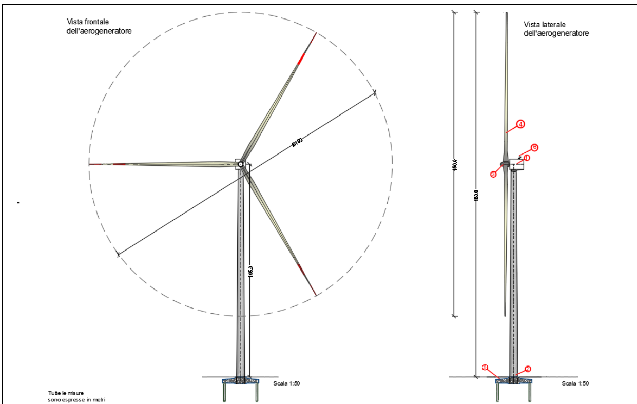
Figura 3.9 - Schema aerogeneratore H totale 200 m, diametro rotore fino a 155,0 m
