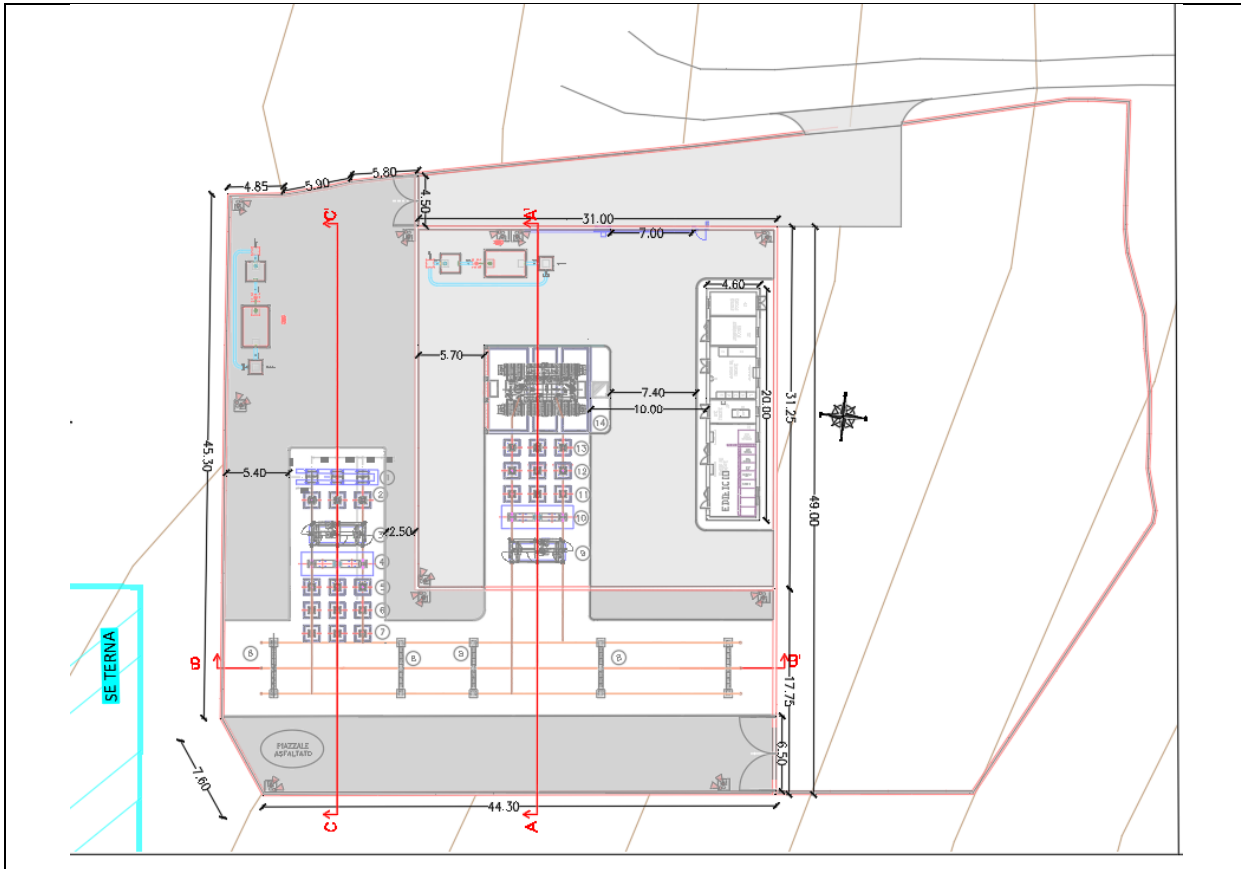
Figura 3.11 - Planimetria stazione utente ed ampliamenti futuri
