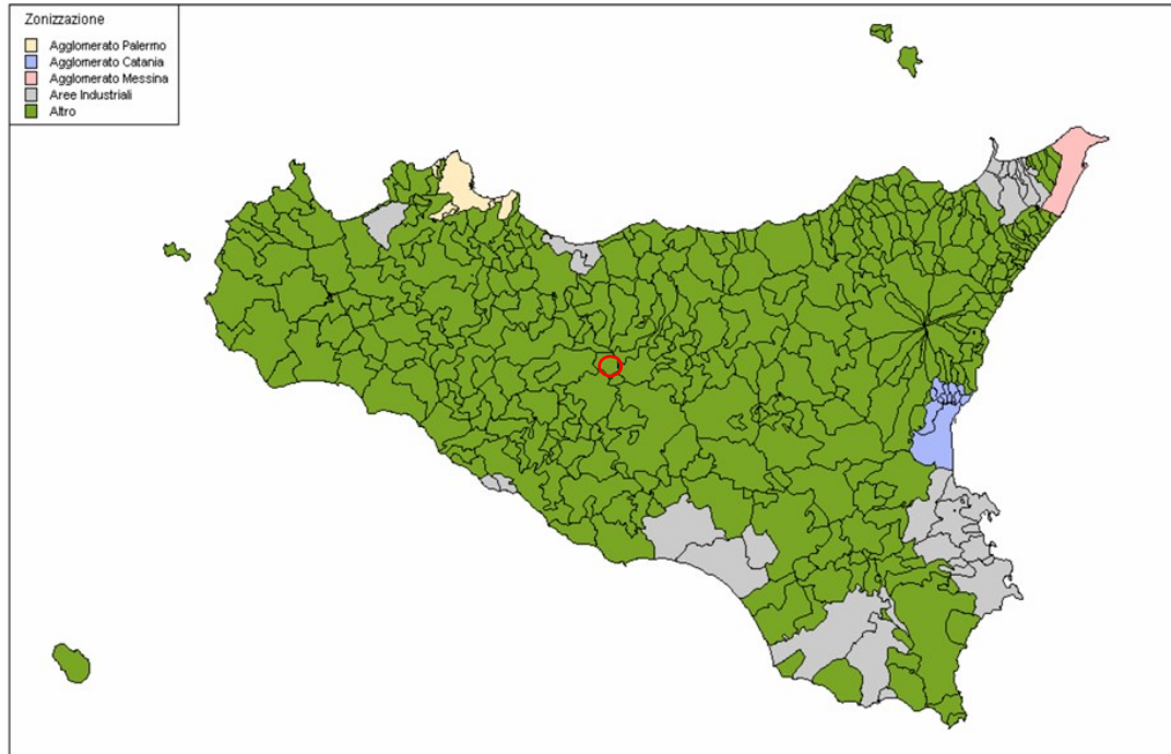
Figura 15 - Zonizzazione e classificazione del territorio della Regione Siciliana con indicazione dell'area di impianto (cerchietto rosso).
