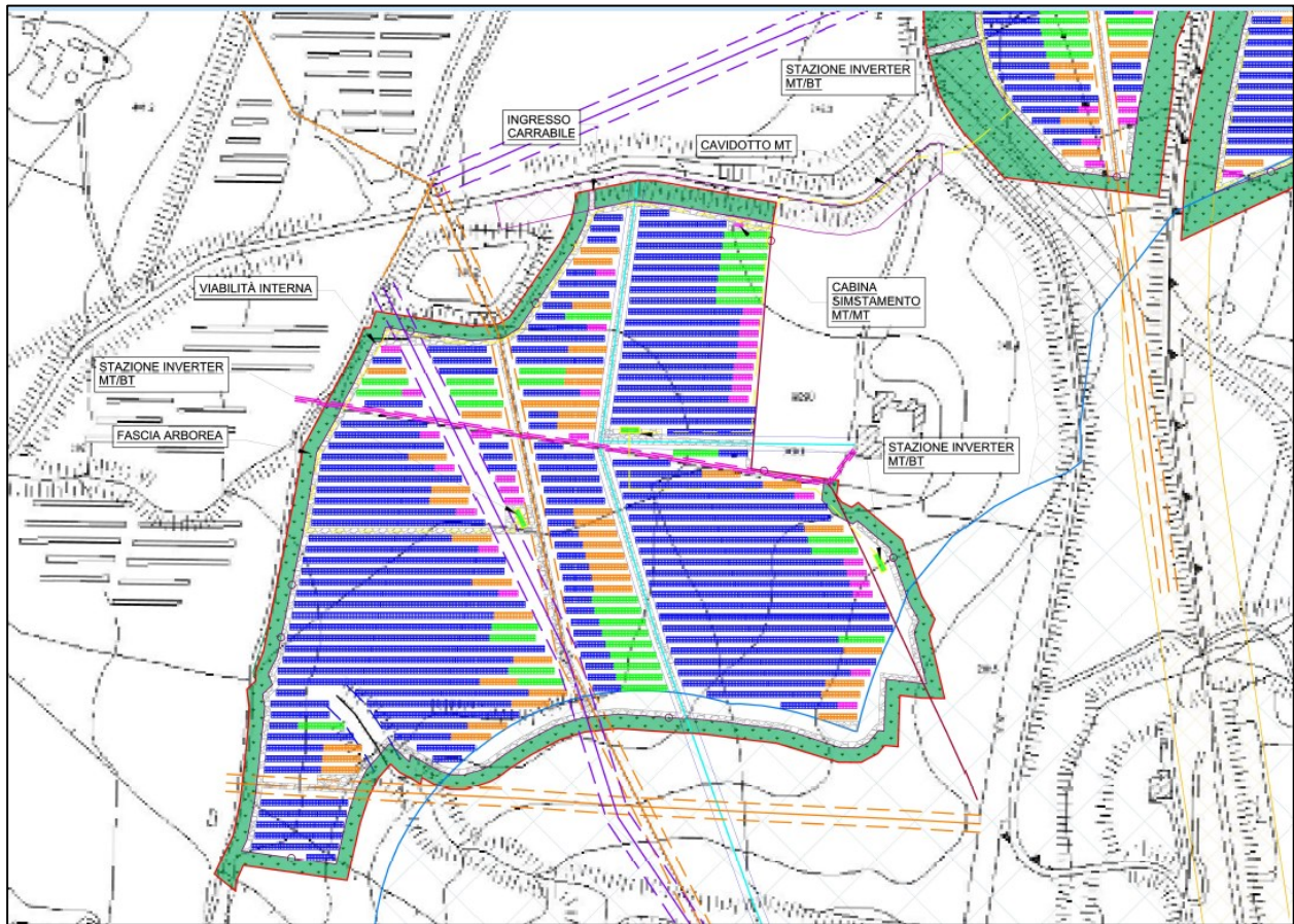
Figura 62 - Layout di impianto (sottoimpianto 4)
