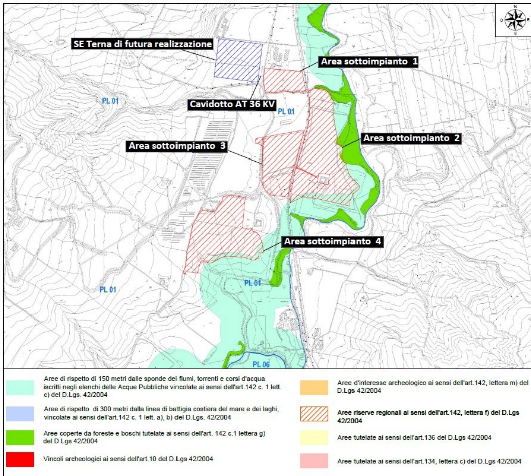
Figura 36 - Vincoli paesaggistici
