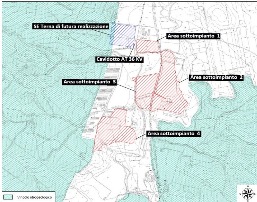
Figura 44 - Vincolo idrogeologico
