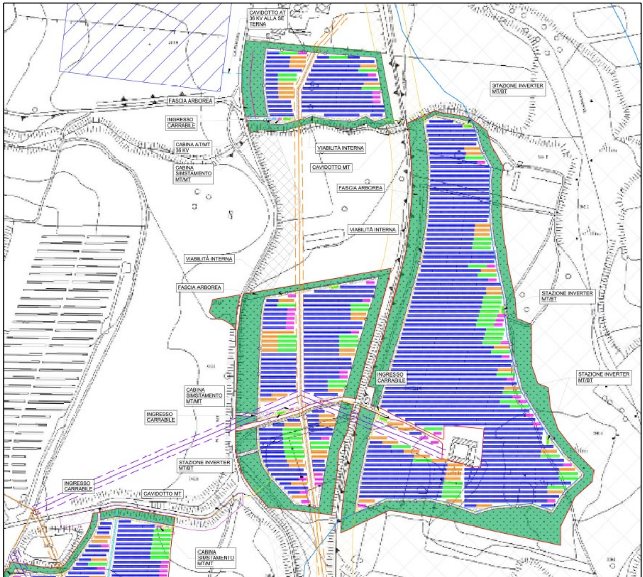
Figura 61 - Layout di impianto (sottoimpianti 1 – 2 – 3)
