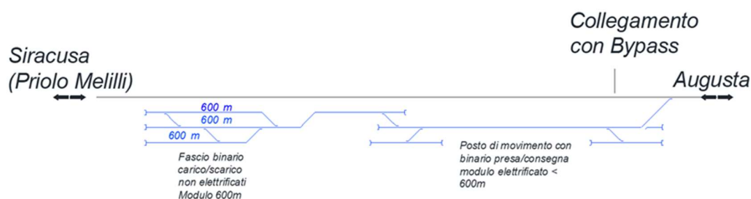
Figura 9-2 - Layout funzionale scenario progetto
