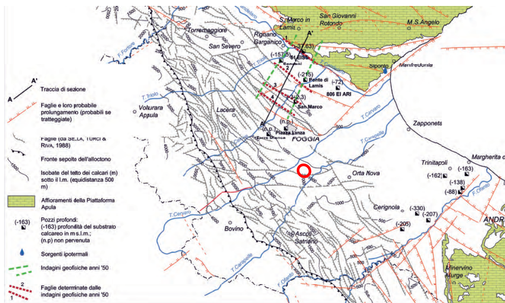
Fig. 14.6 - Lineamenti strutturali del Gargano e del Tavoliere con indicazione dei risultati delle indagini geosismiche e geofisiche condotte nella prima metà del secolo scorso. Indicazione dei pozzi profondi ubicati in destra Ofanto, delle sorgenti ipoterziali e della Punta del ... Structural setting of Gargano and Tavoliere with indication of the results from geophysical and geophysical surveys carried out in the first half of the 20th century. The wells located in the right bank of the Ofanto river, the geothermal springs and Punta del ...
