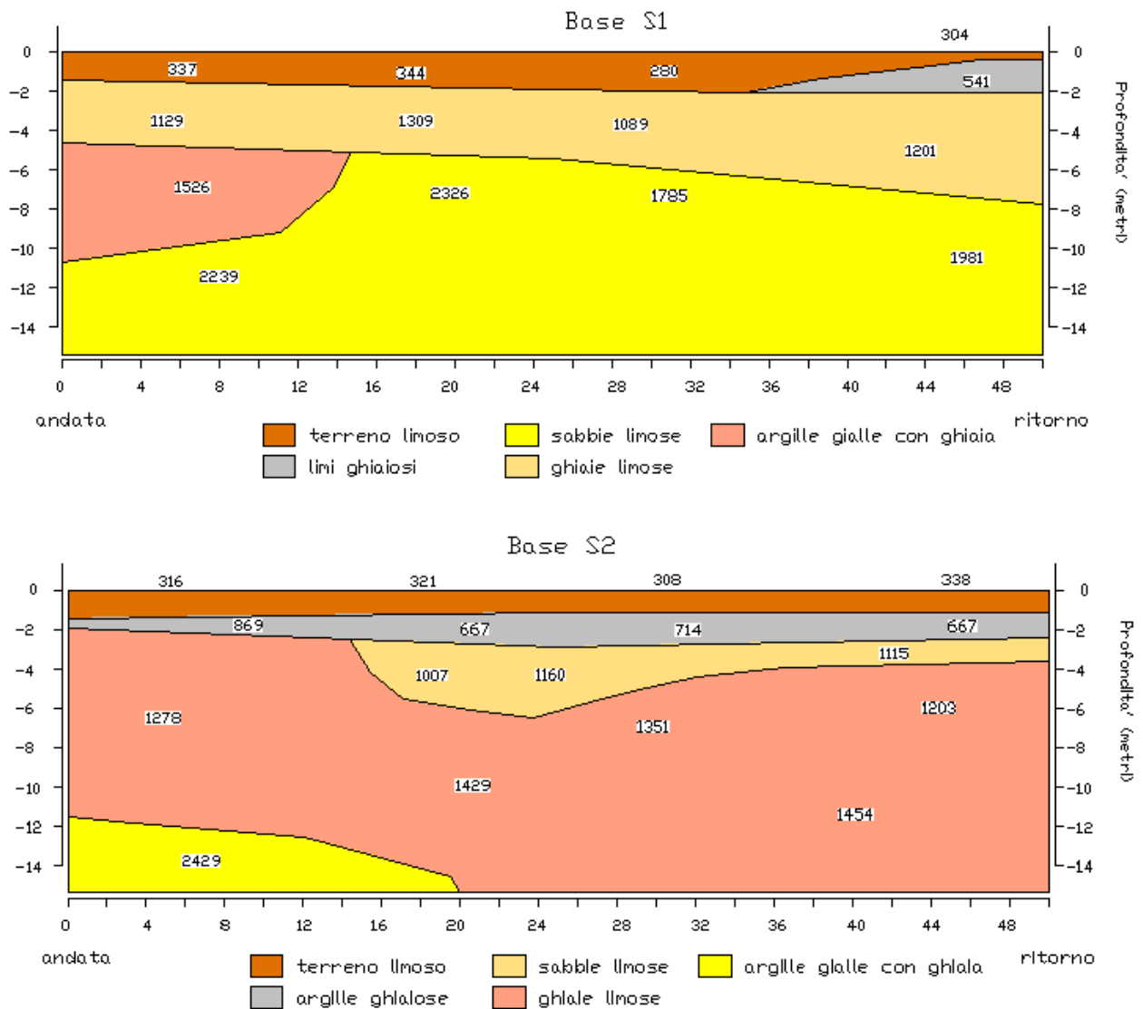
Interpretazione sismo-stratigrafica, Vp
