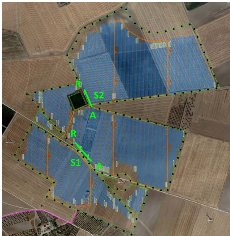
Ubicazione indagine sismica
