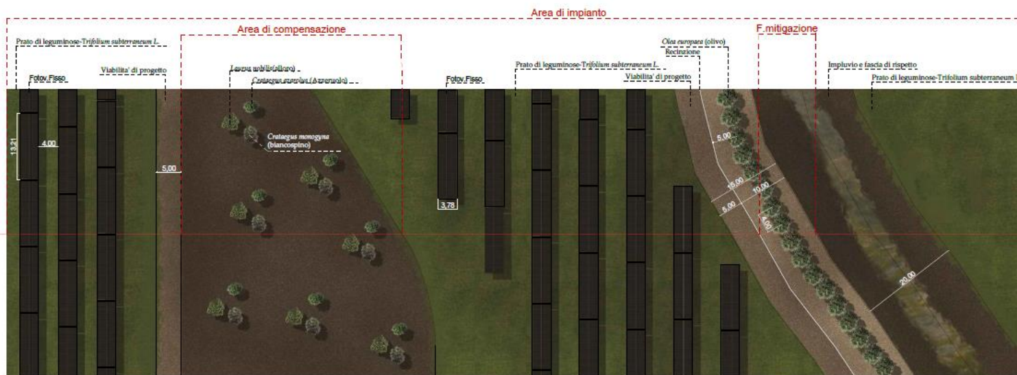
Figura 4: planimetria che mostra l'area di impianto, l'area di compensazione, la fascia di mitigazione e l'impluvio.
