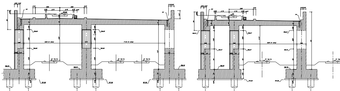
Figura 8-8 Sezioni trasversali
