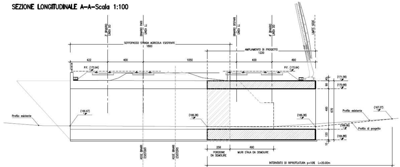
Figura 8-26 Sezione longitudinale
