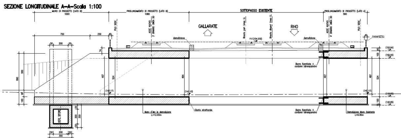
Figura 8-12 Sezione longitudinale
