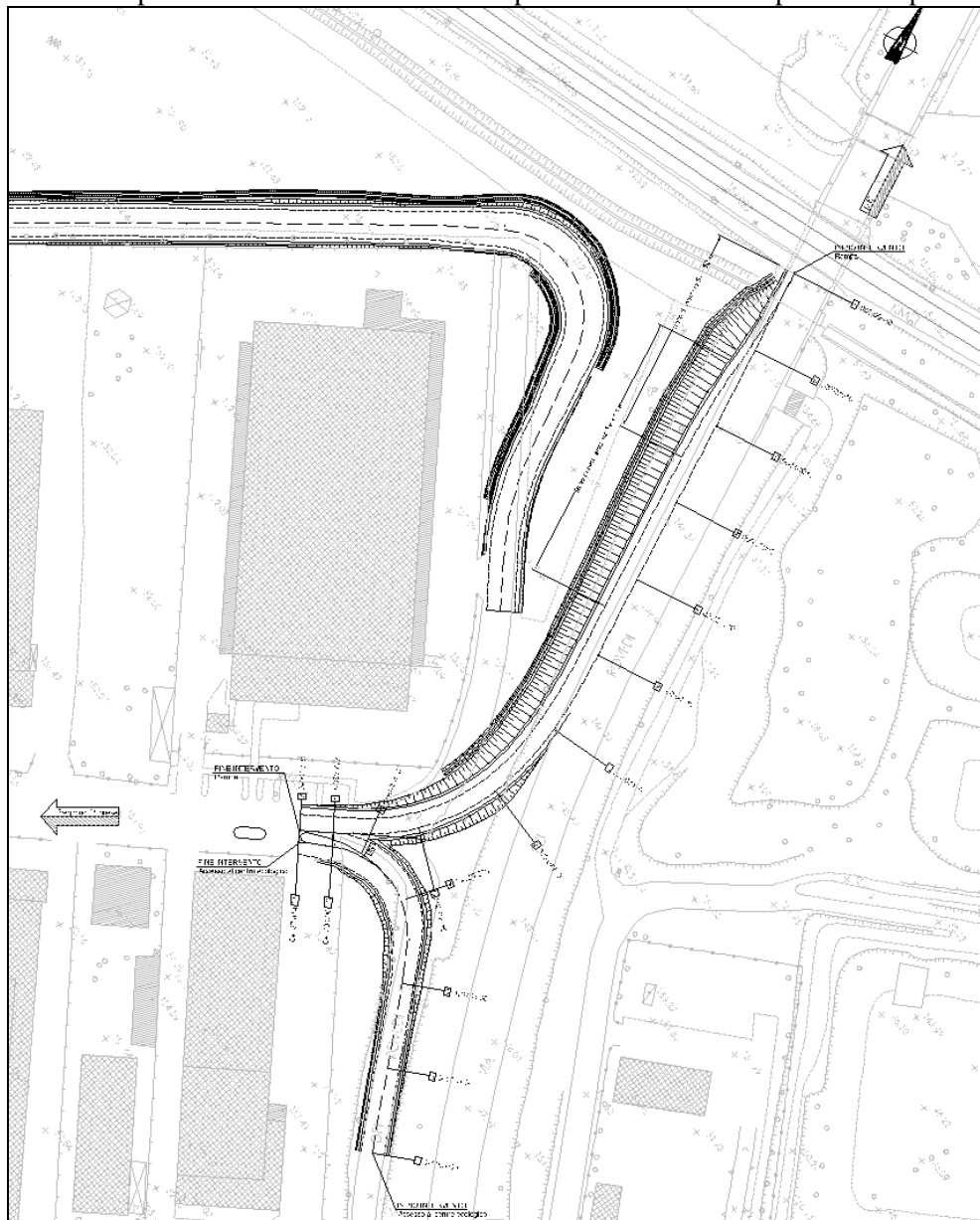
Figura 9-20 Planimetria di progetto
