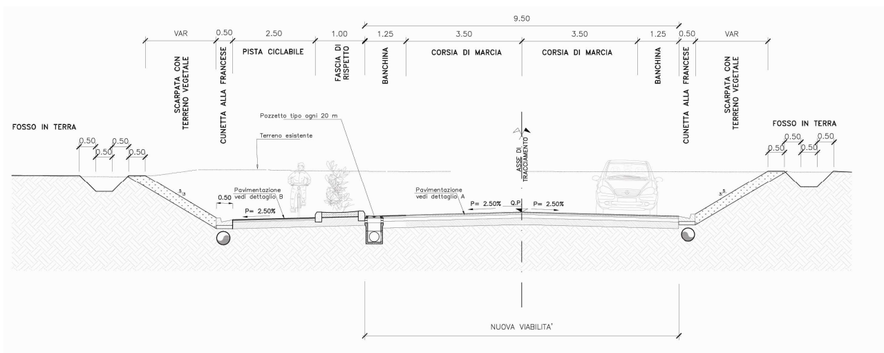
Figura 9-16 Sezione tipo in trincea
