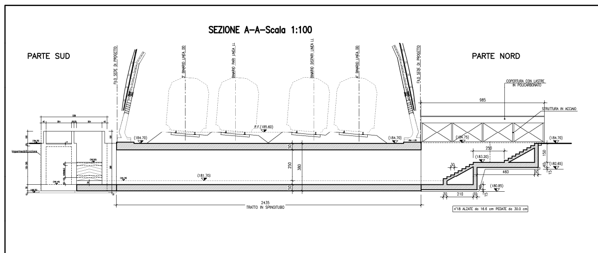
Figura 8-35 Sezione trasversale
