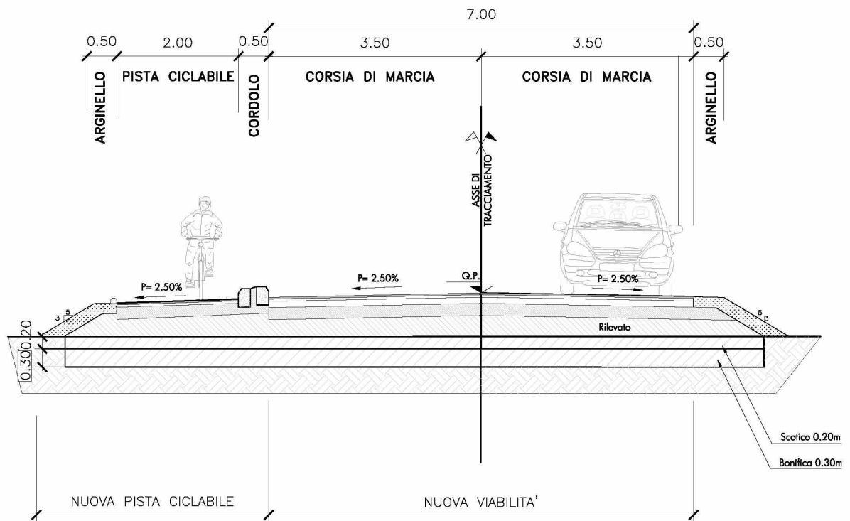
Figura 9-11 Sezione tipo
