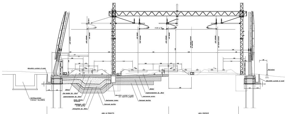
Figura 7-4 Sezione tipo in Vanzago
