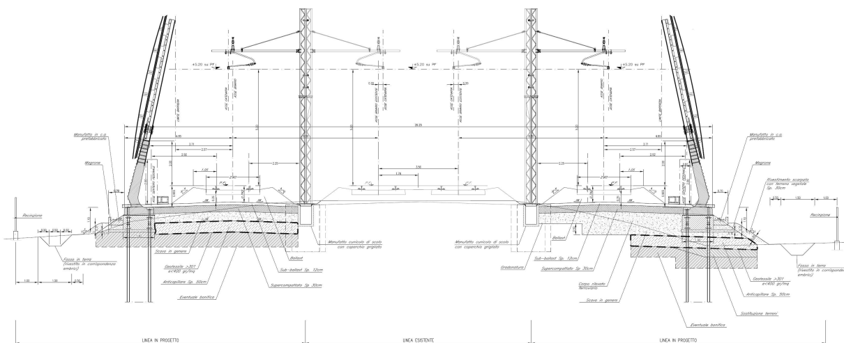
Figura 7-1 Sezione tipo in quadruplicamento
