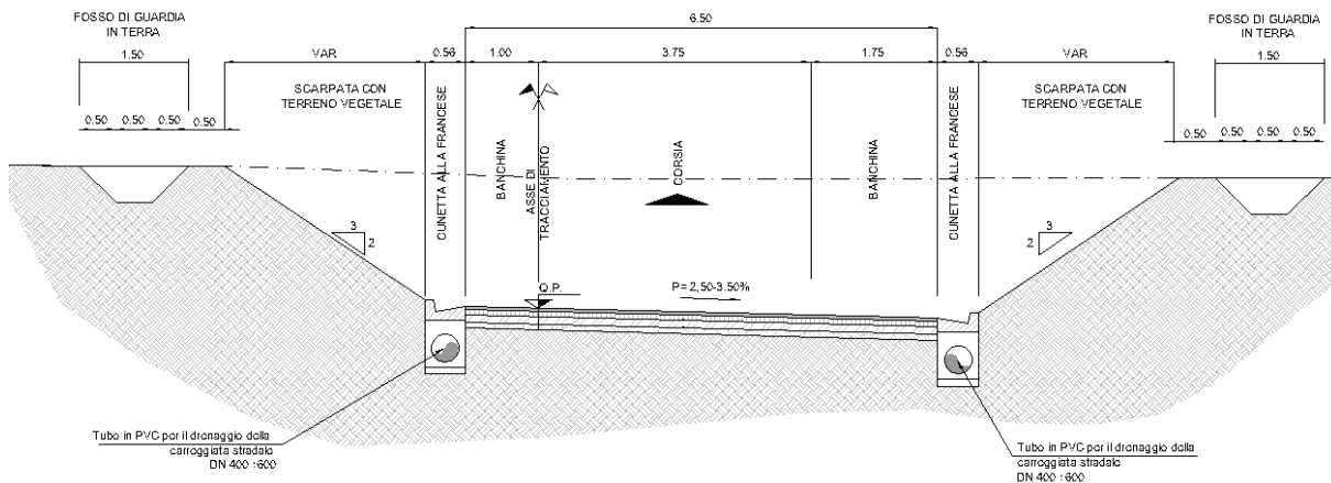
Figura 9-21 Sezione tipo rampa 2
