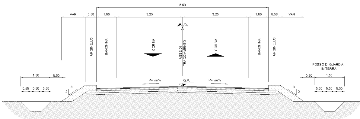
Figura 9-19 Sezione tipo ramo 1
