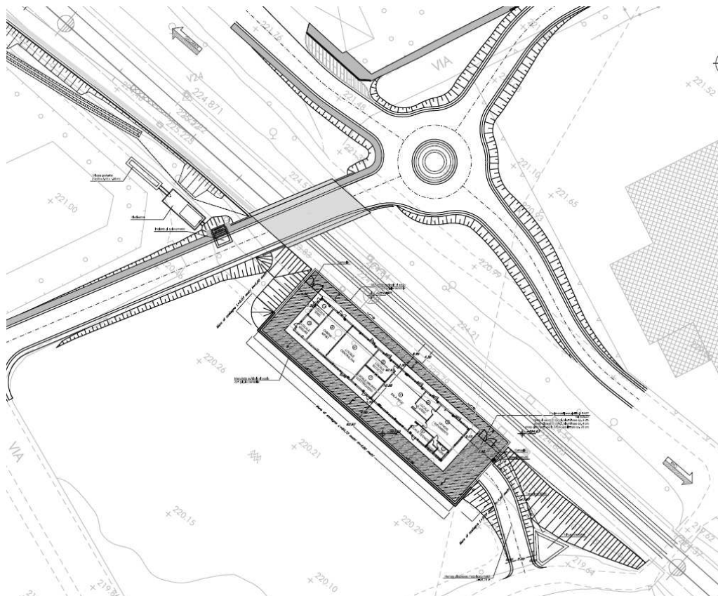
Figura 10-6 Planimetria di progetto
