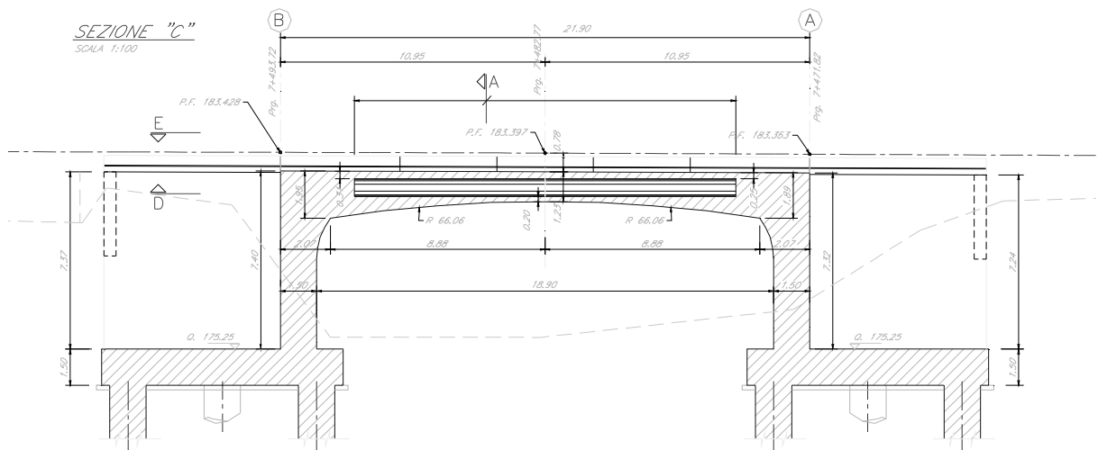
Figura 8-6 Sezione longitudinale
