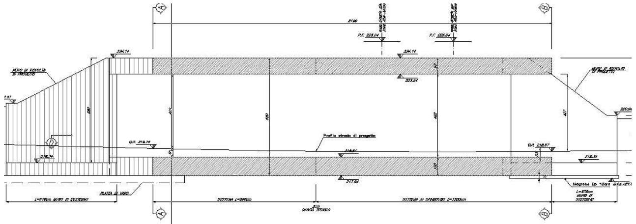
Figura 8-44 Sezione longitudinale
