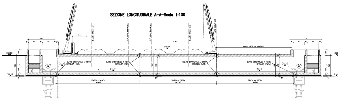
Figura 8-16 Sezione longitudinale
