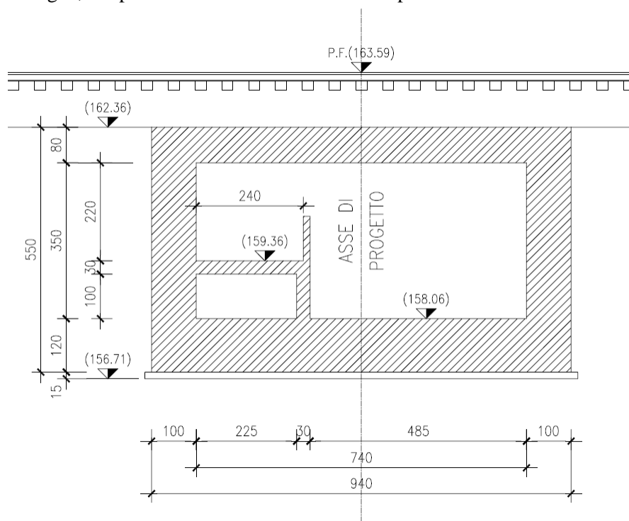
Figura 8-19 Sezione trasversale
