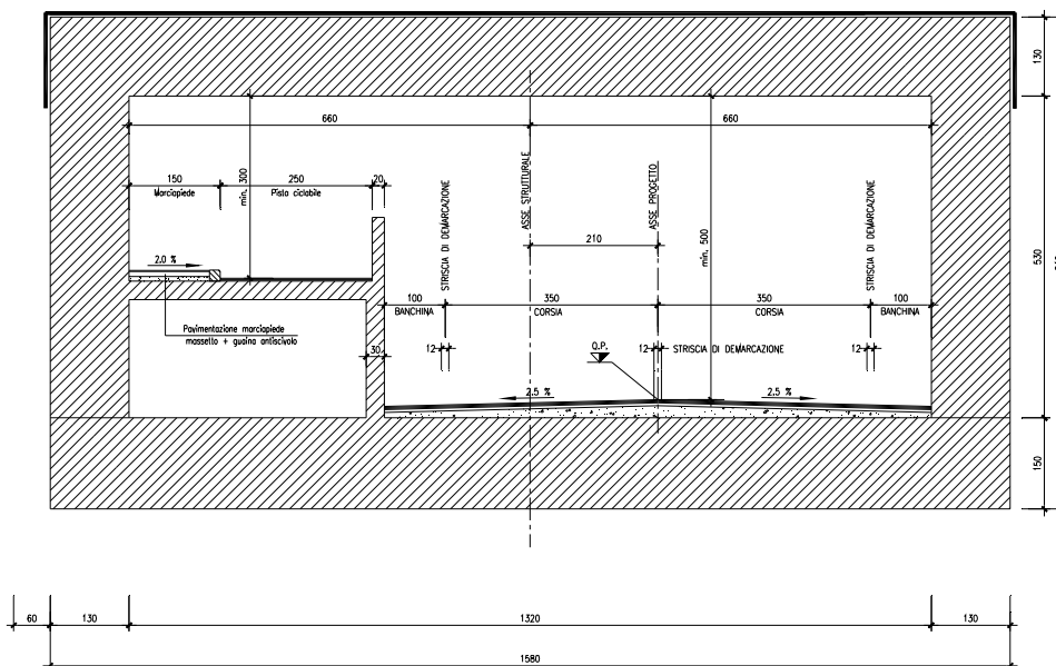
Figura 8-29 Sezione trasversale
