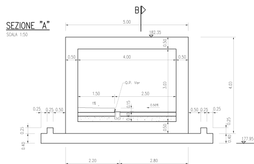
Figura 8-33 Sezione sottopasso
