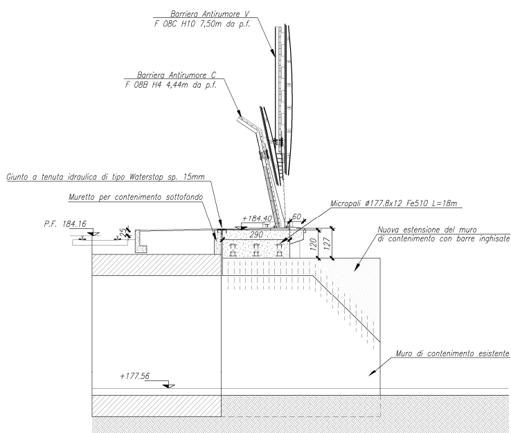
Sezione passerella porta B.A.
