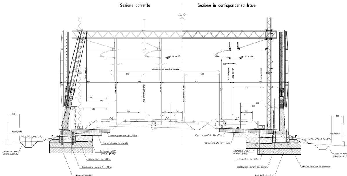
Figura 7-2 Sezione con adeguamento del binario esistente
