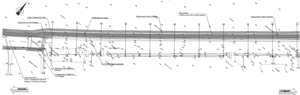
Figura 9-28 Stralcio planimetrico – tratto in affiancamento a via I° Maggio
