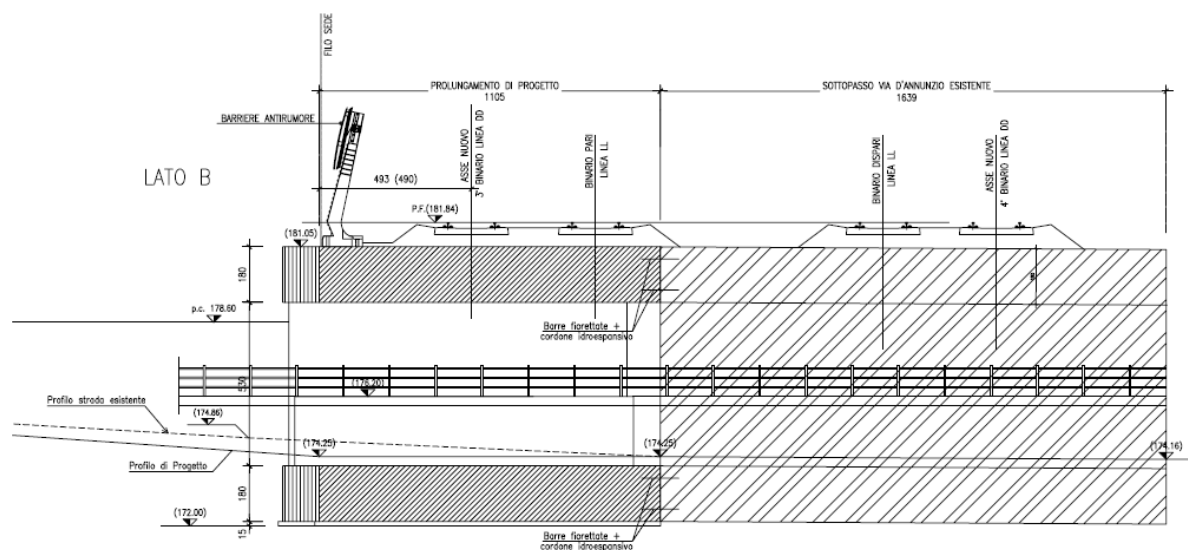
Figura 8-31 Sezione longitudinale
