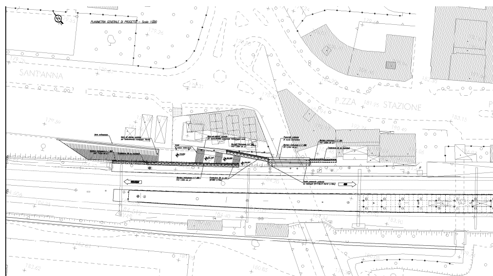
Figura 9-40 Planimetria di intervento
