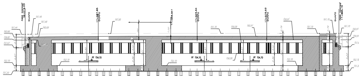
Figura 8-7 Sezioni longitudinali
