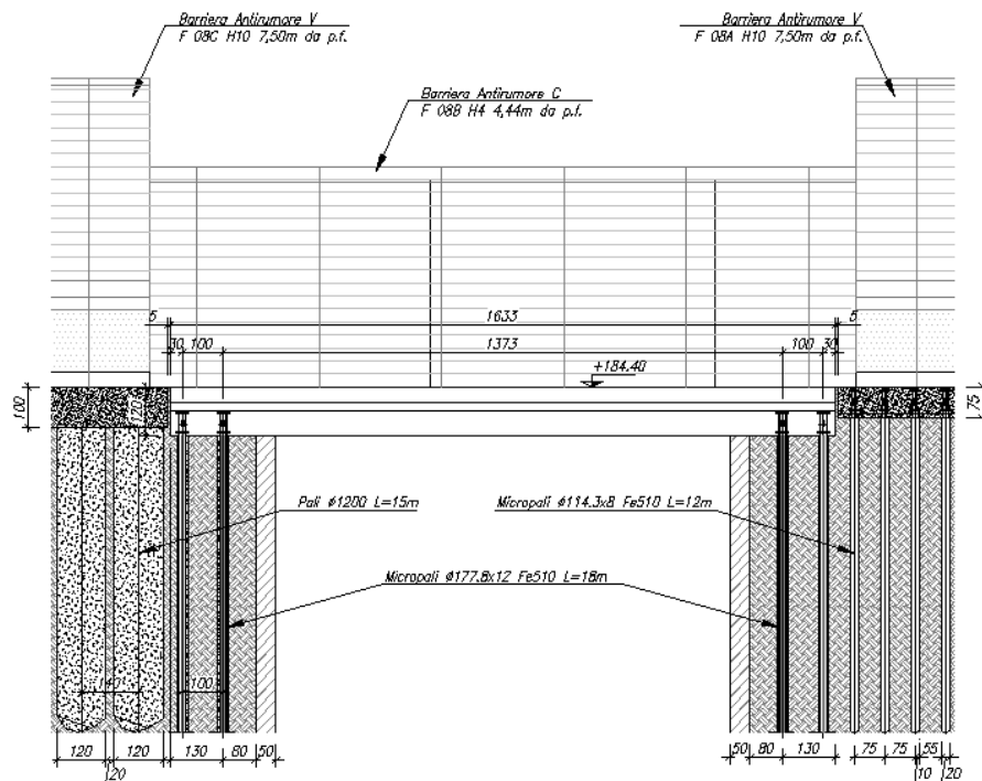
Figura 9-41 Vista passerella
