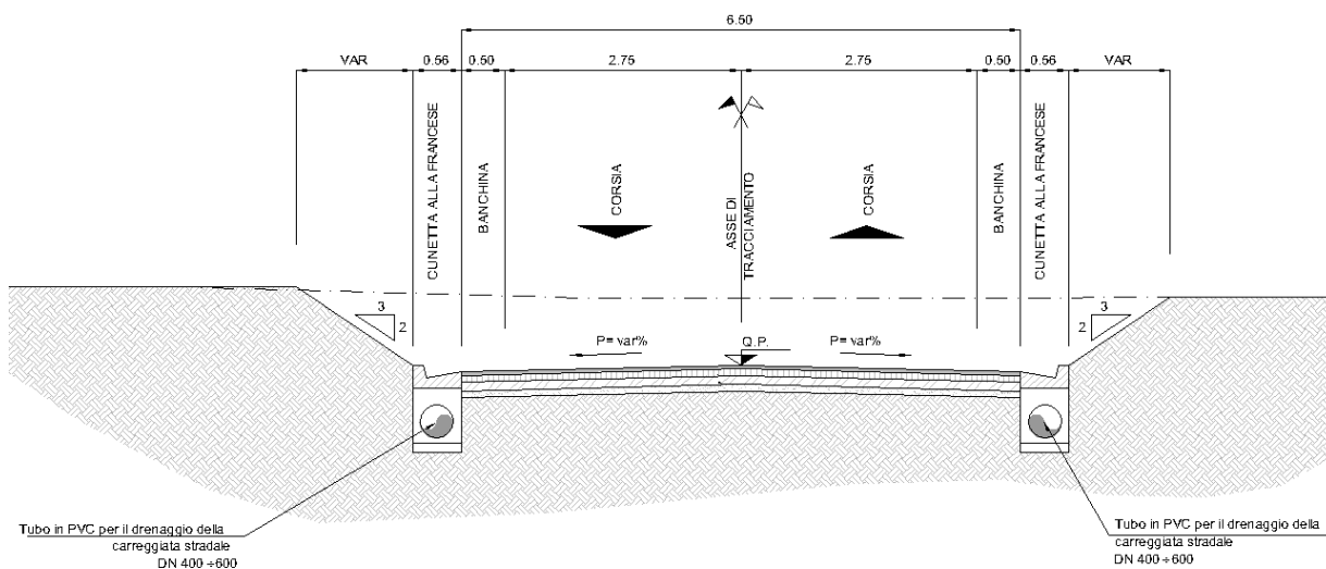
Figura 9-22 Sezione tipo ramo 2
