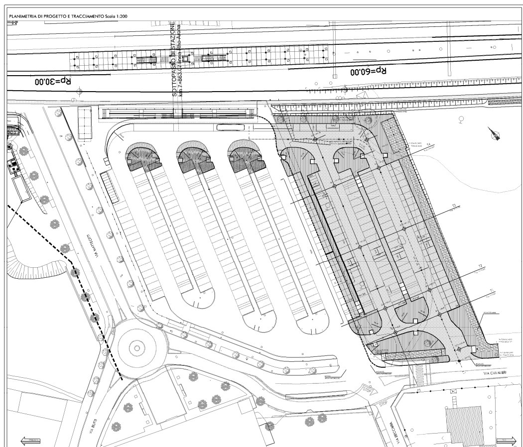
Figura 9-38 Planimetria di intervento
