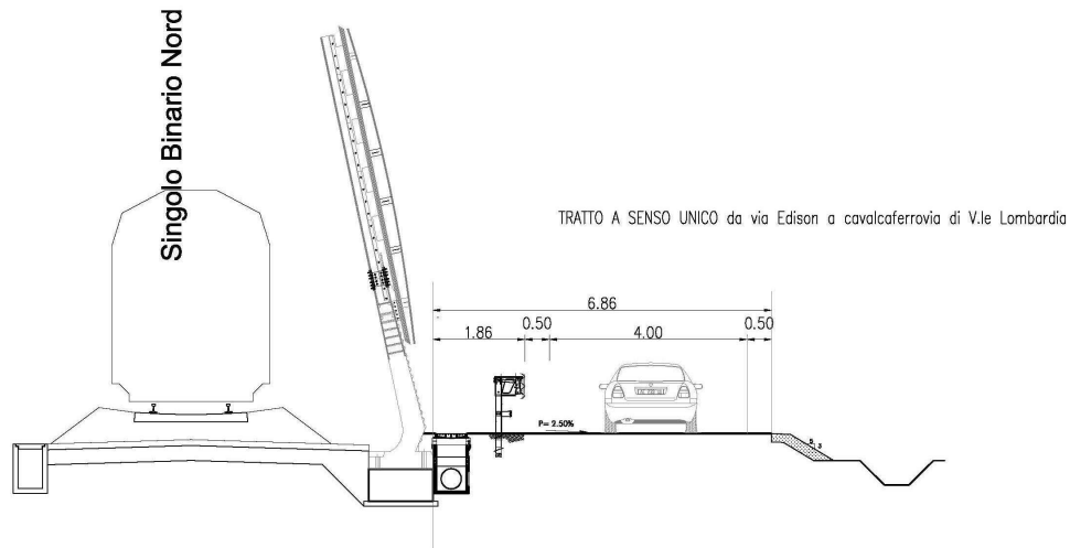
Figura 9-4 – Sezione nel tratto a senso unico
