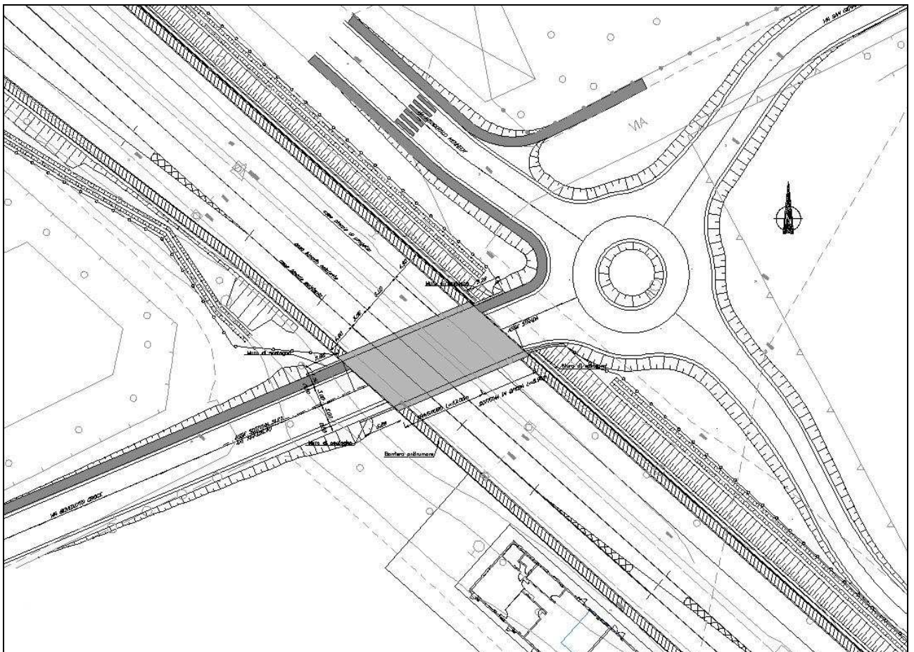
Figura 8-43 Planimetria di progetto
