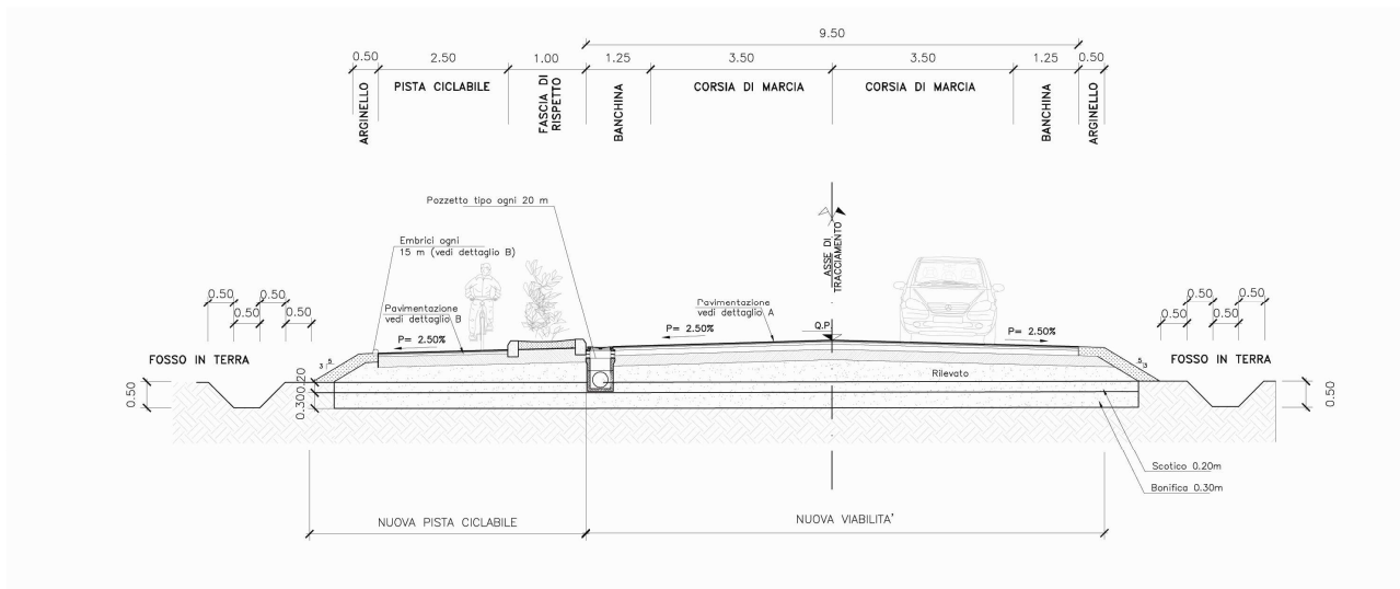
Figura 9-15 Sezioni tipo rilevato
