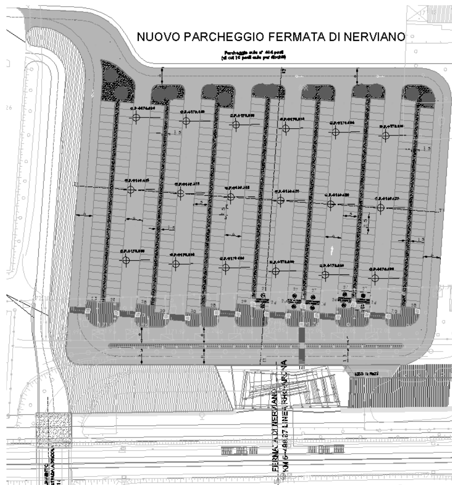
Figura 9-44 Planimetria di intervento
