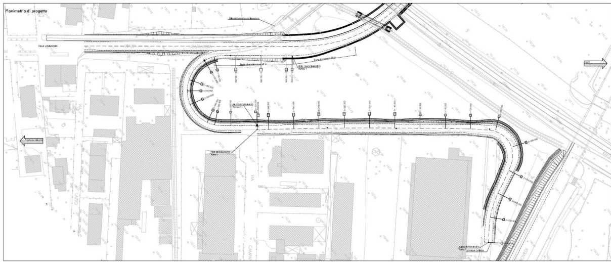
Figura 9-17 Planimetria di progetto
