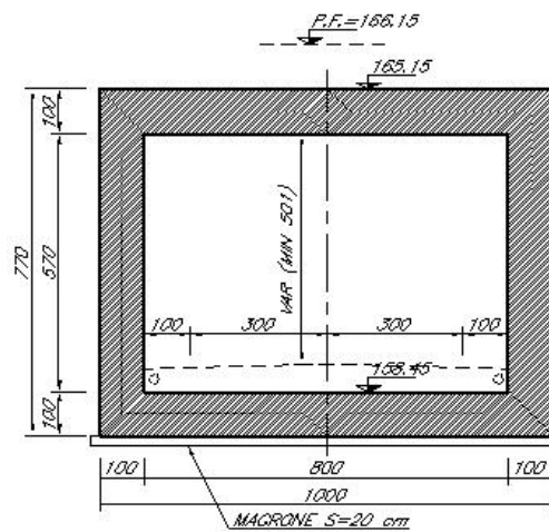
Figura 8-47 Sezione trasversale
