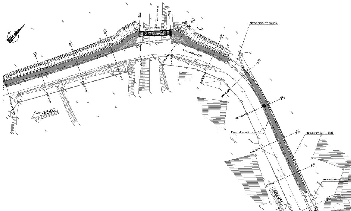
Figura 9-29 Stralcio planimetrico – tratto in affiancamento a via Castellazzo
