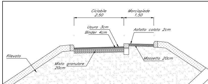
Figura 9-2 Sezione trasversale
