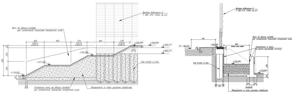
Figura 9-42 Vista scala
