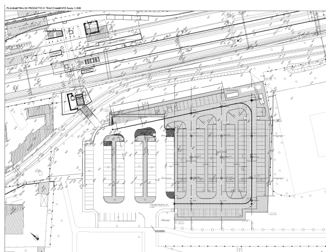
Figura 9-37 Planimetria di intervento
