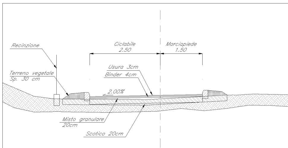
Figura 9-27 Sezione tipo in affiancamento alla carreggiata esistente
