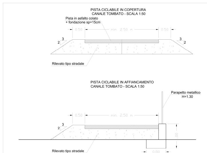
Figura 9-24 Sezioni tipo
