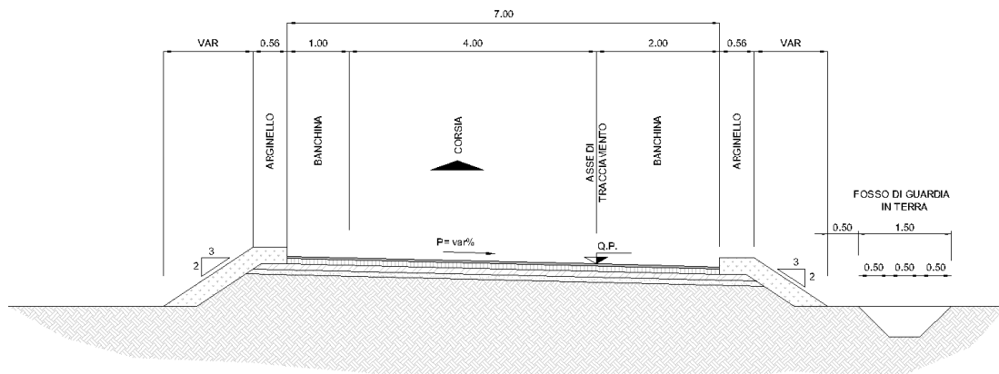
Figura 9-18 Sezione tipo rampa 1
