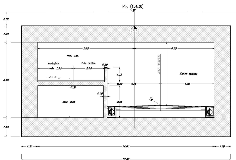
Figura 8-50 Sezione trasversale
