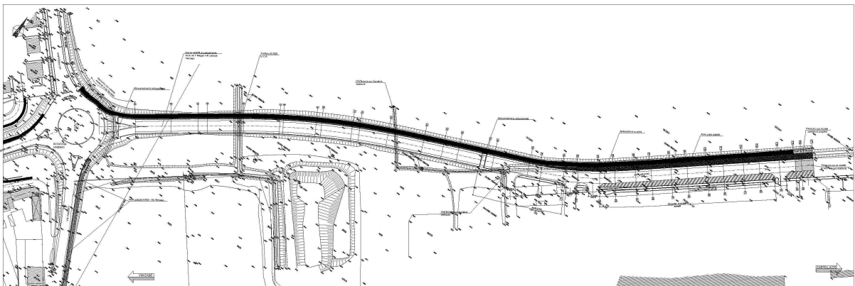
Figura 9-14 Planimetria di progetto
