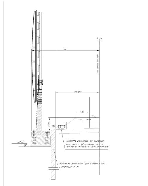
Figura 7-5 Sezione tipo barriera antirumore per rilevato esistente
