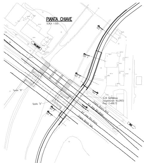
Figura 8-32 Planimetria dell'intervento
