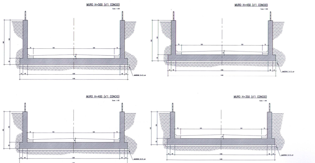
Figura 8-24 Sezione trasversale dei muri ad U
