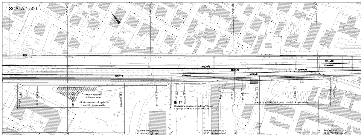
Figura 9-23 Planimetria dell'intervento
