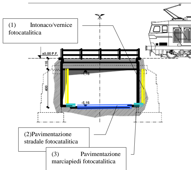
Figura 8-10 Esempio di intervento tipologico
