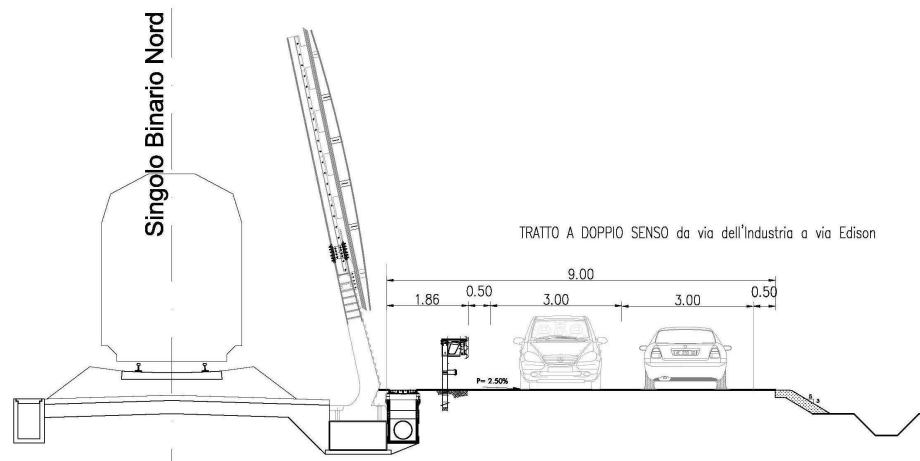
Figura 9-5 Sezione nel tratto a doppio senso di marcia
