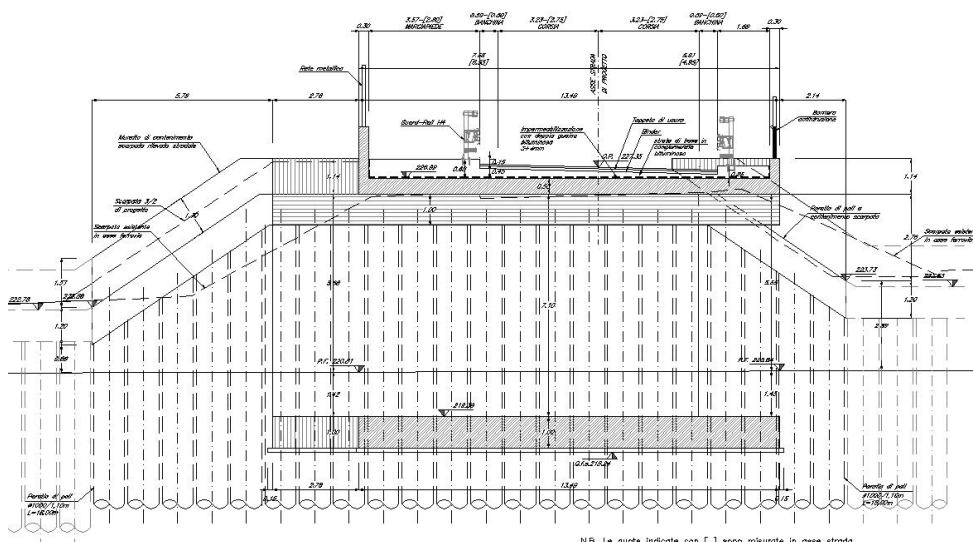
Figura 8-9 Sezione longitudinale
