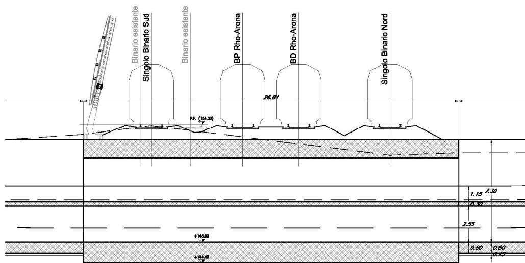
Figura 8-49 Sezione longitudinale
