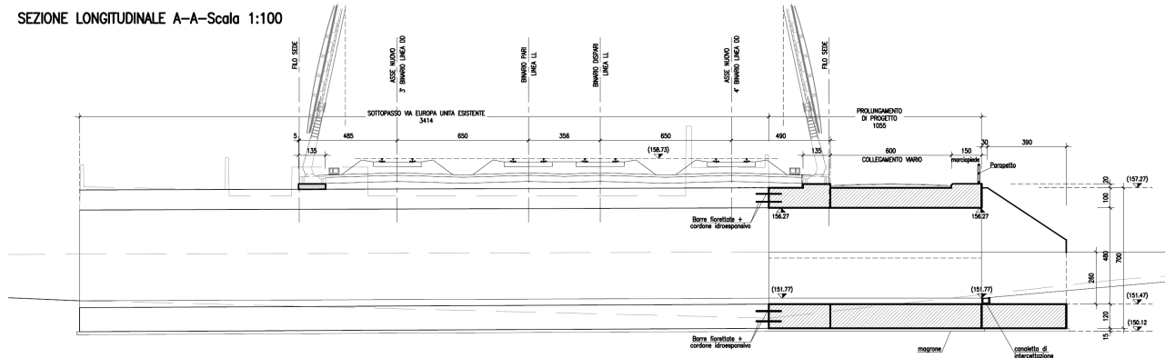
Figura 8-14 Sezione longitudinale
