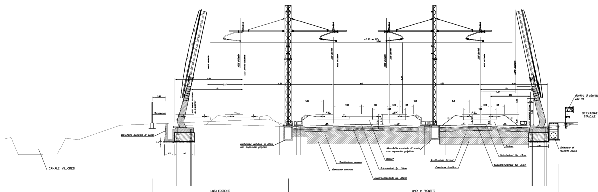
Figura 7-3 Sezione tipo in Pregana Milanese
