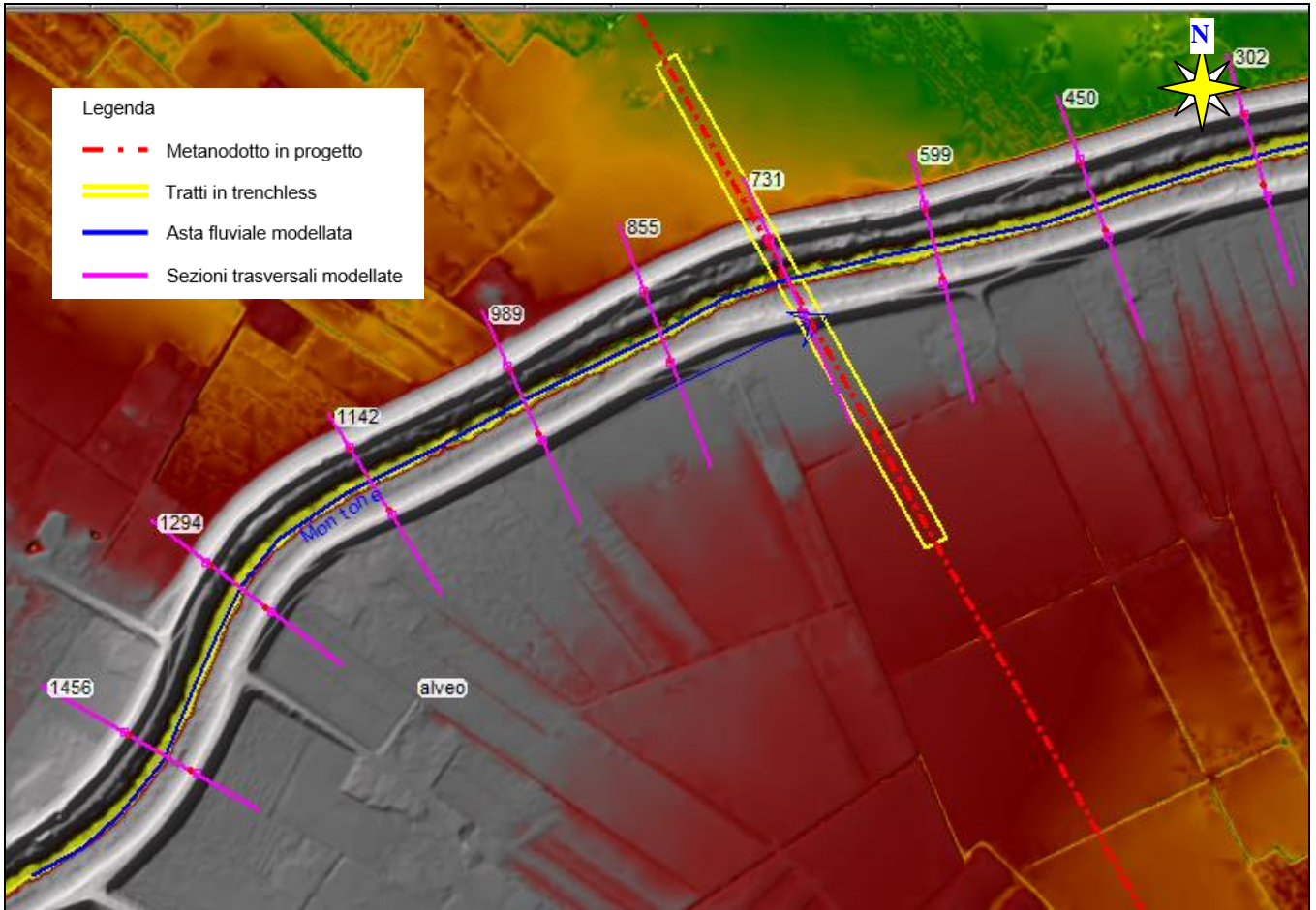
Fig.5.2/A: Schermata del DTM, con tronco d'alveo analizzato e sezioni di input nella modellazione
