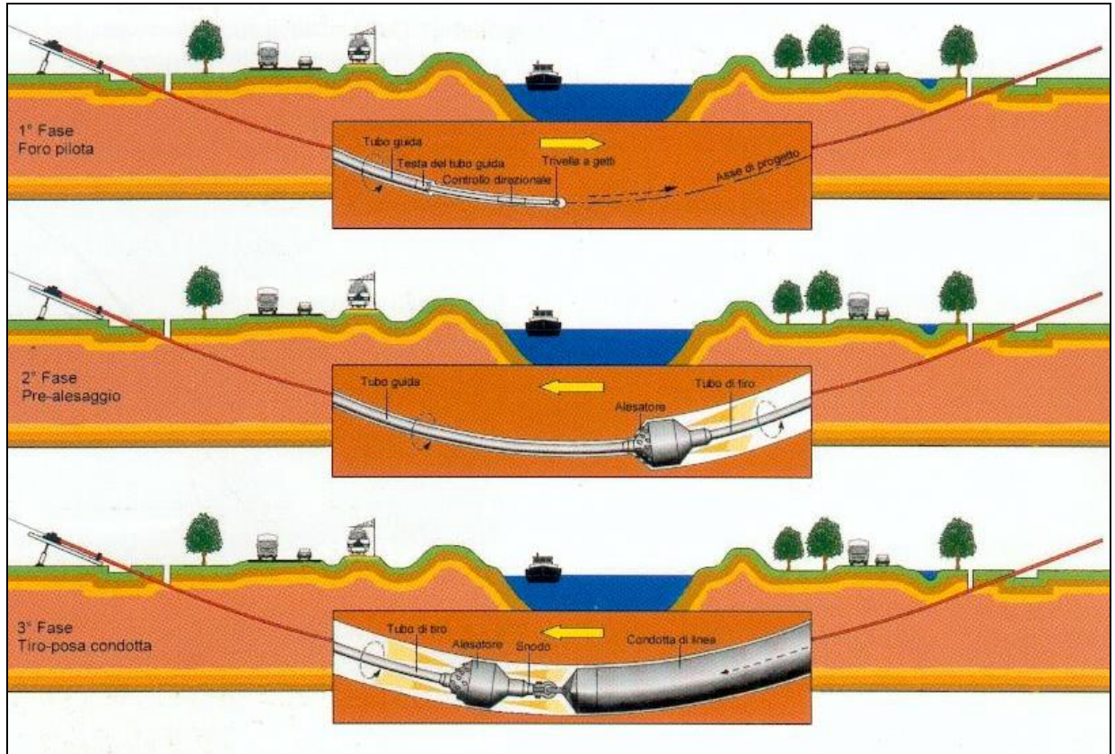
Fig.7.4/A: T.O.C.- Fasi di lavoro
