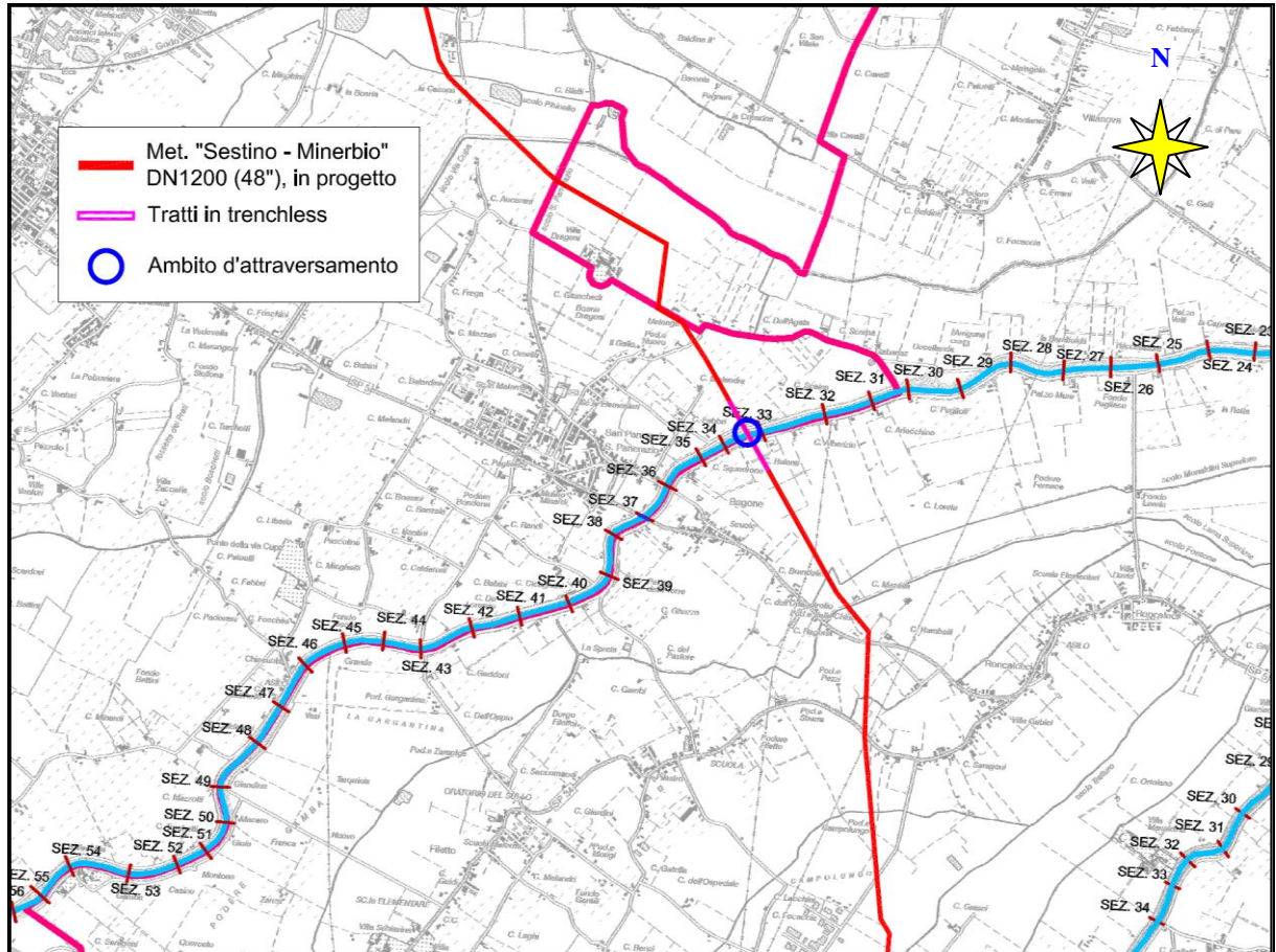
Fig.4.4/A: Stralcio della Tav.2 – con individuazione ambito attraversamento del Montone
