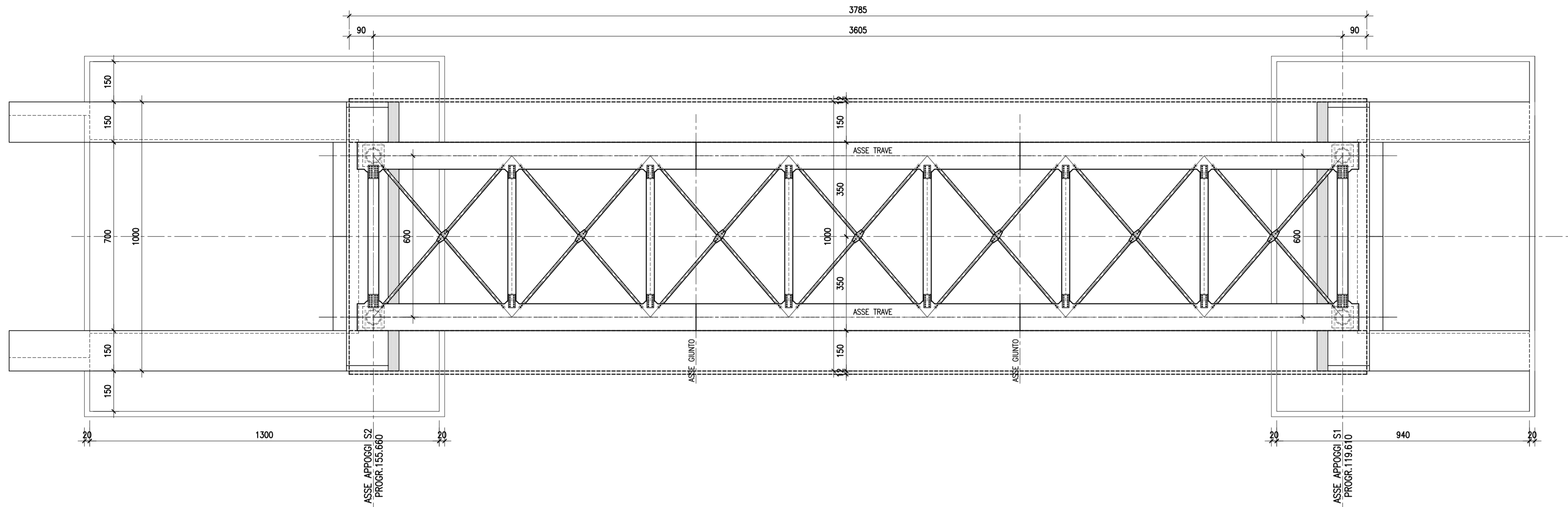
PIANTA FONDAZIONI—Scala 1:100
