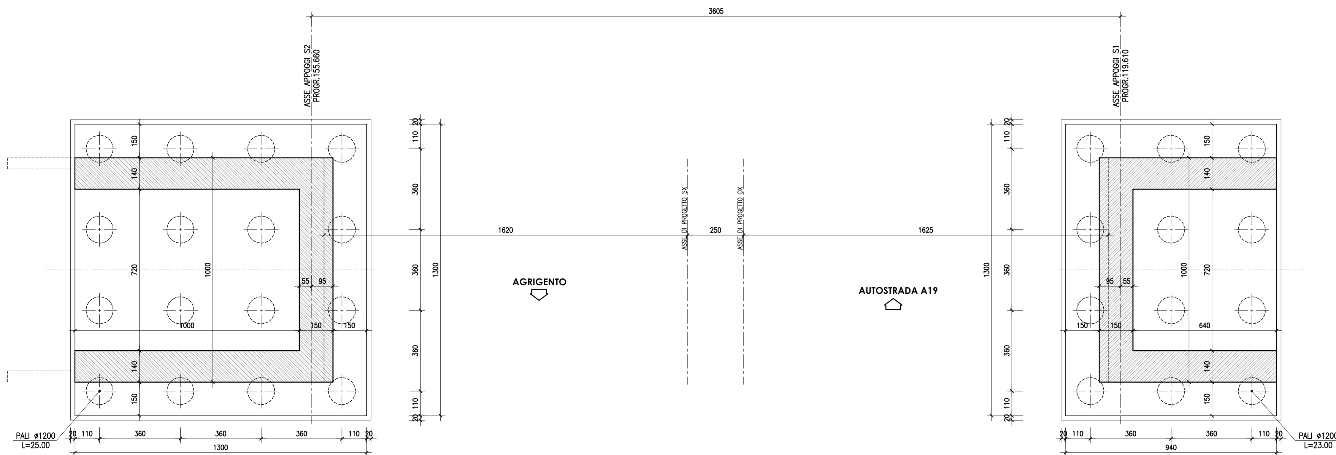
PIANTA FONDAZIONI—Scala 1:100
