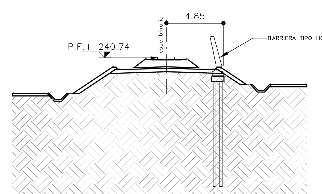
SEZIONE BB SCALA 1 : 200
