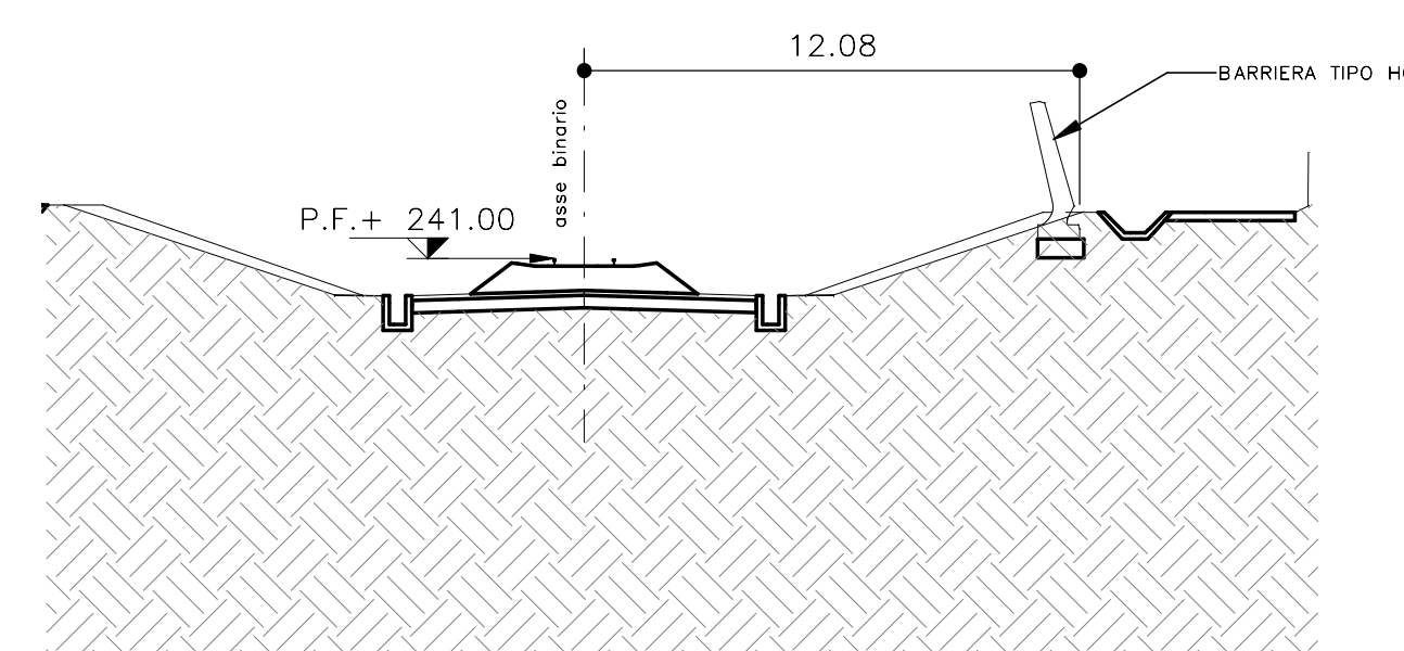
SEZIONE AA SCALA 1 : 200
