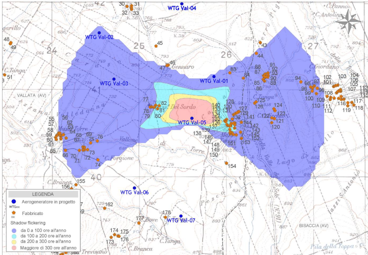
Figura 6 - Mappa di impatto potenziale per l'aerogeneratore WTG Val-05
