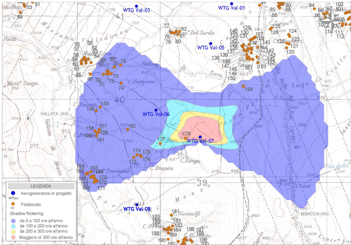
Figura 8 - Mappa di impatto potenziale per l'aerogeneratore WTG Val-07
