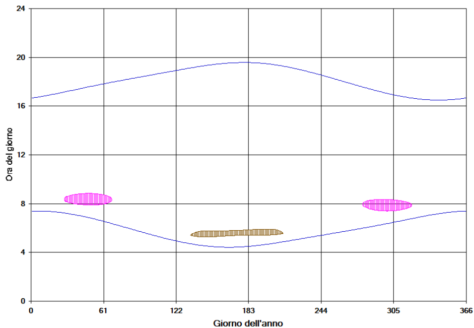
Figura 20 – Calendario dell’ombra nelle condizioni caso peggiore per il fabbricato 167
