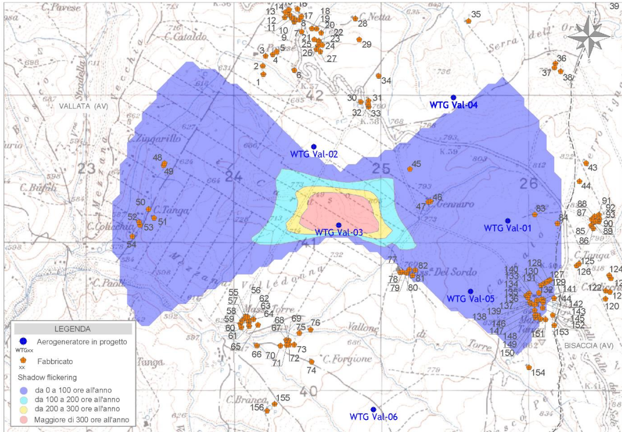
Figura 4 - Mappa di impatto potenziale per l'aerogeneratore WTG Val-03
