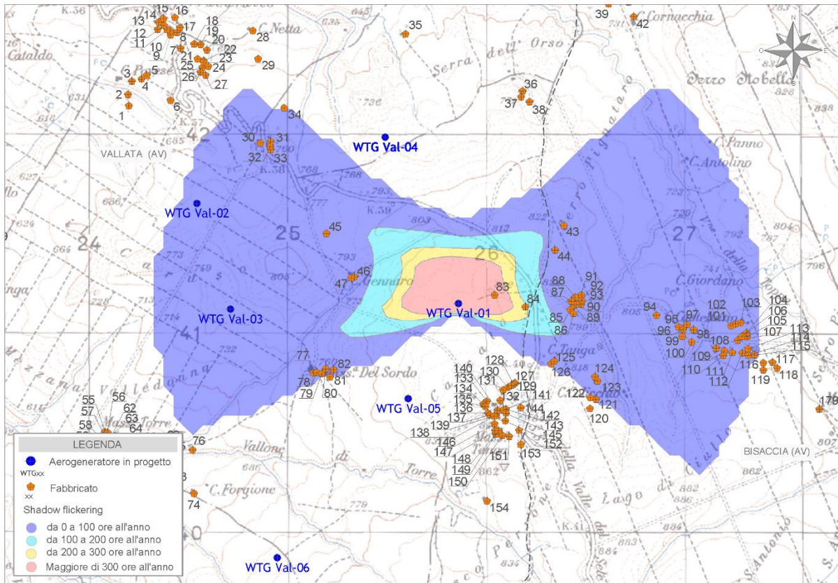
Figura 2 - Mappa di impatto potenziale per l'aerogeneratore WTG Val-01
