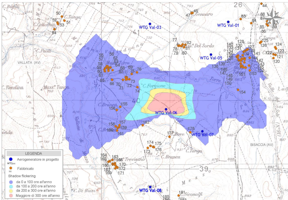
Figura 7 - Mappa di impatto potenziale per l'aerogeneratore WTG Val-06
