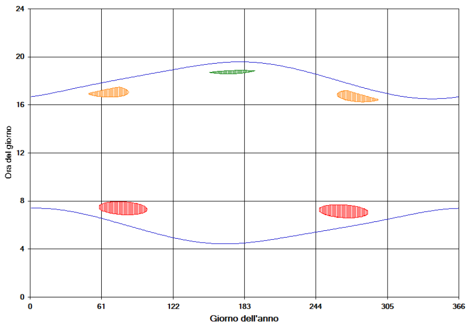
Figura 12 – Calendario dell'ombra nelle condizioni caso peggiore per il fabbricato 47
