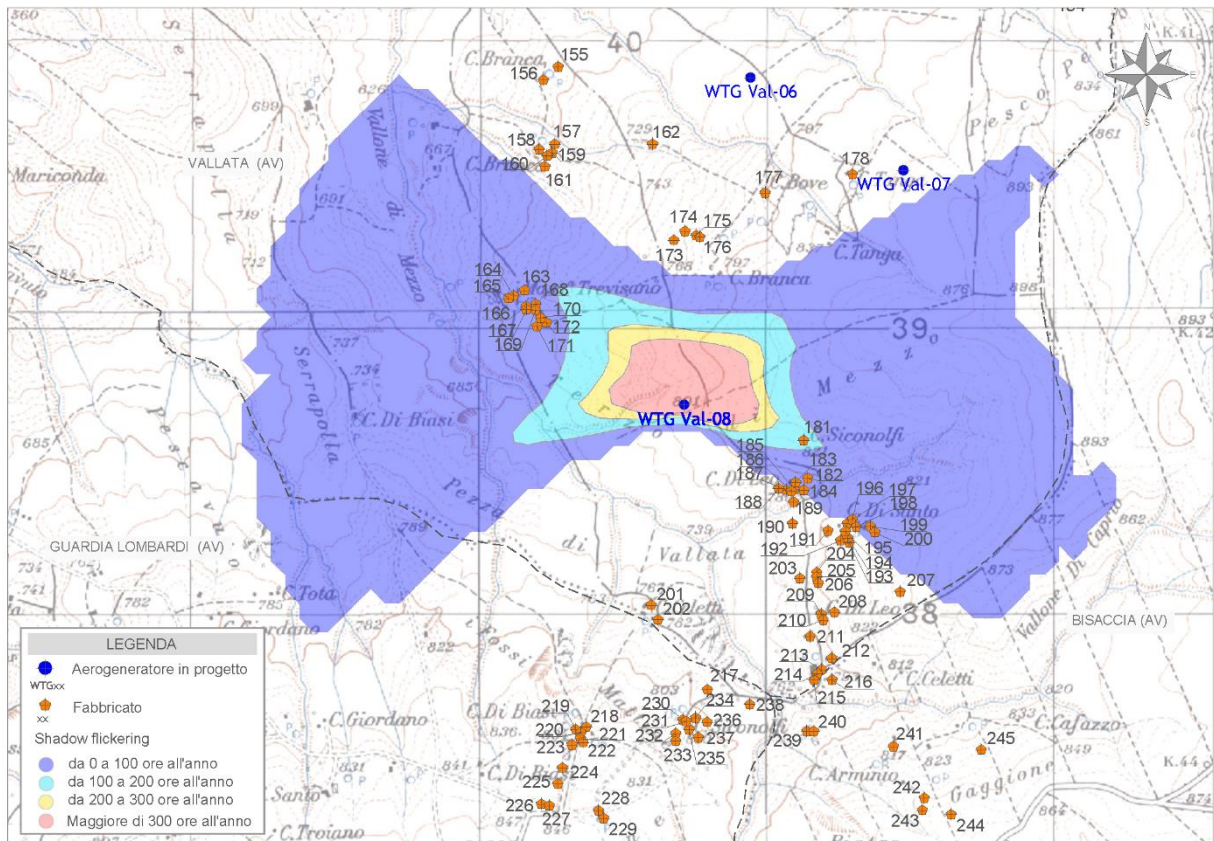
Figura 9 - Mappa di impatto potenziale per l'aerogeneratore WTG Val-08
