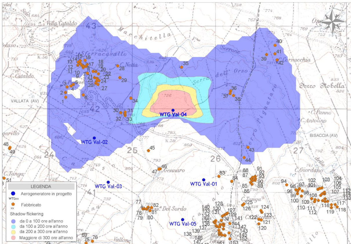
Figura 5 - Mappa di impatto potenziale per l'aerogeneratore WTG Val-04
