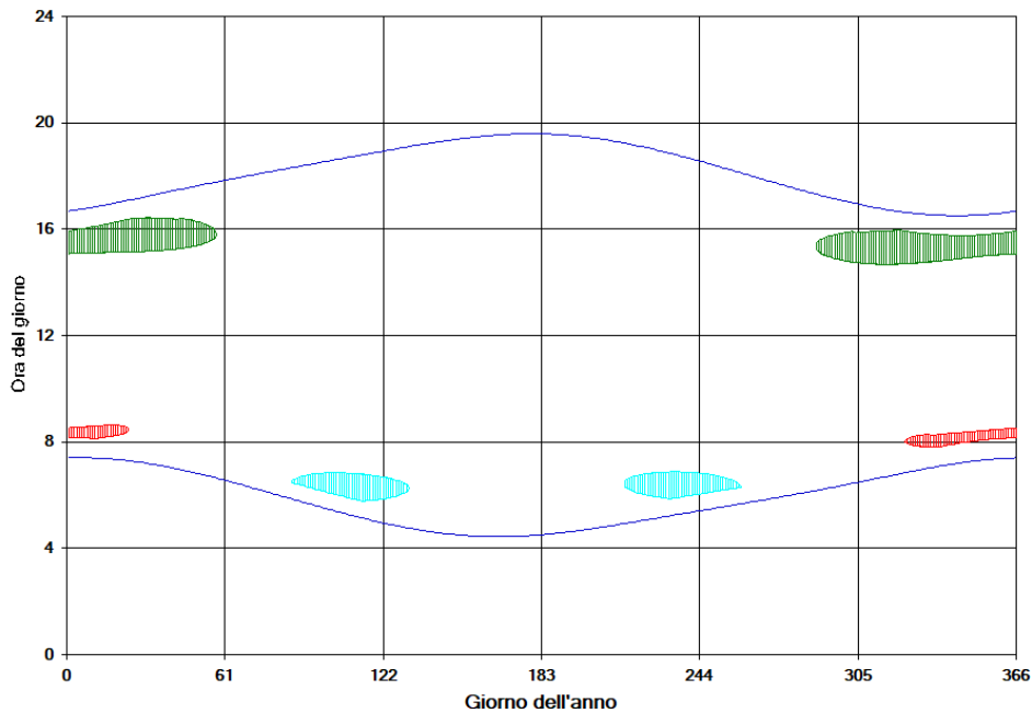
Figura 10 – Calendario dell'ombra nelle condizioni caso peggiore per il fabbricato 32
