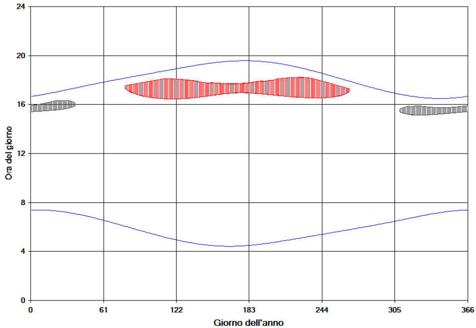
Figura 16 – Calendario dell'ombra nelle condizioni caso peggiore per il fabbricato 84
