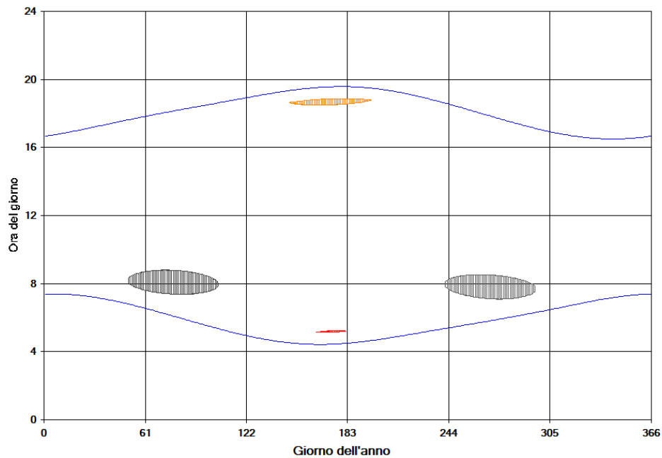
Figura 15 – Calendario dell'ombra nelle condizioni caso peggiore per il fabbricato 82
