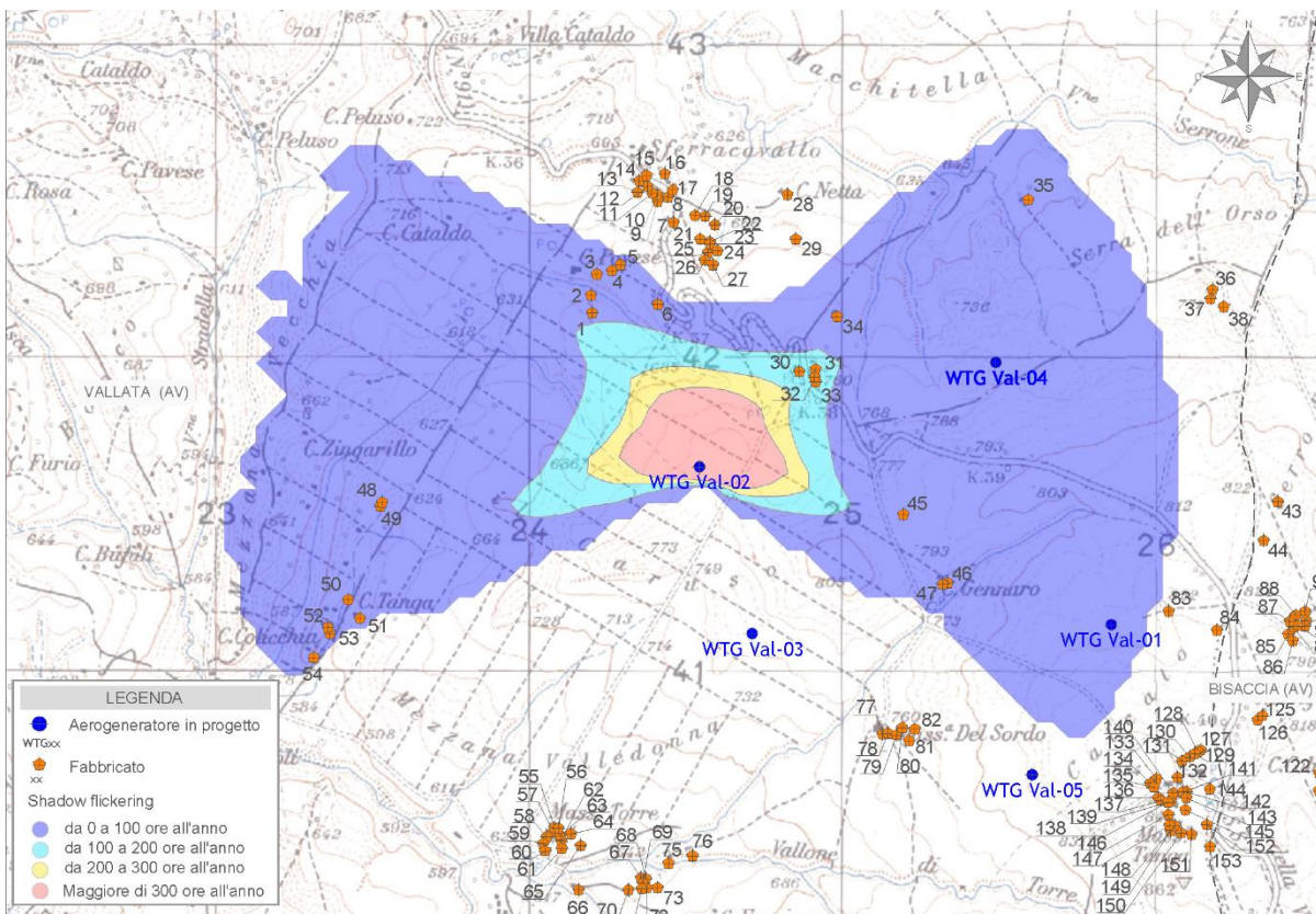
Figura 3 - Mappa di impatto potenziale per l'aerogeneratore WTG Val-02
