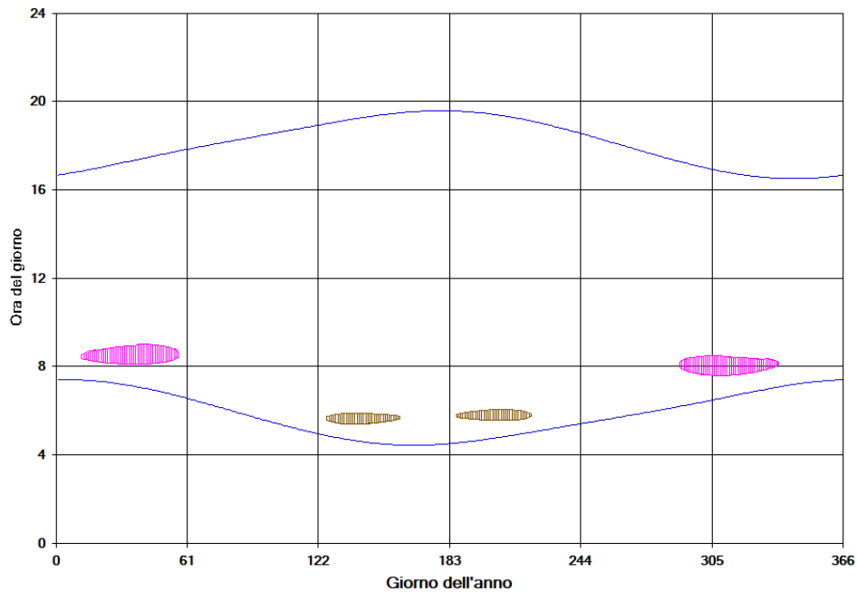
Figura 18 – Calendario dell'ombra nelle condizioni caso peggiore per il fabbricato 163
