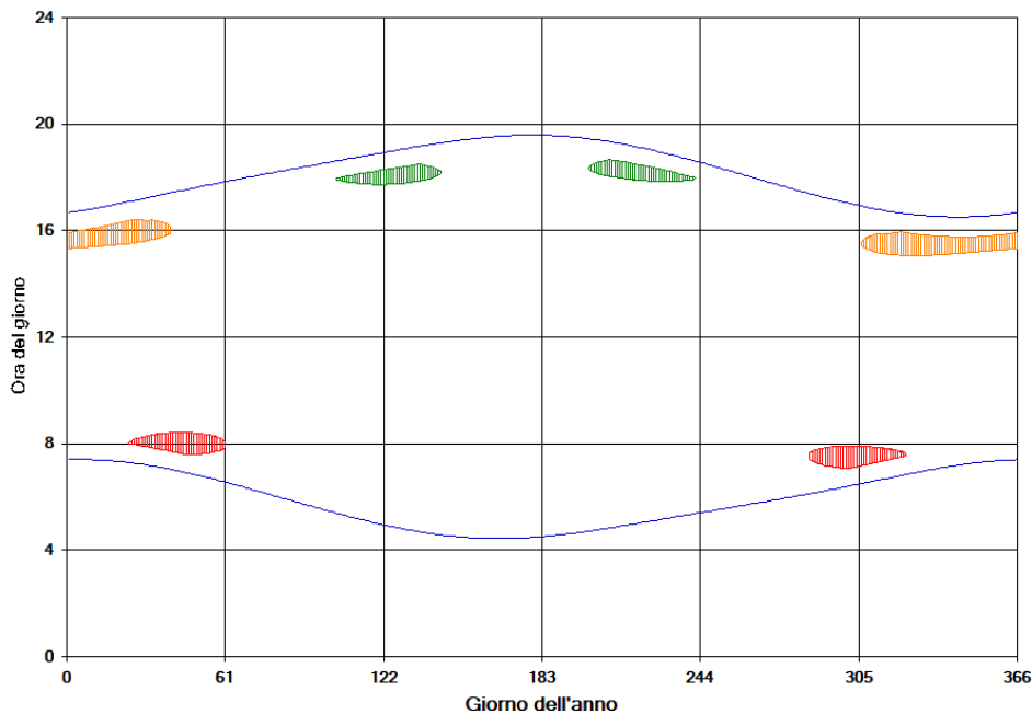
Figura 11 – Calendario dell'ombra nelle condizioni caso peggiore per il fabbricato 45
