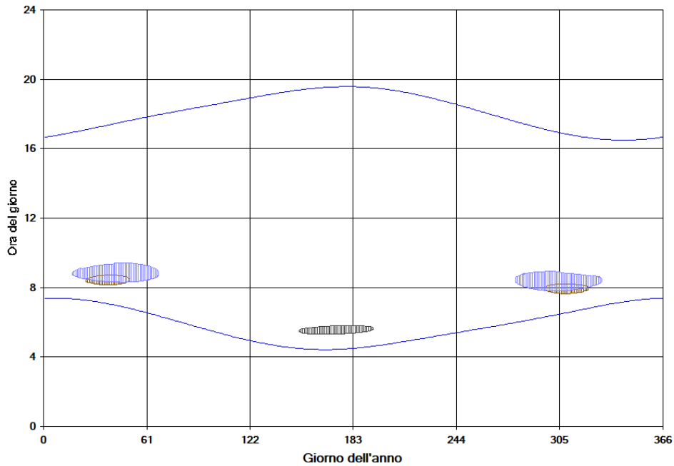
Figura 14 – Calendario dell'ombra nelle condizioni caso peggiore per il fabbricato 74
