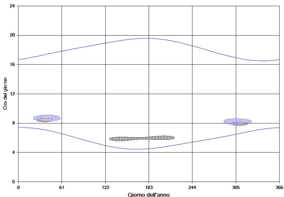
Figura 13 – Calendario dell'ombra nelle condizioni caso peggiore per il fabbricato 71
