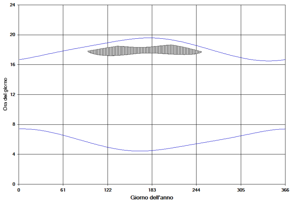
Figura 17 – Calendario dell'ombra nelle condizioni caso peggiore per il fabbricato 138
