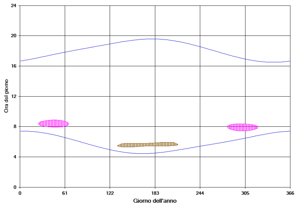
Figura 19 – Calendario dell'ombra nelle condizioni caso peggiore per il fabbricato 166
