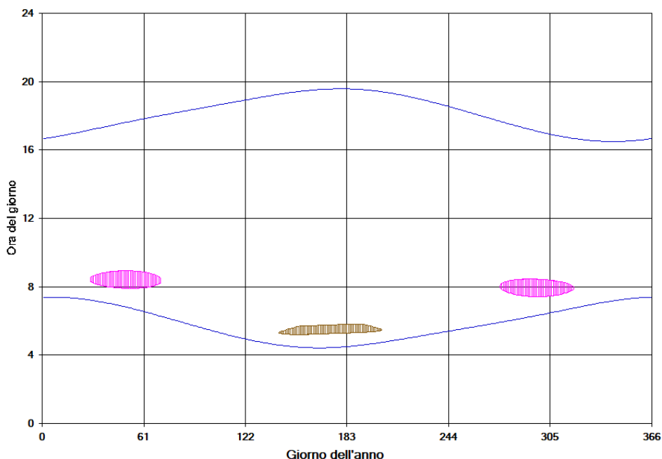
Figura 21 – Calendario dell’ombra nelle condizioni caso peggiore per il fabbricato 170
