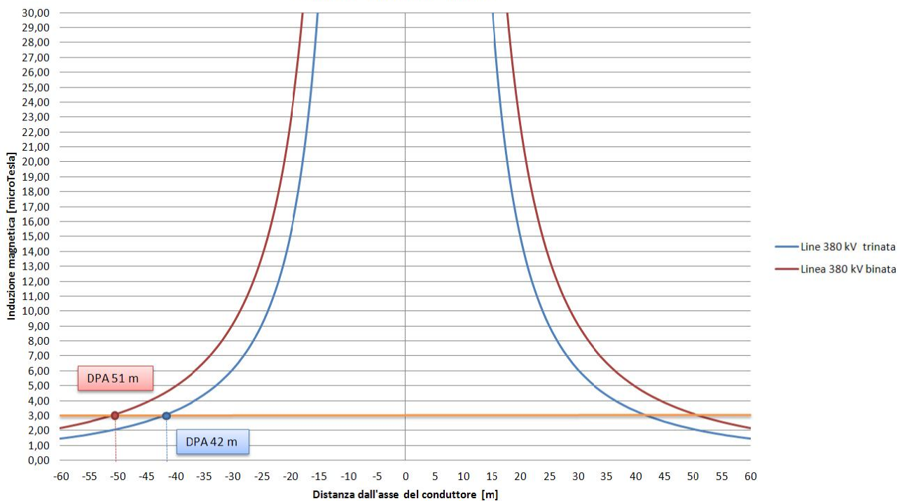
DPA linea 380 kV binata e trinata
