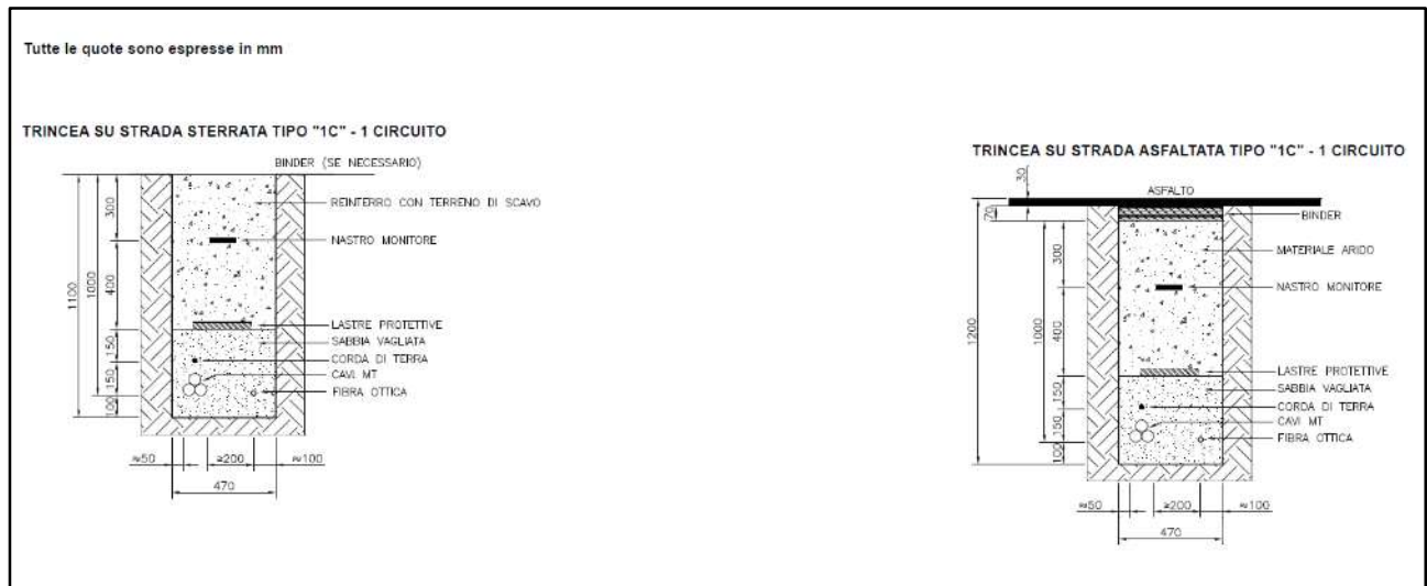
Figura 2.3.3.2: Sezioni tipiche delle trincee cavidotto per una terna di cavi in parallelo su strada sterrata e asphaltata
