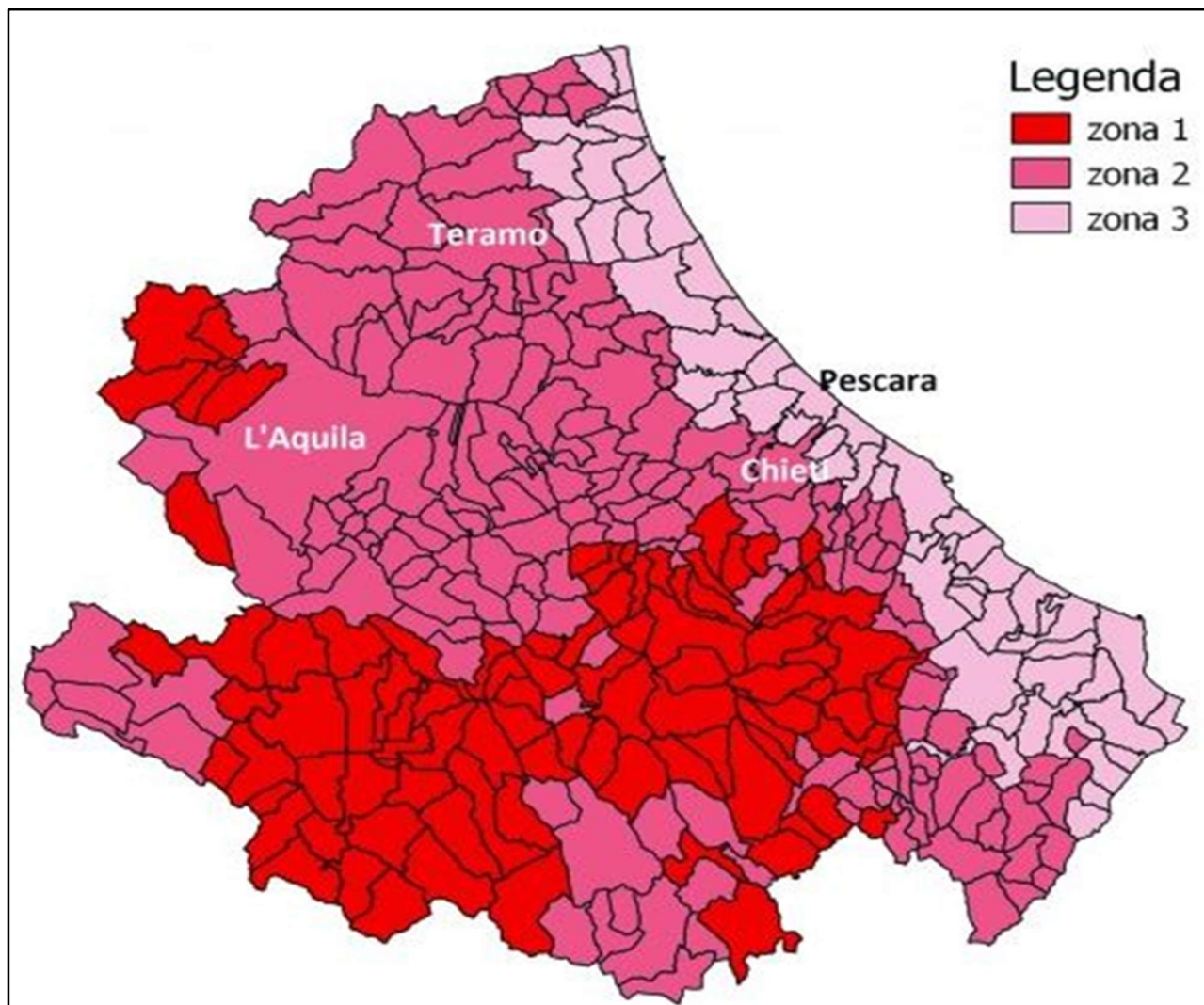
Figura 8.3.1: Regione Abruzzo - Mappa delle zone sismiche
