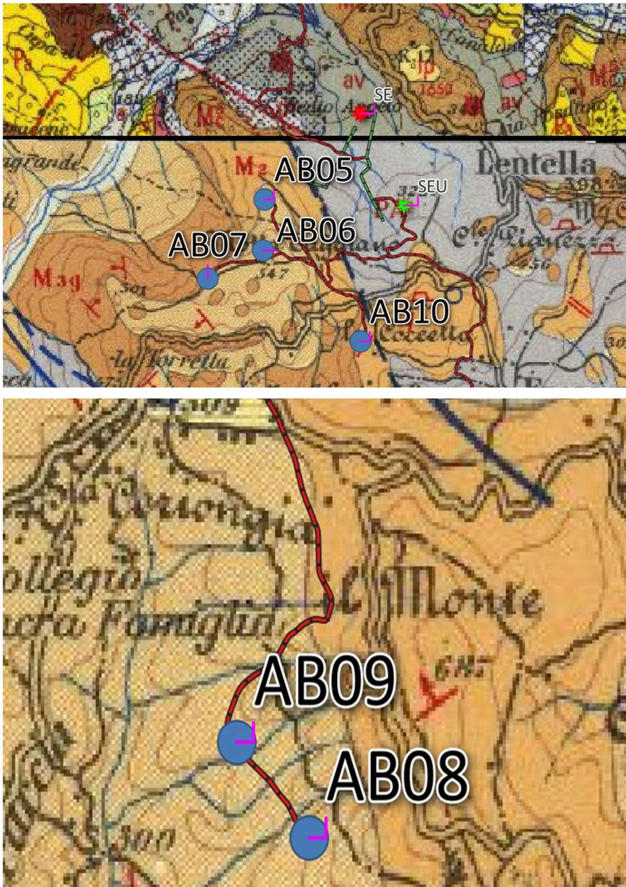
Figura 8.2.3: Carta geologica d'Italia Fg. 148 e Fg. 154
