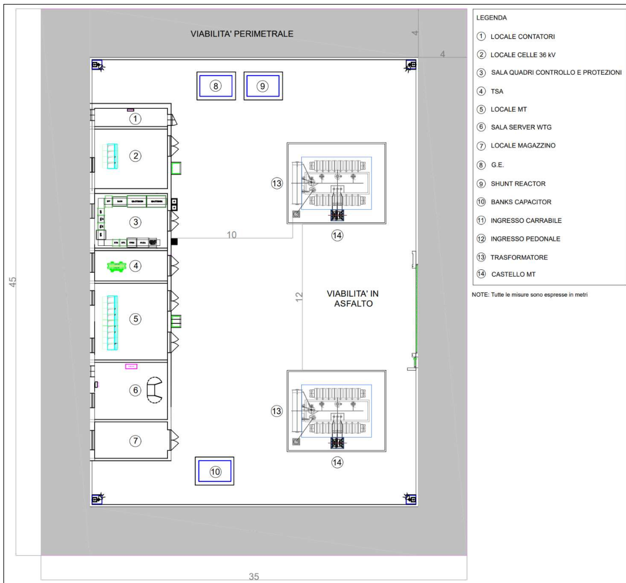
Figura 6.3.2.1: Planimetria elettromeccanica della Stazione Elettrica Utente 36/33 kV
