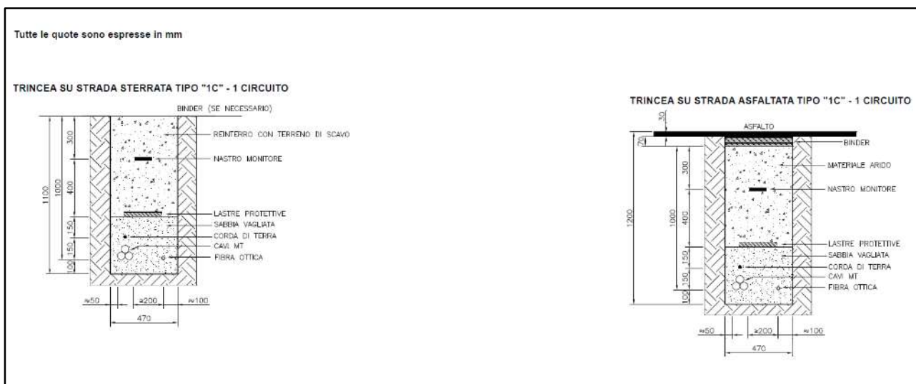
Figura 6.3.3.2: Sezioni tipiche delle trincee cavidotto per una trincea di cavi in parallelo su strada sterrata e asfaltata
