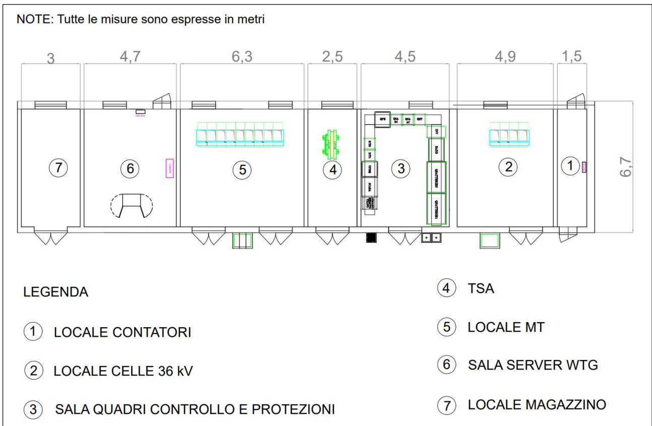
Figura 6.3.2.2: Pianta edificio di controllo SEU 36/33 kV
