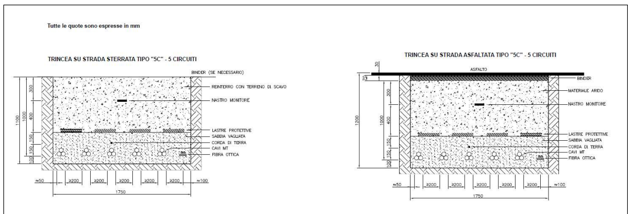
Figura 6.3.3.6: Sezioni tipiche delle trincee cavidotto per cinque terne di cavi in parallelo su strada sterrata e asfaltata
