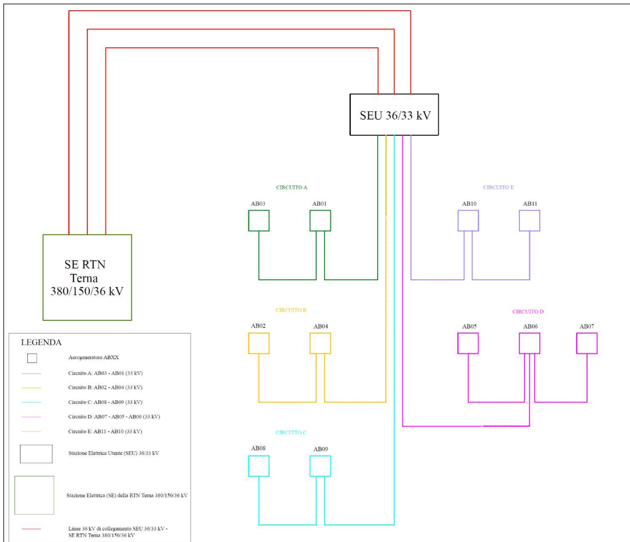
Figura 6.3.3.1: Schema a blocchi del Parco Eolico Abruzzo
