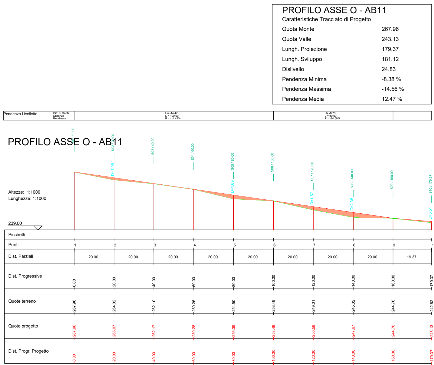
PLANIMETRIA PIAZZOLA AB011 E PROFILO O-AB011 SU CURVE DI LIVELLO_SCALE 1:1.000
