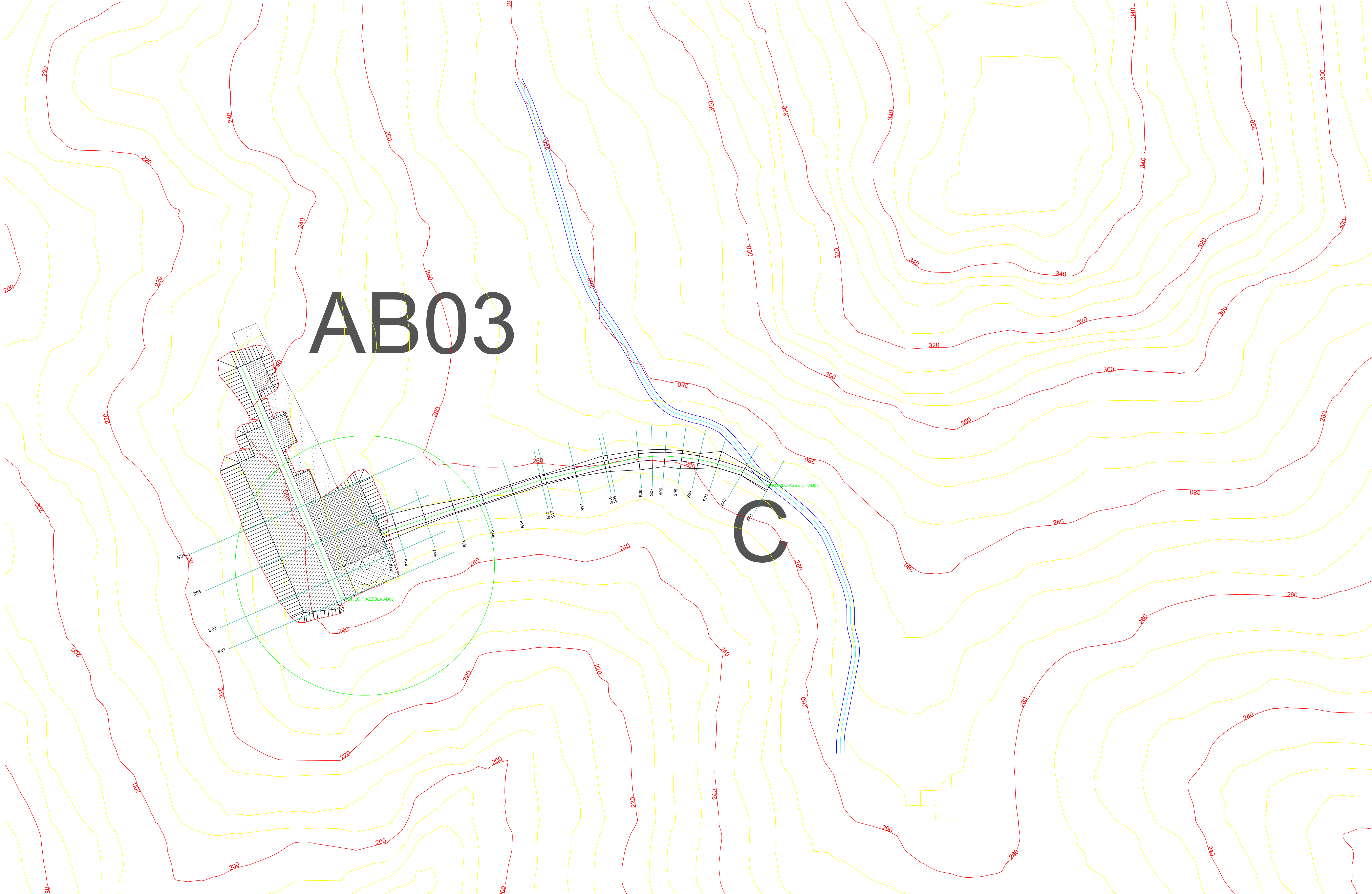
PLANIMETRIA PIAZZOLA AB03 E PROFILO C-AB03 SU CURVE DI LIVELLO_SALA 1:1.000
