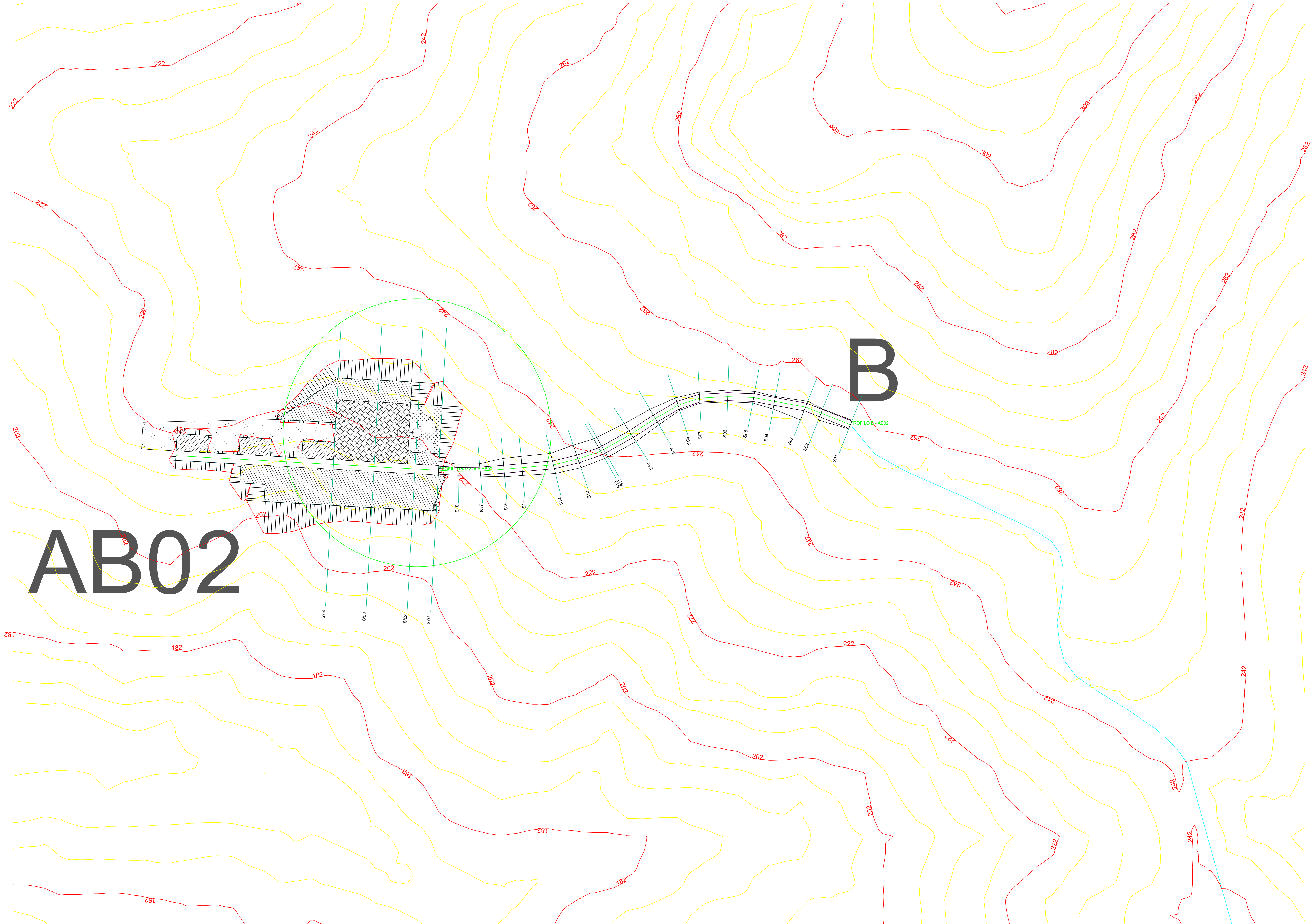
PLANIMETRIA PIAZZOLA AB02 E PROFILO B-AB02 SU CURVE DI LIVELLO_SCALE 1:1.000
