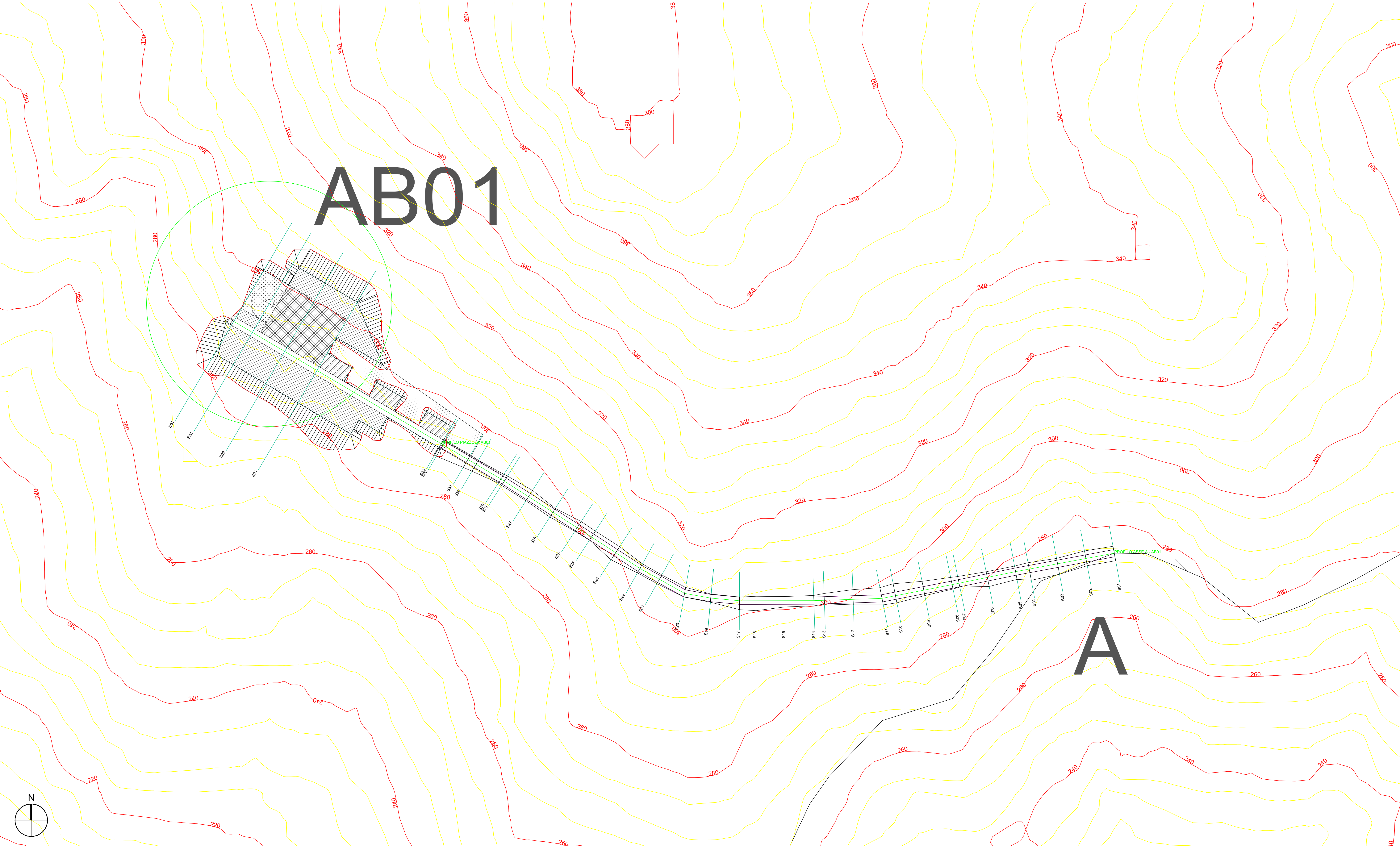
PLANIMETRIA PIAZZOLA AB01 E PROFILO A-AB01 SU CURVE DI LIVELLO_SCALE 1:1.000
