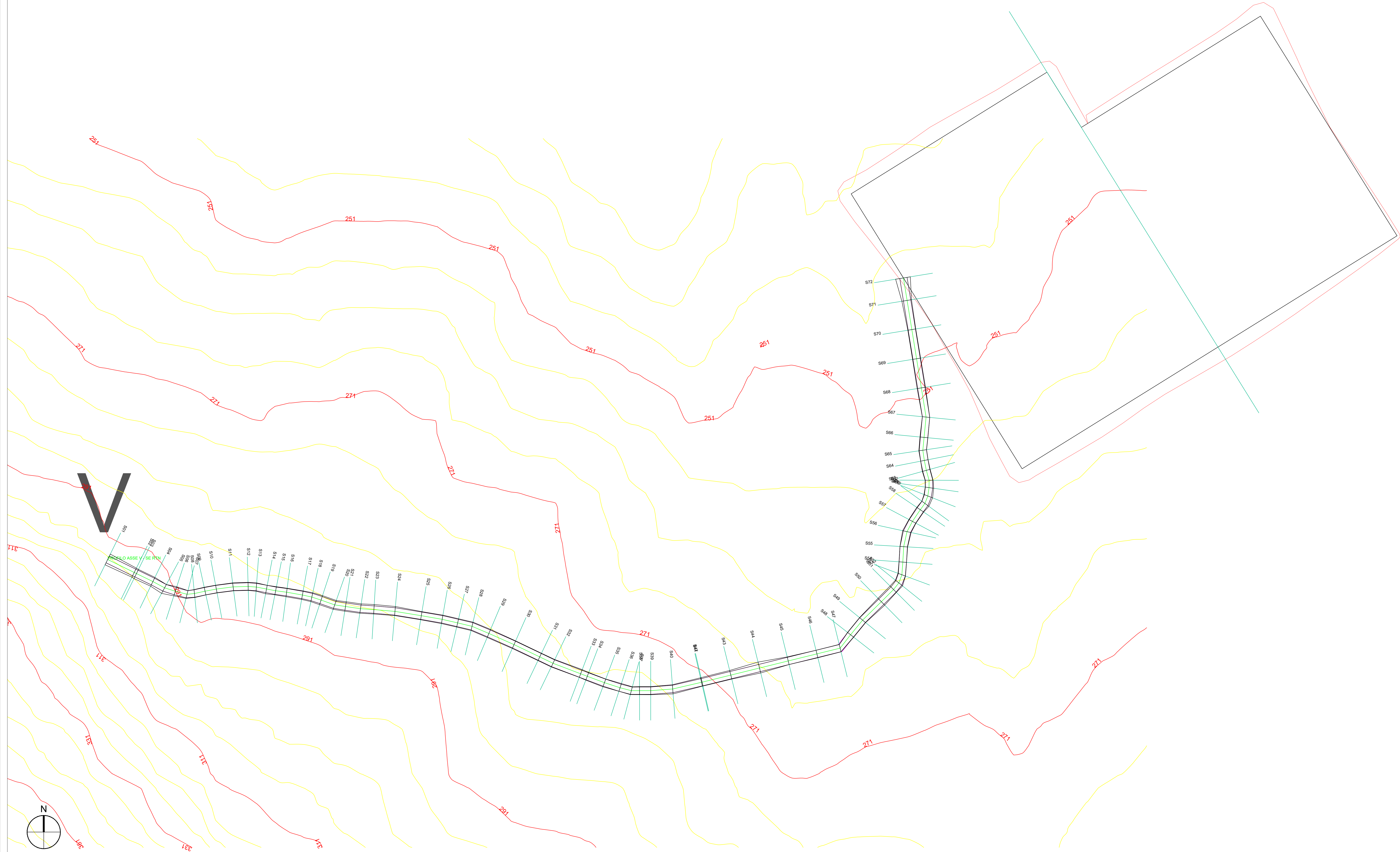
PLANIMETRIA PROFILO VIABILITA' RTN SU CURVE DI LIVELLO_SCALE 1:1.000
