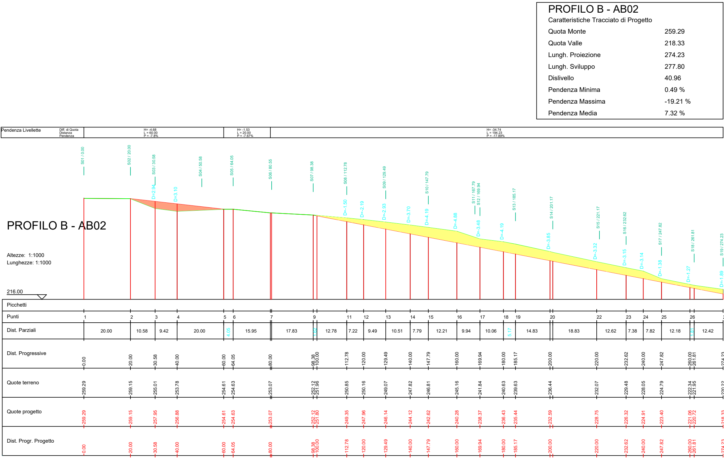
PLANIMETRIA PIAZZOLA AB02 E PROFILO B-AB02 SU CURVE DI LIVELLO_SCALE 1:1.000
