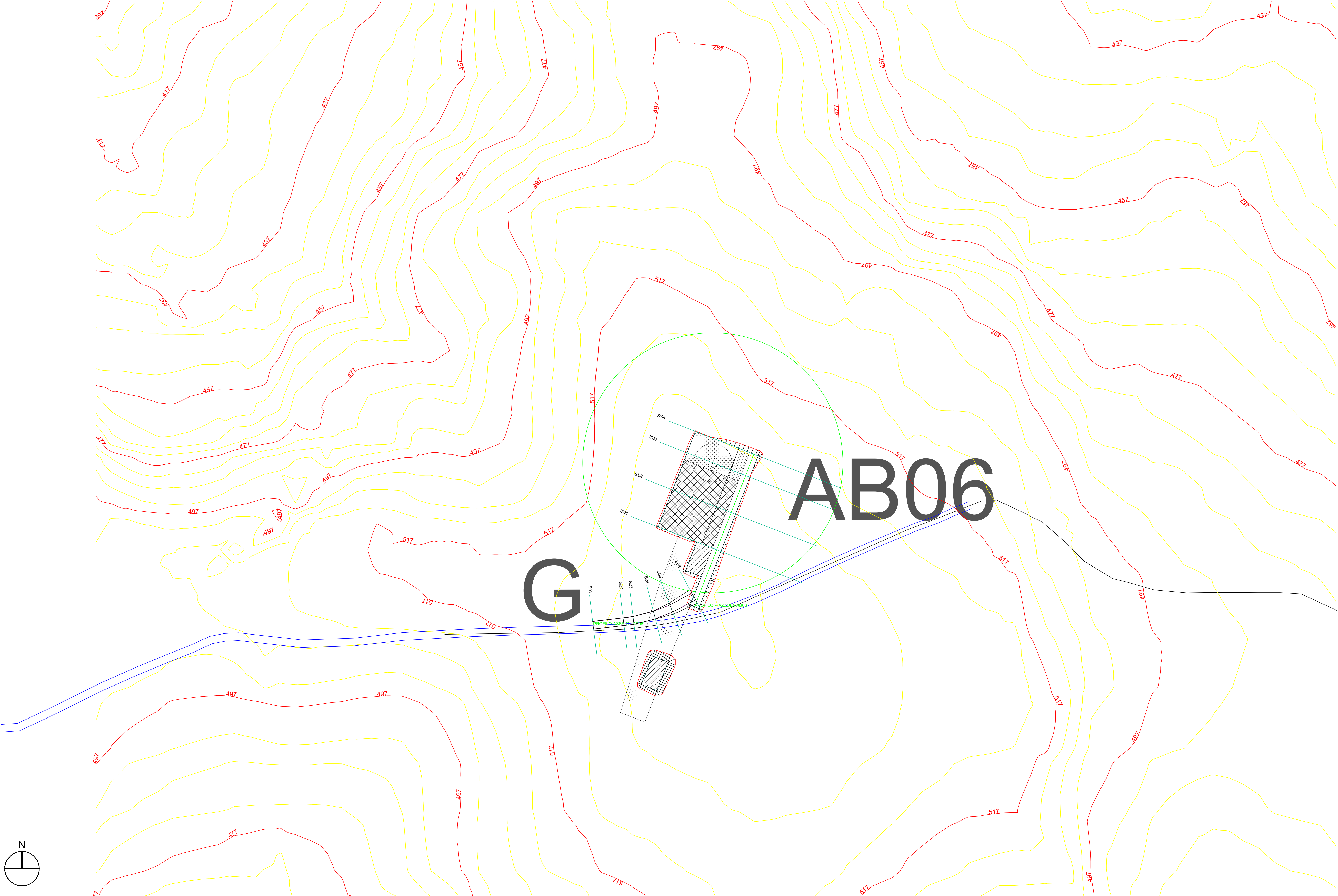
PLANIMETRIA PIAZZOLA AB06 E PROFILO G-AB06 SU CURVE DI LIVELLO_SCALE 1:1.000
