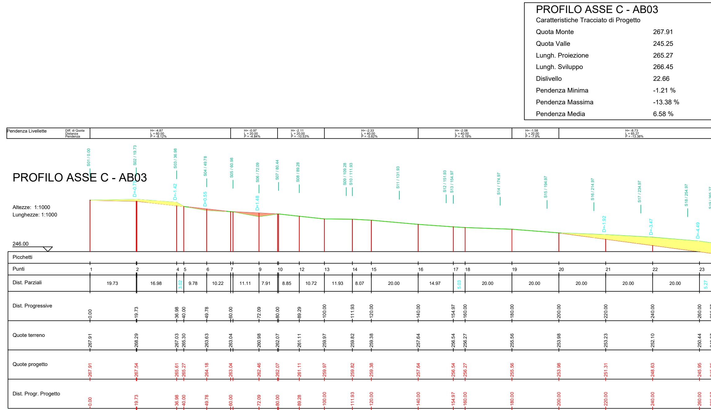
PLANIMETRIA PIAZZOLA AB03 E PROFILO C-AB03 SU CURVE DI LIVELLO_SALA 1:1.000
