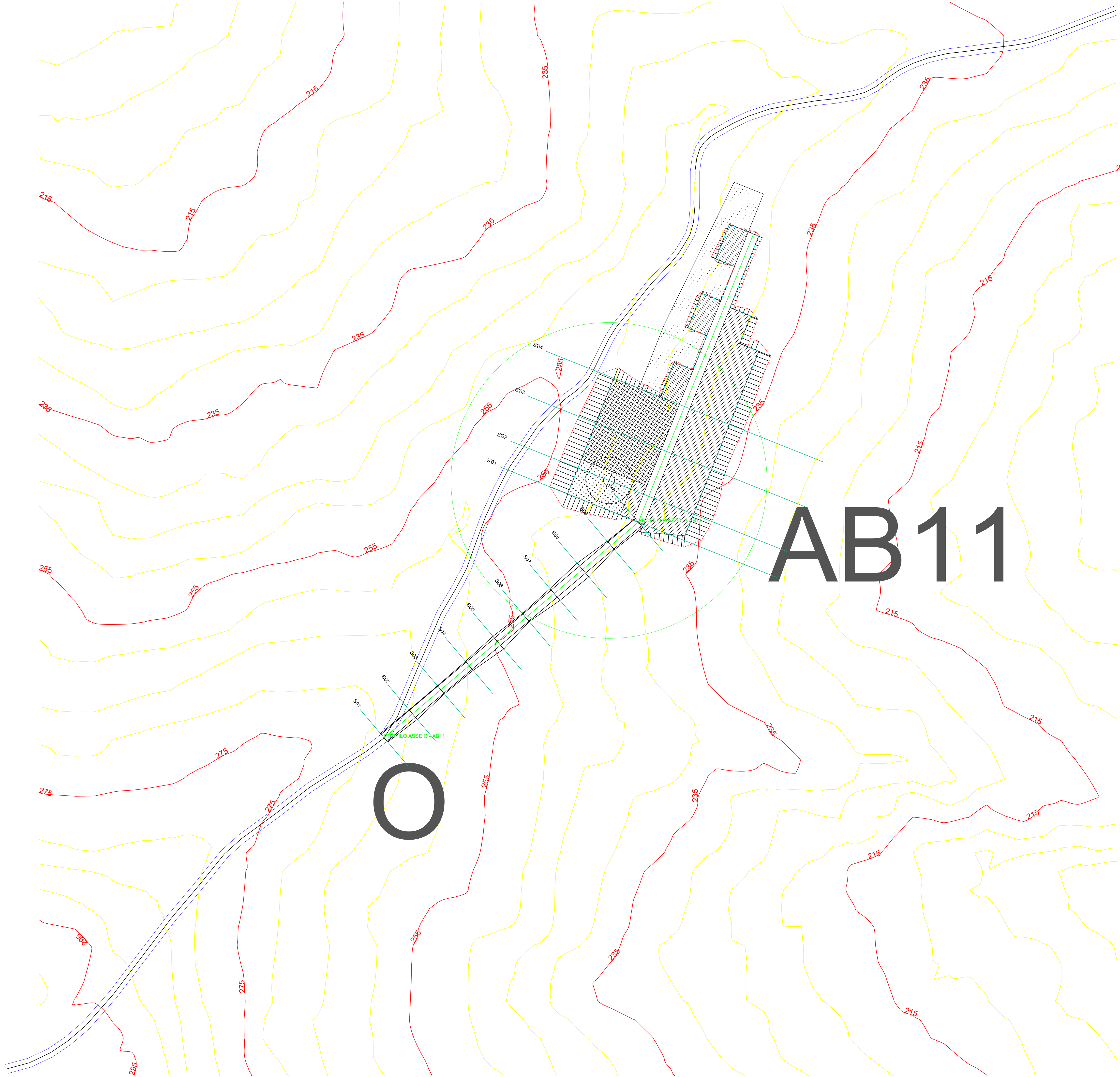
PLANIMETRIA PIAZZOLA AB011 E PROFILO O-AB011 SU CURVE DI LIVELLO_SCALE 1:1.000
