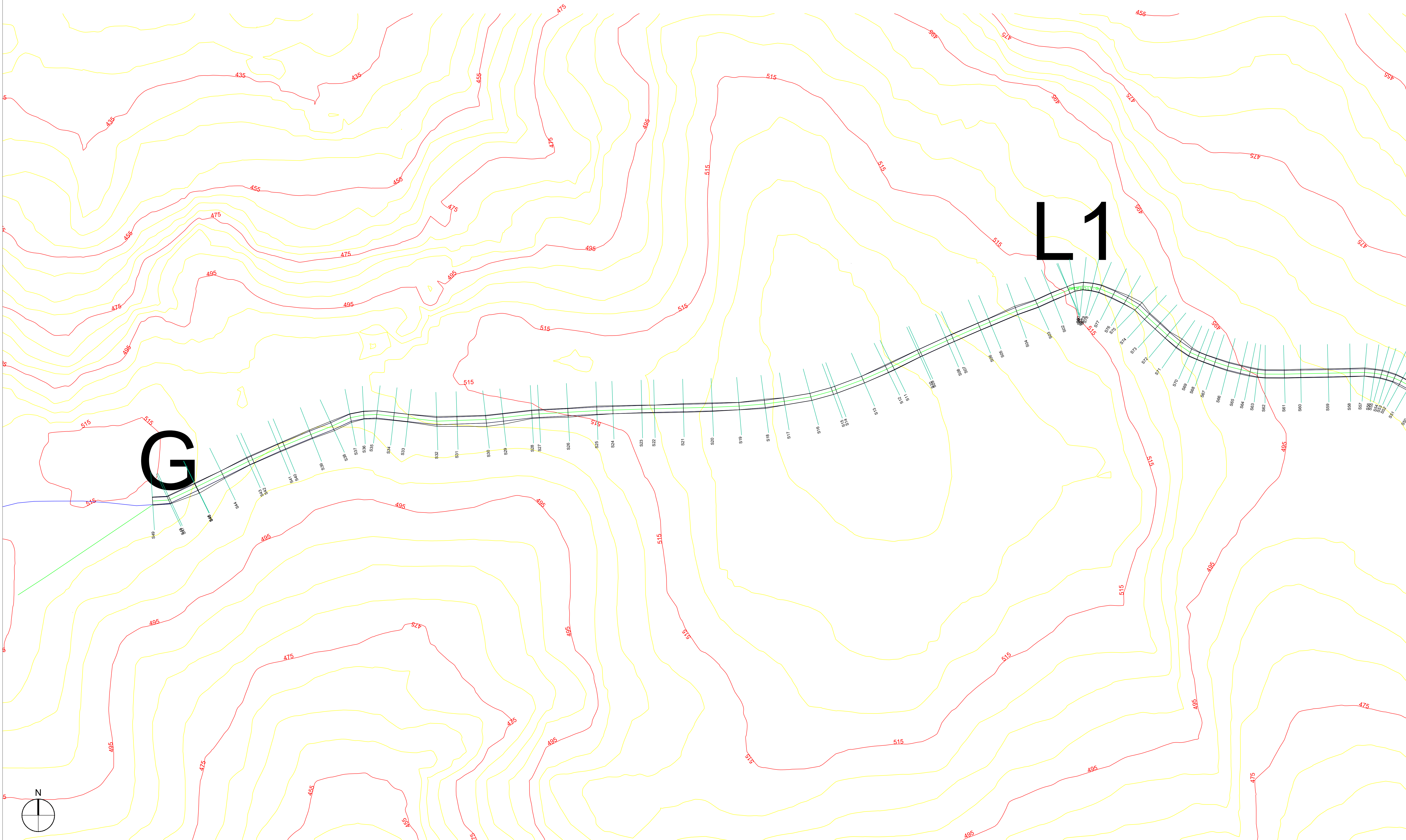
PLANIMETRIA PROFILO L1 - G SU CURVE DI LIVELLO_SCALA 1:1.000
