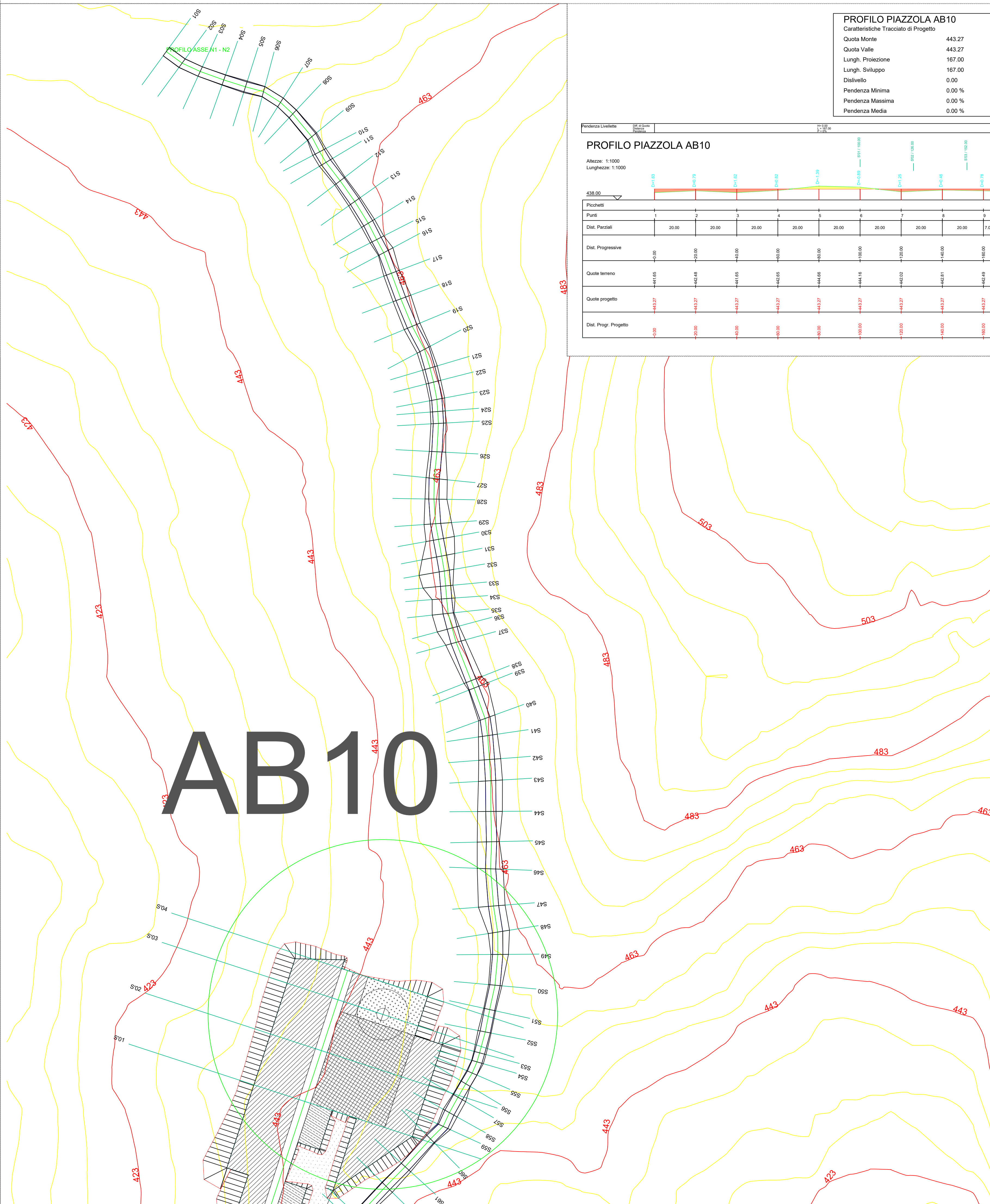
PLANIMETRIA PIAZZOLA AB10 E PROFILO N-AB010 SU CURVE DI LIVELLO, SCALA 1:1.000
