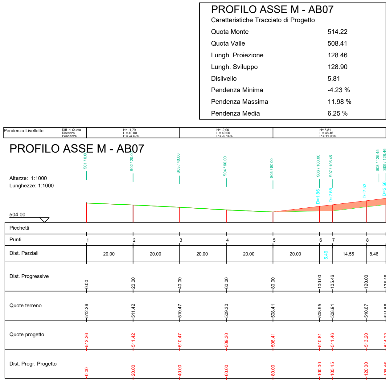
PLANIMETRIA PIAZZOLA AB07 E PROFILO M-AB07 SU CURVE DI LIVELLO_SCALE 1:1.000
