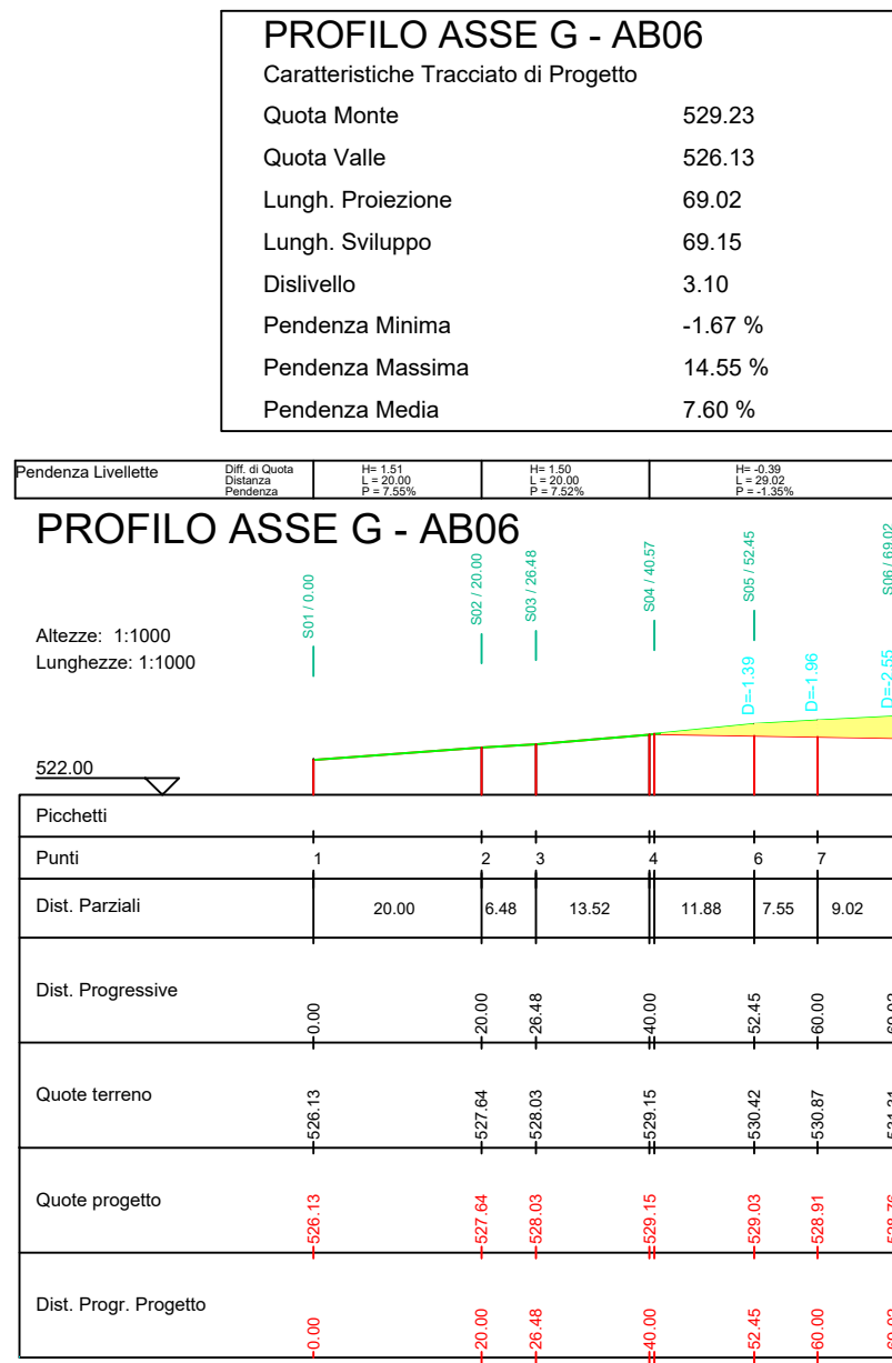
PLANIMETRIA PIAZZOLA AB06 E PROFILO G-AB06 SU CURVE DI LIVELLO_SCALE 1:1.000
