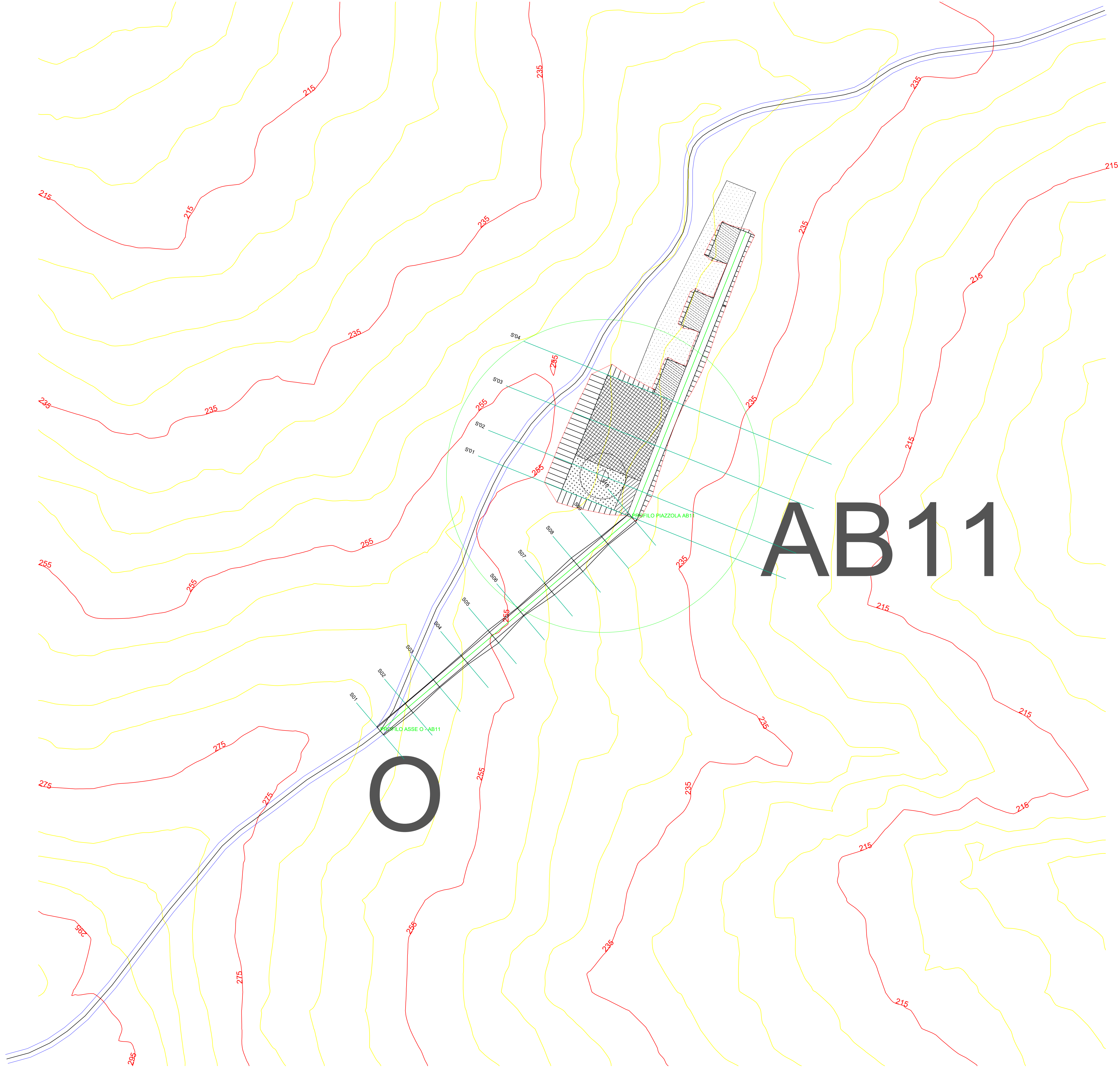
PLANIMETRIA PIAZZOLA AB011(SENZA AREA STOCCAGGIO PALE) E PROFILO O - AB011 SU CURVE DI LIVELLO_SCALE 1:1.000
