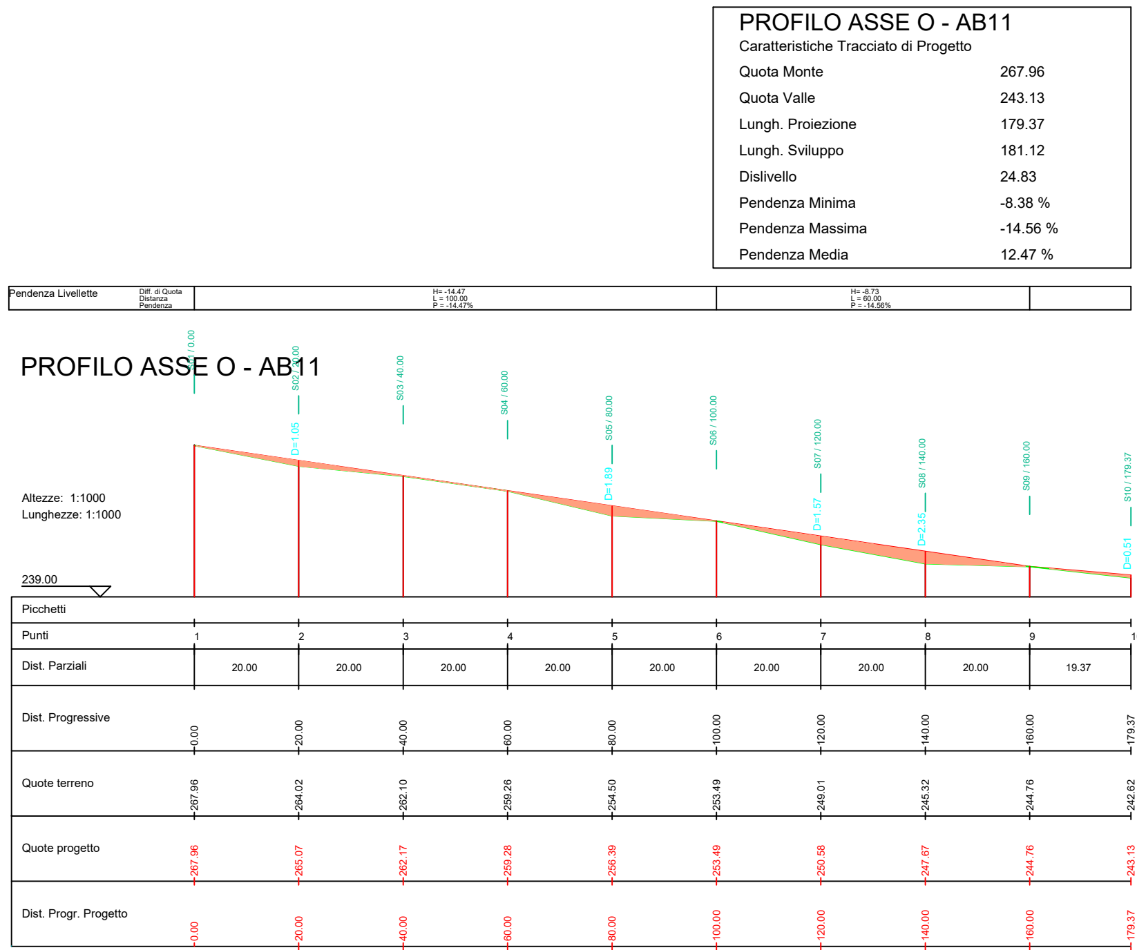
PLANIMETRIA PIAZZOLA AB011(SENZA AREA STOCCAGGIO PALE) E PROFILO O - AB011 SU CURVE DI LIVELLO_SCALE 1:1.000
