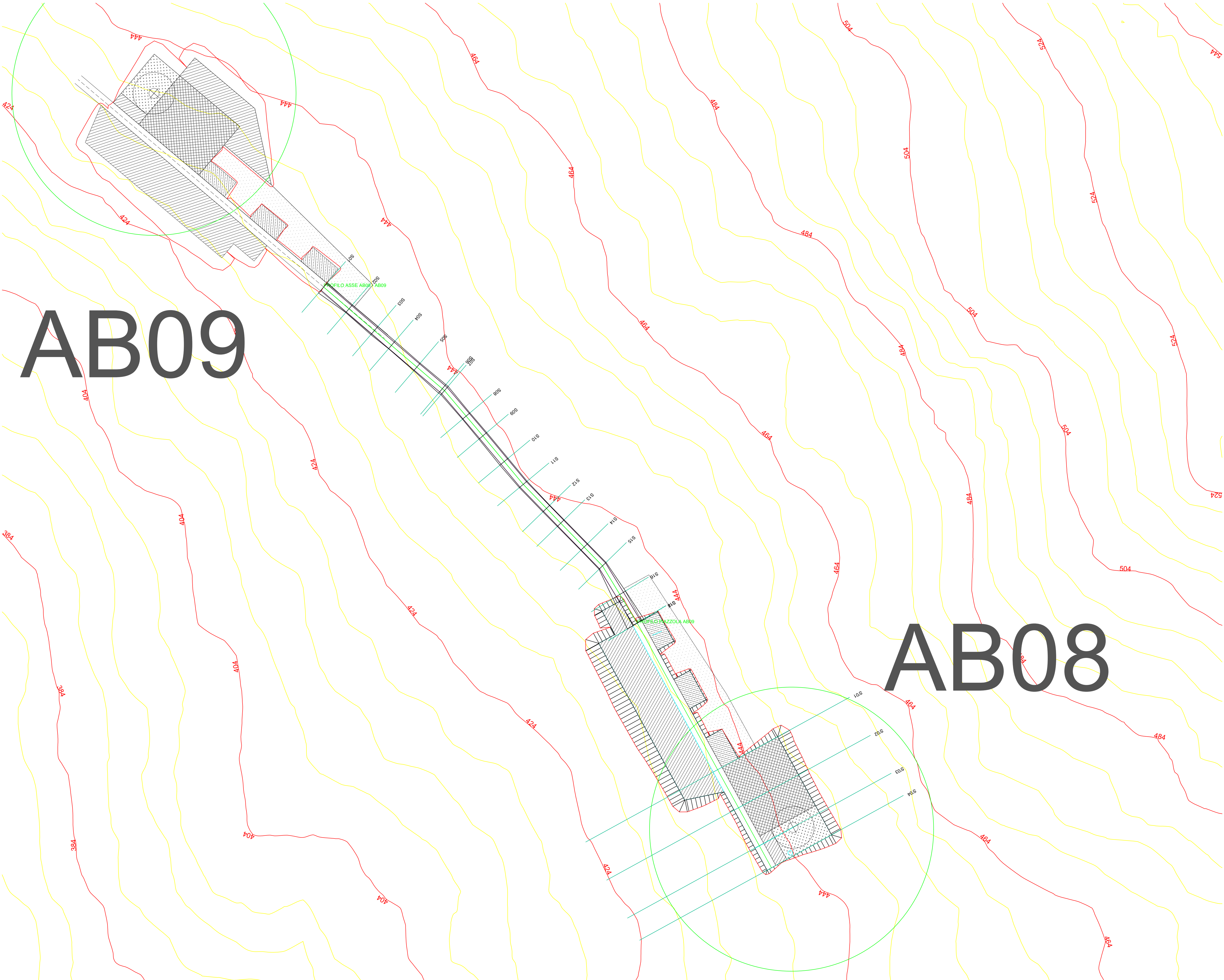
PLANIMETRIA PIAZZOLA AB08 - AB09 SU CURVE DI LIVELLO_SCALE 1:1.000
