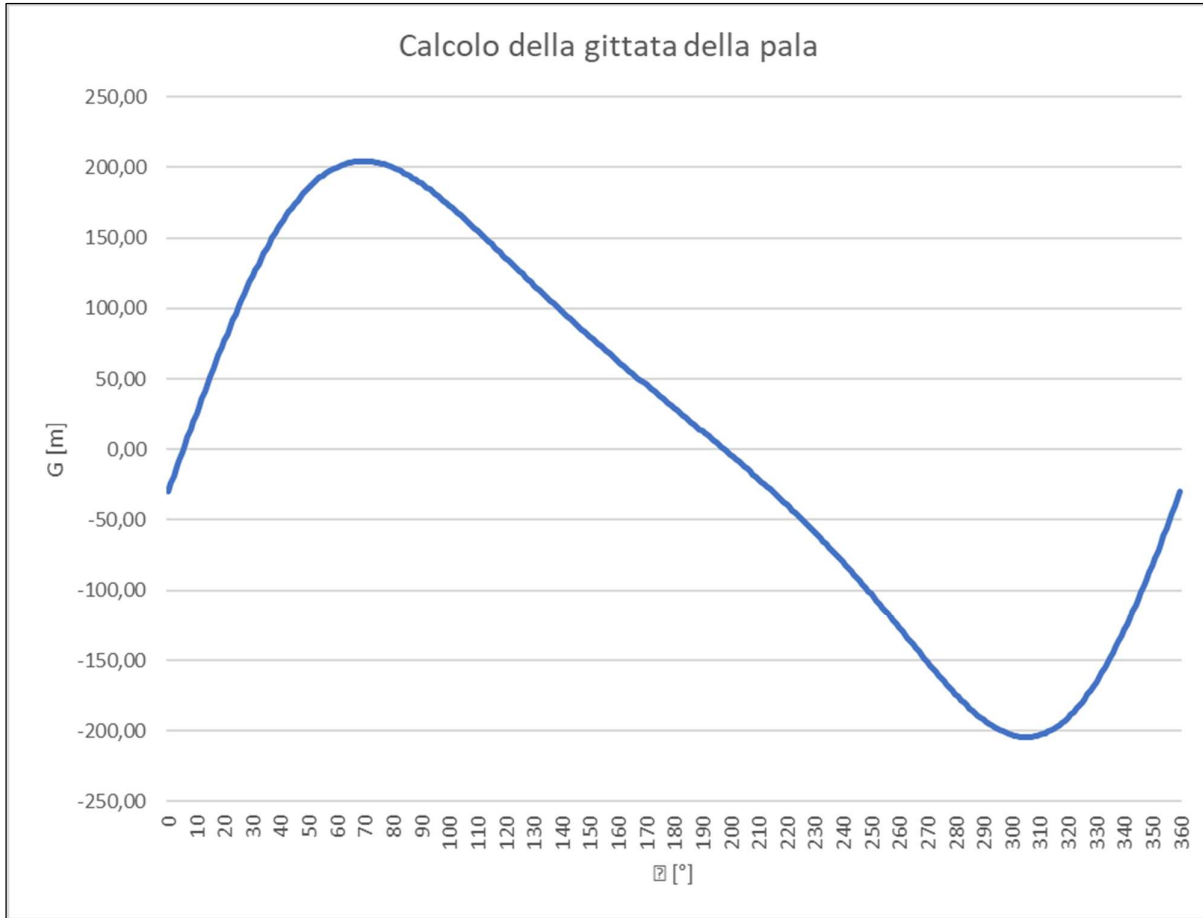
Figura 7.2: Rappresentazione grafica della gittata della pala
