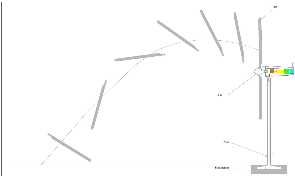
Figura 5.1: Traiettoria teorica pala in caso di rottura
