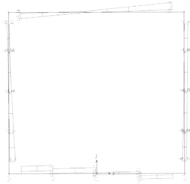
Figura 8 - Inv_TA – Diagramma del taglio
