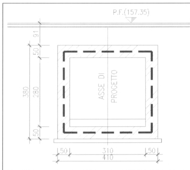
Figura 2 – Sezione trasversale
