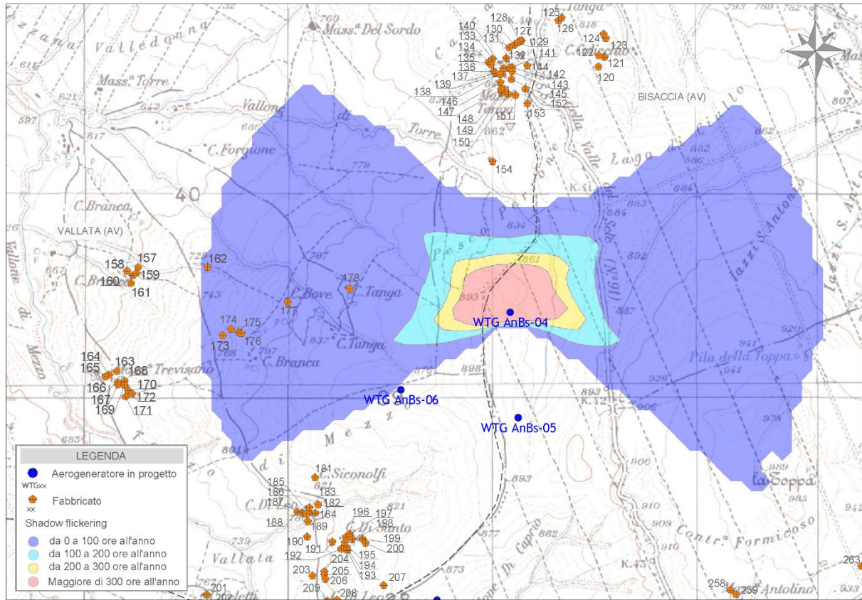
Figura 5 - Mappa di impatto potenziale per l'aerogeneratore WTG AnBs-04
