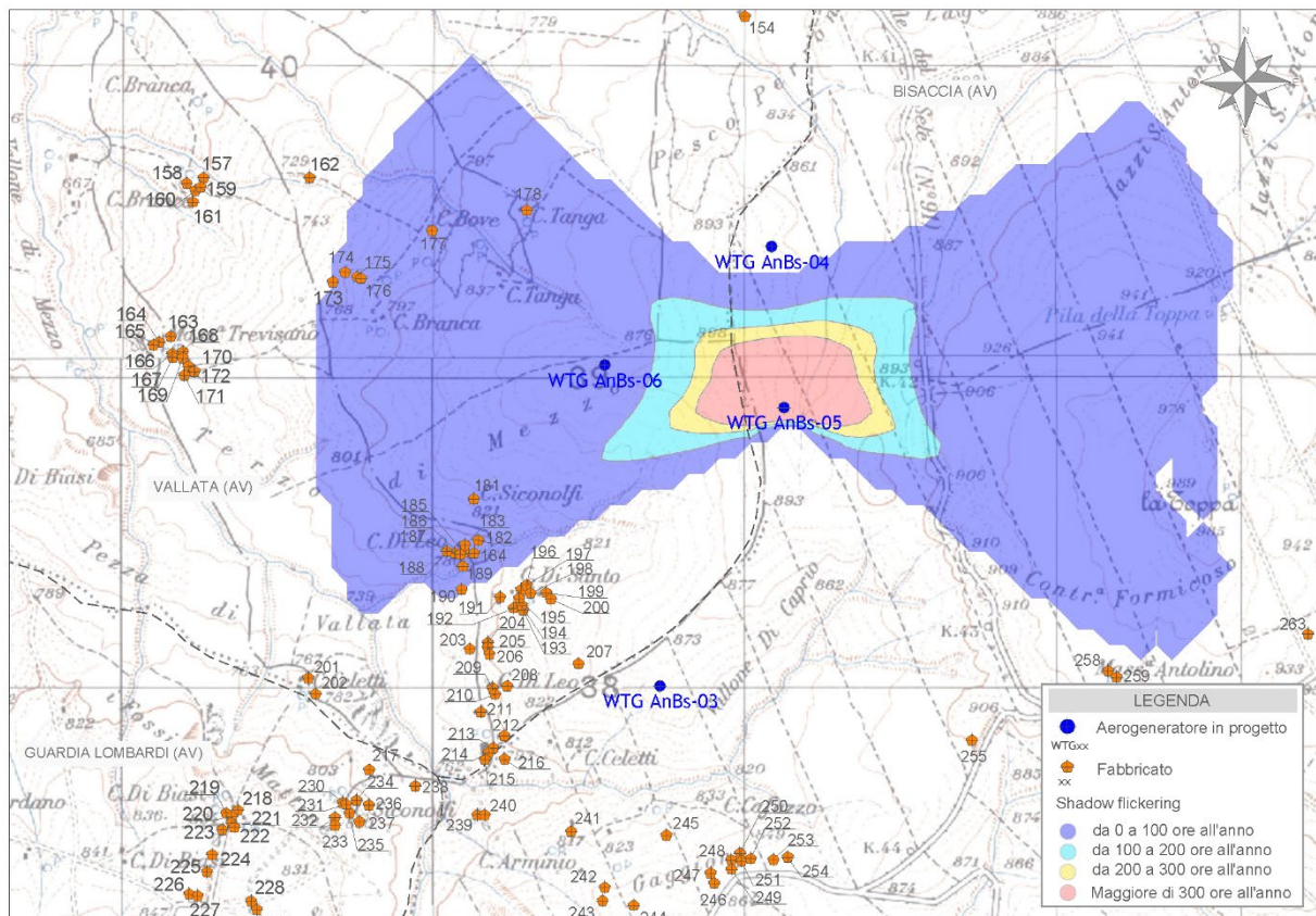
Figura 6 - Mappa di impatto potenziale per l'aerogeneratore WTG AnBs-05
