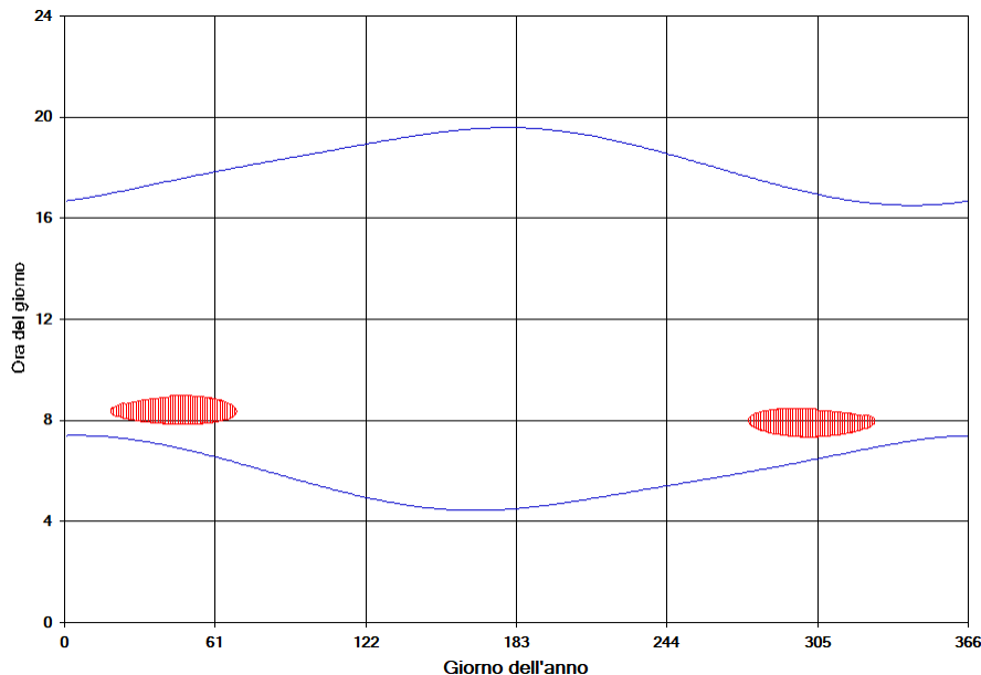
Figura 22 – Calendario dell'ombra nelle condizioni caso peggiore per il fabbricato 195
