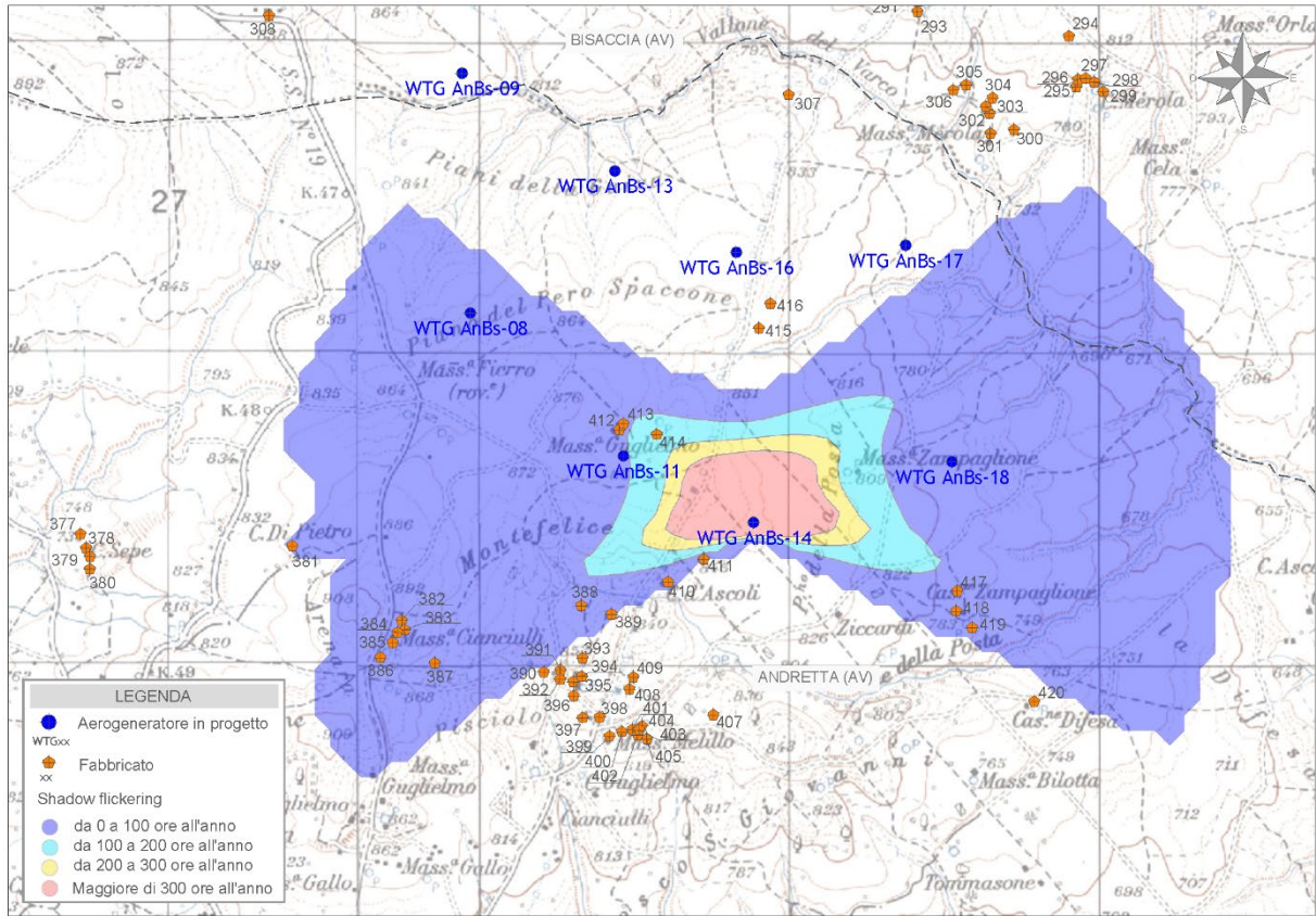
Figura 15 - Mappa di impatto potenziale per l'aerogeneratore WTG AnBs-14
