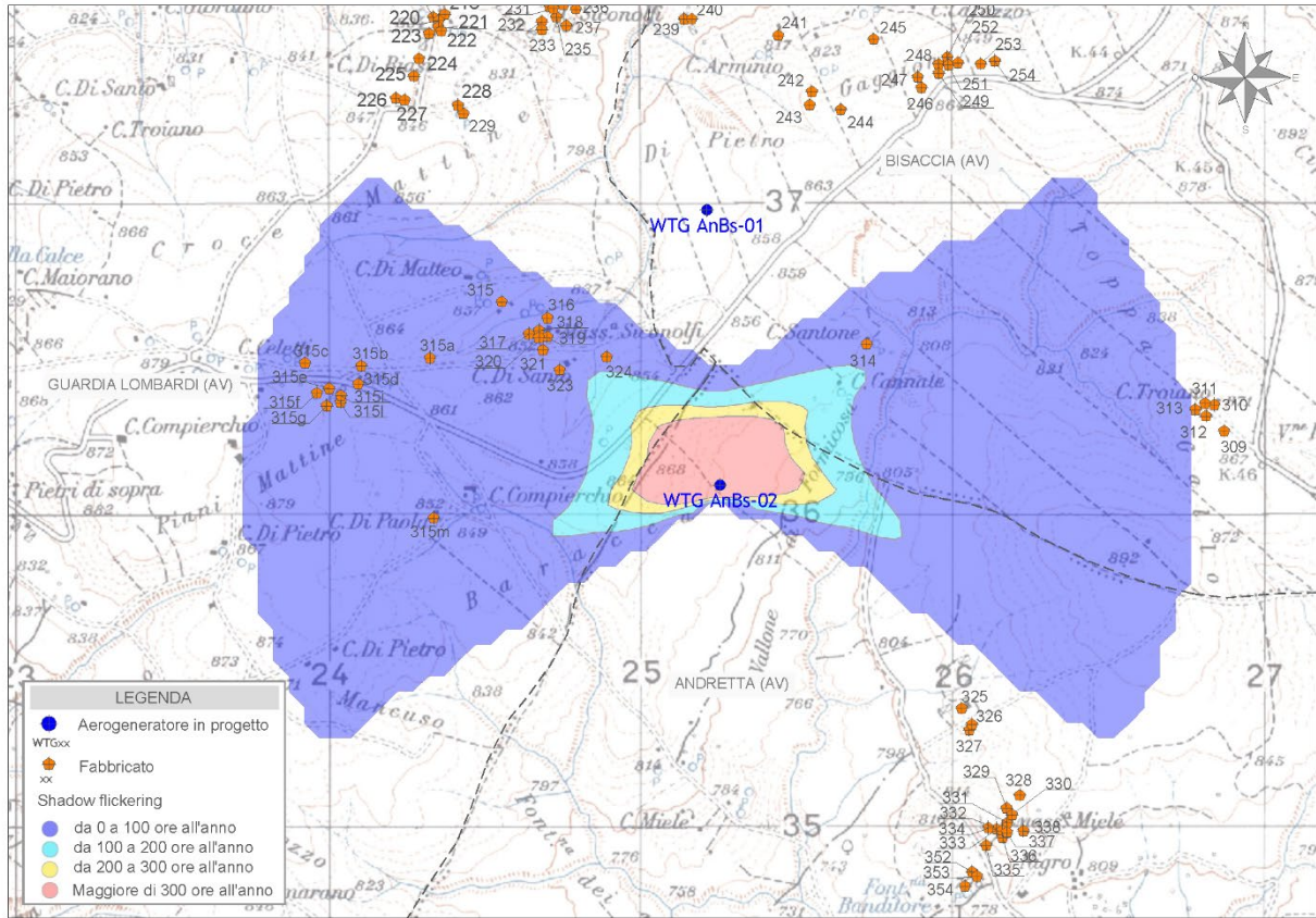
Figura 3 - Mappa di impatto potenziale per l'aerogeneratore WTG AnBs-02
