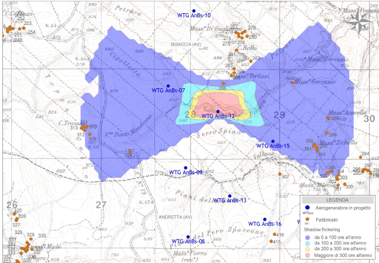
Figura 13- Mappa di impatto potenziale per l'aerogeneratore WTG AnBs-12
