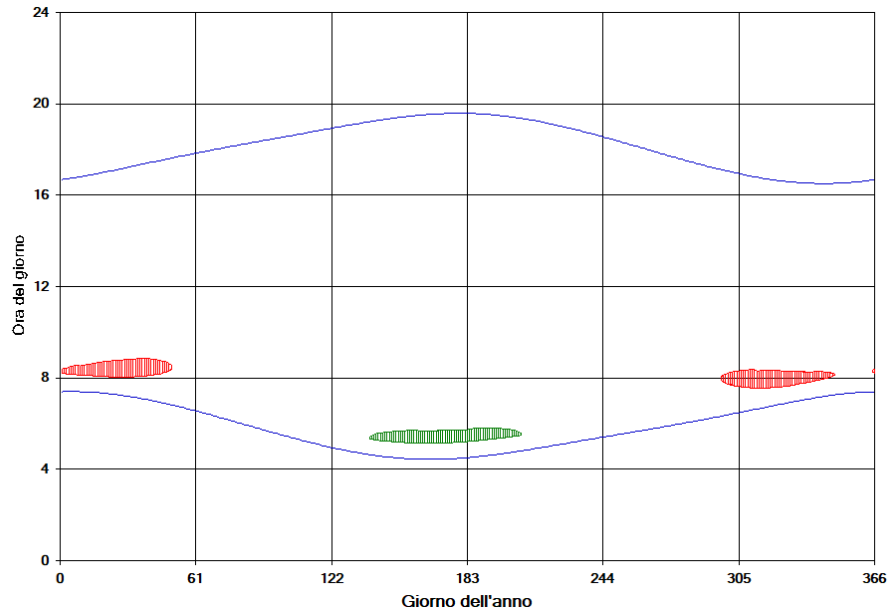
Figura 21 – Calendario dell'ombra nelle condizioni caso peggiore per il fabbricato 183
