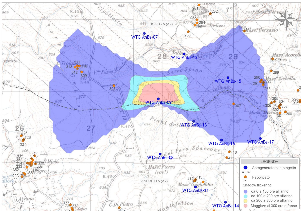
Figura 10 - Mappa di impatto potenziale per l'aerogeneratore WTG AnBs-09
