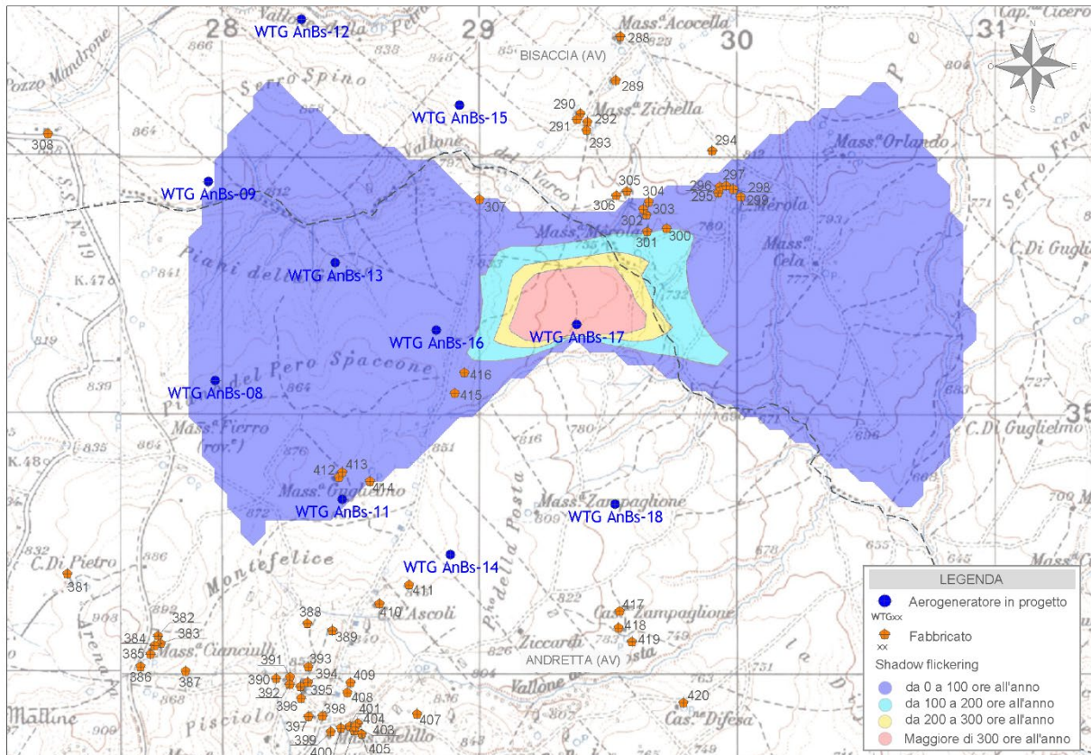
Figura 18 - Mappa di impatto potenziale per l'aerogeneratore WTG AnBs-17
