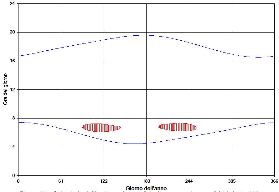
Figura 25 – Calendario dell'ombra nelle condizioni caso peggiore per il fabbricato 210
