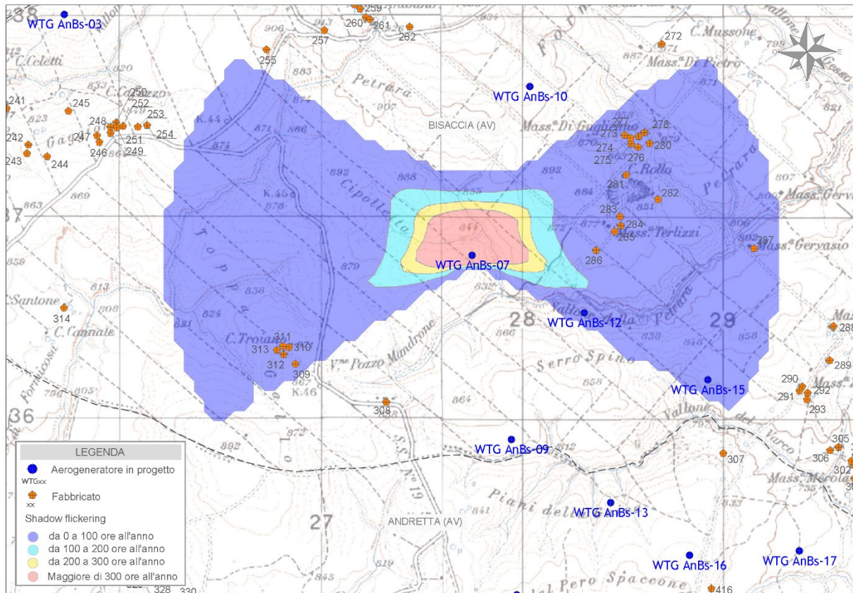
Figura 8 - Mappa di impatto potenziale per l'aerogeneratore WTG AnBs-07
