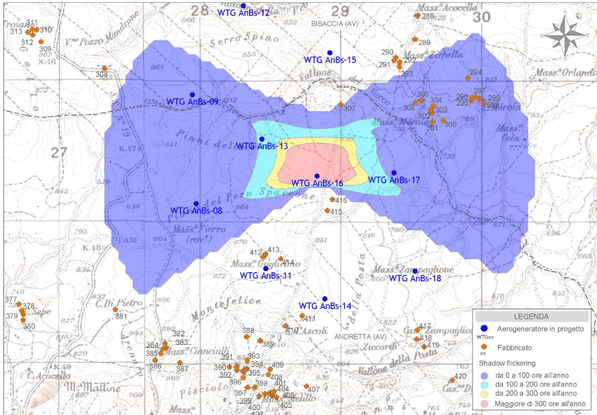
Figura 17 - Mappa di impatto potenziale per l'aerogeneratore WTG AnBs-16
