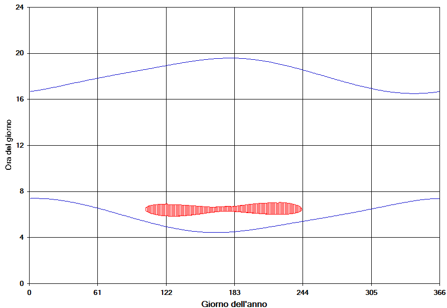
Figura 26 – Calendario dell'ombra nelle condizioni caso peggiore per il fabbricato 211
