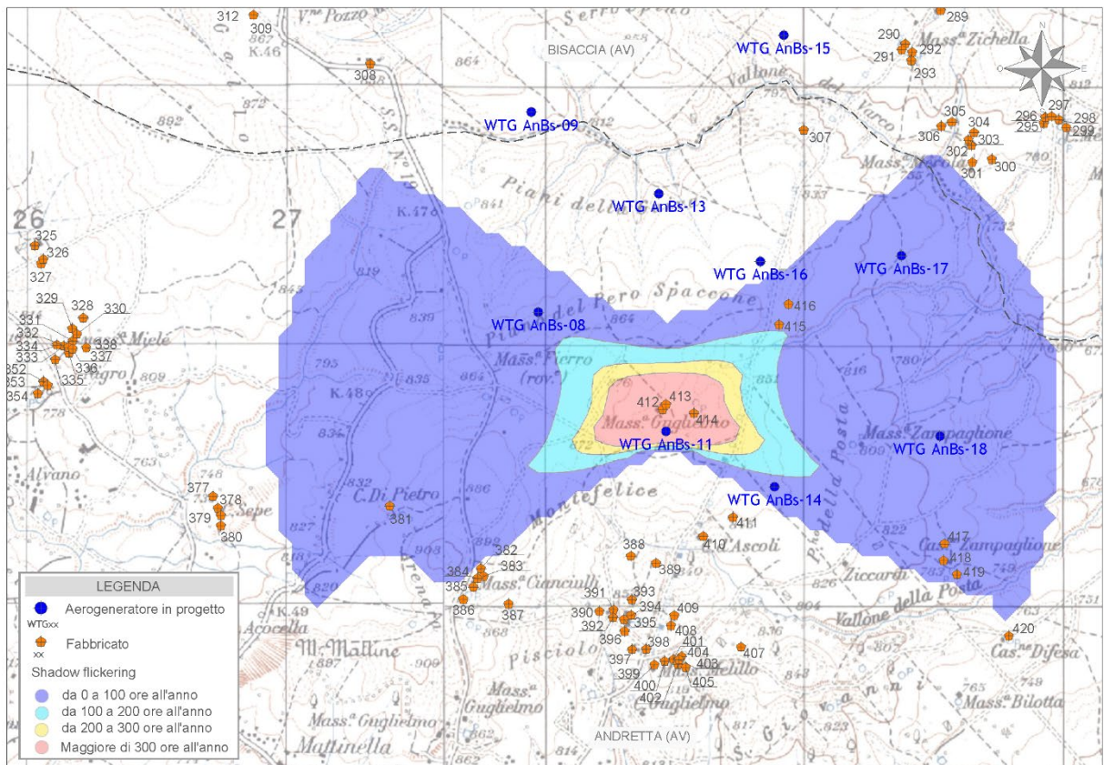
Figura 12 - Mappa di impatto potenziale per l'aerogeneratore WTG AnBs-11
