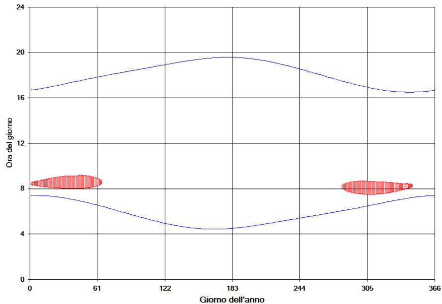
Figura 23 – Calendario dell'ombra nelle condizioni caso peggiore per il fabbricato 198
