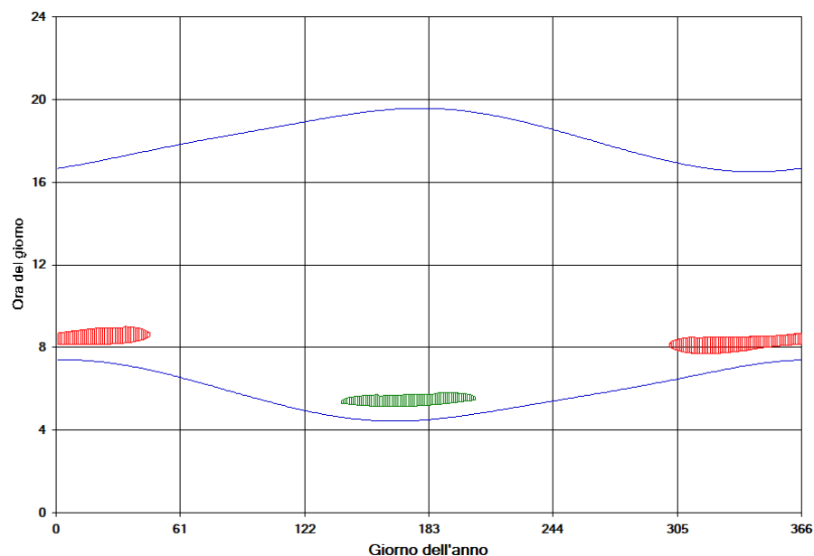
Figura 20- Calendario dell'ombra nelle condizioni caso peggiore per il fabbricato 182
