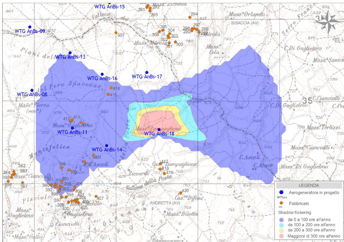
Figura 19 - Mappa di impatto potenziale per l'aerogeneratore WTG AnBs-18
