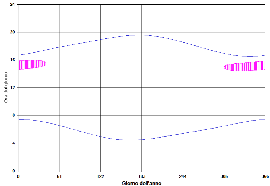
Figura 28 – Calendario dell'ombra nelle condizioni caso peggiore per il fabbricato 243
