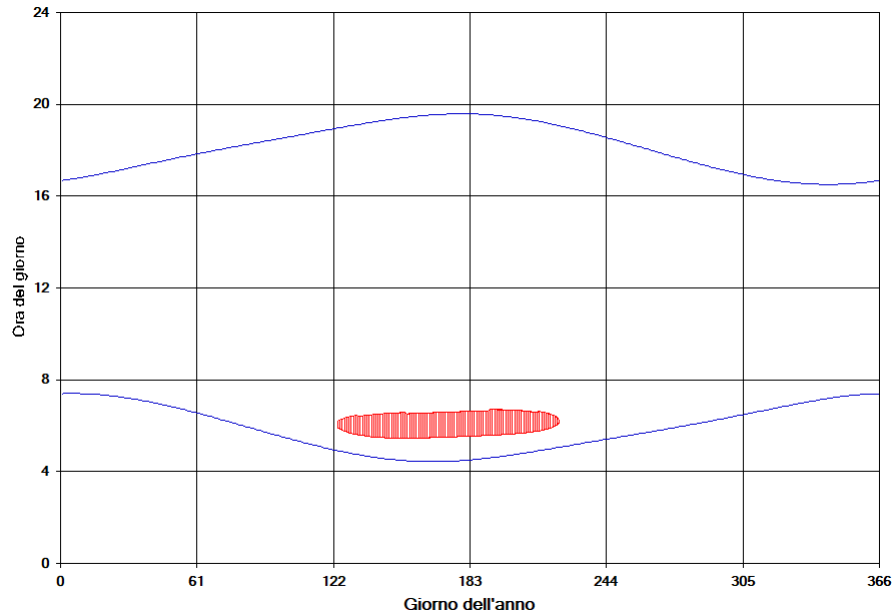
Figura 27 – Calendario dell'ombra nelle condizioni caso peggiore per il fabbricato 212
