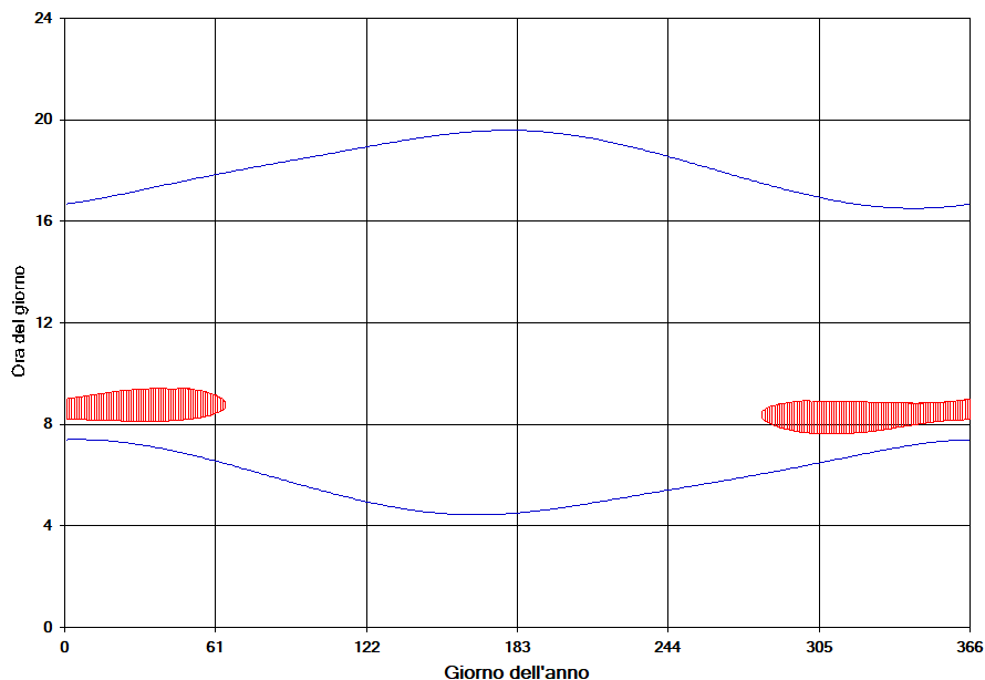
Figura 24 – Calendario dell'ombra nelle condizioni caso peggiore per il fabbricato 200
