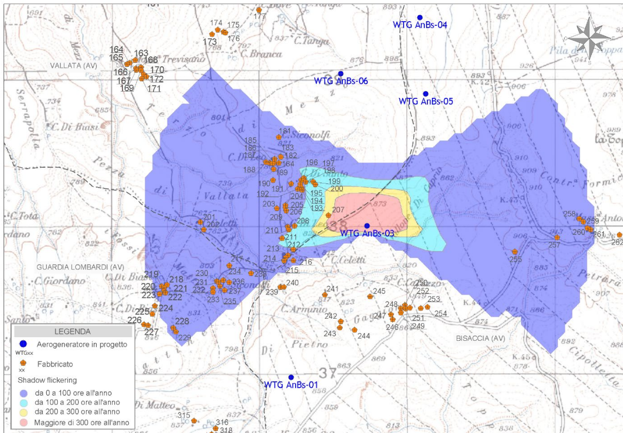
Figura 4 - Mappa di impatto potenziale per l'aerogeneratore WTG AnBs-03
