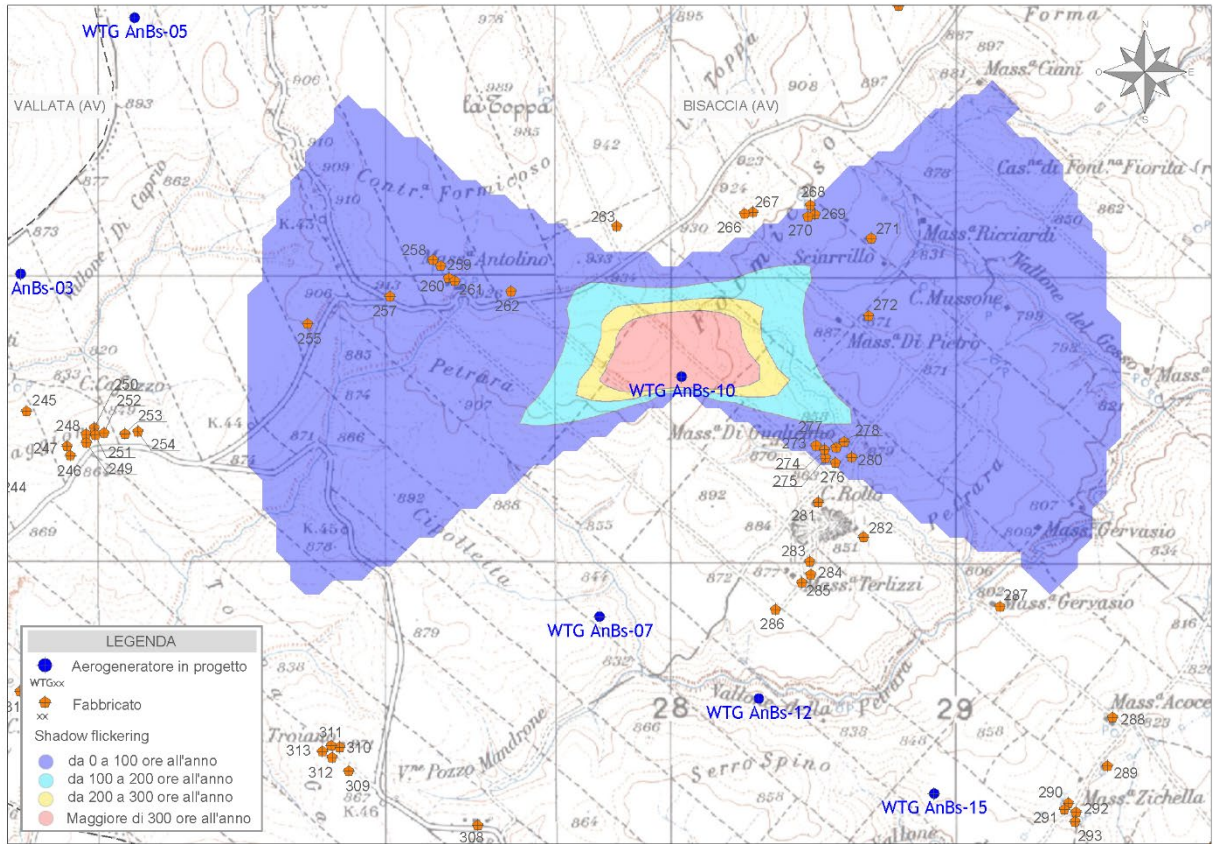
Figura 11- Mappa di impatto potenziale per l'aerogeneratore WTG AnBs-10
