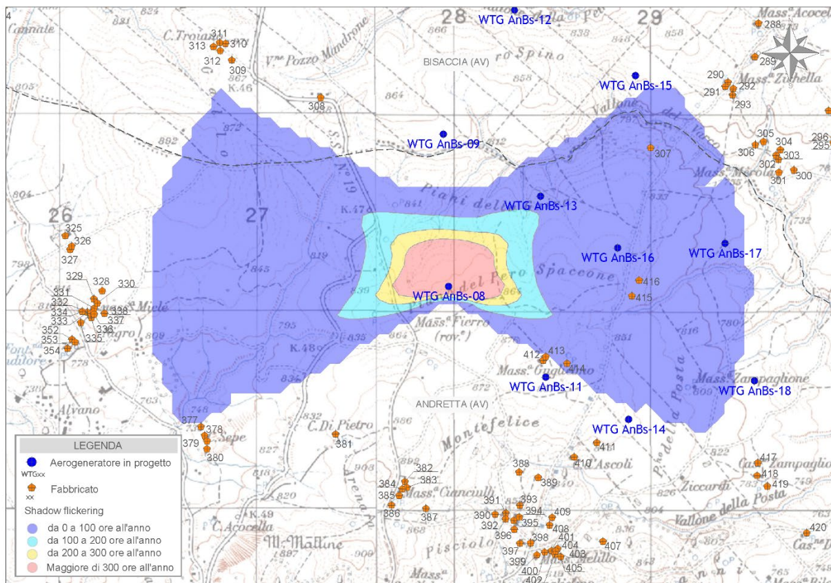
Figura 9 - Mappa di impatto potenziale per l'aerogeneratore WTG AnBs-08
