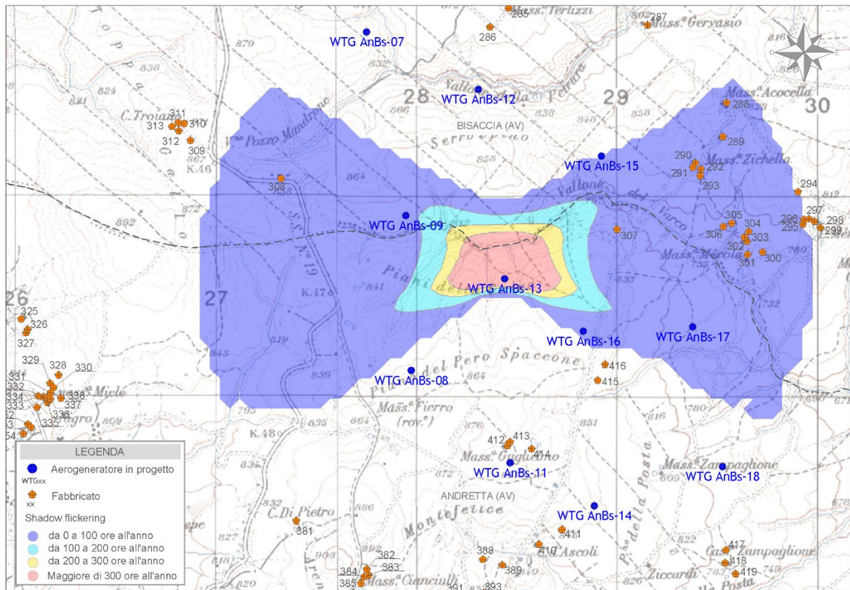
Figura 14 - Mappa di impatto potenziale per l'aerogeneratore WTG AnBs-13
