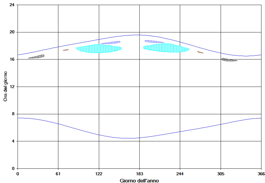
Figura 30 – Calendario dell'ombra nelle condizioni caso peggiore per il fabbricato 291
