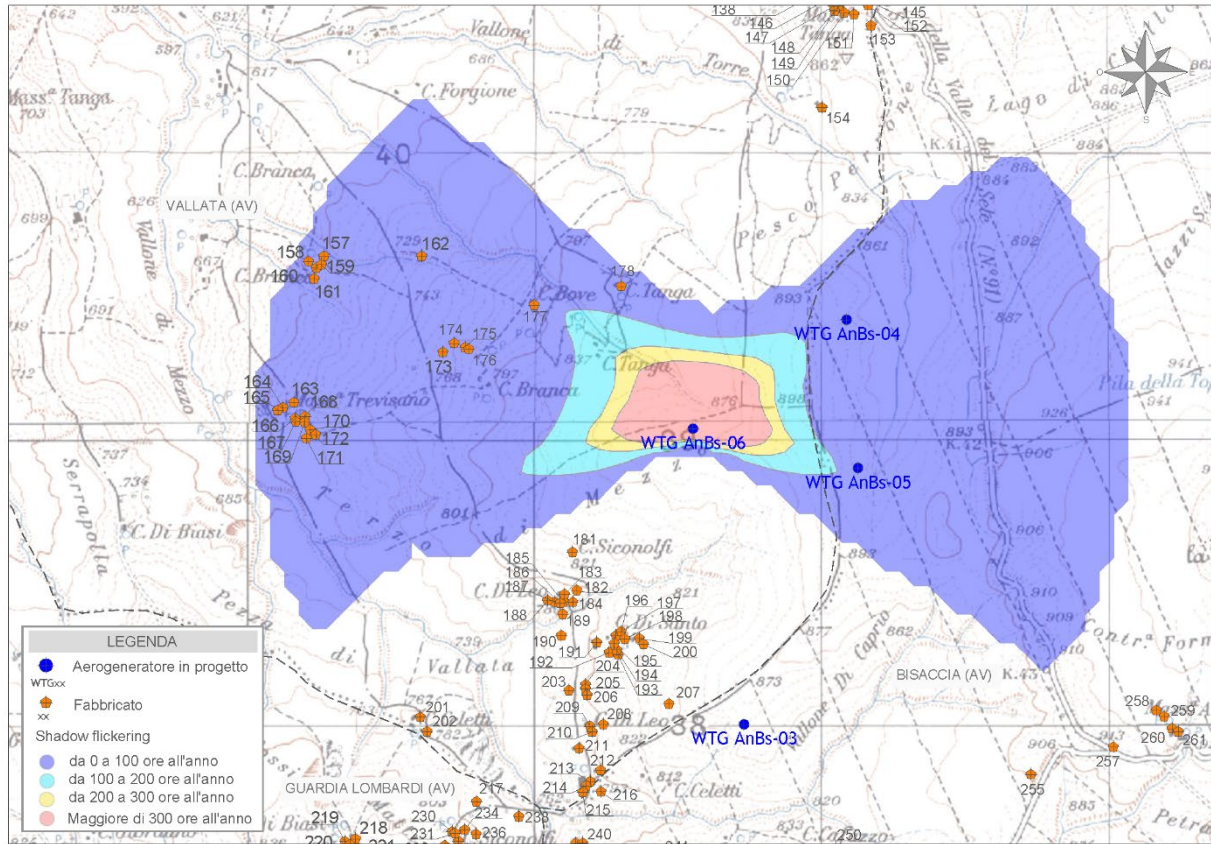
Figura 7 - Mappa di impatto potenziale per l'aerogeneratore WTG AnBs-06
