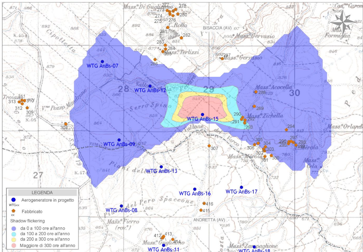
Figura 16 - Mappa di impatto potenziale per l'aerogeneratore WTG AnBs-15
