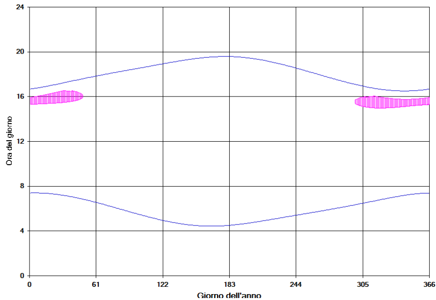
Figura 29– Calendario dell'ombra nelle condizioni caso peggiore per il fabbricato 244
