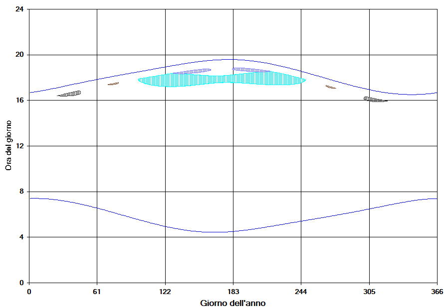
Figura 31 – Calendario dell'ombra nelle condizioni caso peggiore per il fabbricato 293
