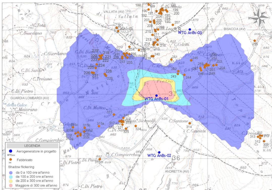
Figura 2 - Mappa di impatto potenziale per l'aerogeneratore WTG AnBs-01
