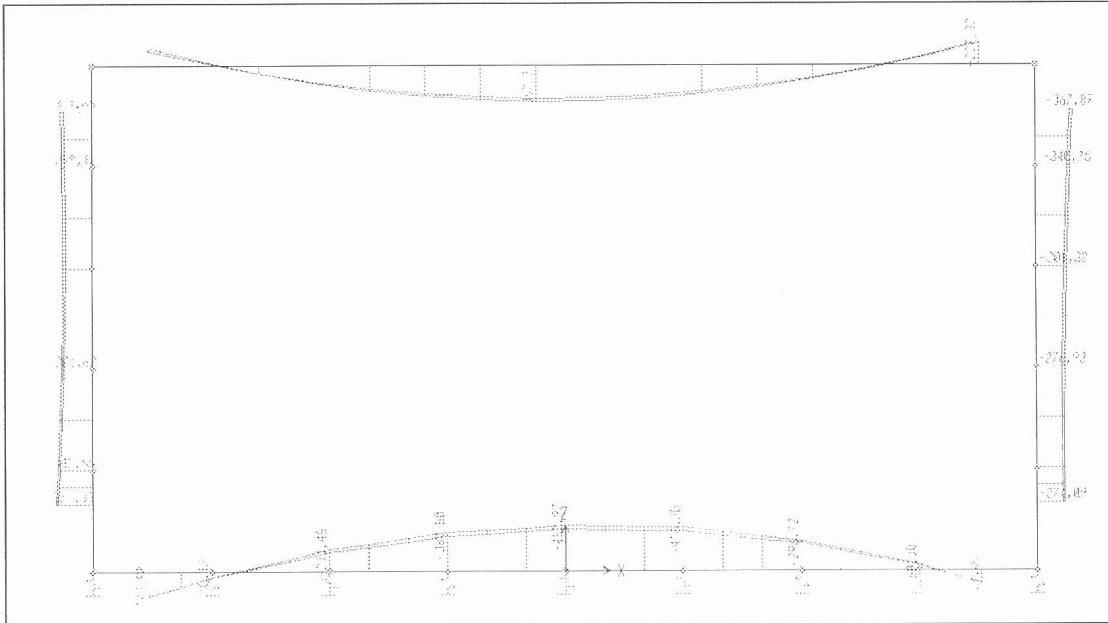
Figura 9 - Inv_Sisma – Diagramma del momento flettente
