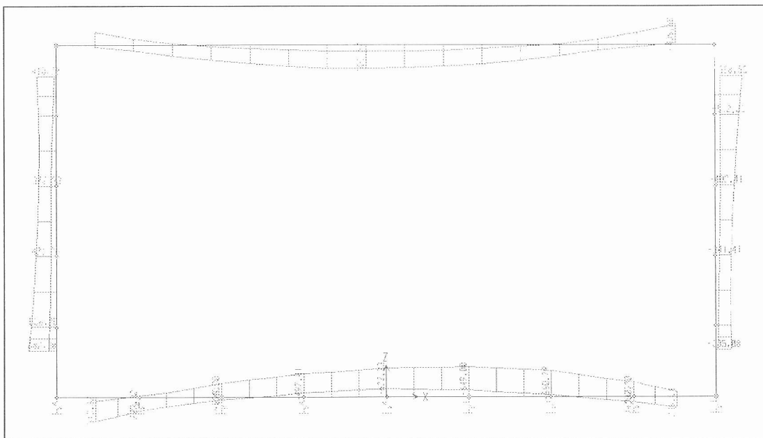
Figura 6 - Inv_TA – Diagramma del momento flettente
