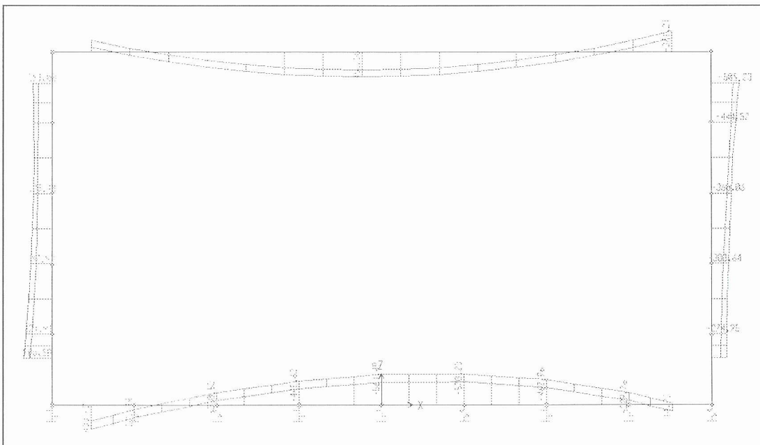
Figura 12 - Inv_Fessurazione – Diagramma del momento flettente
