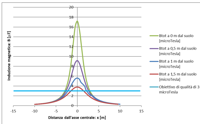
Andamento del campo magnetico generato composto da cinque terne da 630 mm 2
