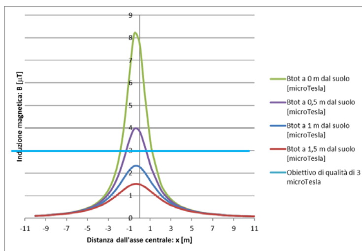
Andamento del campo magnetico generato dal cavidotto, composto da due terne da 630 mm 2
