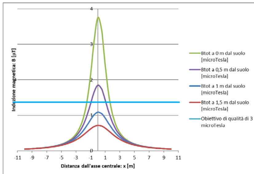
Andamento del campo magnetico generato dal cavidotto, composto da due terne una da 120 mm 2 e una da 400 mm 2
