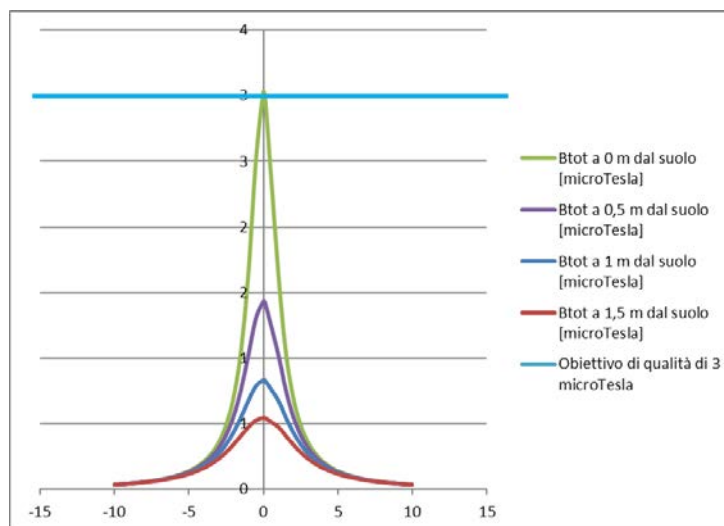
Andamento del campo magnetico generato dal cavidotto, composto da una terna da 120 mm 2
