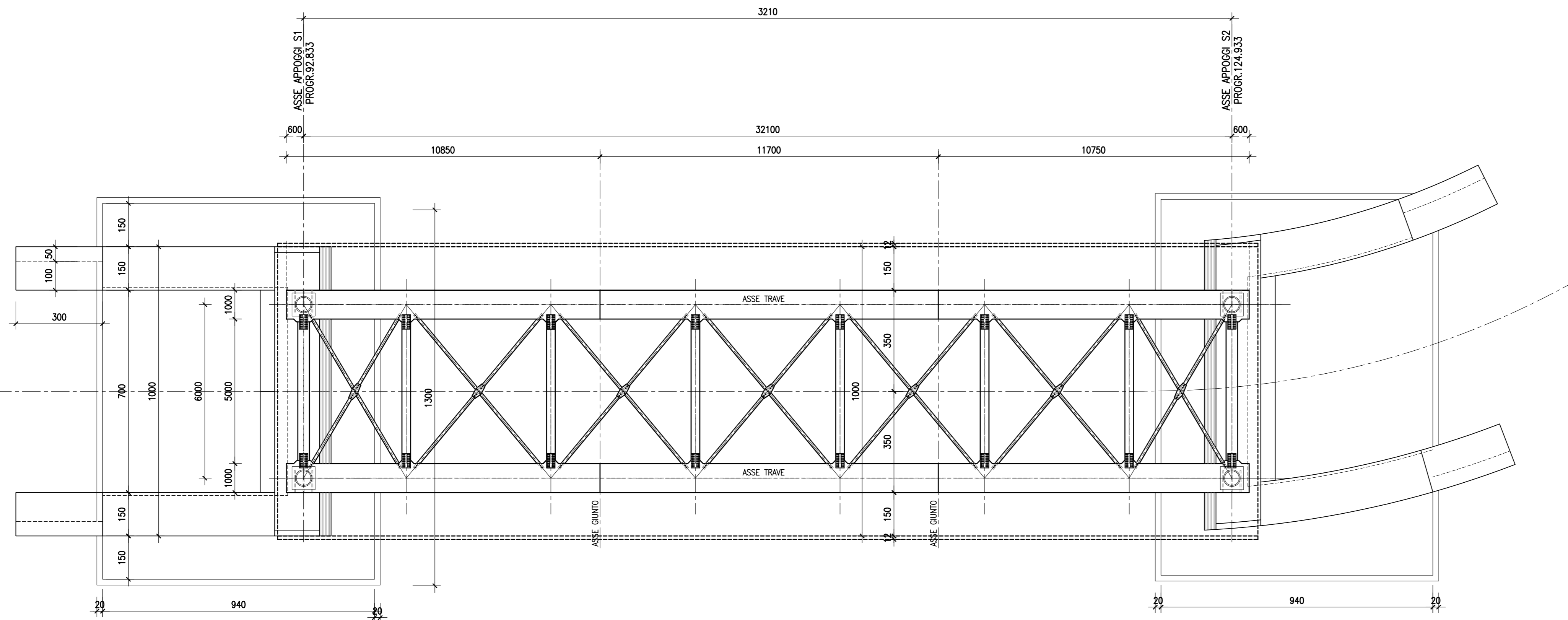
PIANTA IMPALCATO—Scala 1:100
