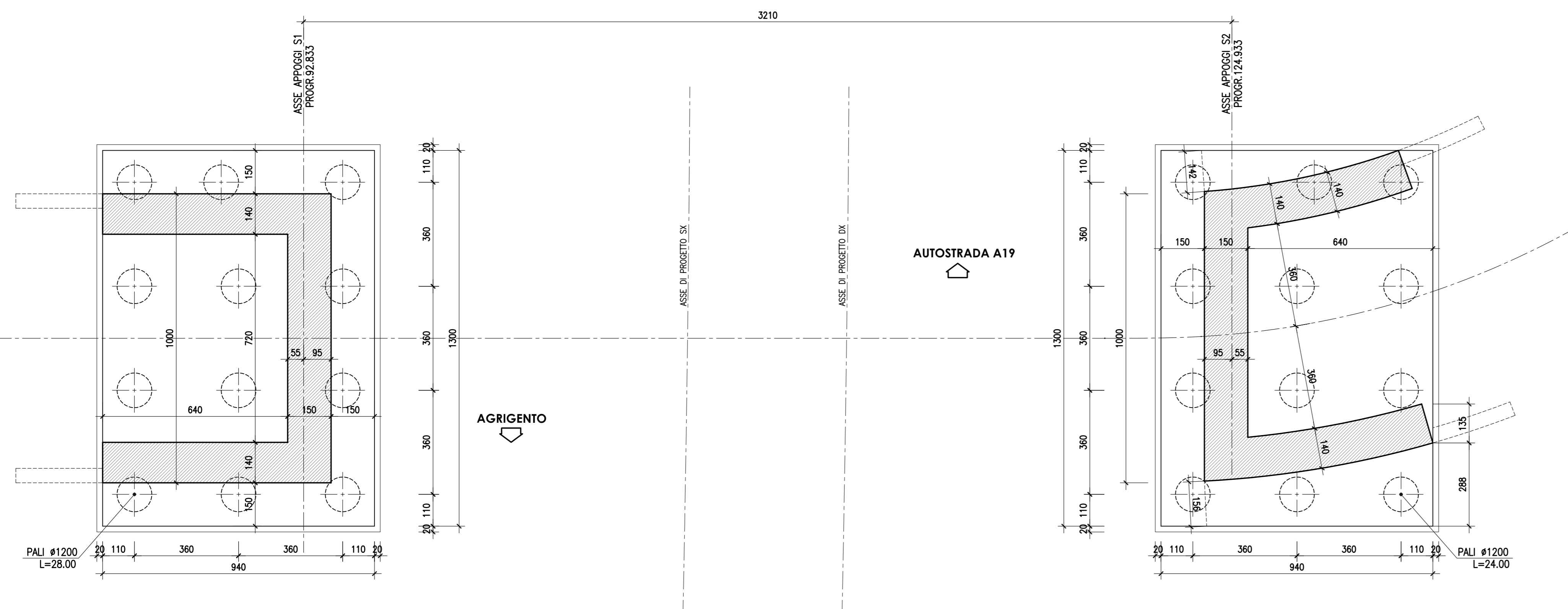
PIANTA FONDAZIONI—Scala 1:100
