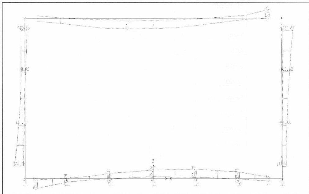
Figura 6 - Inv_TA – Diagramma del momento flettente
