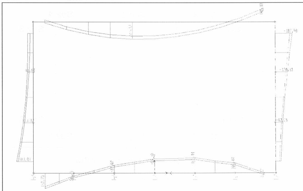
Figura 12 - Inv_Fessurazione – Diagramma del momento flettente
