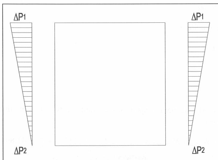
Figura 5 - Diagrammi delle sovraspinte sismiche applicate ai piedritti
