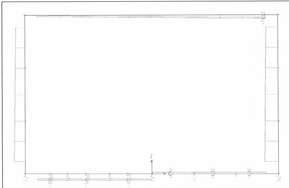
Figura 13 - Inv_ Fessurazione – Diagramma dello sforzo
