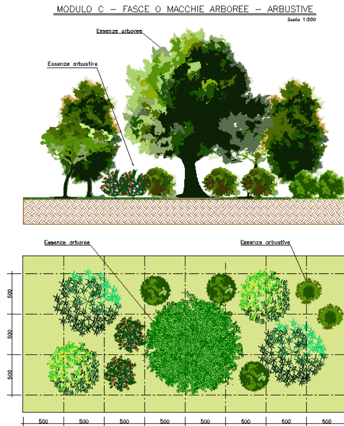
Figura 4-3 – MODULO C – Fasce o macchie arboreo-arbustive: sesto d'impianto e sezione tipologica
