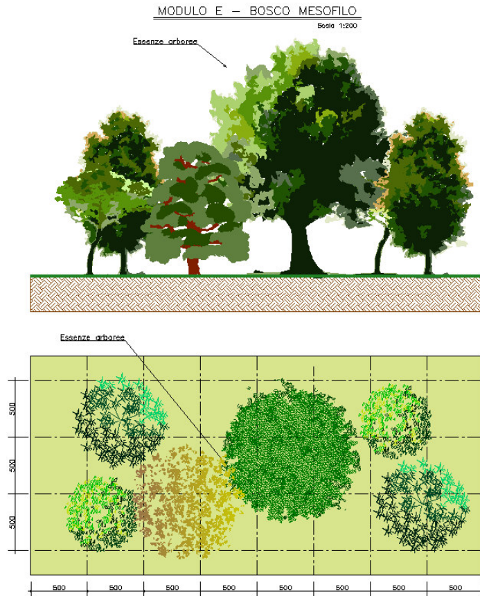
Figura 4-5 – MODULO E – Bosco mesofilo: sesto d'impianto e sezione tipologica
