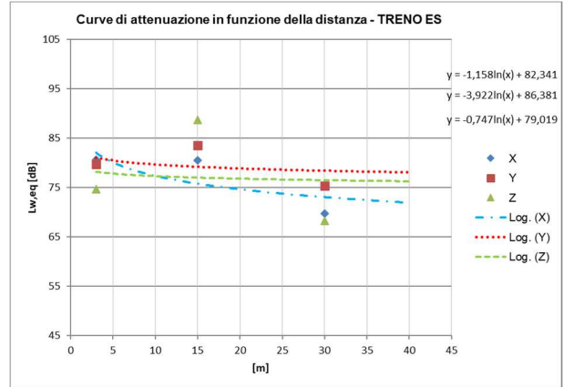
Figura 10 - Curva di attenuazione del L_{w,eq} in funzione della distanza dal binario, ricavata dai rilievi sperimentali sull'attuale linea in esercizio lungo gli assi x, y e z, in corrispondenza delle SEZ. 1 e valutata considerando le velocità di progetto a sinistra a 250 km/h per TIPOLOGIA TRENO IC-EC a destra a 300 km/h – TIPOLOGIA TRENO ES per t. coperto
