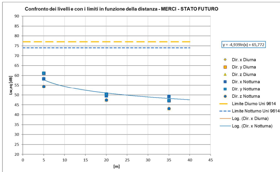
Figura 66 – Curve di attenuazione in funzione della distanza relativa al traffico ferroviario di progetto – tratti allo scoperto, TRENI MERCI a 100 km/h
