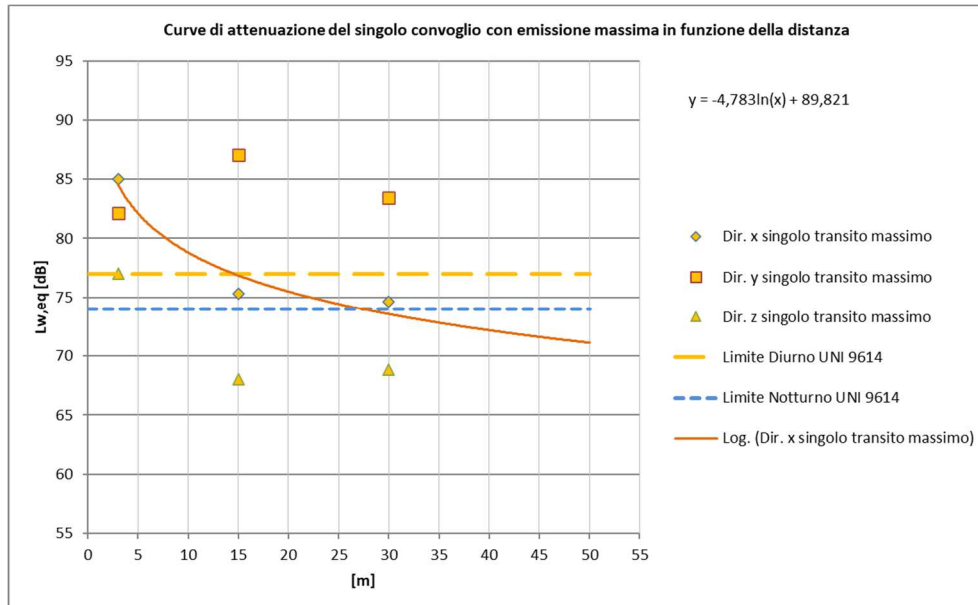
Figura 46 – Curva di attenuazione in funzione della distanza relativa al transito massimo – tratti al coperto
