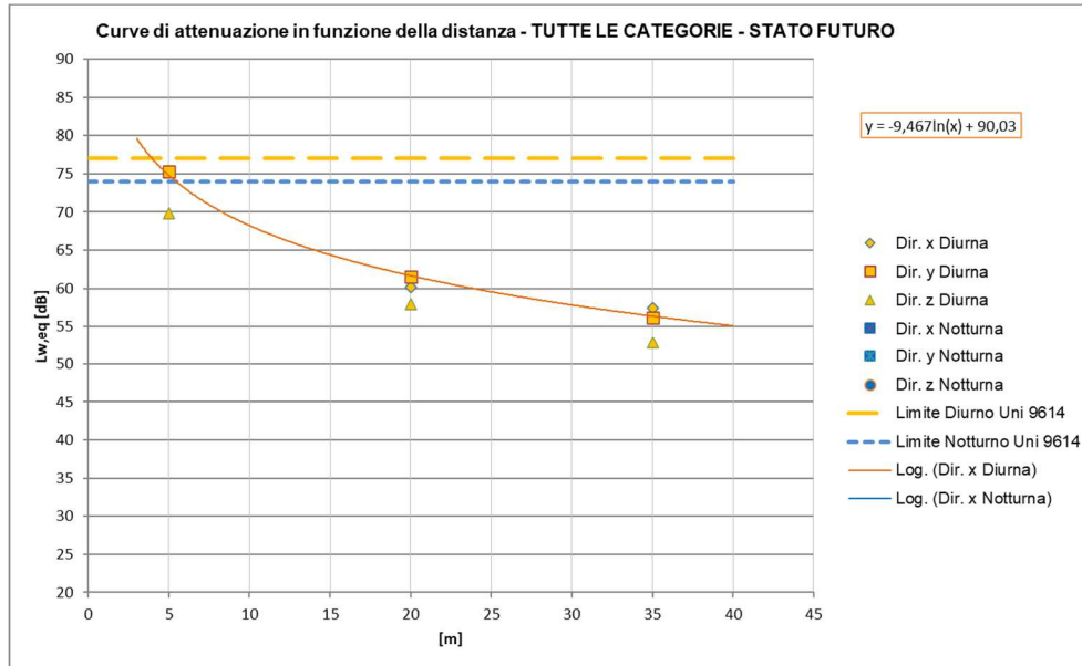
Figura 77 – Curve di attenuazione in funzione della distanza relativa al traffico ferroviario di progetto – tratti allo scoperto, Treni TUTTE LE CATEGORIE
