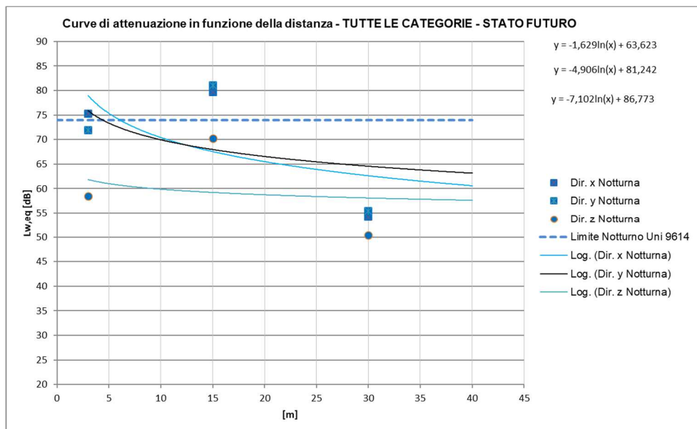
Figura 58 – Curve di attenuazione in funzione della distanza relativa al traffico ferroviario di progetto – tratti allo scoperto INTERNO AGLI EDIFICI, Treni TUTTE LE CATEGORIE, periodo notturno
