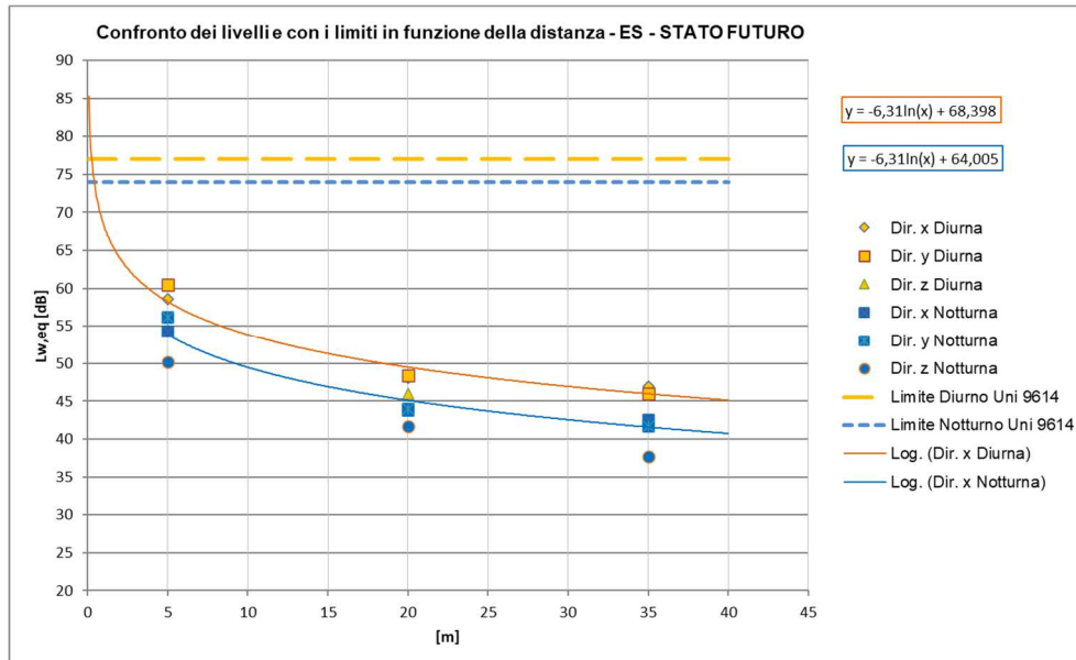
Figura 81 – Curve di attenuazione in funzione della distanza relativa al traffico ferroviario di progetto – tratti allo scoperto, TRENI ES a 100 km/h
