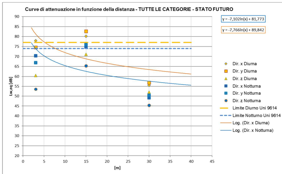
Figura 56 – Curve di attenuazione in funzione della distanza relativa al traffico ferroviario di progetto – tratti allo scoperto, Treni TUTTE LE CATEGORIE
