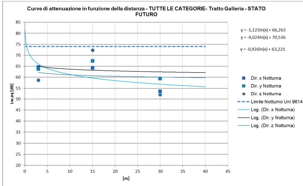
Figura 39 – Curve di attenuazione in funzione della distanza relativa al traffico ferroviario di progetto – tratti al coperto INTERNO AGLI EDIFICI, Treni TUTTE LE CATEGORIE, periodo notturno
