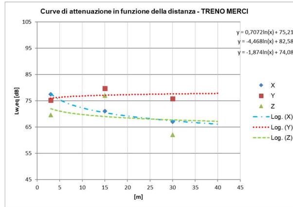
Figura 14 - Curva di attenuazione del L_{w,eq} in funzione della distanza dal binario, ricavata dai rilievi sperimentali sull'attuale linea in esercizio lungo gli assi x, y e z, in corrispondenza delle SEZ. 1 e valutata considerando le velocità di progetto di 100 km/h – TIPOLOGIA TRENO MERCI per t. coperto/roccia
