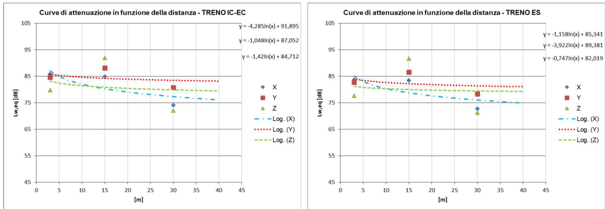
Figura 12 - Curva di attenuazione del L_{w,eq} in funzione della distanza dal binario, ricavata dai rilievi sperimentali sull'attuale linea in esercizio lungo gli assi x, y e z, in corrispondenza delle SEZ. 1 e valutata considerando le velocità di progetto a sinistra a 250 km/h per TIPOLOGIA TRENO IC-EC a destra a 300 km/h – TIPOLOGIA TRENO ES per t. coperto/roccia
