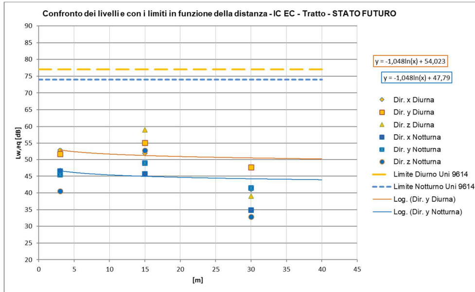
Figura 40 – Curve di attenuazione in funzione della distanza relativa al traffico ferroviario di progetto – tratti al coperto, TRENI IC-EC a 100km/h
