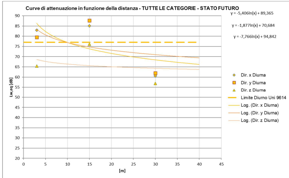
Figura 57 – Curve di attenuazione in funzione della distanza relativa al traffico ferroviario di progetto – tratti allo scoperto INTERNO AGLI EDIFICI, Treni TUTTE LE CATEGORIE, periodo diurno
