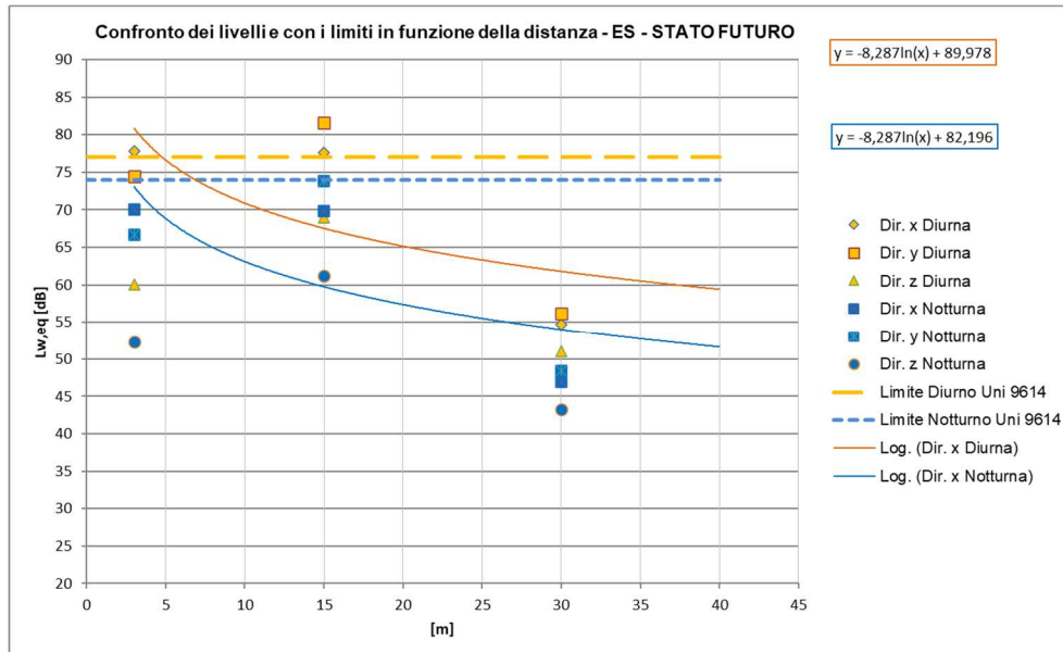
Figura 54 – Curve di attenuazione in funzione della distanza relativa al traffico ferroviario di progetto – tratti allo scoperto, TRENI ES a 300km/h
