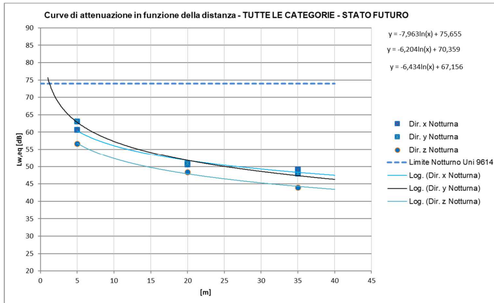
Figura 84 – Curve di attenuazione in funzione della distanza relativa al traffico ferroviario di progetto – tratti allo scoperto INTERNO AGLI EDIFICI, Treni TUTTE LE CATEGORIE, periodo notturno
