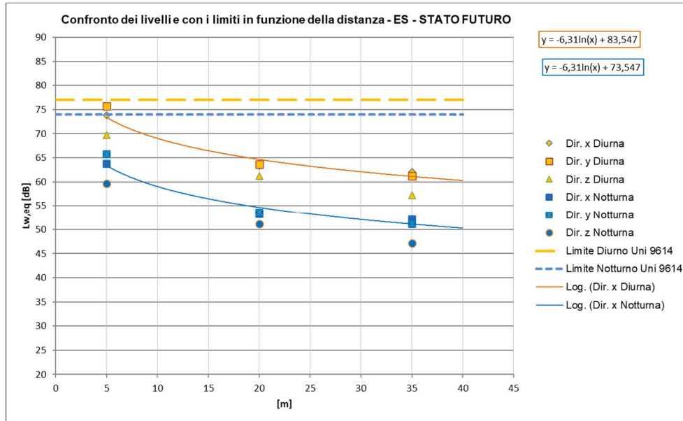
Figura 65 – Curve di attenuazione in funzione della distanza relativa al traffico ferroviario di progetto – tratti allo scoperto, TRENI ES a 300 km/h
