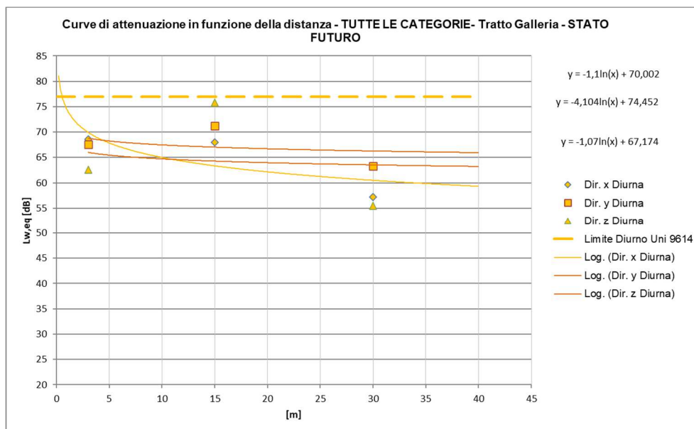
Figura 38 – Curve di attenuazione in funzione della distanza relativa al traffico ferroviario di progetto – tratti al coperto INTERNO AGLI EDIFICI, Treni TUTTE LE CATEGORIE, periodo diurno
