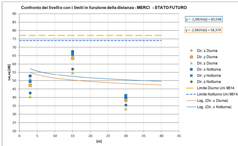
Figura 49 – Curve di attenuazione in funzione della distanza relativa al traffico ferroviario di progetto – tratti allo scoperto, TRENI MERCI a 100km/h
