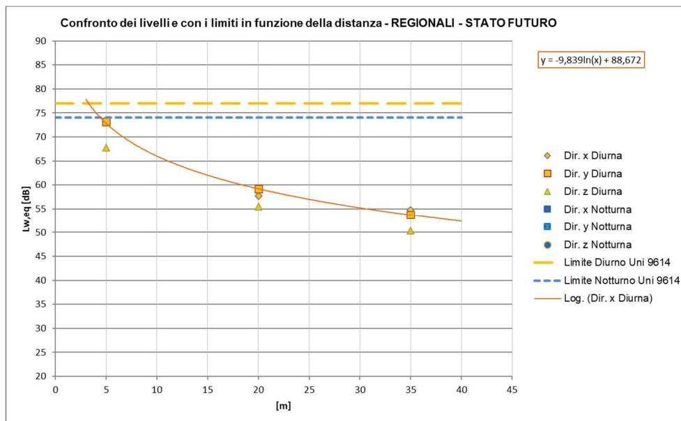
Figura 79 – Curve di attenuazione in funzione della distanza relativa al traffico ferroviario di progetto – tratti allo scoperto, TRENI REG a 100 km/h
