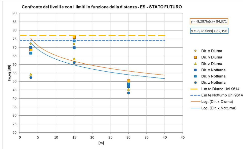
Figura 60 – Curve di attenuazione in funzione della distanza relativa al traffico ferroviario di progetto – tratti allo scoperto, TRENI ES a 300km/h
