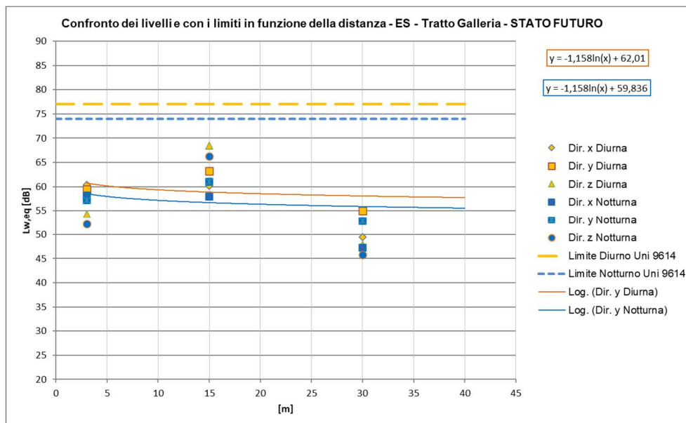
Figura 36 – Curve di attenuazione in funzione della distanza relativa al traffico ferroviario di progetto – tratti al coperto, TRENI ES a 300km/h
