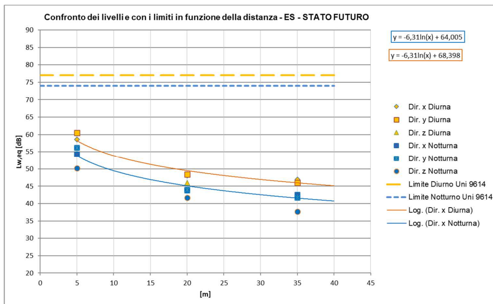
Figura 71 – Curve di attenuazione in funzione della distanza relativa al traffico ferroviario di progetto – tratti allo scoperto, TRENI ES a 100 km/h
