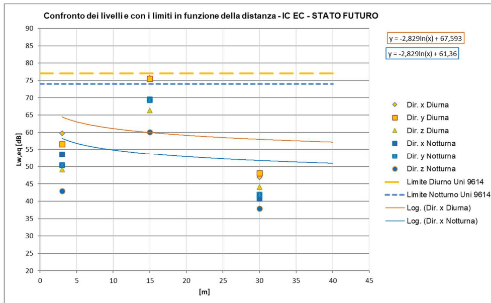
Figura 59 – Curve di attenuazione in funzione della distanza relativa al traffico ferroviario di progetto – tratti allo scoperto, TRENI IC-EC a 250km/h
