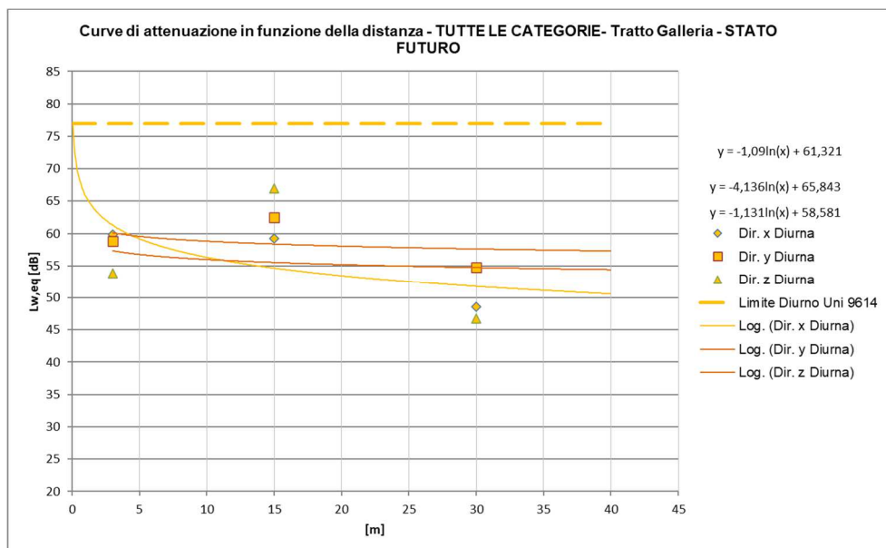
Figura 43 – Curve di attenuazione in funzione della distanza relativa al traffico ferroviario di progetto – tratti al coperto INTERNO AGLI EDIFICI, Treni TUTTE LE CATEGORIE, periodo diurno
