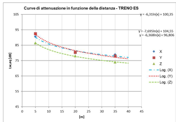
Figura 20 - Curva di attenuazione del L_{w,eq} in funzione della distanza dal binario, ricavata dai rilievi sperimentali sull'attuale linea in esercizio lungo gli assi x, y e z, in corrispondenza delle SEZ. 3 e valutata considerando le velocità di progetto a sinistra a 250 km/h per TIPOLOGIA TRENO IC-EC a destra a 300 km/h – TIPOLOGIA TRENO ES per t. scoperto/rilevato
