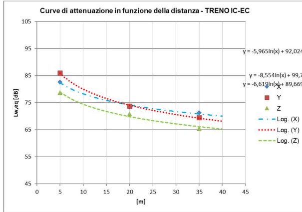
Figura 21 - Curva di attenuazione del L_{w,eq} in funzione della distanza dal binario, ricavata dai rilievi sperimentali sull'attuale linea in esercizio lungo gli assi x, y e z, in corrispondenza delle SEZ. 3 e valutata considerando le velocità di progetto a sinistra a 100 km/h per TIPOLOGIA TRENO IC-EC a destra a 100 km/h – TIPOLOGIA TRENO ES per t. scoperto/rilevato
