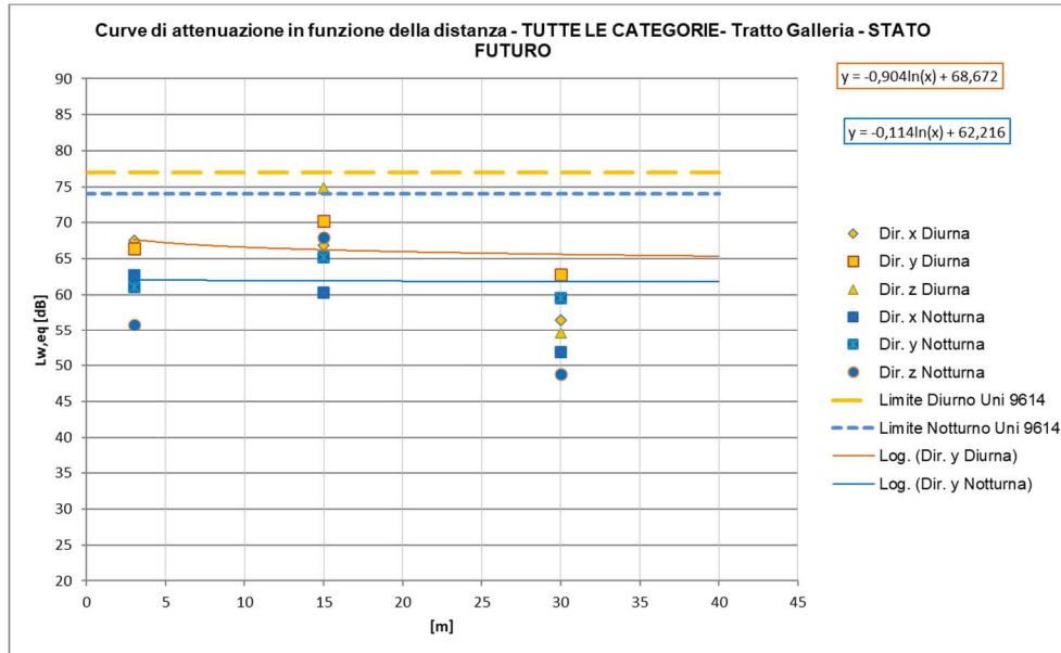
Figura 32 – Curve di attenuazione in funzione della distanza relativa al traffico ferroviario di progetto – tratti al coperto, Treni TUTTE LE CATEGORIE
