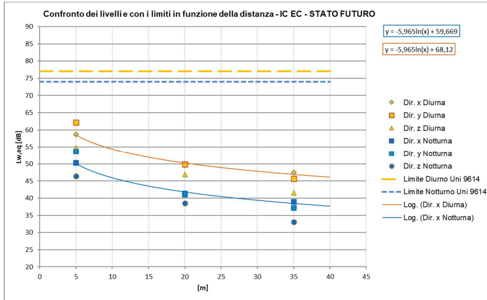
Figura 70 – Curve di attenuazione in funzione della distanza relativa al traffico ferroviario di progetto – tratti allo scoperto, TRENI IC-EC a 100 km/h
