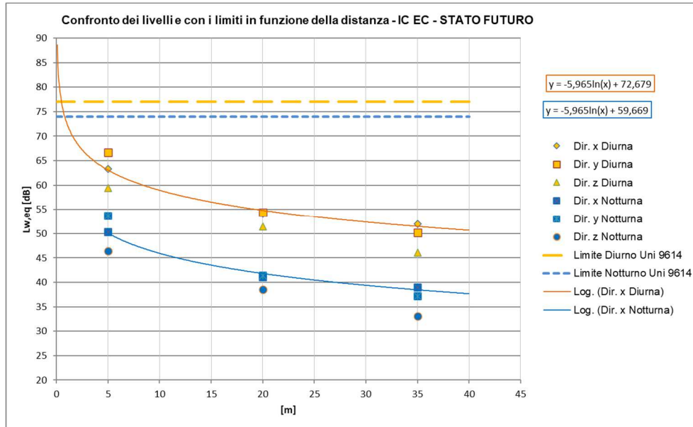
Figura 80 – Curve di attenuazione in funzione della distanza relativa al traffico ferroviario di progetto – tratti allo scoperto, TRENI IC-EC a 100 km/h
