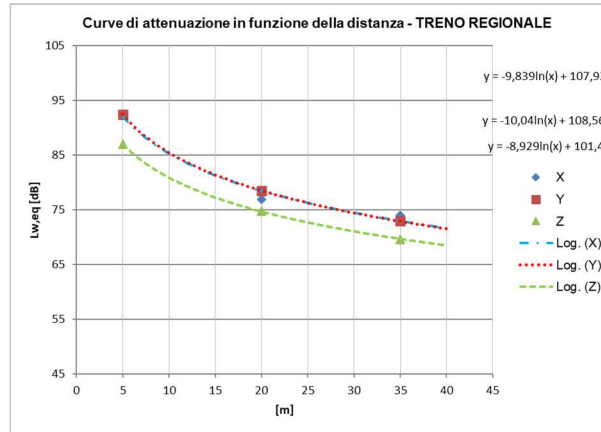
Figura 19 - Curva di attenuazione del L_{w,eq} in funzione della distanza dal binario, ricavata dai rilievi sperimentali sull'attuale linea in esercizio lungo gli assi x, y e z, in corrispondenza delle SEZ. 3 e valutata considerando le velocità di progetto a sinistra a 100 km/h per TIPOLOGIA TRENO REG per t. scoperto/rilevato
