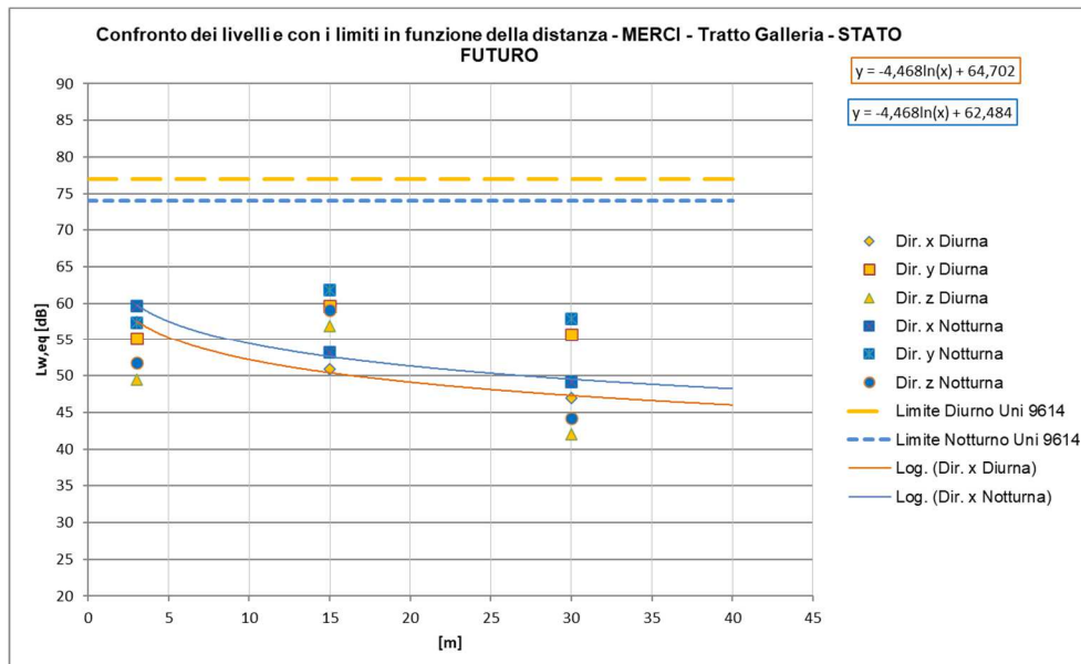
Figura 31 – Curve di attenuazione in funzione della distanza relativa al traffico ferroviario di progetto – tratti al coperto, TRENI MERCI a 100km/h
