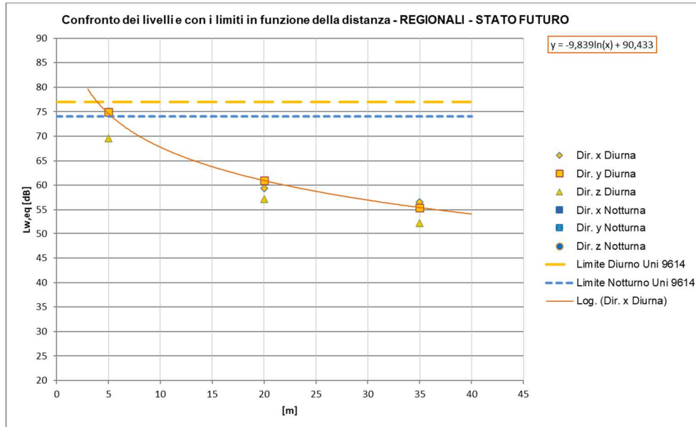
Figura 75 – Curve di attenuazione in funzione della distanza relativa al traffico ferroviario di progetto – tratti allo scoperto, TRENI REG a 100 km/h
