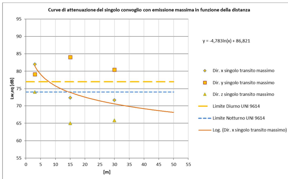
Figura 45 – Curva di attenuazione in funzione della distanza relativa al transito massimo – tratti al coperto
