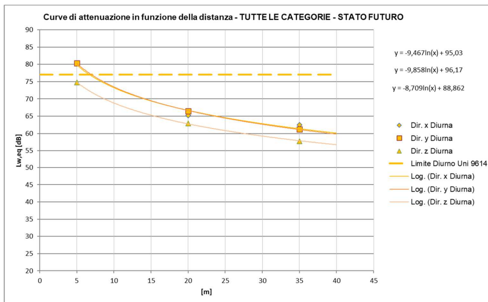
Figura 78 – Curve di attenuazione in funzione della distanza relativa al traffico ferroviario di progetto – tratti allo scoperto INTERNO AGLI EDIFICI, Treni TUTTE LE CATEGORIE, periodo diurno
