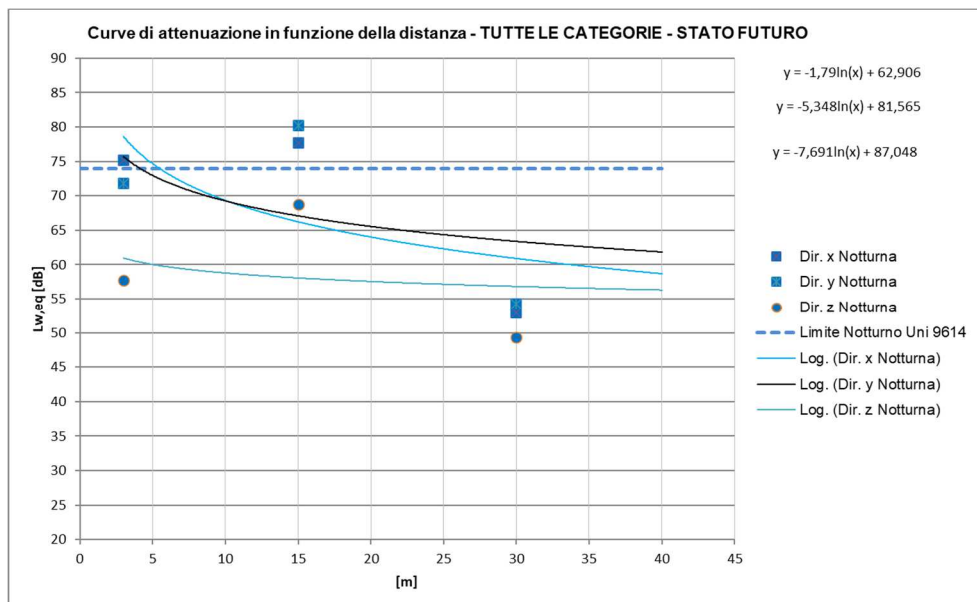
Figura 63 – Curve di attenuazione in funzione della distanza relativa al traffico ferroviario di progetto – tratti allo scoperto INTERNO AGLI EDIFICI, Treni TUTTE LE CATEGORIE, periodo notturno
