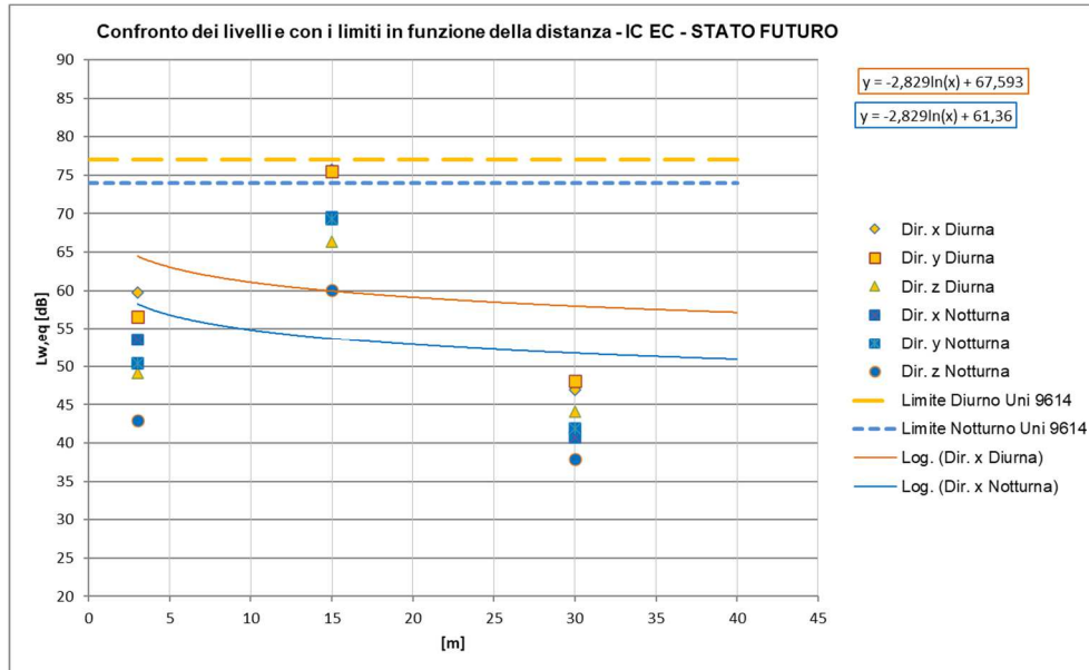
Figura 53 – Curve di attenuazione in funzione della distanza relativa al traffico ferroviario di progetto – tratti allo scoperto, TRENI IC-EC a 250km/h
