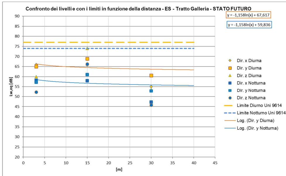
Figura 30 – Curve di attenuazione in funzione della distanza relativa al traffico ferroviario di progetto – tratti al coperto, TRENI ES a 300km/h
