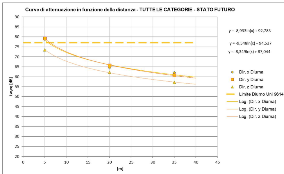
Figura 83 – Curve di attenuazione in funzione della distanza relativa al traffico ferroviario di progetto – tratti allo scoperto INTERNO AGLI EDIFICI, Treni TUTTE LE CATEGORIE, periodo diurno
