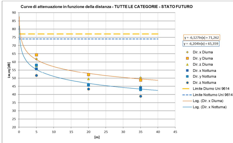
Figura 72 – Curve di attenuazione in funzione della distanza relativa al traffico ferroviario di progetto – tratti allo scoperto, Treni TUTTE LE CATEGORIE
