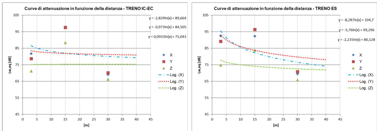
Figura 15 - Curva di attenuazione del L_{w,eq} in funzione della distanza dal binario, ricavata dai rilievi sperimentali sull'attuale linea in esercizio lungo gli assi x, y e z, in corrispondenza delle SEZ. 2 e valutata considerando le velocità di progetto a sinistra a 250 km/h per TIPOLOGIA TRENO IC-EC a destra a 300 km/h – TIPOLOGIA TRENO ES per t. scoperto/viadotto
