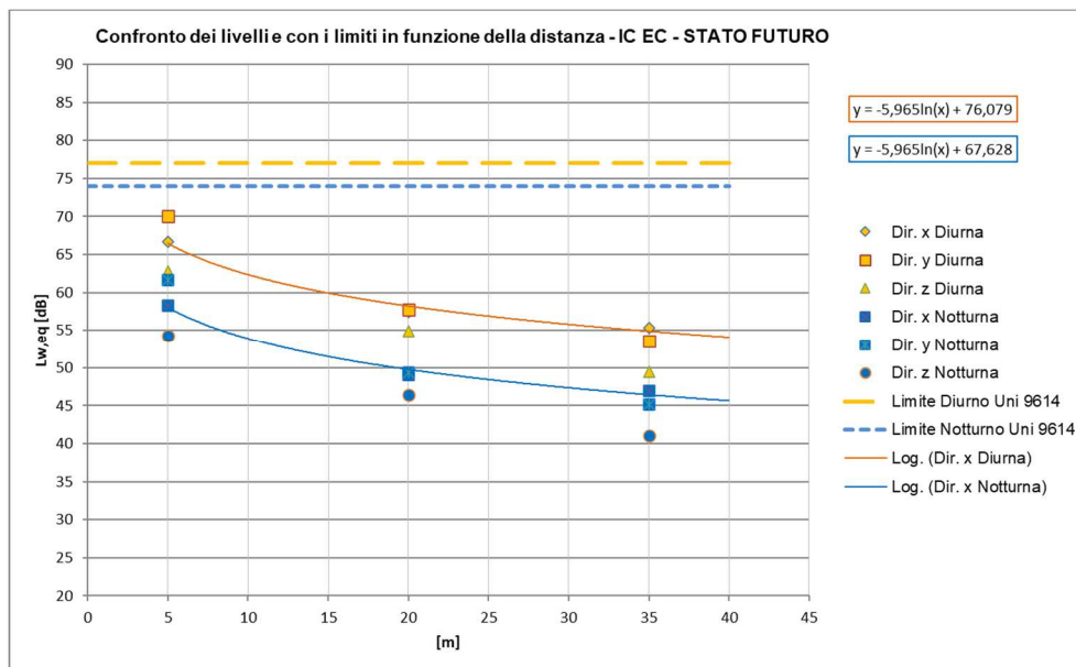
Figura 64 – Curve di attenuazione in funzione della distanza relativa al traffico ferroviario di progetto – tratti allo scoperto, TRENI IC-EC a 250 km/h
