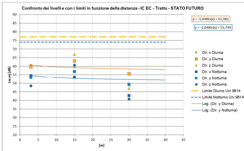
Figura 29 – Curve di attenuazione in funzione della distanza relativa al traffico ferroviario di progetto – tratti al coperto, TRENI IC-EC a 250km/h
