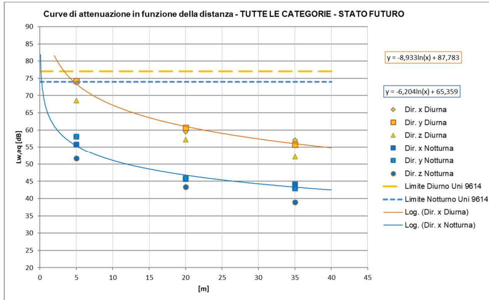
Figura 82 – Curve di attenuazione in funzione della distanza relativa al traffico ferroviario di progetto – tratti allo scoperto, Treni TUTTE LE CATEGORIE
