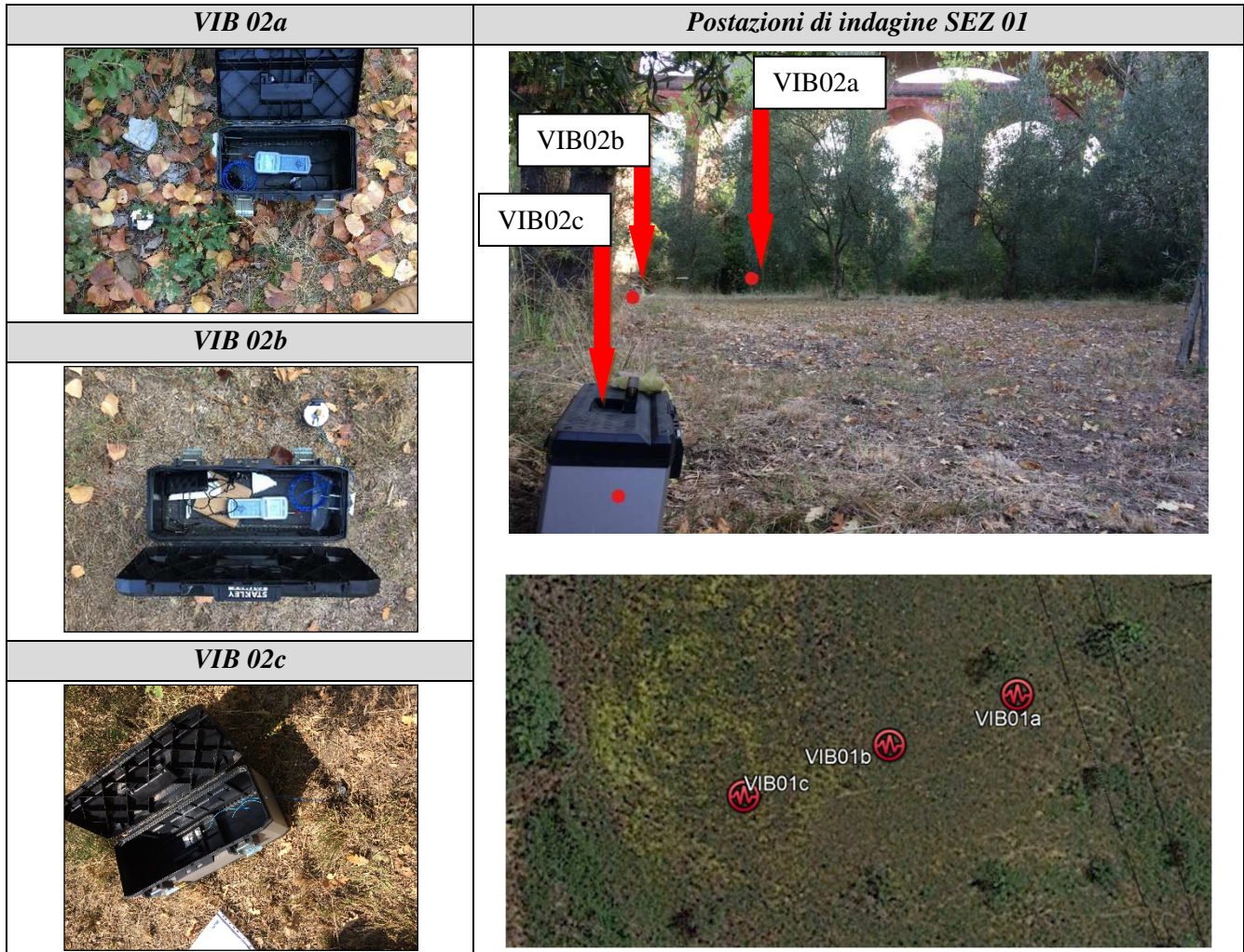
Figura 7 - Report fotografico postazioni di misura (Asse x: parallelo alla linea; Asse Y: ortogonale alla linea; Asse Z verticale)
