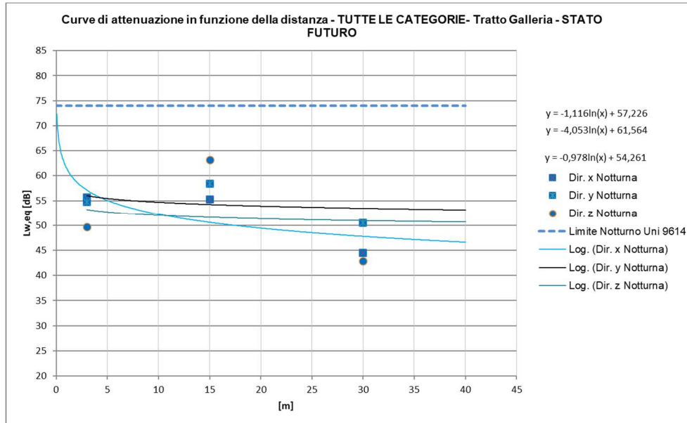
Figura 44 – Curve di attenuazione in funzione della distanza relativa al traffico ferroviario di progetto – tratti al coperto INTERNO AGLI EDIFICI, Treni TUTTE LE CATEGORIE, periodo notturno
