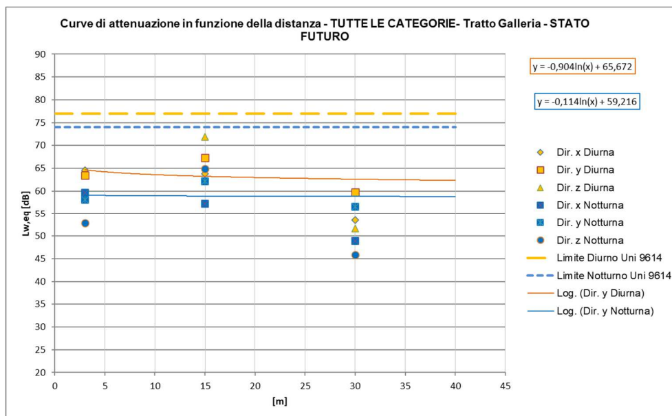
Figura 26 – Curve di attenuazione in funzione della distanza relativa al traffico ferroviario di progetto – tratti al coperto, Treni TUTTE LE CATEGORIE
