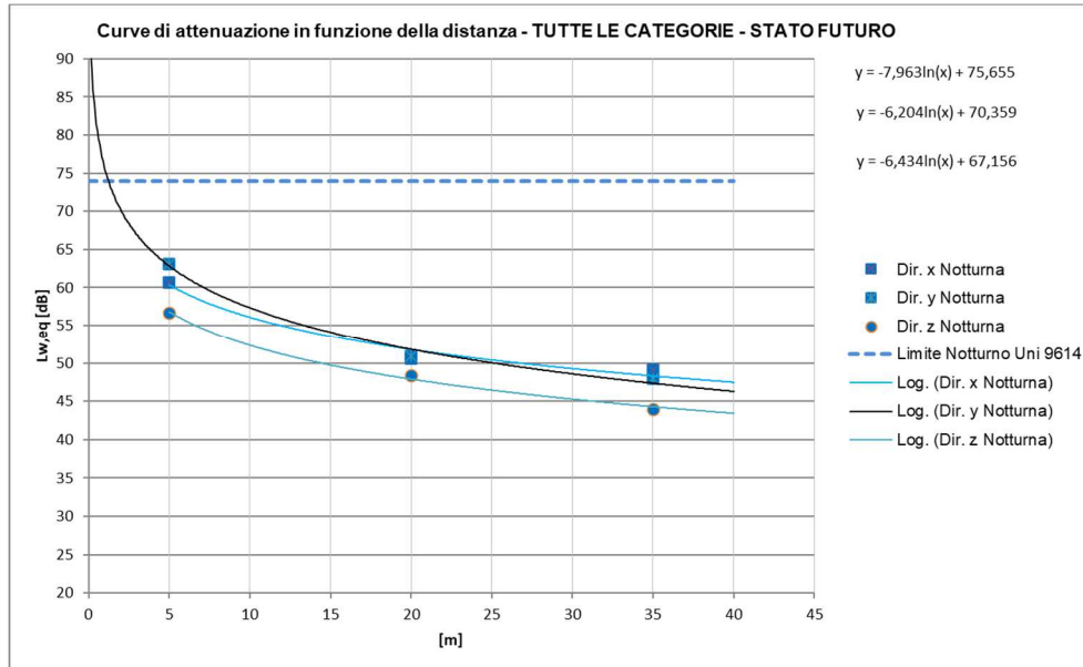
Figura 74 – Curve di attenuazione in funzione della distanza relativa al traffico ferroviario di progetto – tratti allo scoperto INTERNO AGLI EDIFICI, Treni TUTTE LE CATEGORIE, periodo notturno
