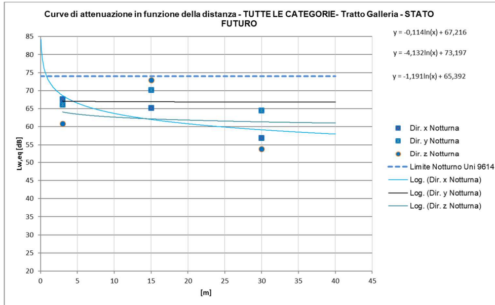
Figura 34 – Curve di attenuazione in funzione della distanza relativa al traffico ferroviario di progetto – tratti al coperto INTERNO AGLI EDIFICI, Treni TUTTE LE CATEGORIE, periodo notturno
