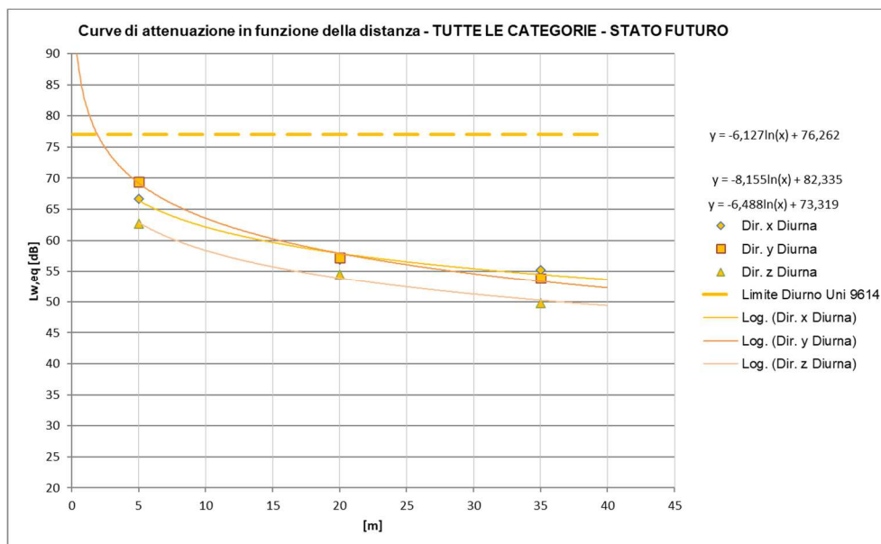
Figura 73 – Curve di attenuazione in funzione della distanza relativa al traffico ferroviario di progetto – tratti allo scoperto INTERNO AGLI EDIFICI, Treni TUTTE LE CATEGORIE, periodo diurno
