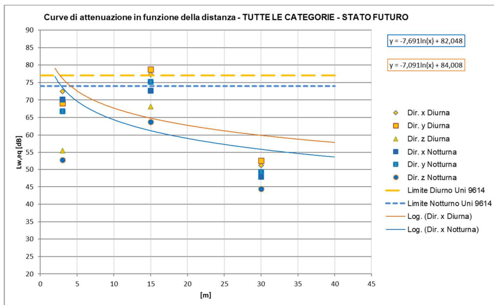
Figura 61 – Curve di attenuazione in funzione della distanza relativa al traffico ferroviario di progetto – tratti allo scoperto, Treni TUTTE LE CATEGORIE
