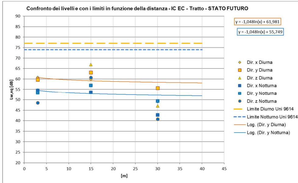
Figura 35 – Curve di attenuazione in funzione della distanza relativa al traffico ferroviario di progetto – tratti al coperto, TRENI IC-EC a 250km/h
