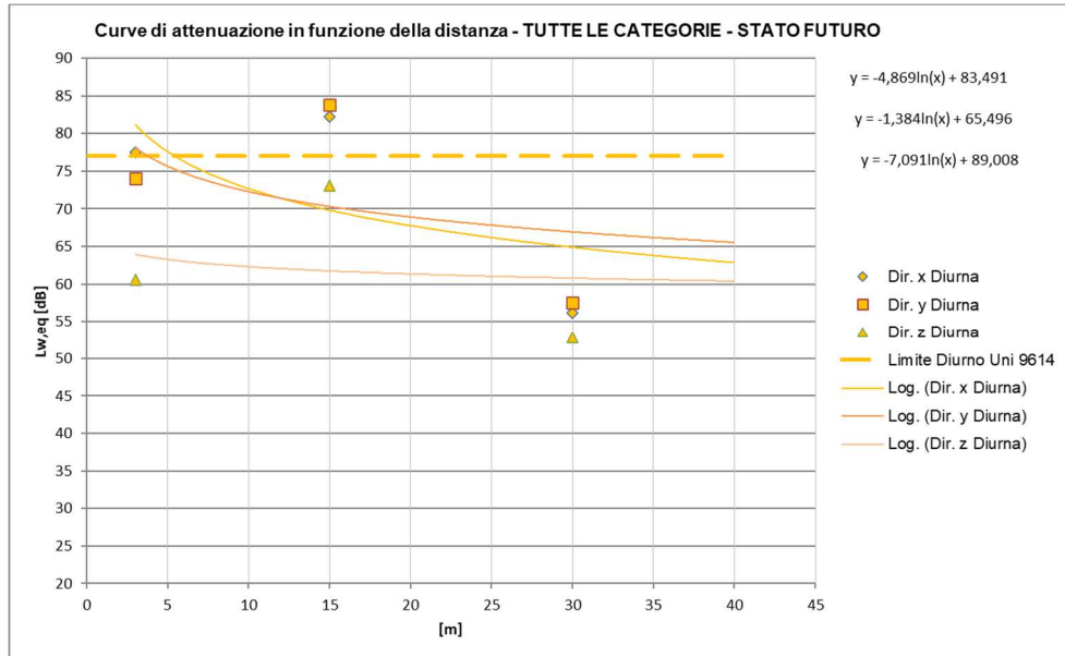
Figura 62 – Curve di attenuazione in funzione della distanza relativa al traffico ferroviario di progetto – tratti allo scoperto INTERNO AGLI EDIFICI, Treni TUTTE LE CATEGORIE, periodo diurno
