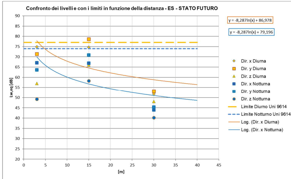
Figura 48 – Curve di attenuazione in funzione della distanza relativa al traffico ferroviario di progetto – tratti allo scoperto, TRENI ES a 300km/h
