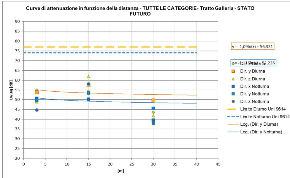
Figura 42 – Curve di attenuazione in funzione della distanza relativa al traffico ferroviario di progetto – tratti al coperto, Treni TUTTE LE CATEGORIE
