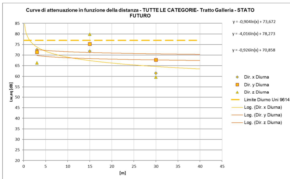
Figura 33 – Curve di attenuazione in funzione della distanza relativa al traffico ferroviario di progetto – tratti al coperto INTERNO AGLI EDIFICI, Treni TUTTE LE CATEGORIE, periodo diurno
