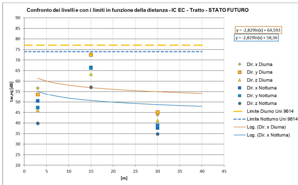
Figura 47 – Curve di attenuazione in funzione della distanza relativa al traffico ferroviario di progetto – tratti allo scoperto, TRENI IC-EC a 250km/h
