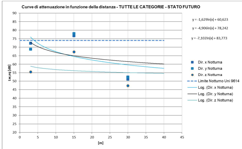
Figura 52 – Curve di attenuazione in funzione della distanza relativa al traffico ferroviario di progetto – tratti allo scoperto INTERNO AGLI EDIFICI, Treni TUTTE LE CATEGORIE, periodo notturno
