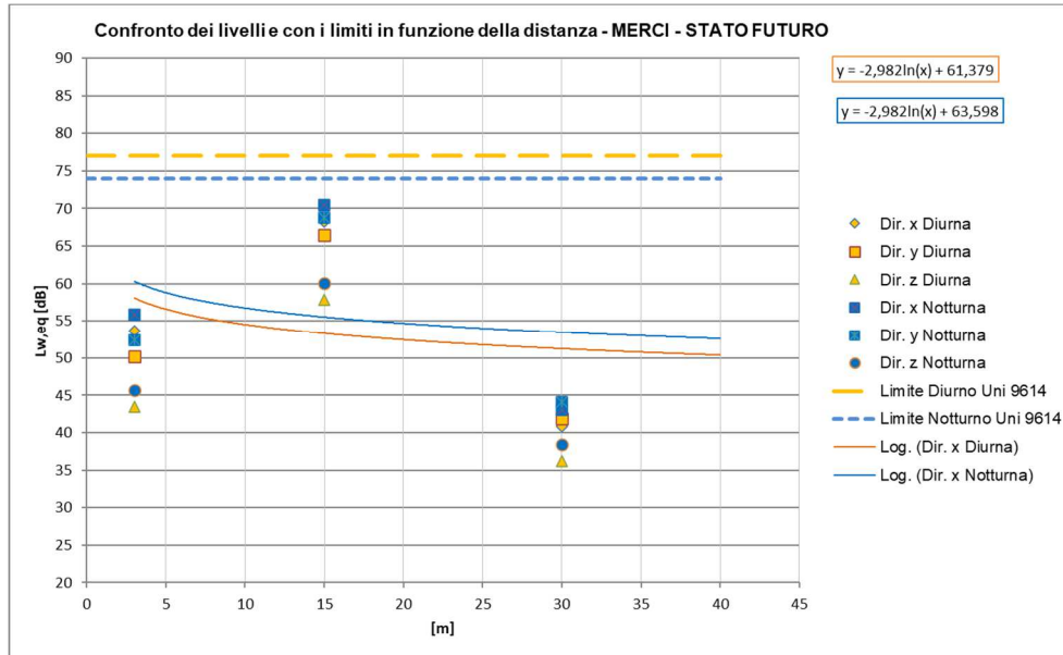
Figura 55 – Curve di attenuazione in funzione della distanza relativa al traffico ferroviario di progetto – tratti allo scoperto, TRENI MERCI a 100km/h
