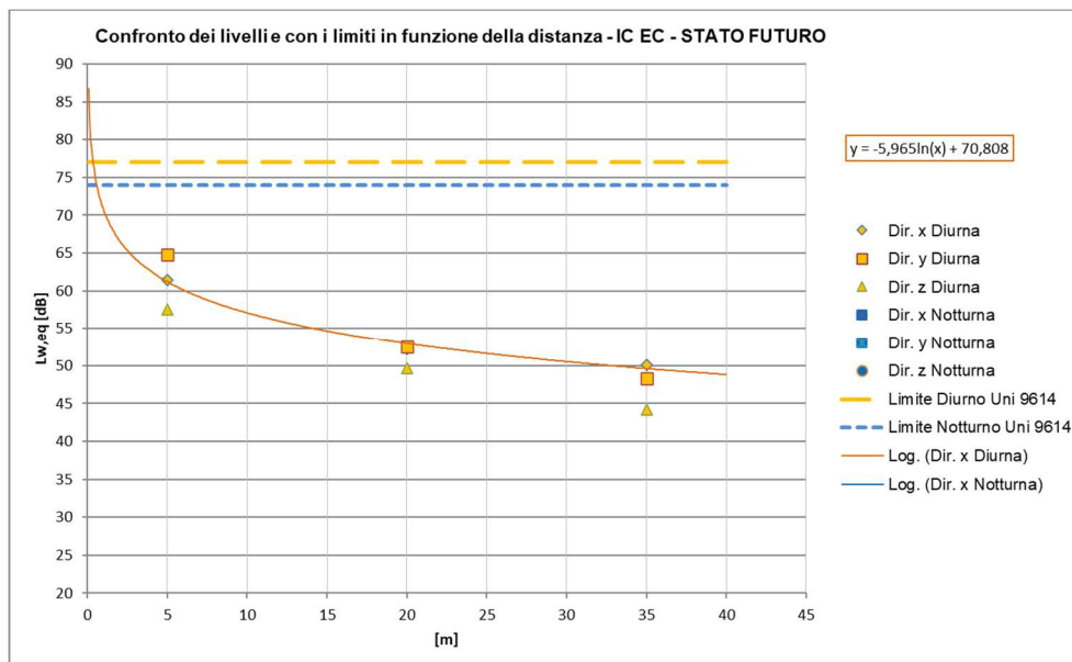
Figura 76 – Curve di attenuazione in funzione della distanza relativa al traffico ferroviario di progetto – tratti allo scoperto, TRENI IC-EC a 100 km/h
