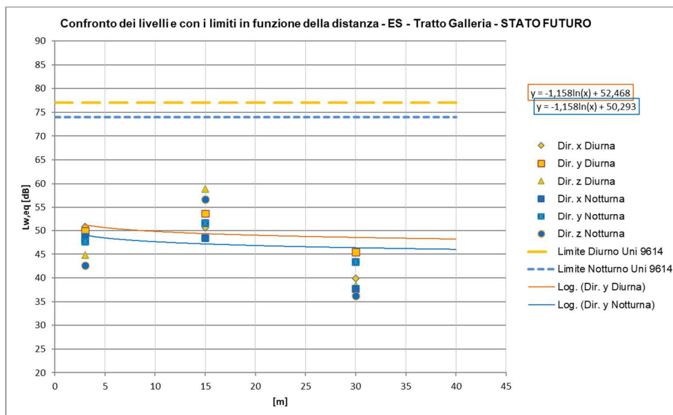
Figura 41 – Curve di attenuazione in funzione della distanza relativa al traffico ferroviario di progetto – tratti al coperto, TRENI ES a 100km/h
