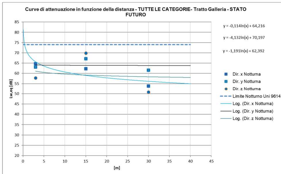
Figura 28 – Curve di attenuazione in funzione della distanza relativa al traffico ferroviario di progetto – tratti al coperto INTERNO AGLI EDIFICI, Treni TUTTE LE CATEGORIE, periodo notturno
