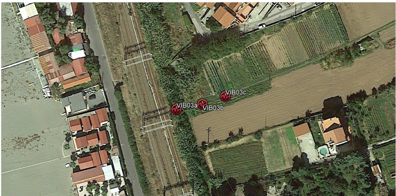
Figura 8 - Ortofoto area di indagine e postazioni di misura SEZ.3
