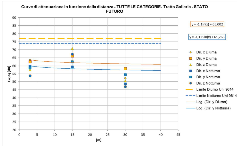
Figura 37 – Curve di attenuazione in funzione della distanza relativa al traffico ferroviario di progetto – tratti al coperto, Treni TUTTE LE CATEGORIE
