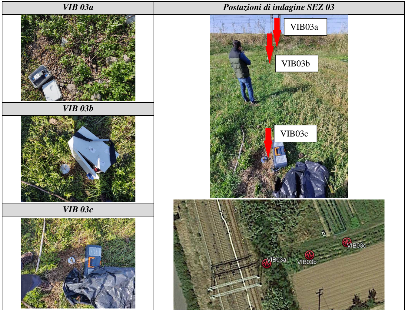
Figura 9 - Report fotografico postazioni di misura (Asse x: parallelo alla linea; Asse Y: ortogonale alla linea; Asse Z verticale)
