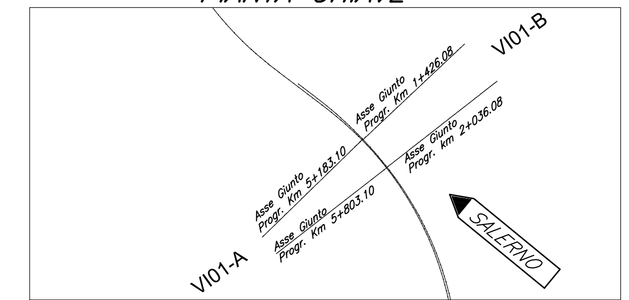
PIANTA CHIAVE
