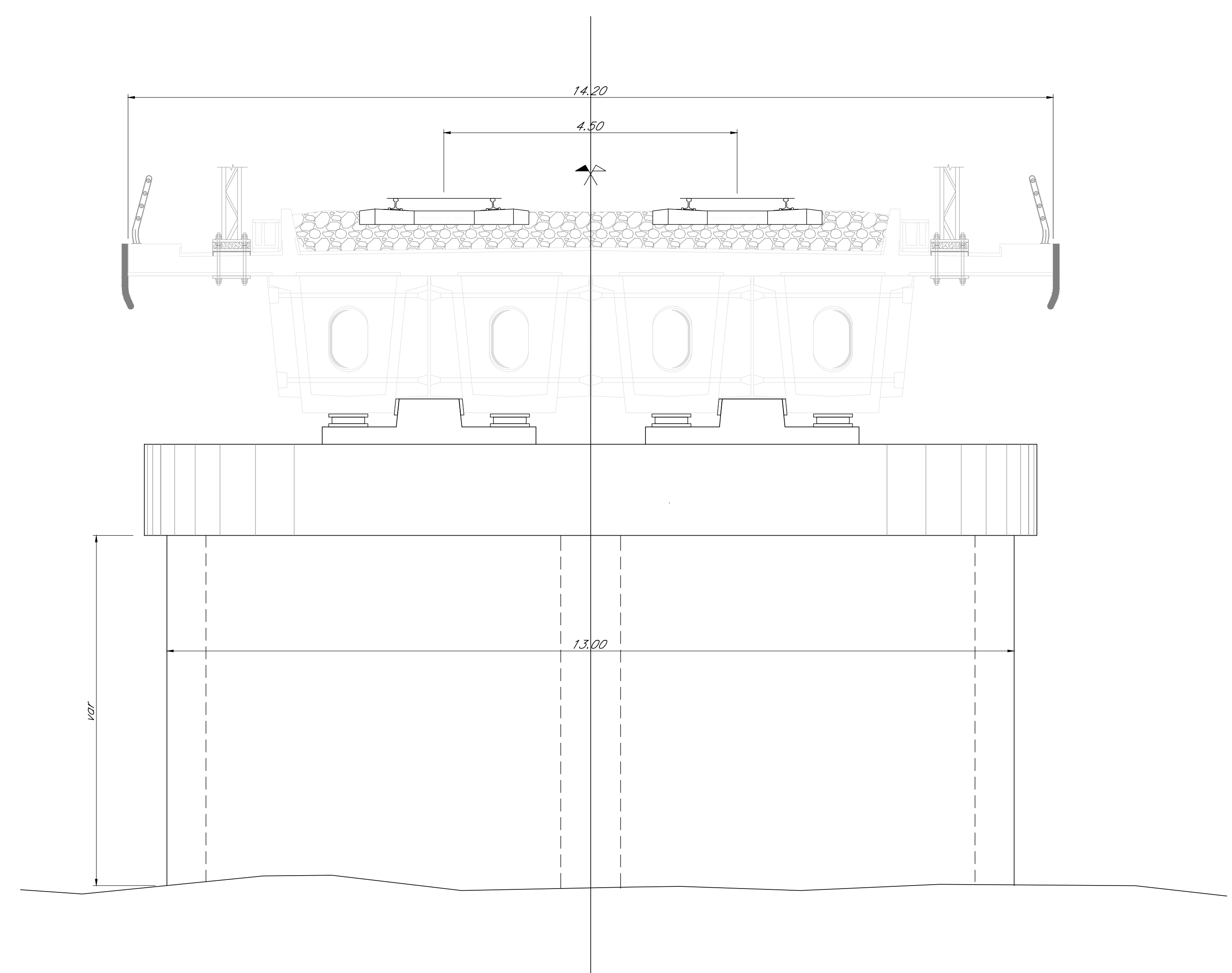
SEZIONE TRASVERSALE PILA CAMPATA L=25.00m Scala 1:50
