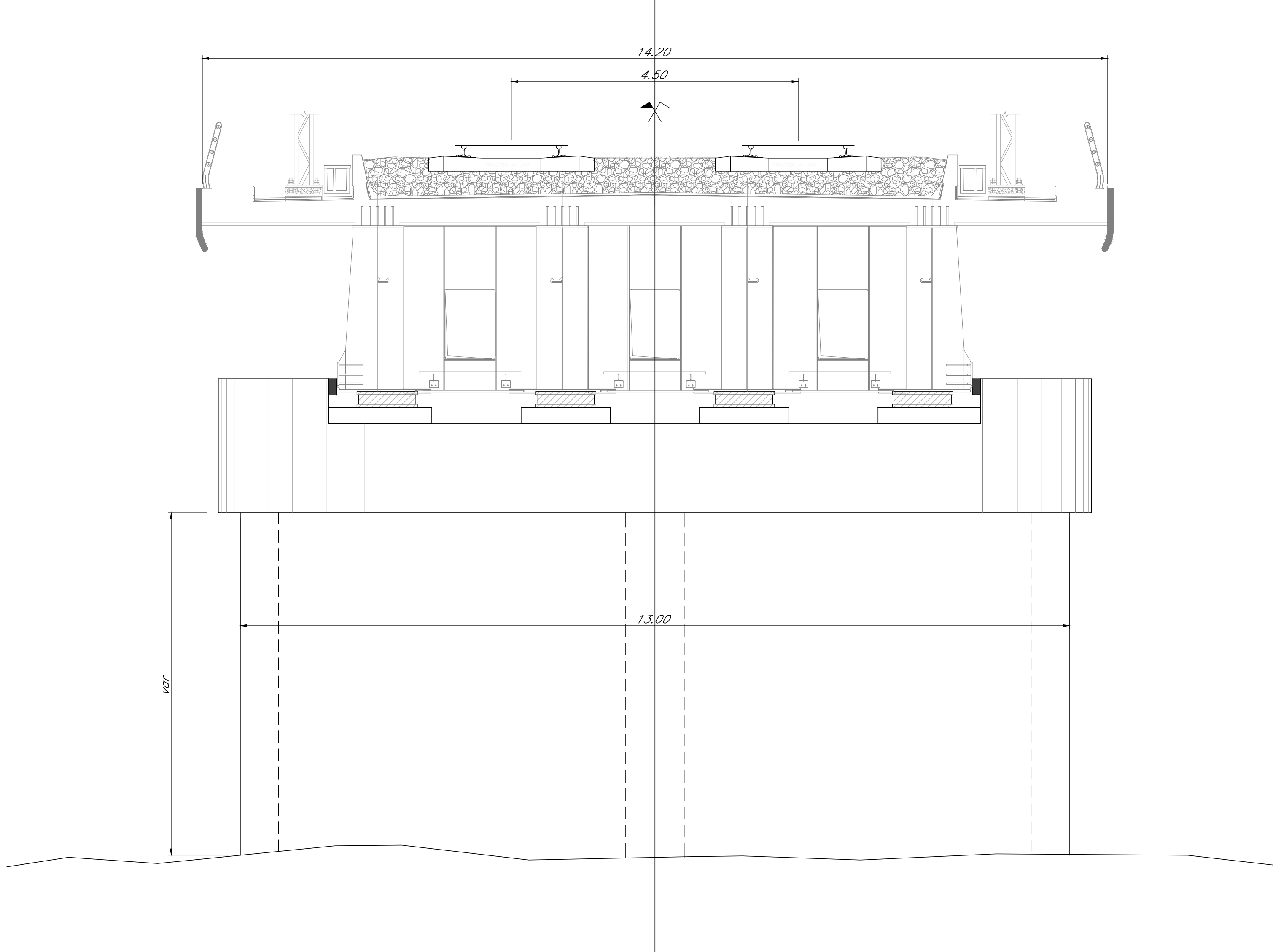
SEZIONE TRASVERSALE PILA CAMPATA L=40.00m Scala 1:50
