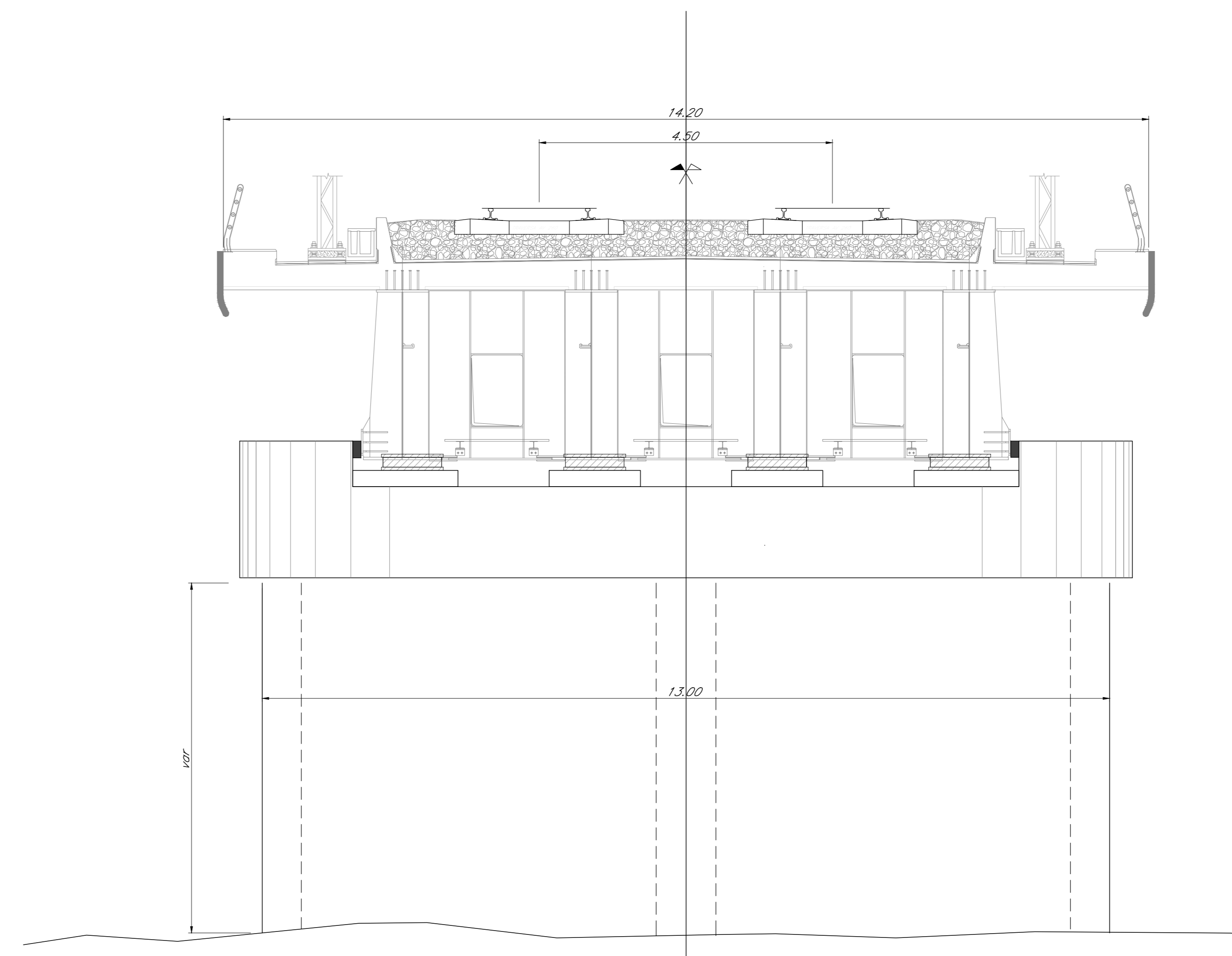
SEZIONE TRASVERSALE PILA CAMPATA L=40.00m Scala 1:50
