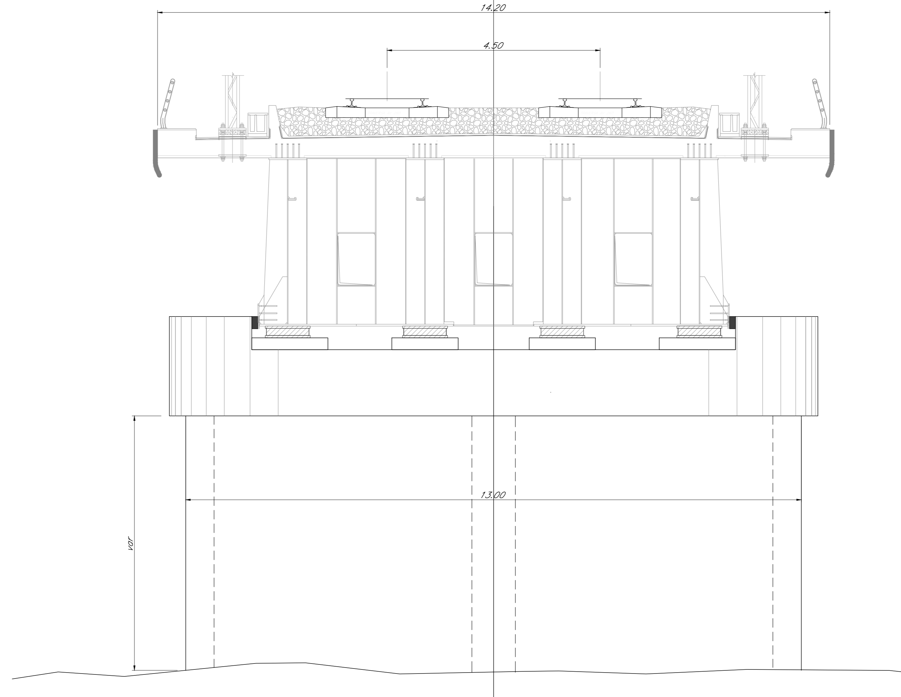
SEZIONE TRASVERSALE PILA CAMPATA L=50.00m Scala 1:50
