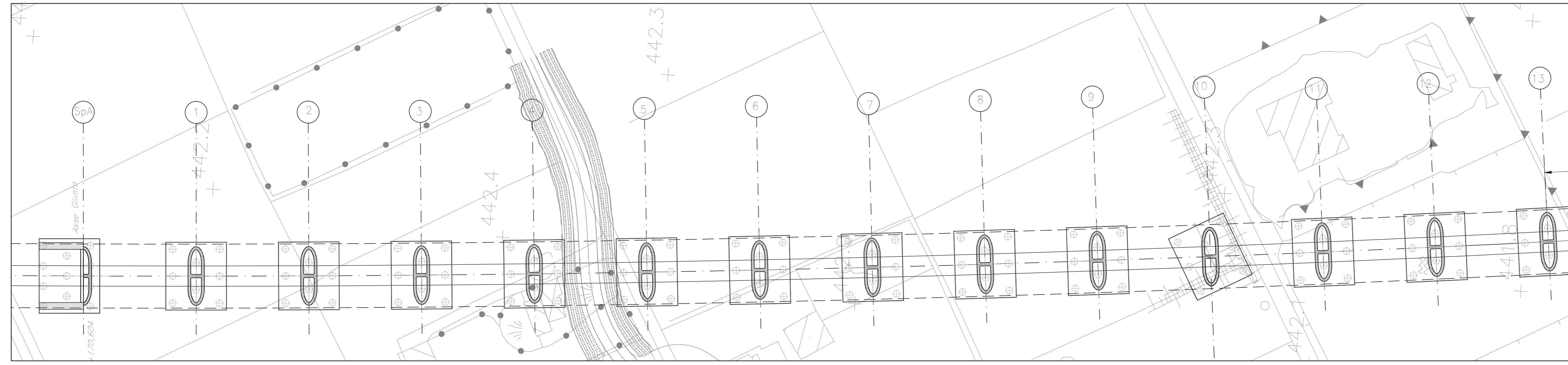
PIANTA FONDAZIONI Scale 1:500
