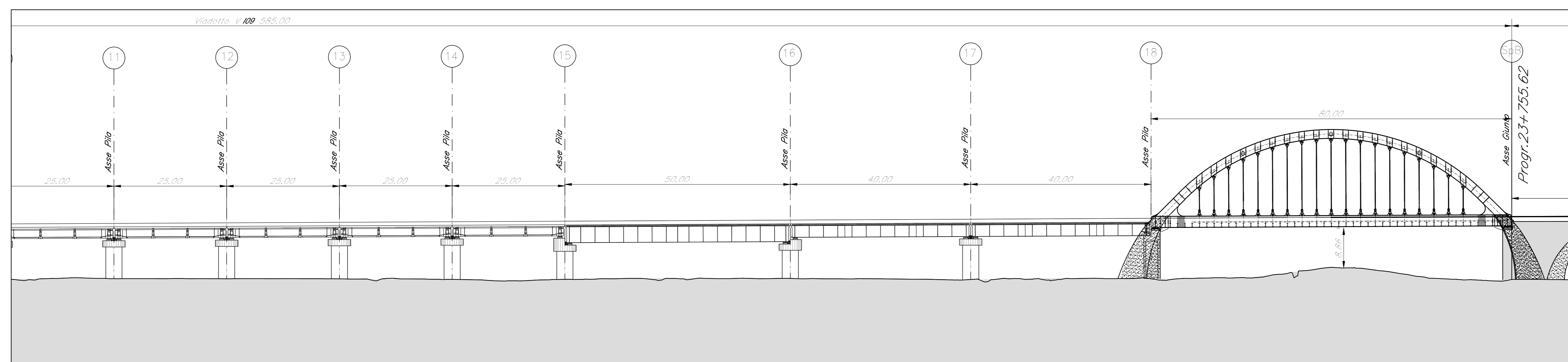
PROSPETTO Scale 1:500
