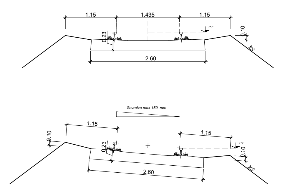
Dettaglio 1 - Andamento traversa in rettilo ed in curva SCALA 1:50
