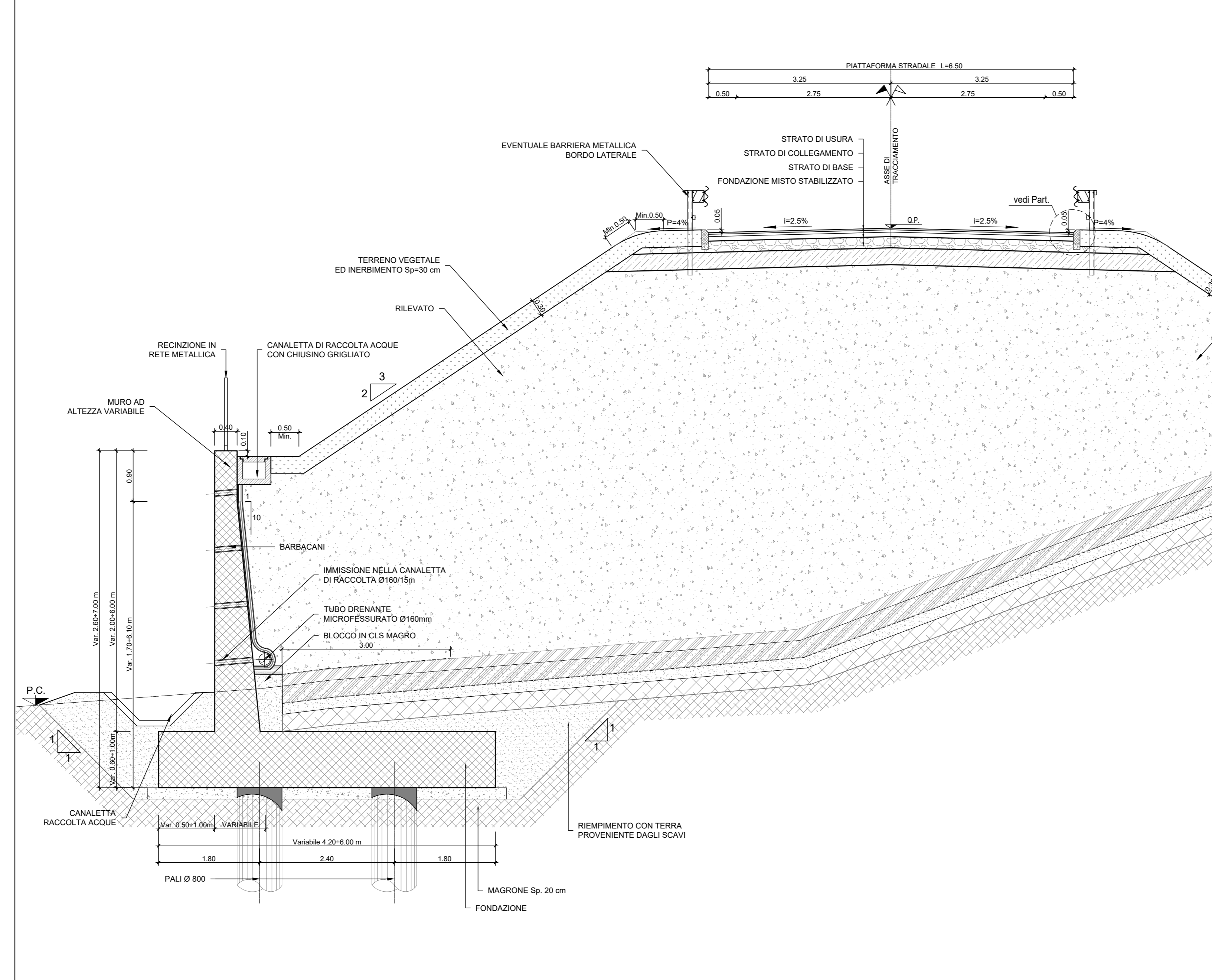
NV02 SEZIONE TIPO IN RILEVATO CON MURO DI SOTTOSCARPA (TIPO S-1) SCALA 1:50
