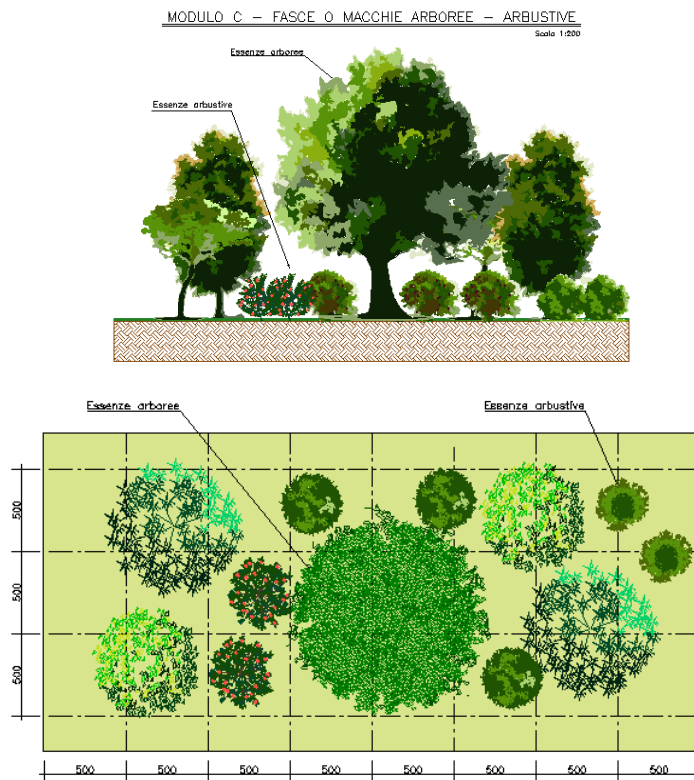
Figura 4-3 – MODULO C – Fasce o macchie arboreo-arbustive: sesto d'impianto e sezione tipologica
