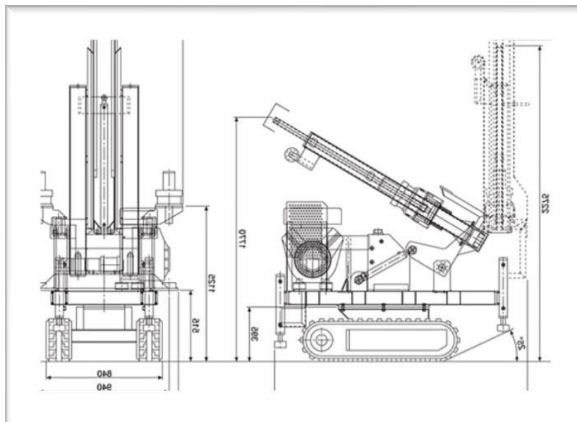
Figura 29. Tipologico del carotiere meccanico.
