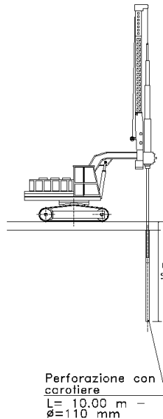
Figura 9. Carotaggi archeologici-Layout.
