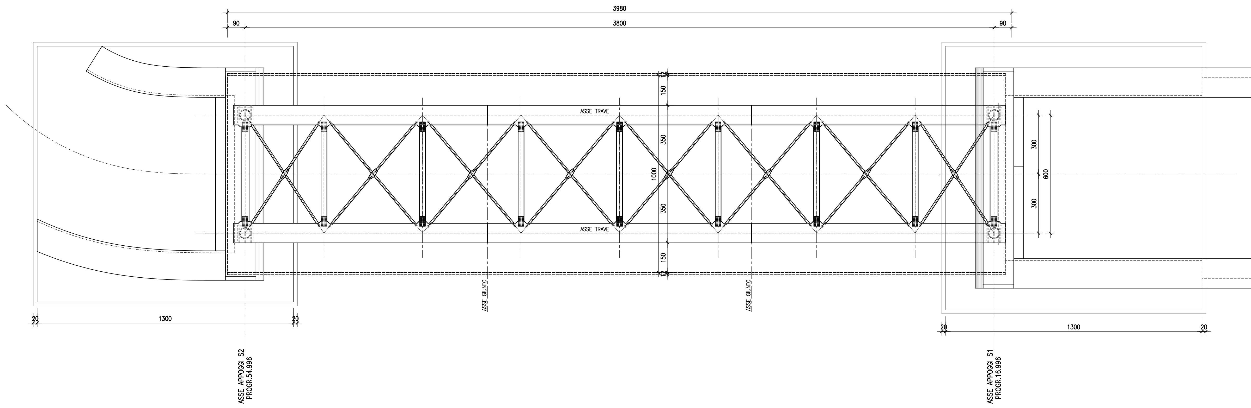
PIANTA IMPALCATO—Scala 1:100
