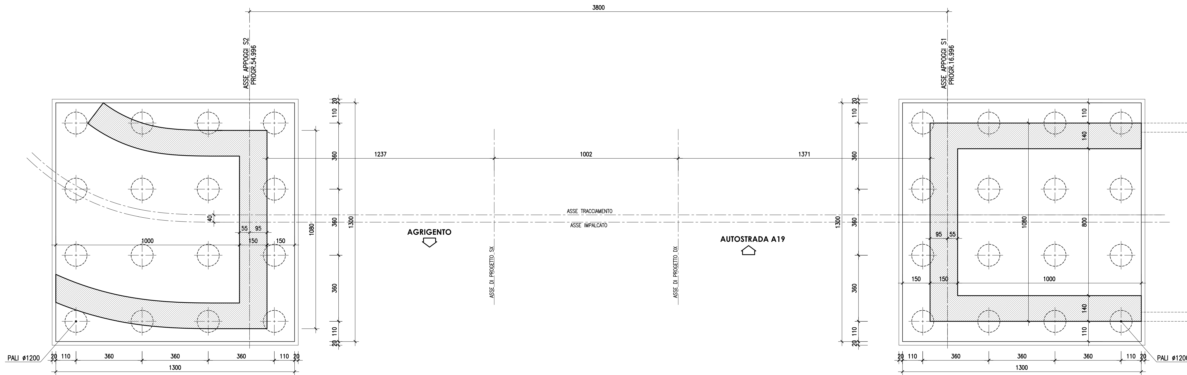
PIANTA FONDAZIONI—Scala 1:100
