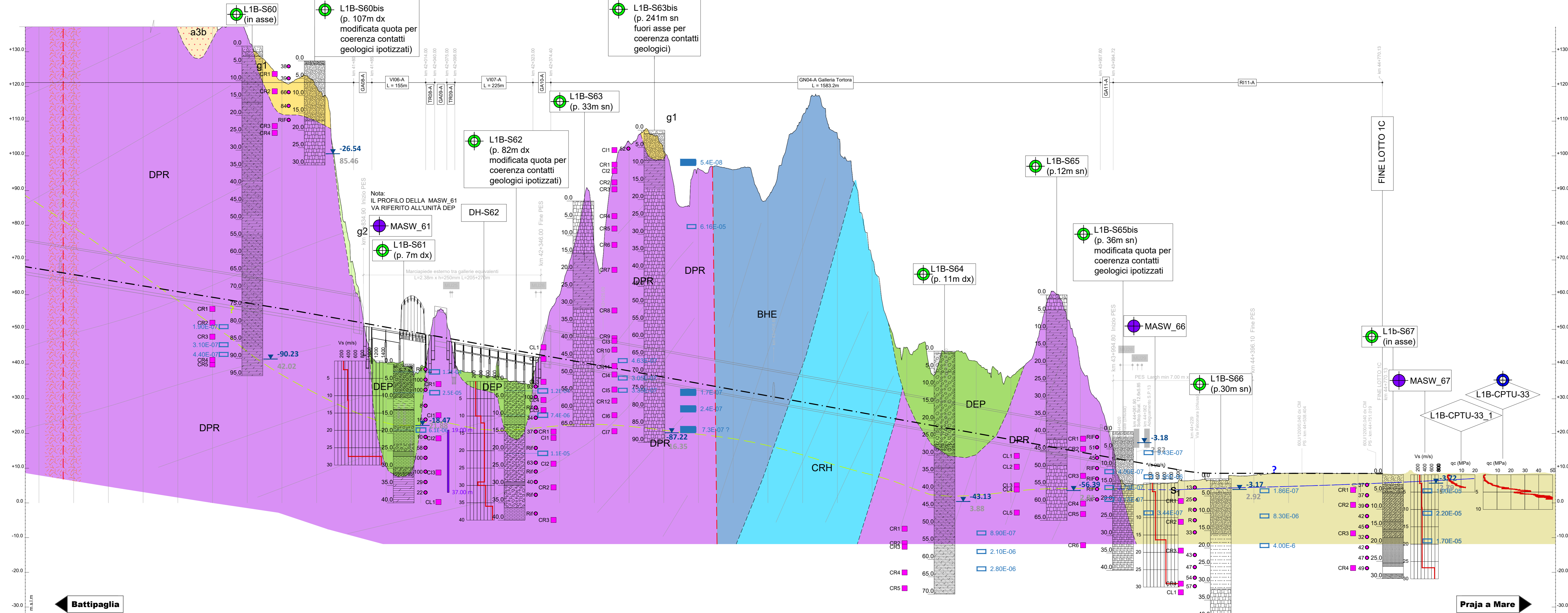
PROFILO ASSE BINARIO PARI SCALA H=1/5000 V=1/500
