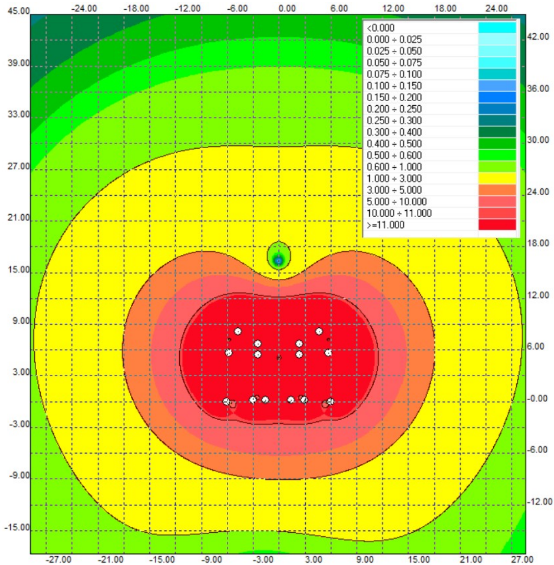
Figura 4: Figura 4: Mappa cromatica campi magnetici sezione tipologica linea 2x25 kV
