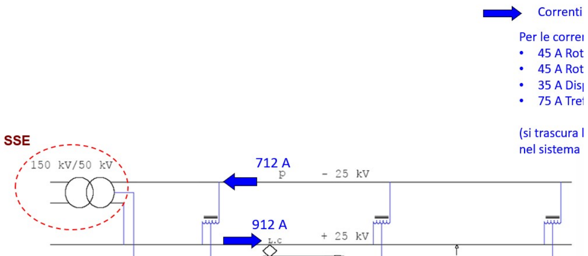
Figura 3: Correnti complessive sistema 2x25 kV
