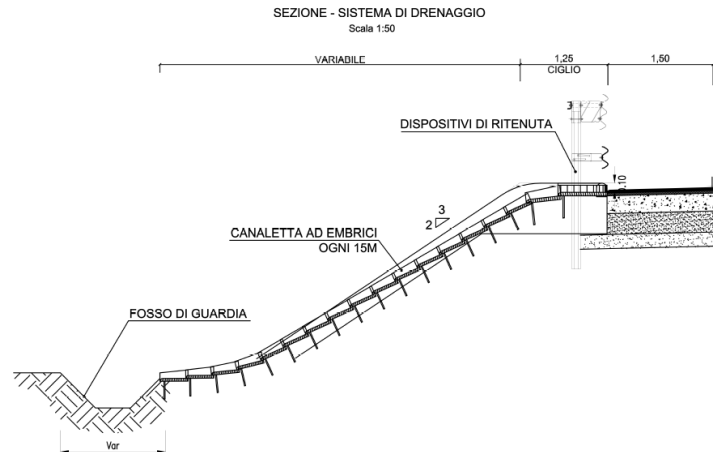
Figura 4-15 Tratto in rettilo - drenaggio con embrici
