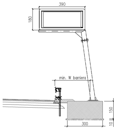
Figura 4-12 Portale a messaggio variabile
