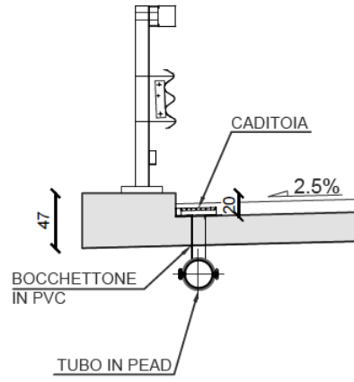
Figura 4-19 Tratti in viadotto - drenaggio con caditoia
