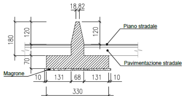
Figura 4-7 Opera a protezione della pila a "Setto" – sezione trasversale
