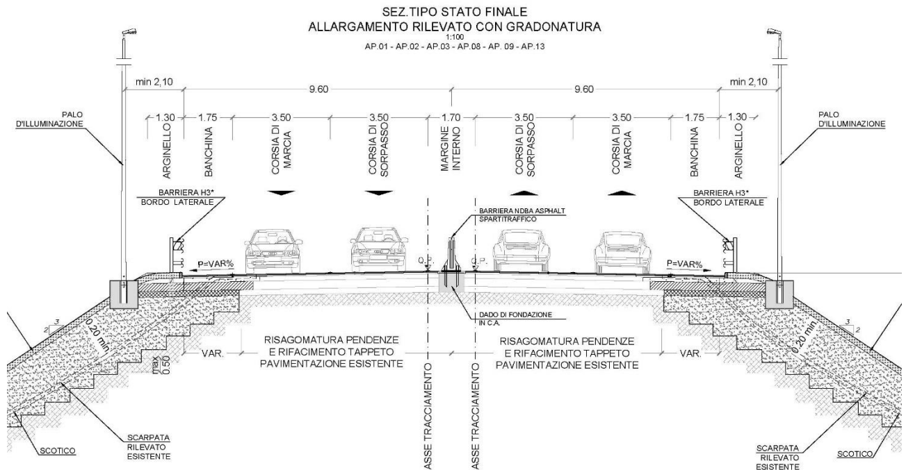
Figura 4-1 Sezione tipo per l'intervento di riquilifica
