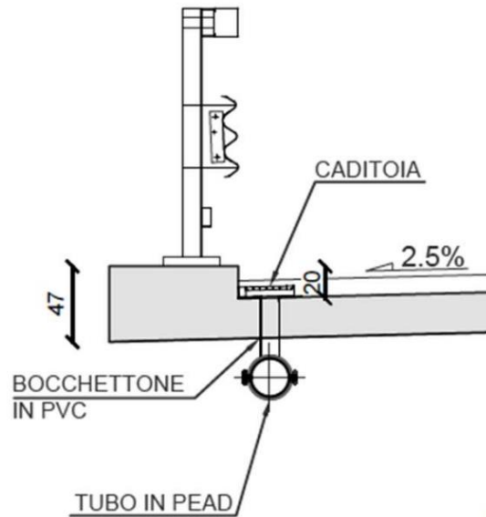
Figura 5-8 Tratti in viadotto – drenaggio con caditoia
