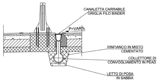
Figura 4-16 Tratti in curva - drenaggio con canaletta continua della carreggiata esterna
