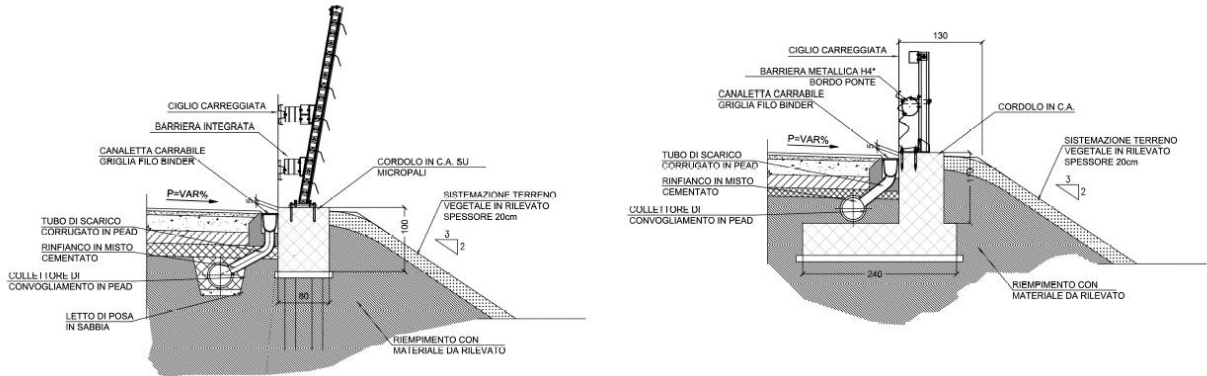
Figura 4-18 Tratti con barriera integrata – drenaggio con canaletta continua
