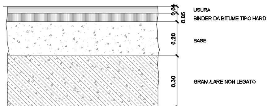
Figura 4-14 Sezione tipo della pavimentazione per l'intervento di riqualifica
