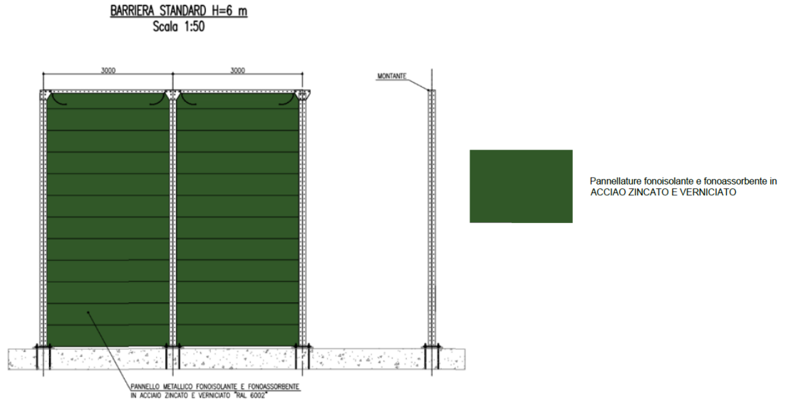
Figura 6-6 Tipologico barriera standard
