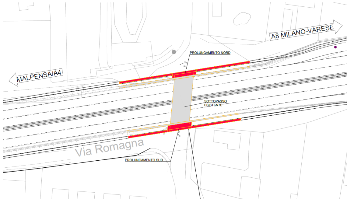
Figura 4-5 Stralcio planimetrico sottopasso via Correnti
