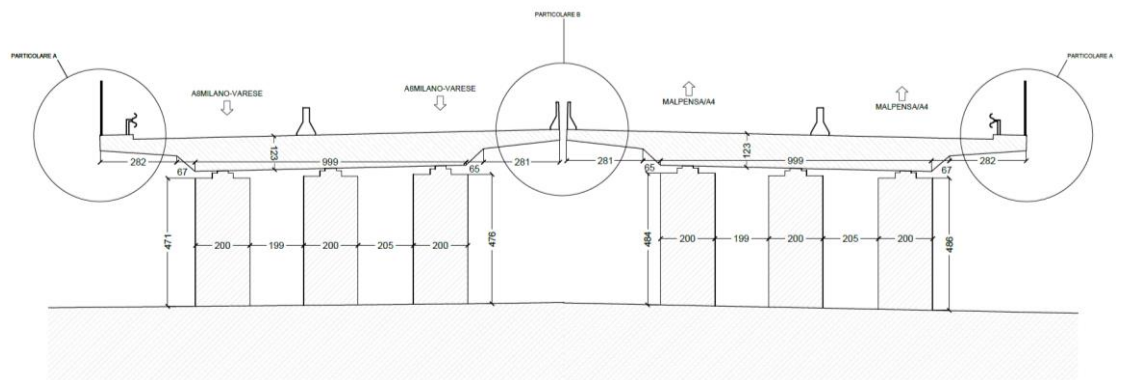
Figura 4-2 Viadotto su SP 20 Busto - individuazione sbalzi oggetto di riqualifica
