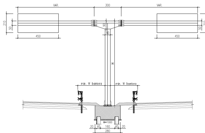
Figura 4-11 Portale a farfalla
