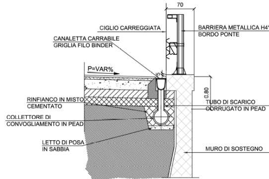
Figura 4-17 Tratti con muri laterali di sostegno – drenaggio con canaletta continua
