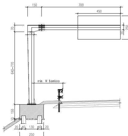
Figura 4-10 Portale a bandiera
