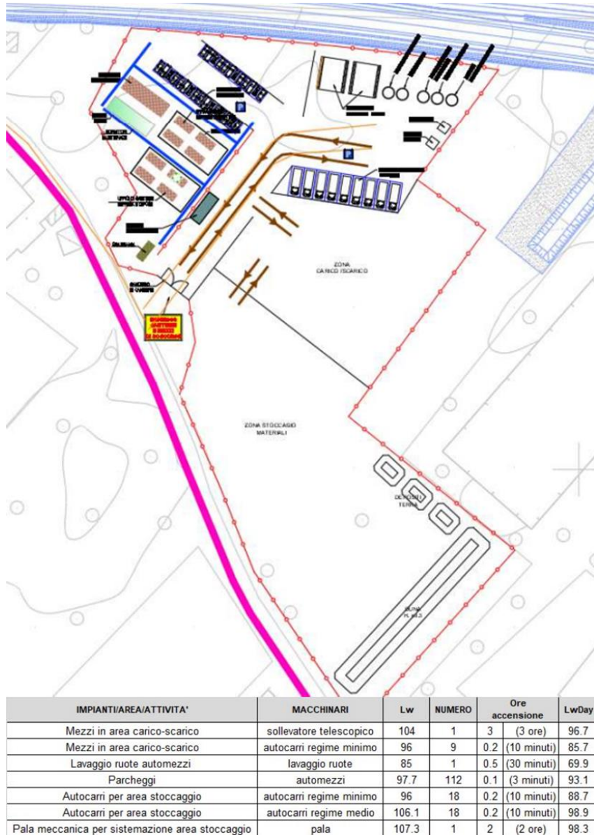
Figura 5-1 CO01: Layout di cantiere e sorgenti
