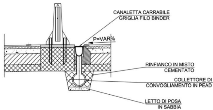
Figura 5-5 Tratti in curva - drenaggio con canaletta continua della carreggiata esterna
