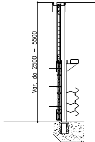
Figura 6-2 Sezione tipologica barriera integrata
