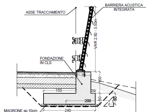
Figura 4-6 Opera di sostegno tipo
