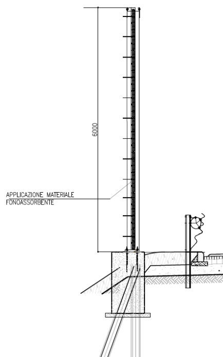
Figura 6-1 Sezione tipologico barriera standard
