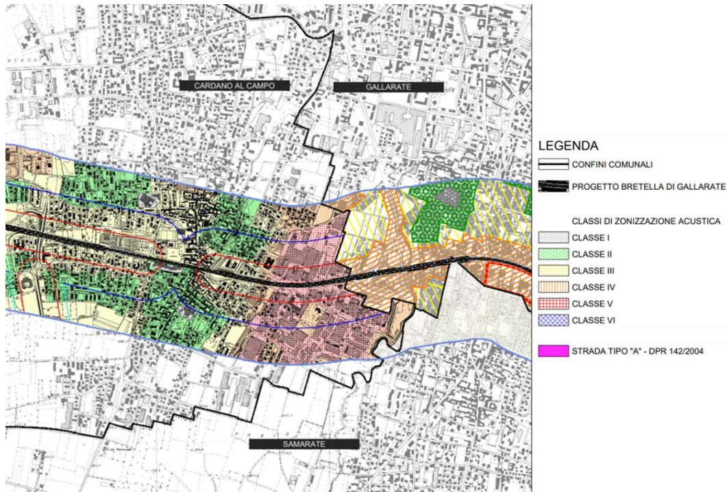
Figura 2-53 Classificazione acustica dell'area d'intervento
