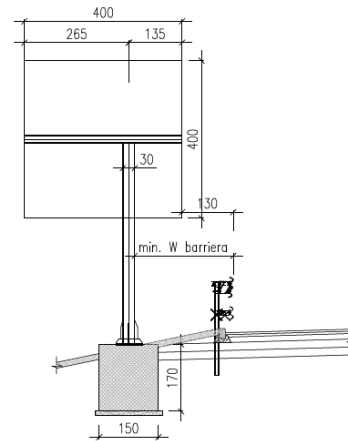
Figura 4-13 Monopalo della segnaletica
