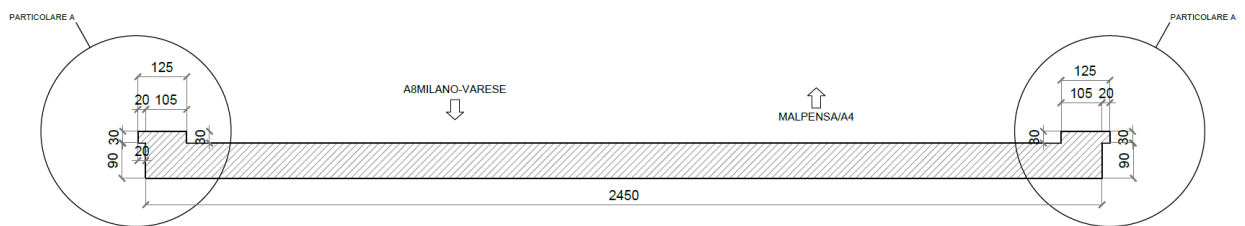
Figura 4-4 Ponte rampa su svincolo Cardano e sovrappasso su SP 15 - individuazione sbalzi oggetti di riqualifica
