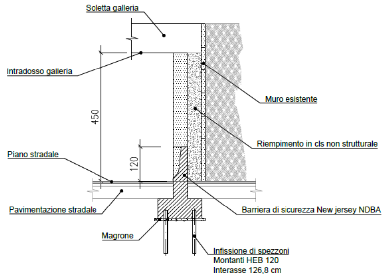
Figura 4-9 Opera a protezione dell'imbocco della galleria – sezione trasversale
