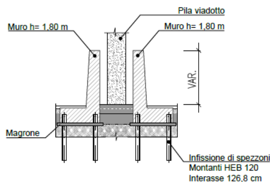
Figura 4-8 Opera a protezione della pila a "Pilastri" – sezione trasversale
