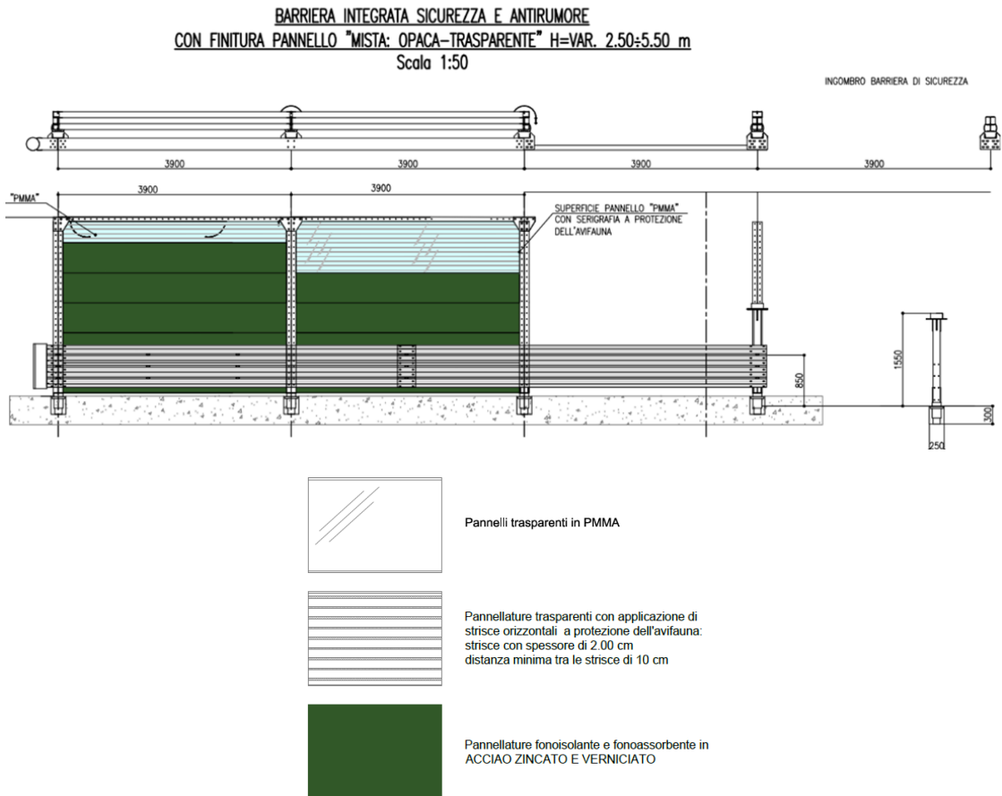
Figura 6-7 Tipologico barriera integrata con finitura pannello "mista: opaca-trasparente"
