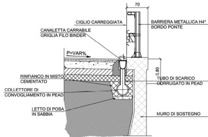
Figura 5-6 Tratti con muri laterali di sostegno – drenaggio con canaletta continua
