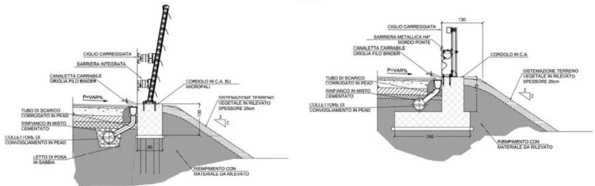
Figura 5-7 Tratti con barriera integrata – drenaggio con canaletta continua
