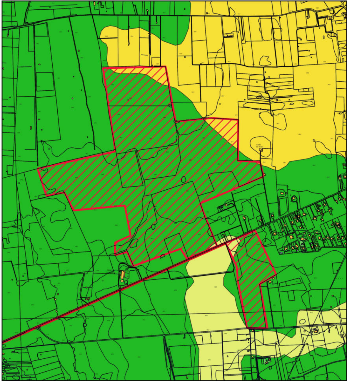
Carta Litologica
