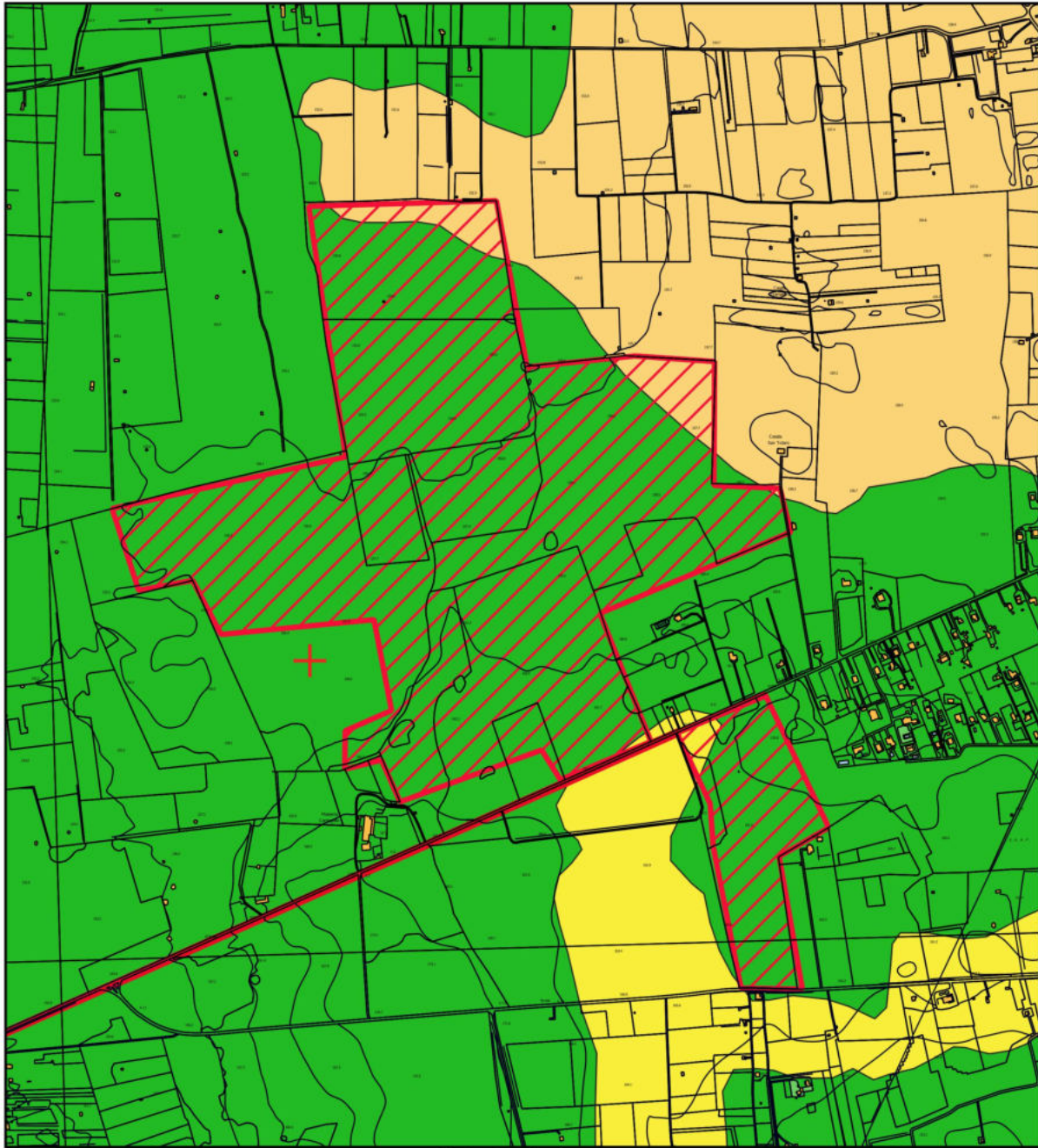
Carta Geologica
