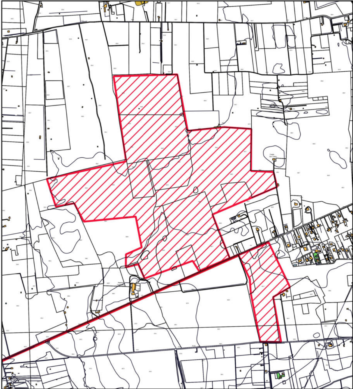
Carta Geomorfologica
