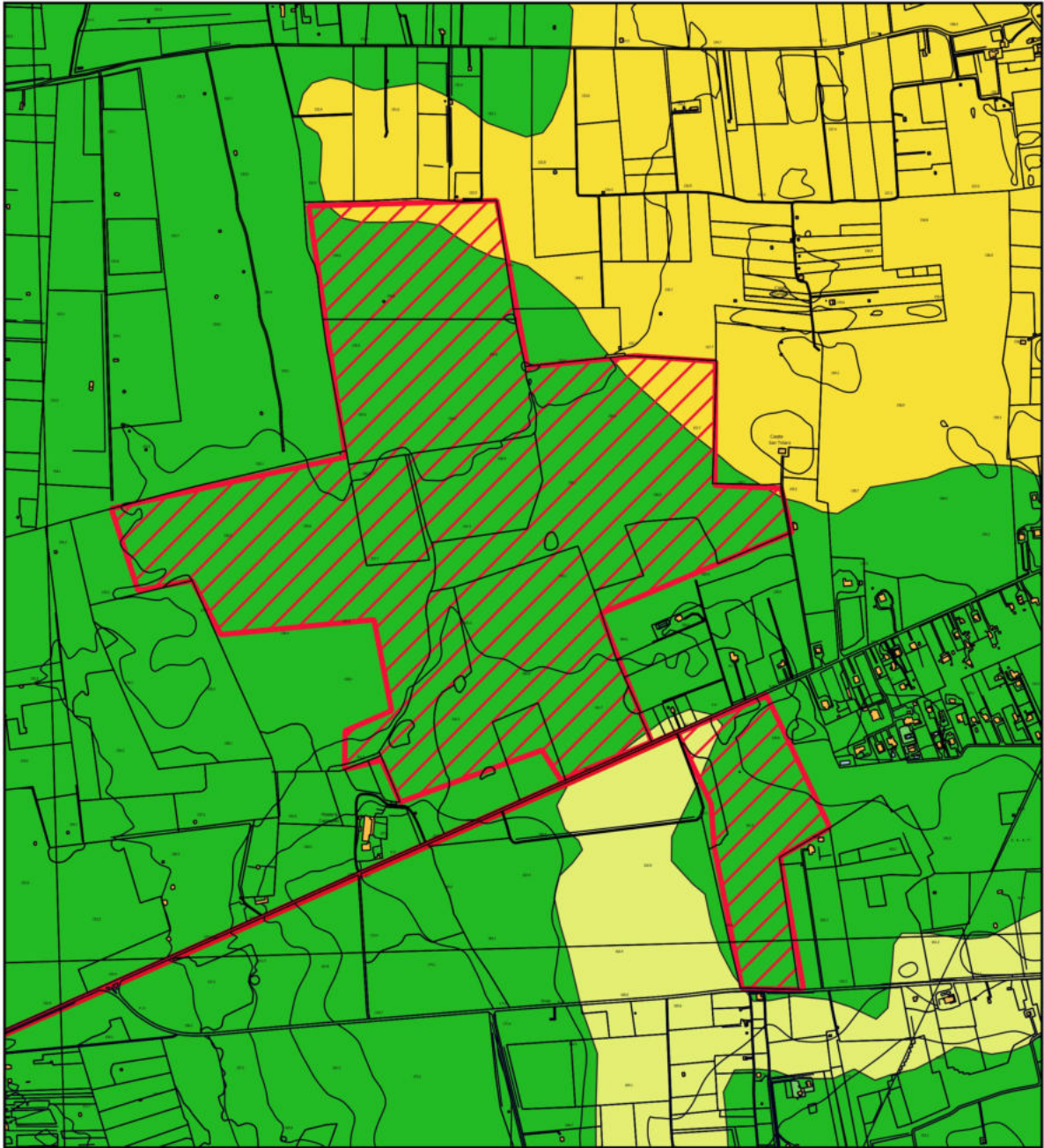
Carta Litologica
