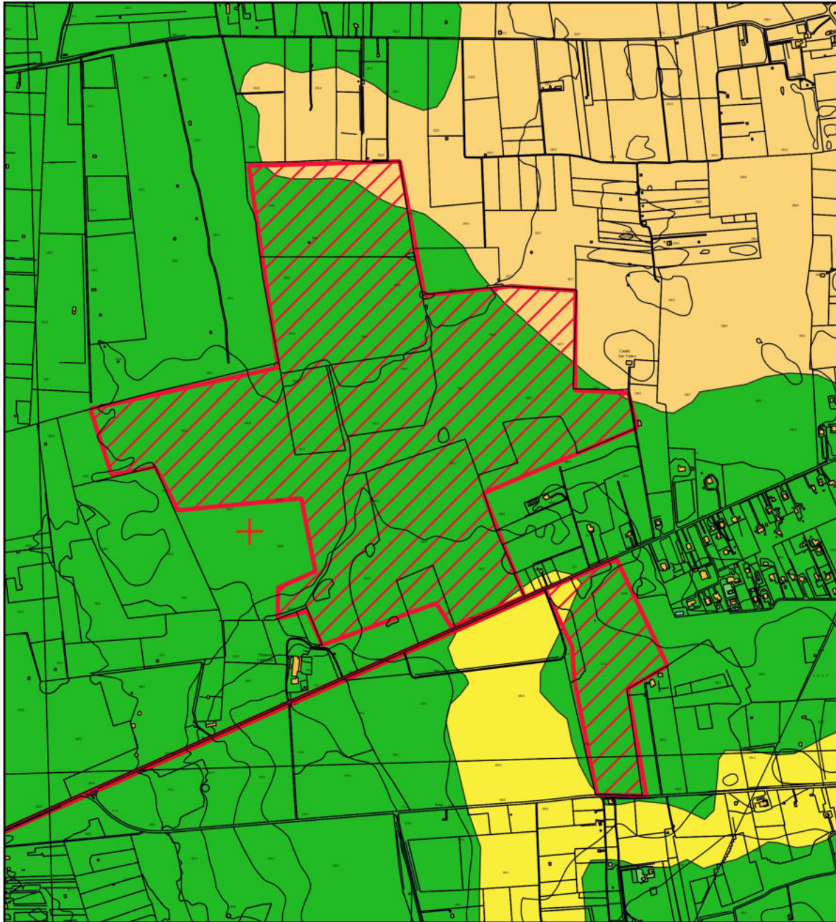
Carta Geologica
